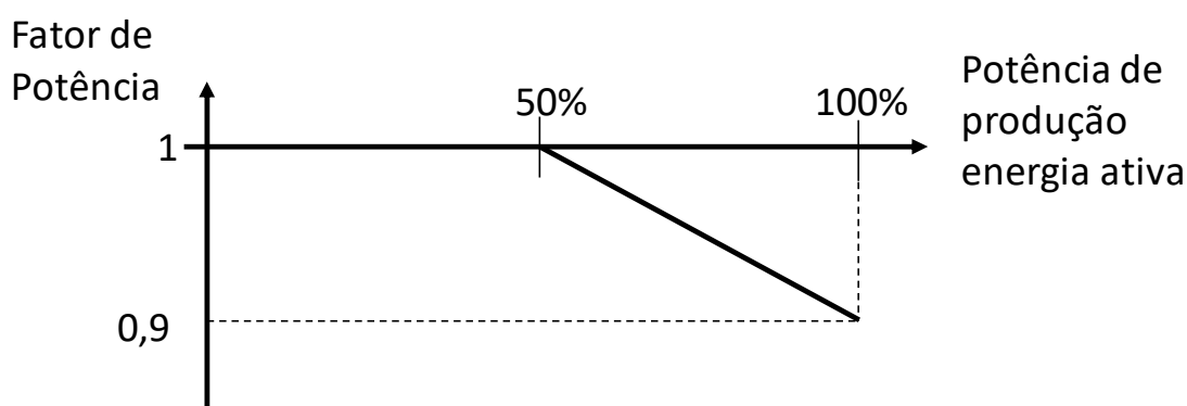
Figura 3 – Curva de operação de contribuição de reativos para inversores com potência nominal P > 6\text{kW}
