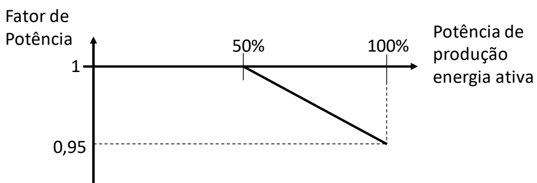
Figura 2 – Curva de operação de contribuição de reativos para inversores com potência nominal de 3\text{kW} < P \leq 6\text{kW}
