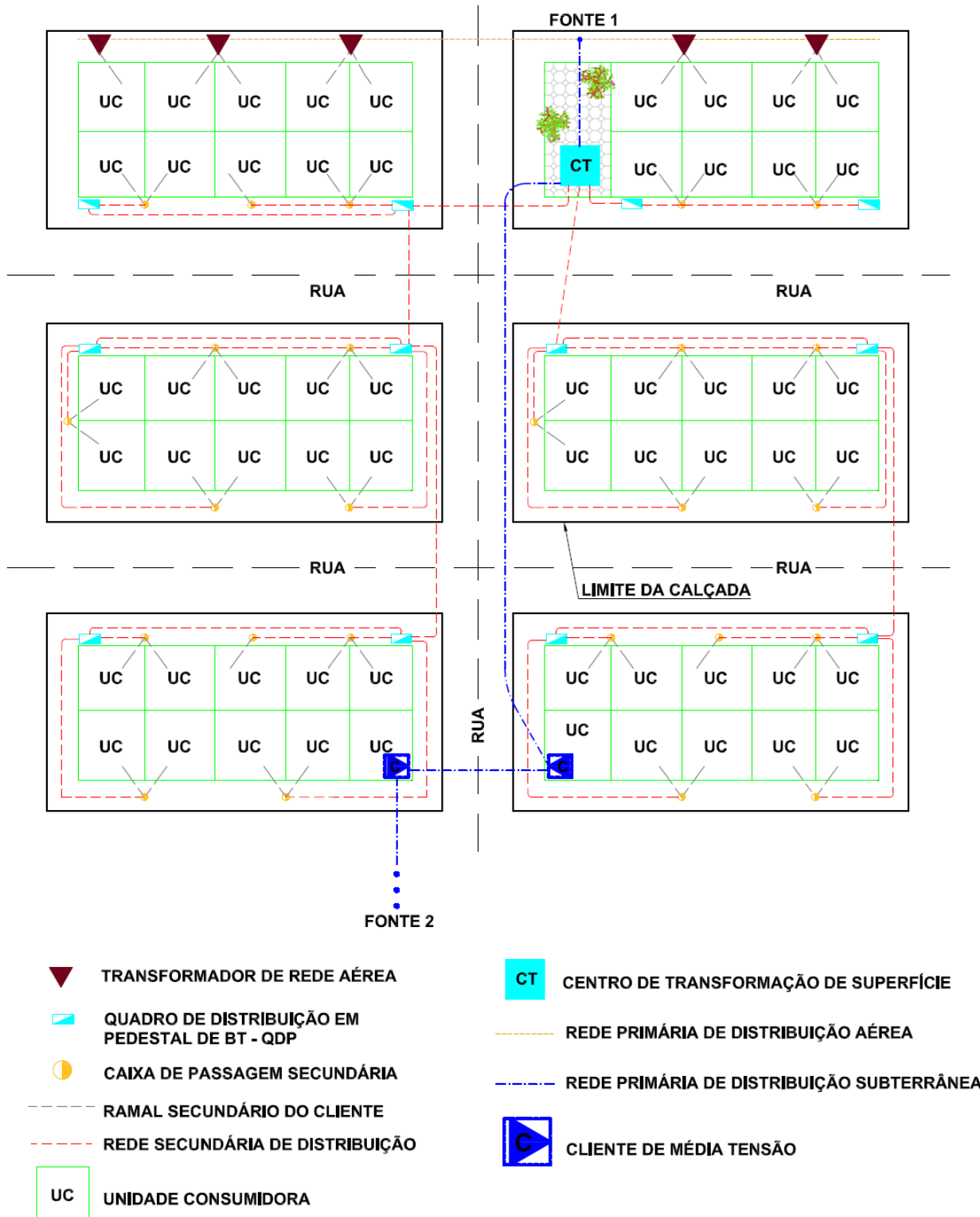
Figura 15 - Conversão Rede Aérea de Baixa Tensão para Rede Subterrânea
