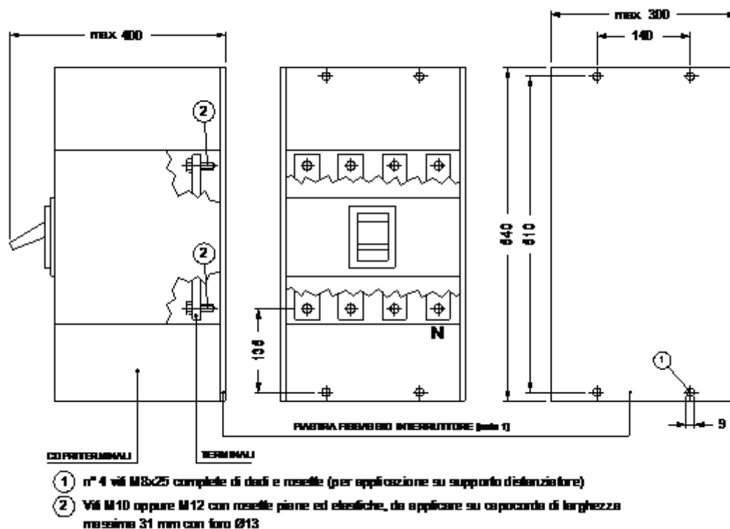
Figura 5 - INTERRUTTORE TIPO DY3103/3-4
