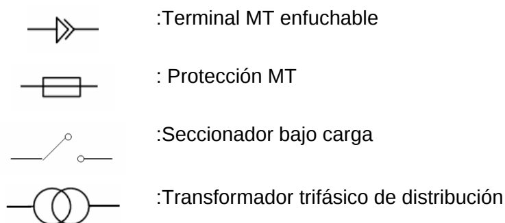
Figura 3: Configuración MT, disposición de elementos
