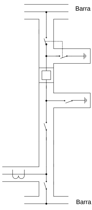
Celda Transformador
