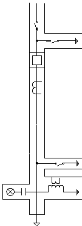
Celda Transformador
