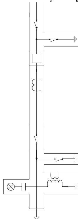
Celda salida de línea y/o acoplamiento
