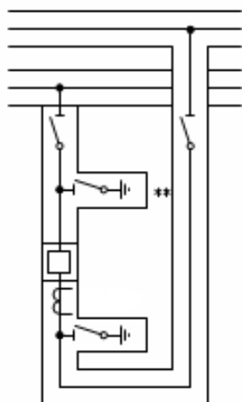
Celda de Acoplamiento
