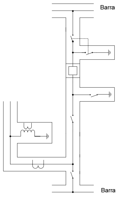
Celda Salida de Línea
