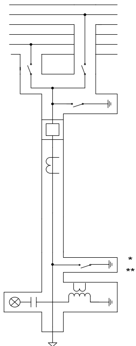
Celda Transformador
