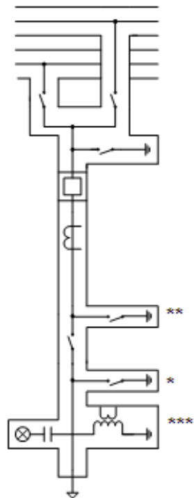
Celda Salida de Línea
