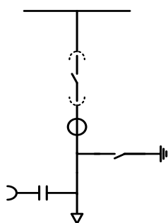
Fig.3: Celda de Salida o SS/AA
