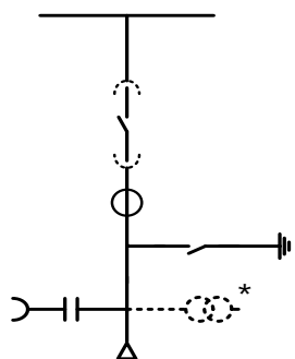
Fig.1 : Celda de Entrada de Transformador
