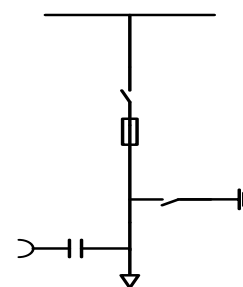
Fig.5 : Celda de SS/AA con seccionador Fusible
