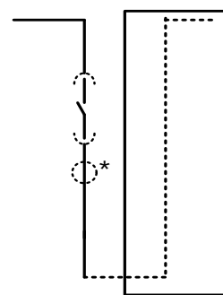
Fig.2 : Celda Acoplamiento y Remonte de Barra
