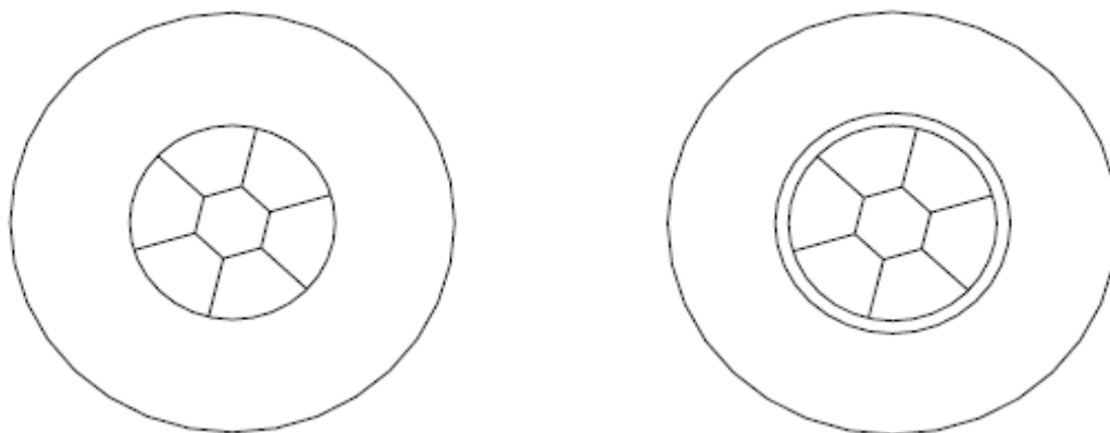
Figura 1: Izquierda) Formación de cable protegido para tensión de red 15 kV y 25 kV. Derecha) Formación de cable protegido para tensión de red de 36 kV.
