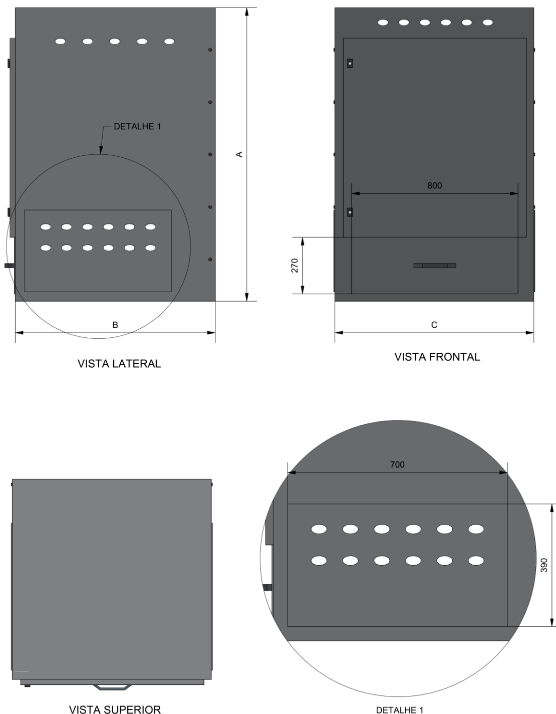
Figura 3 - Caixa de telecomunicações Anti-Furto
