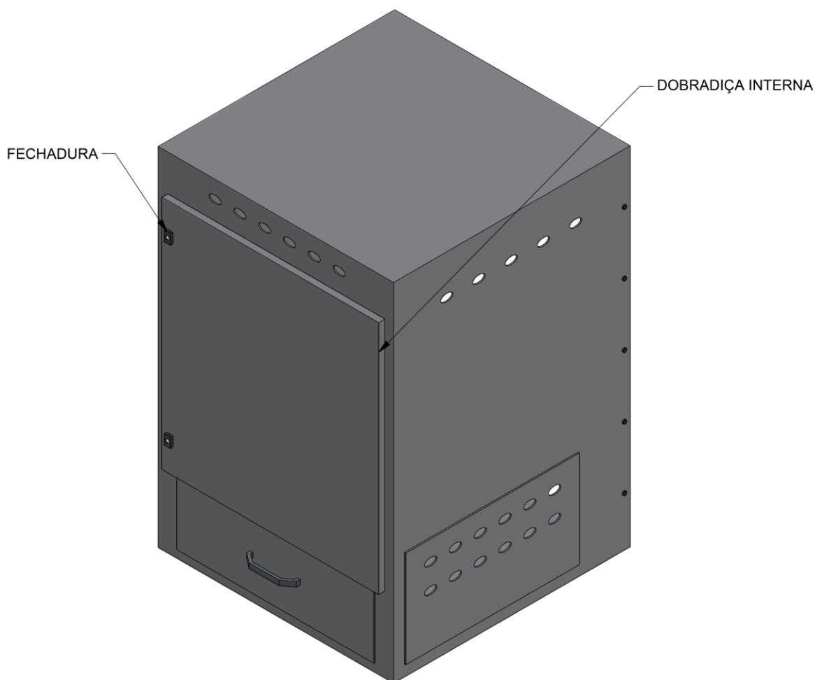
VISTA EM PERSPECTIVA
