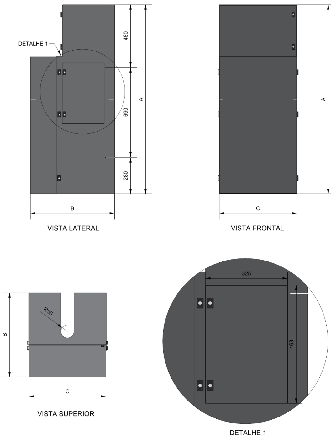
Figura 1 - Caixa de comando Anti-Furto
