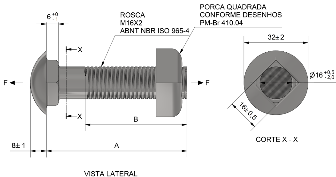
Figura 1 - Parafuso de cabeça Abaulada
