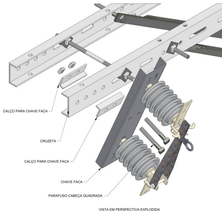
Figura 2 - Detalhe de aplicação de calço peça F86
