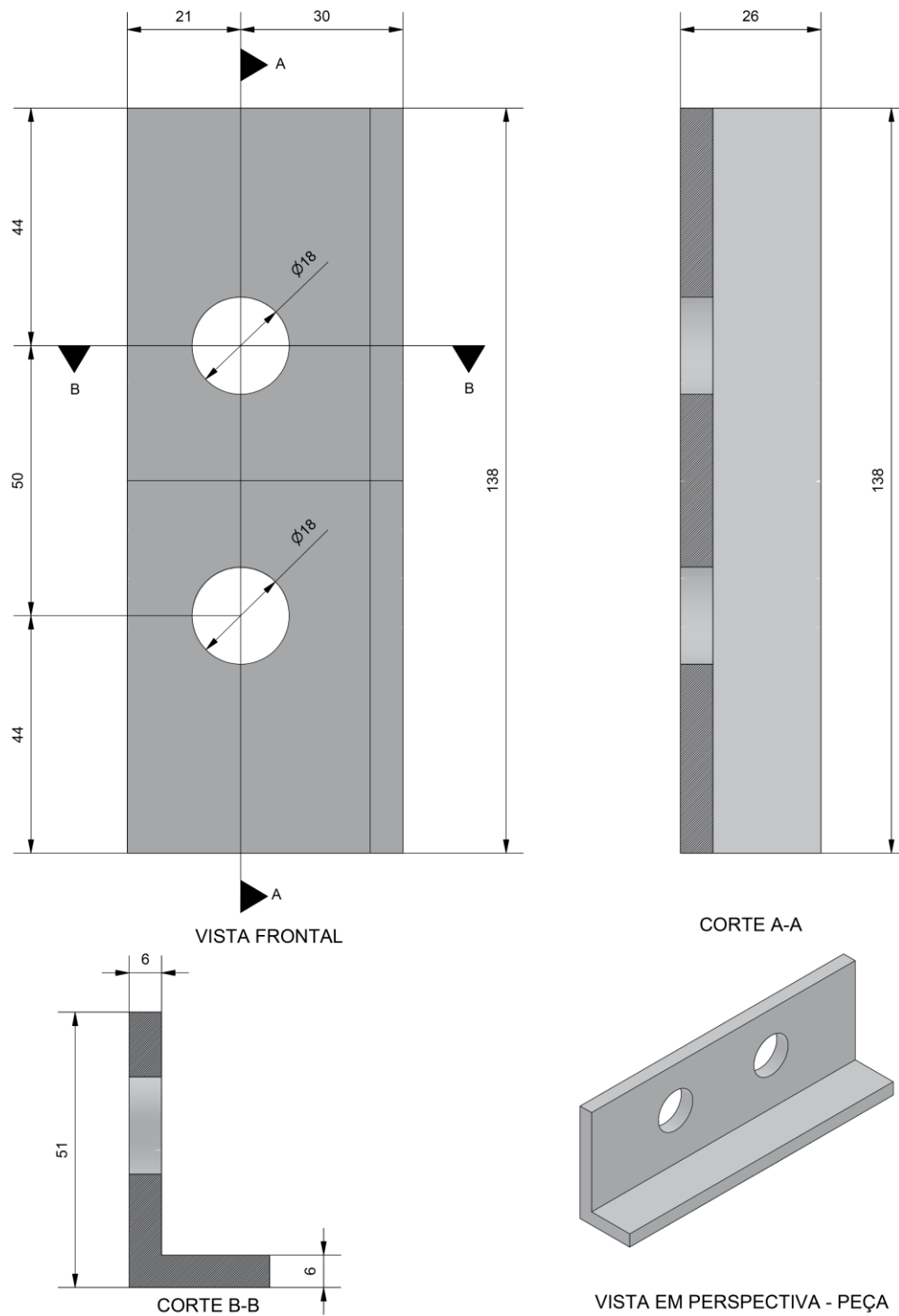
Figura 1 - Calço para chave faca
