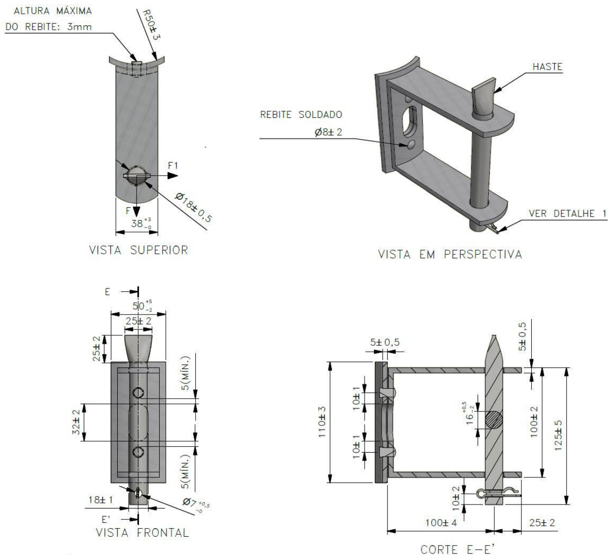
Figura 2 - Armação secundária 1 estribo
