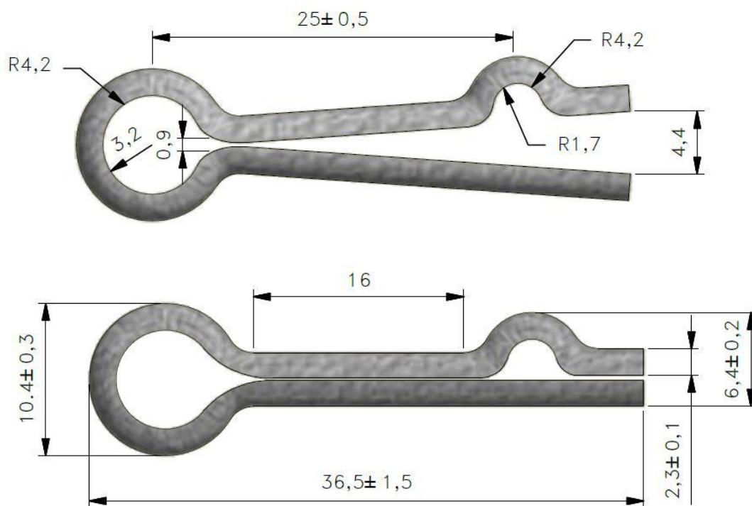
DETALHE 1
