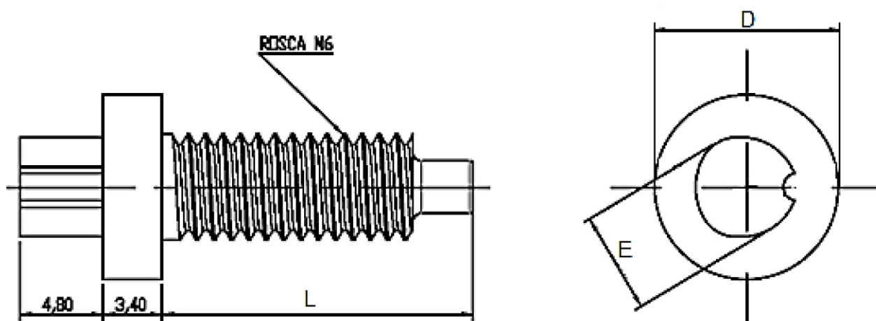
Figura 1 - Parafuso de Segurança
