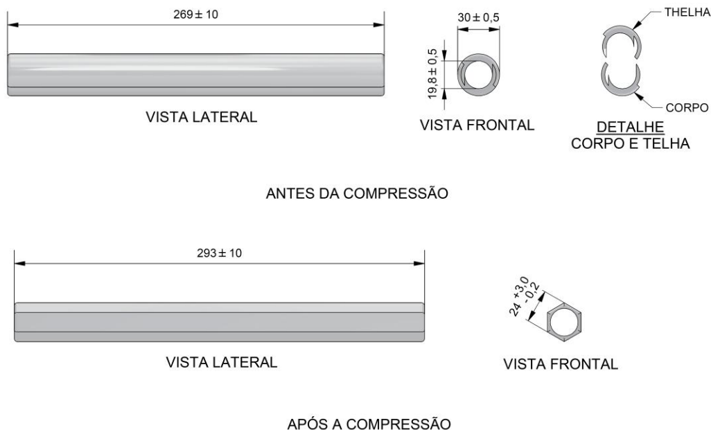
Figura 1 - Luva de Reparo à Compressão para Cabo de Alumínio
