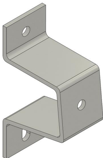
VISTA EM PERSPECTIVA
