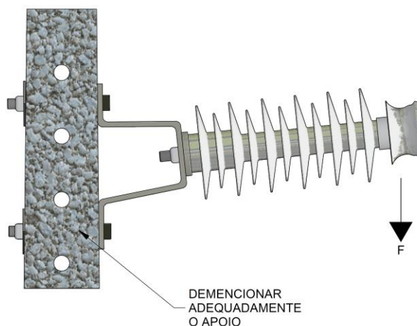
DETALHE - ENSAIO MECÂNICO
