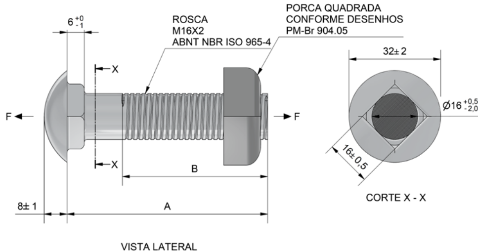
Figura 1 - Parafuso Cabeça abaulada - Liga de alumínio
