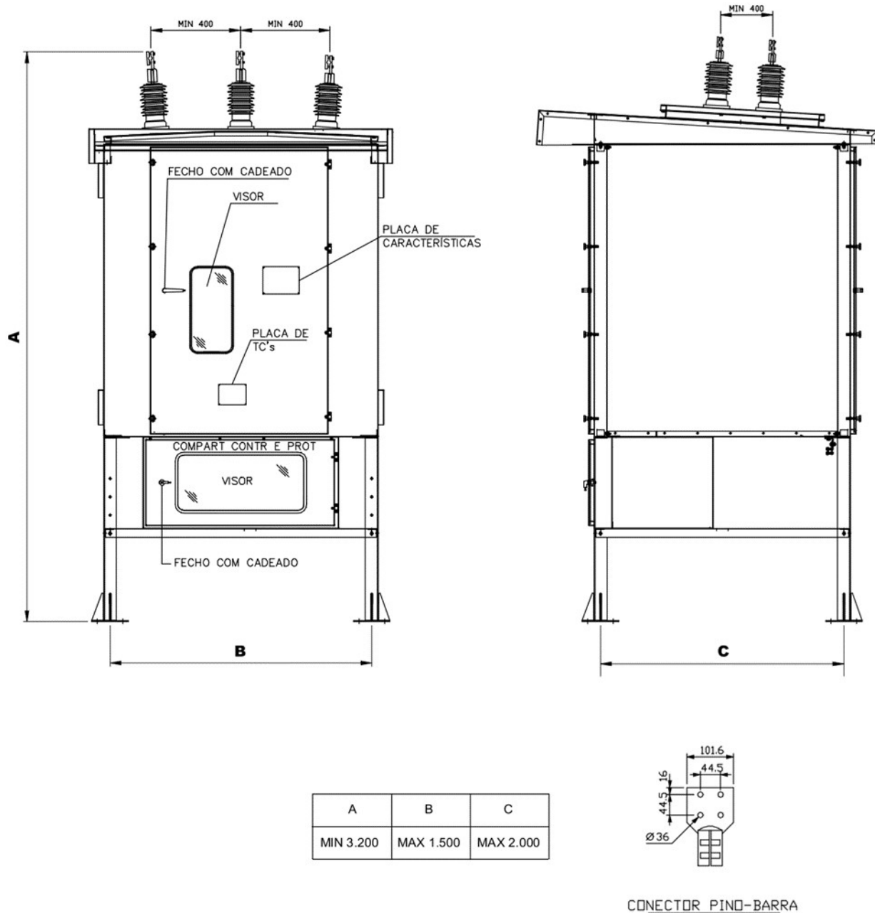
Figura 1 - Disjuntor e dimensões
