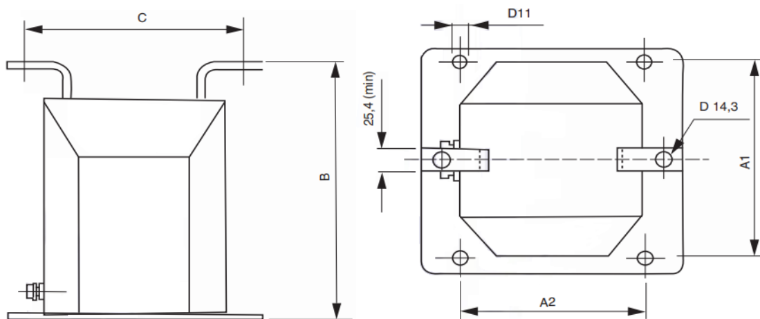
Figura 1 - TC com terminal-barras até 300A (referência Figura A.1 NBR 10021)
