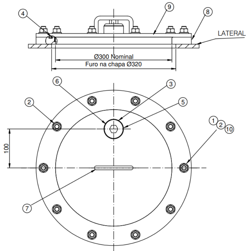
Figura 28 - Janela de inspeção circular do transformador submersível tipo radial (RD)
