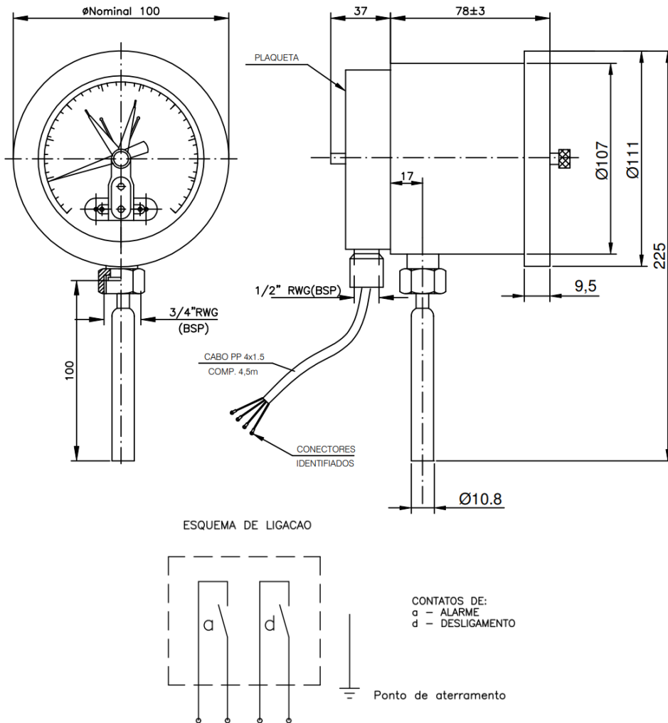
Figura 22 - Termômetro
