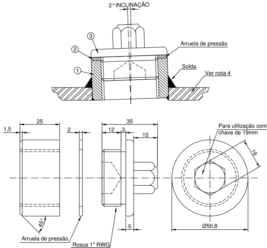
Figura 21 - Bujão para enchimento de óleo e ligação do filtro prensa (RD/RT)
