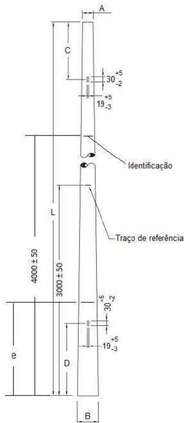
Figura 1 - Dimensões e indicações do poste
