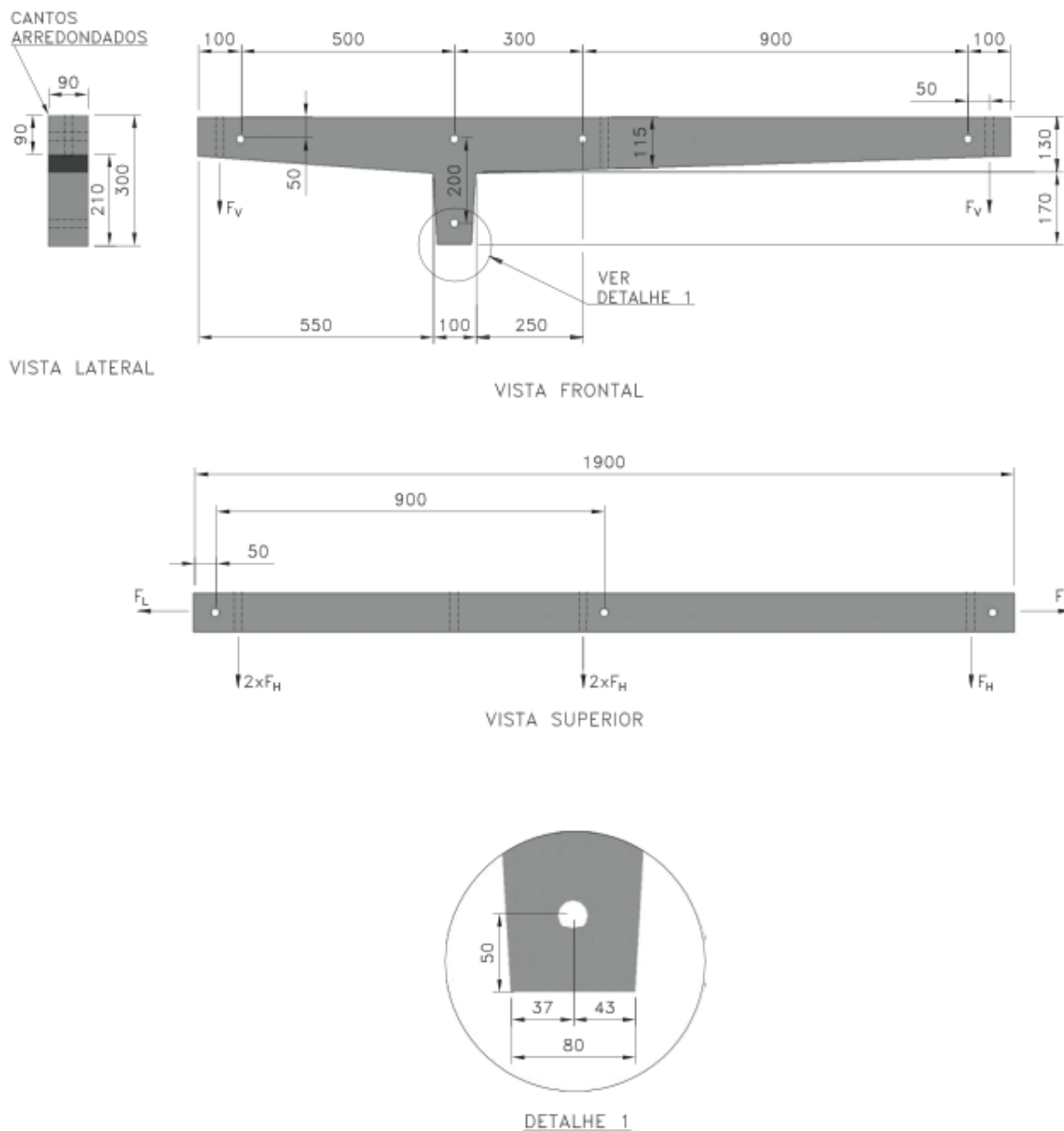
Figura 5 - Cruzeta de concreto armado meio beco - tipo "MB" – 1900mm
