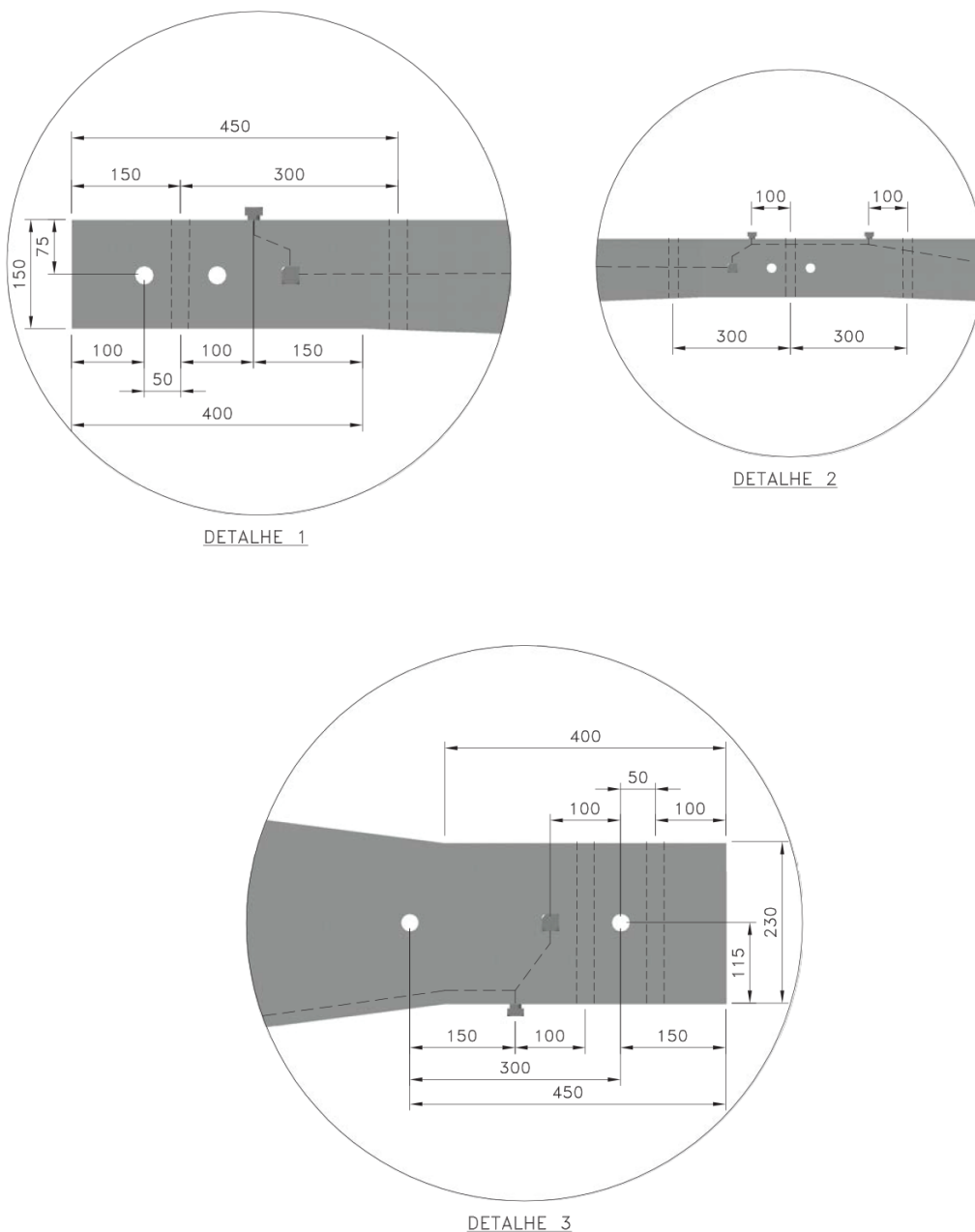
Figura 12 - Cruzeta de concreto armado simples - tipo "H" – 6700mm - detalhes
