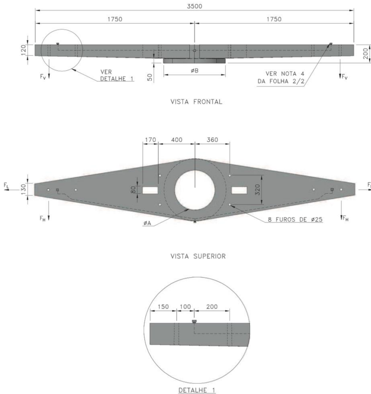
Figura 9 - Cruzeta de concreto armado modelo simples – 3500mm
