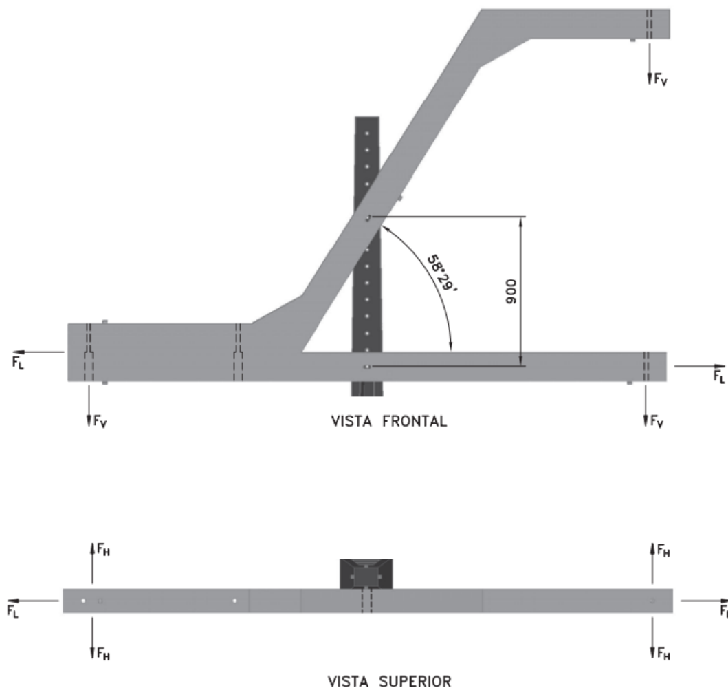
Figura 18 - Cruzetas de concreto armado - Tipo "Z" e "I" esforços
