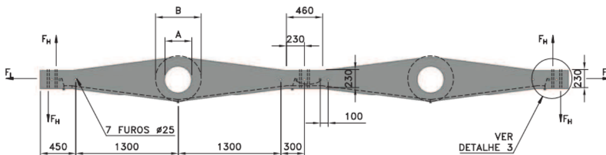
VISTA SUPERIOR
