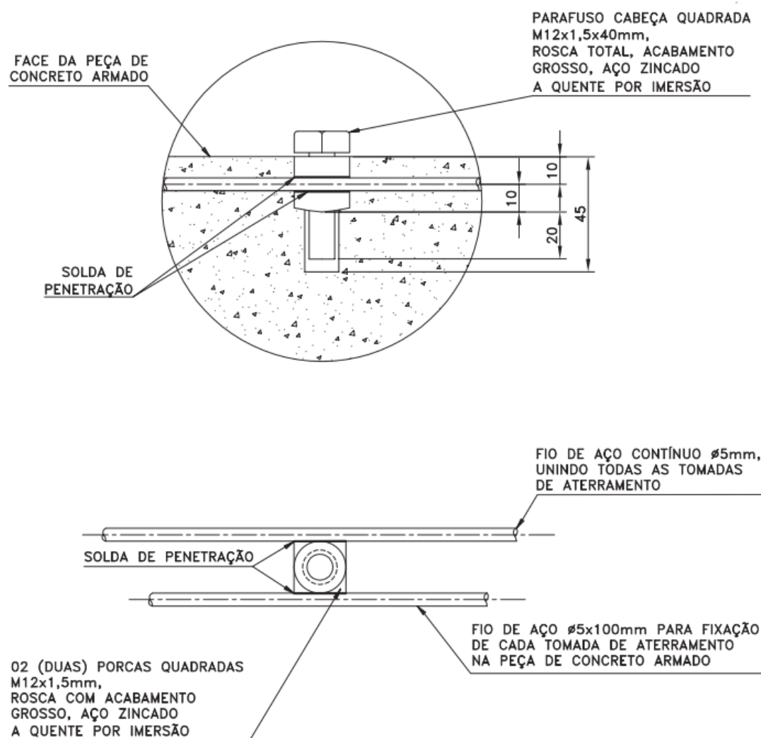
Figura 19 - Tomada de aterramento
