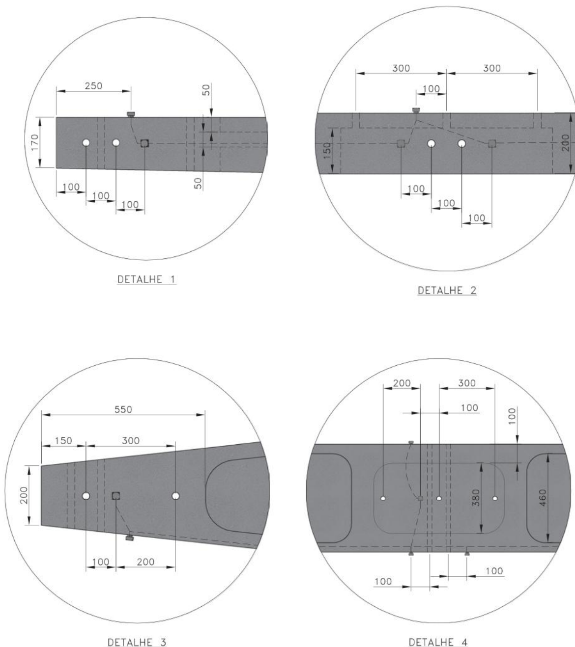
Figura 14 - Cruzeta de concreto armado especial - tipo "H" – 6700mm - detalhes
