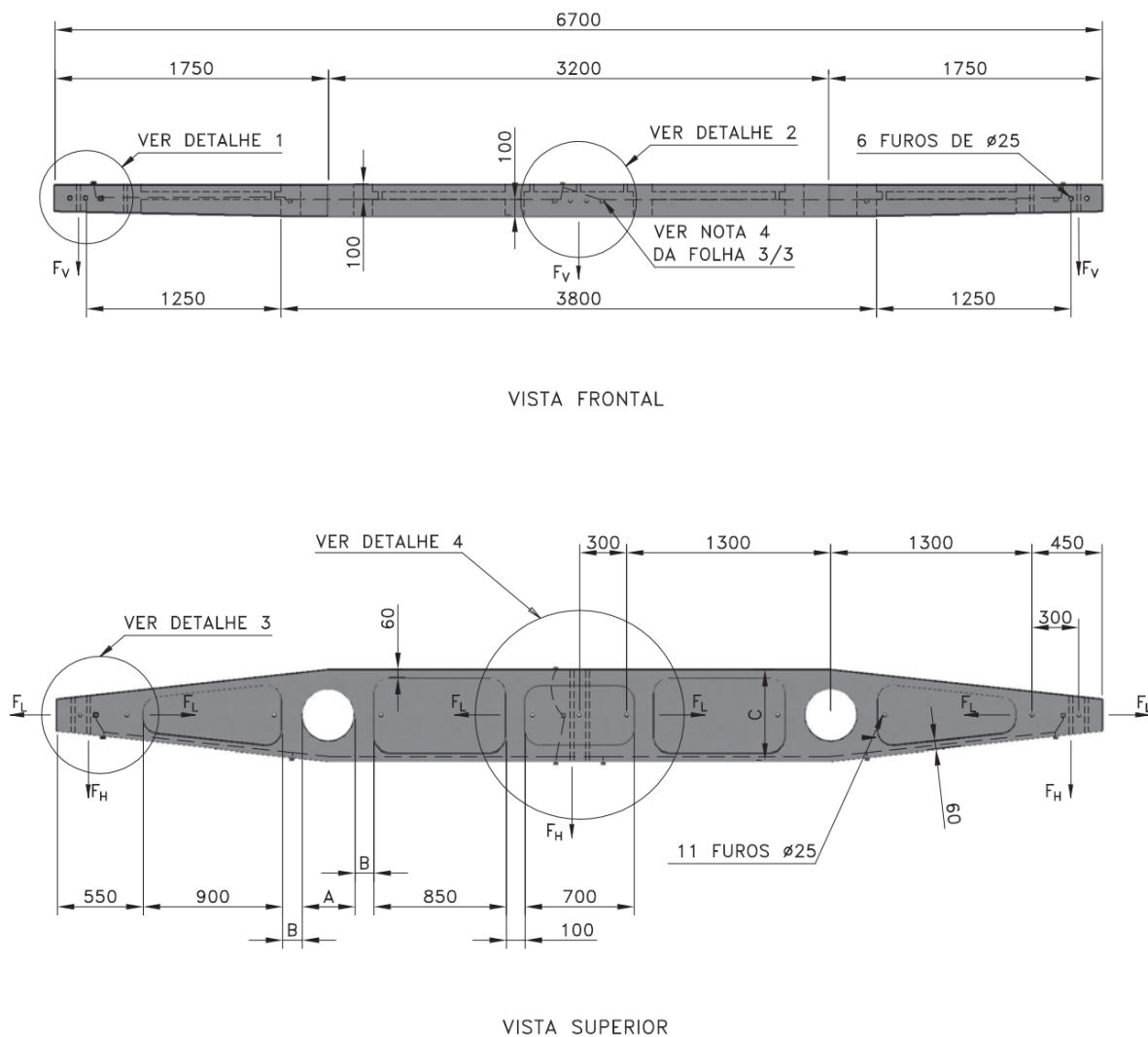
Figura 13 - Cruzeta de concreto armado especial - tipo "H" – 6700mm
