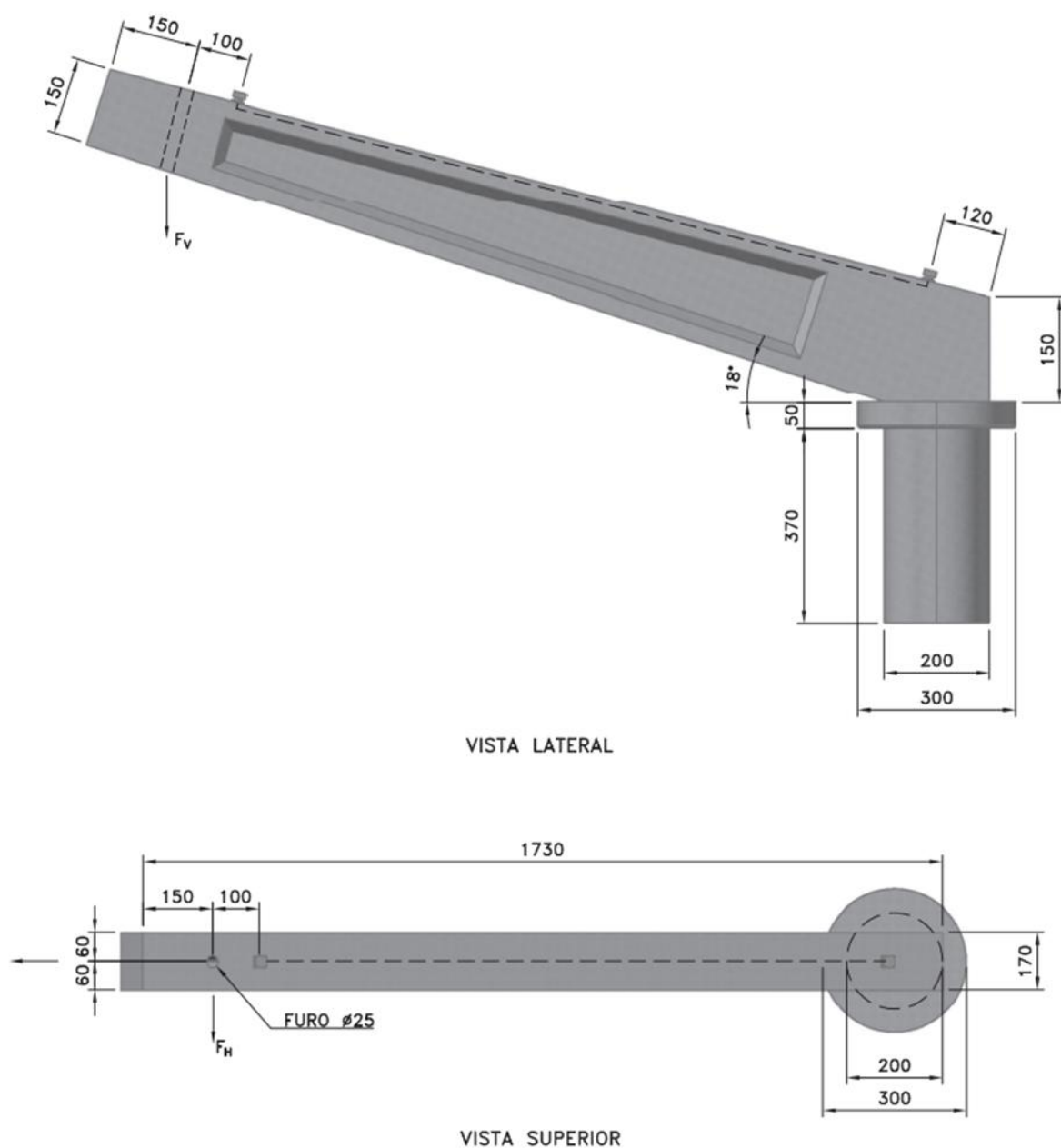
Figura 16 - Cruzeta de concreto armado pivotante
