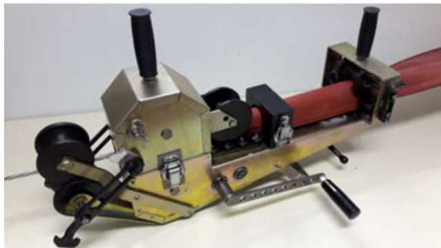
Figura 12 - Desenho Ilustrativo: Ferramentas auxiliares de instalação de proteções Isolantes
