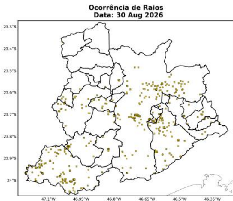
Figura 12: Ocorrências de descargas atmosféricas nuvem-solo detectadas pelo sistema Earth Networks para o dia 30 de Agosto sobre a área de concessão da ENEL-SP.
