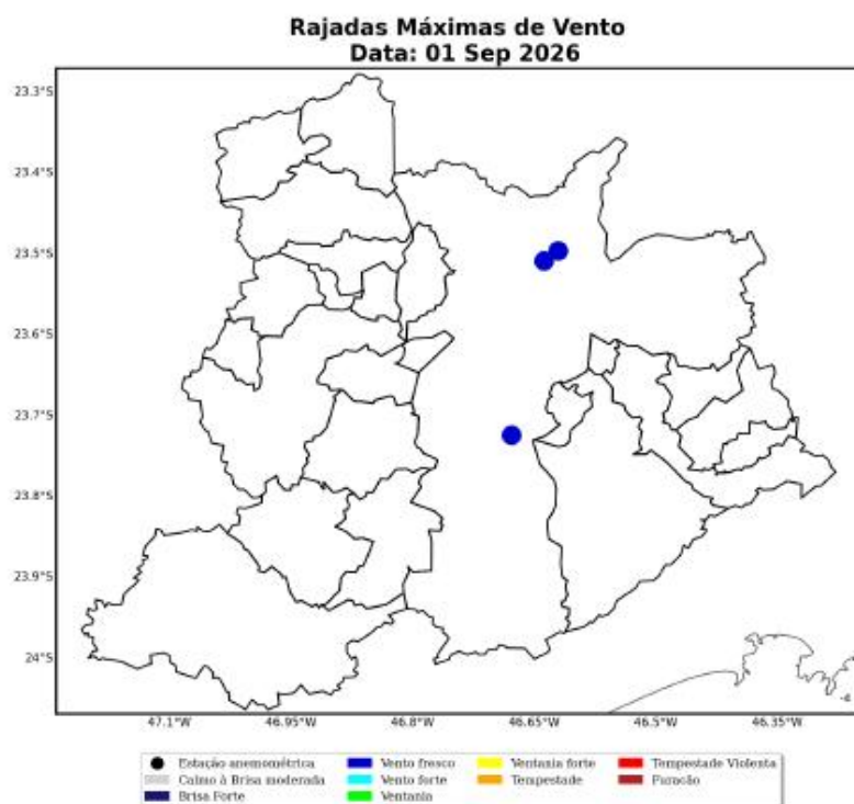
Figura 32: Máxima rajada de vento diária sobre a área de concessão da ENEL-SP para o dia 01 de Setembro, baseado nas estações meteorológicas do INMET.
