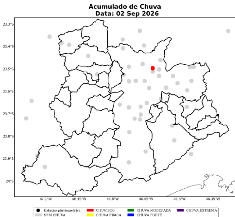
Figura 22: Acumulado diário de precipitação sobre a área de concessão da ENEL-SP para o dia 02 de Setembro, baseado nas estações meteorológicas do INMET e CEMADEN.
