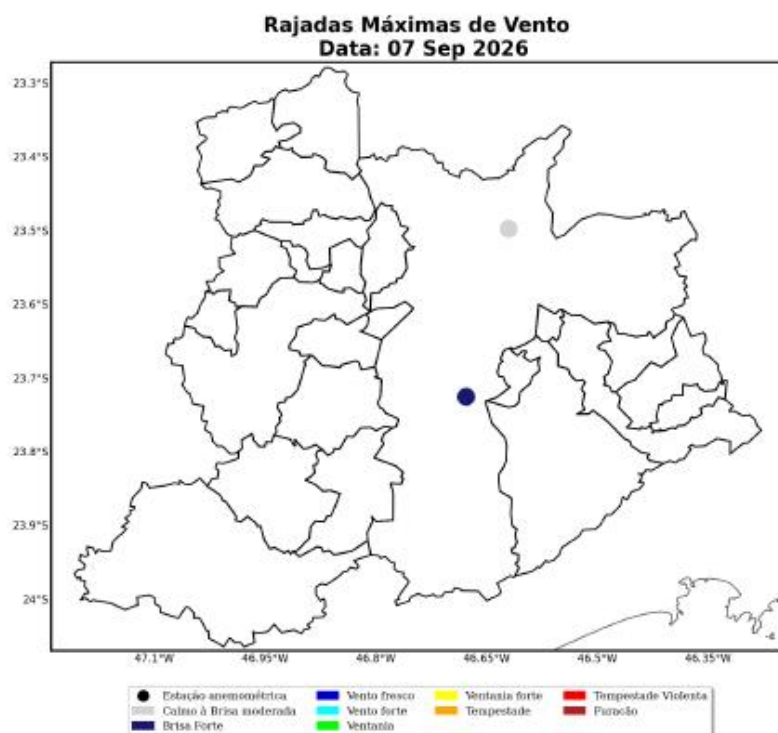
Figura 38: Máxima rajada de vento diária sobre a área de concessão da ENEL-SP para o dia 07 de Setembro, baseado nas estações meteorológicas do INMET.
