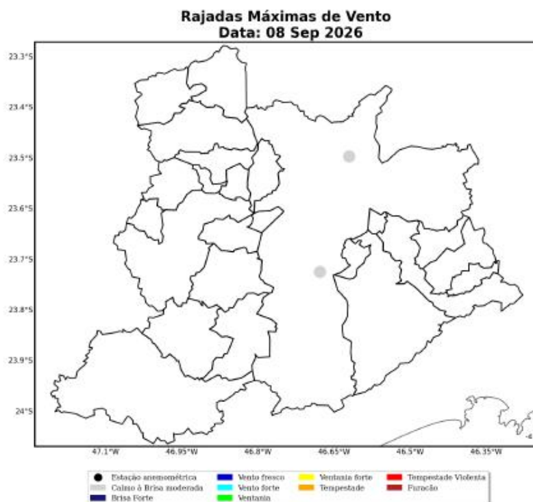
Figura 39: Máxima rajada de vento diária sobre a área de concessão da ENEL-SP para o dia 08 de Setembro, baseado nas estações meteorológicas do INMET.
