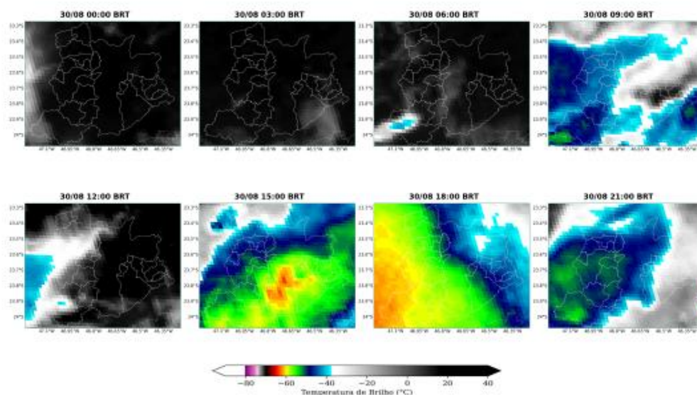
Figura 2: Imagens realçadas do satélite GOES-19 das 00 BRT até 21 BRT (a cada 3 horas) para o dia 30 de Agosto.
