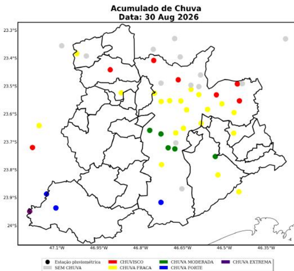
Figura 19: Acumulado diário de precipitação sobre a área de concessão da ENEL-SP para o dia 30 de Agosto, baseado nas estações meteorológicas do INMET e CEMADEN.
