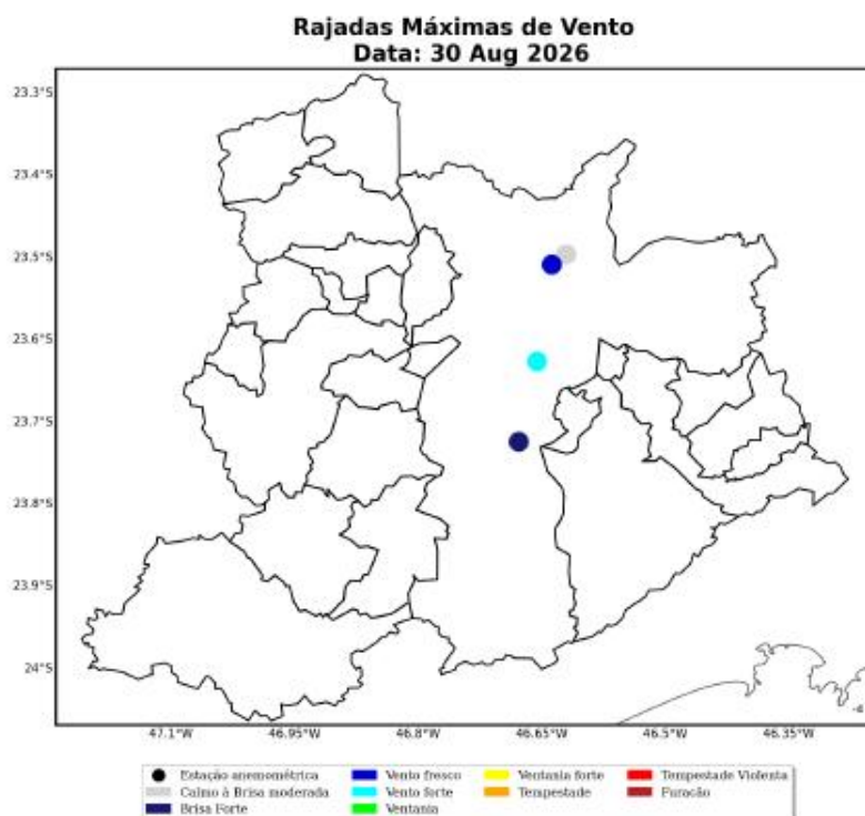
Figura 30: Máxima rajada de vento diária sobre a área de concessão da ENEL-SP para o dia 30 de Agosto, baseado nas estações meteorológicas do INMET.
