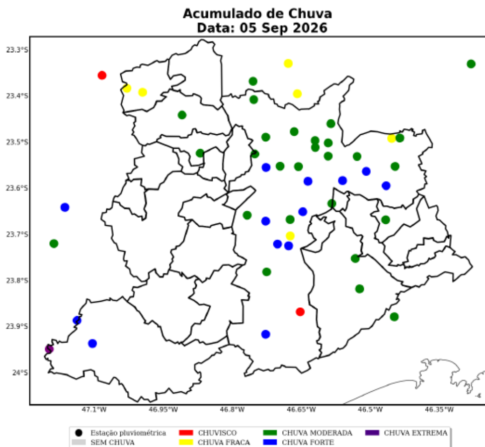
Figura 25: Acumulado diário de precipitação sobre a área de concessão da ENEL-SP para o dia 05 de Setembro, baseado nas estações meteorológicas do INMET e CEMADEN.
