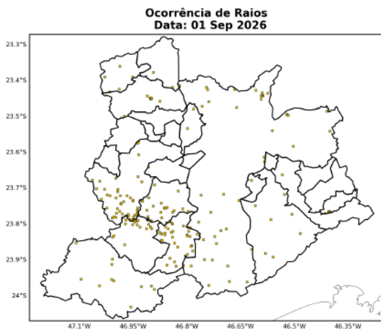
Figura 14: Ocorrências de descargas atmosféricas nuvem-solo detectadas pelo sistema Earth Networks para o dia 01 de Setembro sobre a área de concessão da ENEL-SP.
