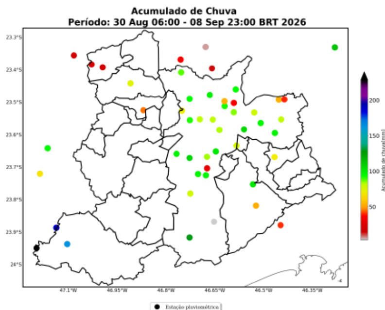
Figura 29: Acumulado de precipitação sobre a área de concessão da ENEL-SP para o período do evento (dias 30 de Agosto a 08 de Setembro de 2026), baseado nas estações meteorológicas do INMET e CEMADEN.
