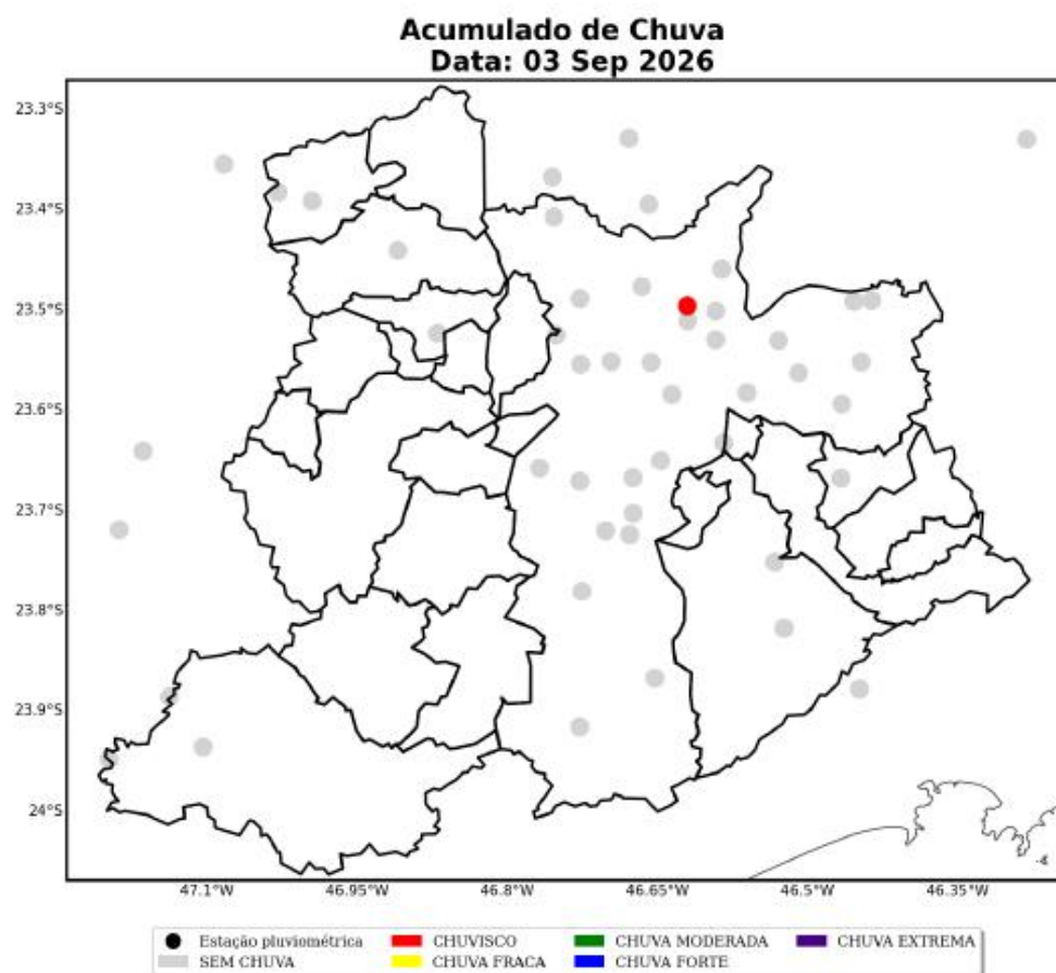
Figura 23: Acumulado diário de precipitação sobre a área de concessão da ENEL-SP para o dia 03 de Setembro, baseado nas estações meteorológicas do INMET e CEMADEN.
