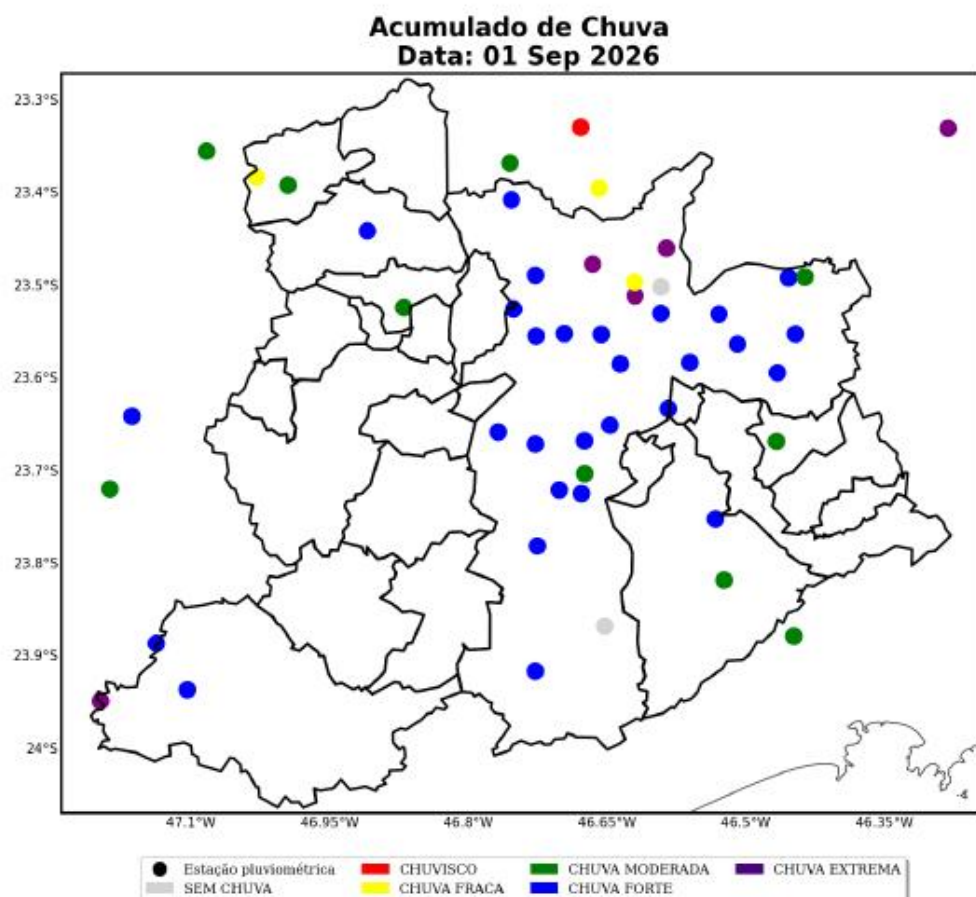
Figura 21: Acumulado diário de precipitação sobre a área de concessão da ENEL-SP para o dia 01 de Setembro, baseado nas estações meteorológicas do INMET e CEMADEN.
