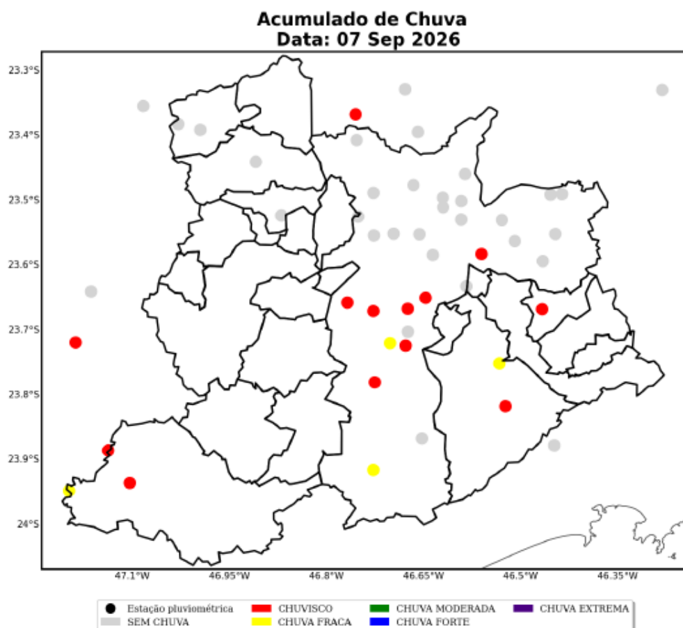
Figura 27: Acumulado diário de precipitação sobre a área de concessão da ENEL-SP para o dia 07 de Setembro, baseado nas estações meteorológicas do INMET e CEMADEN.
