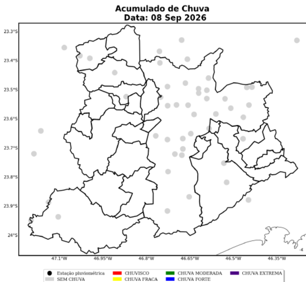
Figura 28: Acumulado diário de precipitação sobre a área de concessão da ENEL-SP para o dia 08 de Setembro, baseado nas estações meteorológicas do INMET e CEMADEN.
