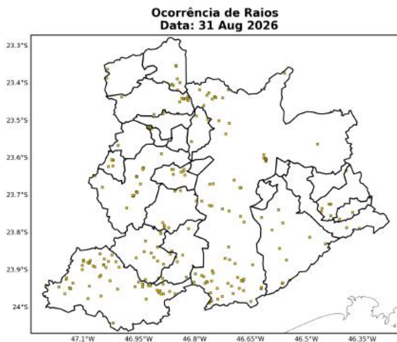
Figura 13: Ocorrências de descargas atmosféricas nuvem-solo detectadas pelo sistema Earth Networks para o dia 31 de Agosto sobre a área de concessão da ENEL-SP.
