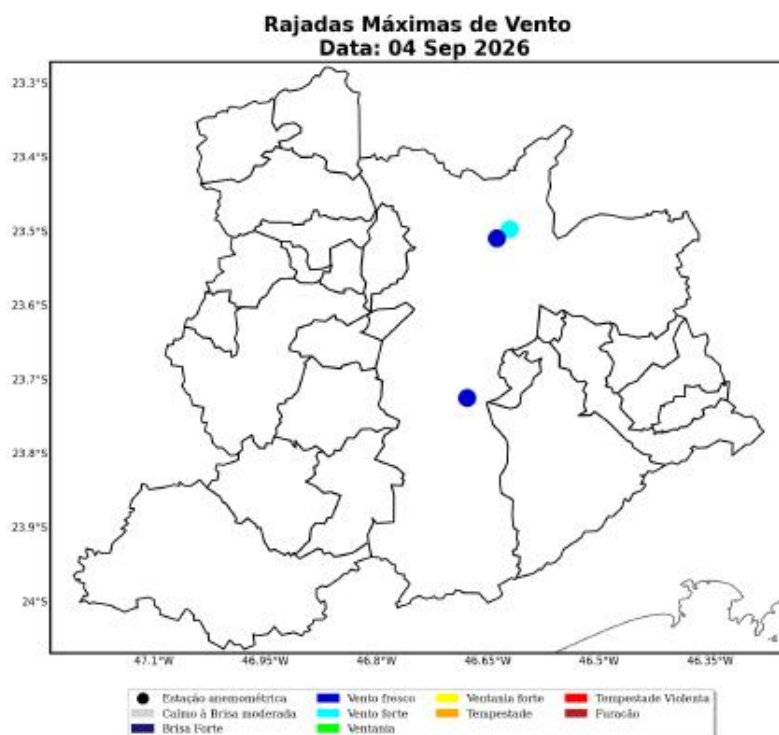
Figura 35: Máxima rajada de vento diária sobre a área de concessão da ENEL-SP para o dia 04 de Setembro, baseado nas estações meteorológicas do INMET.
