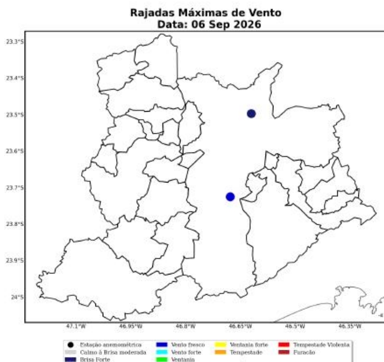
Figura 37: Máxima rajada de vento diária sobre a área de concessão da ENEL-SP para o dia 06 de Setembro, baseado nas estações meteorológicas do INMET.
