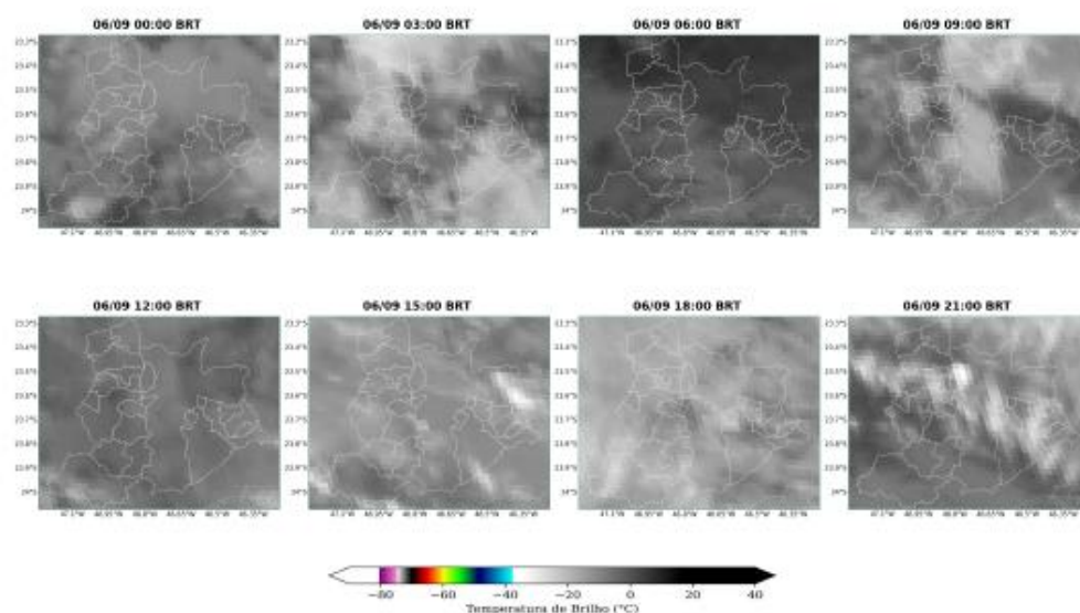
Figura 9: Imagens realçadas do satélite GOES-19 das 00 BRT até 21 BRT (a cada 3 horas) para o dia 06 de Setembro.
