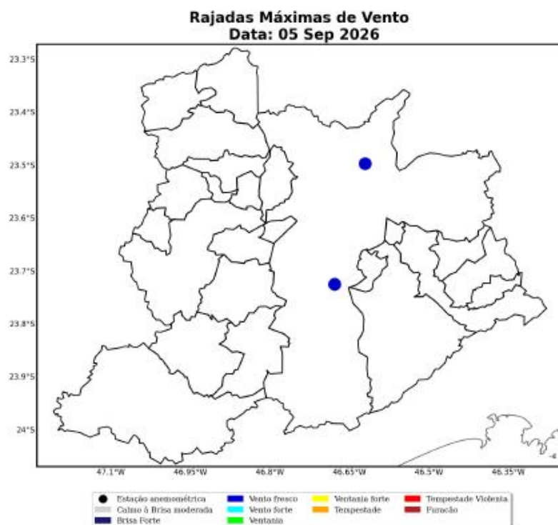
Figura 36: Máxima rajada de vento diária sobre a área de concessão da ENEL-SP para o dia 05 de Setembro, baseado nas estações meteorológicas do INMET.
