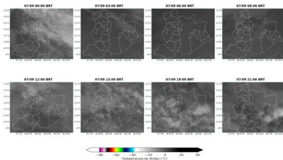
Figura 10: Imagens realizadas do satélite GOES-19 das 00 BRT até 21 BRT (a cada 3 horas) para o dia 07 de Setembro.
