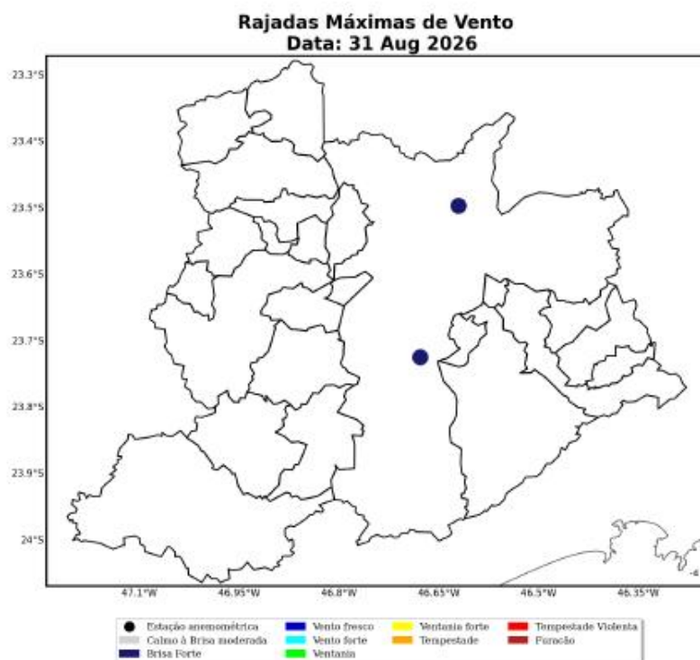
Figura 31: Máxima rajada de vento diária sobre a área de concessão da ENEL-SP para o dia 31 de Agosto, baseado nas estações meteorológicas do INMET.
