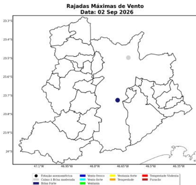
Figura 33: Máxima rajada de vento diária sobre a área de concessão da ENEL-SP para o dia 02 de Setembro, baseado nas estações meteorológicas do INMET.
