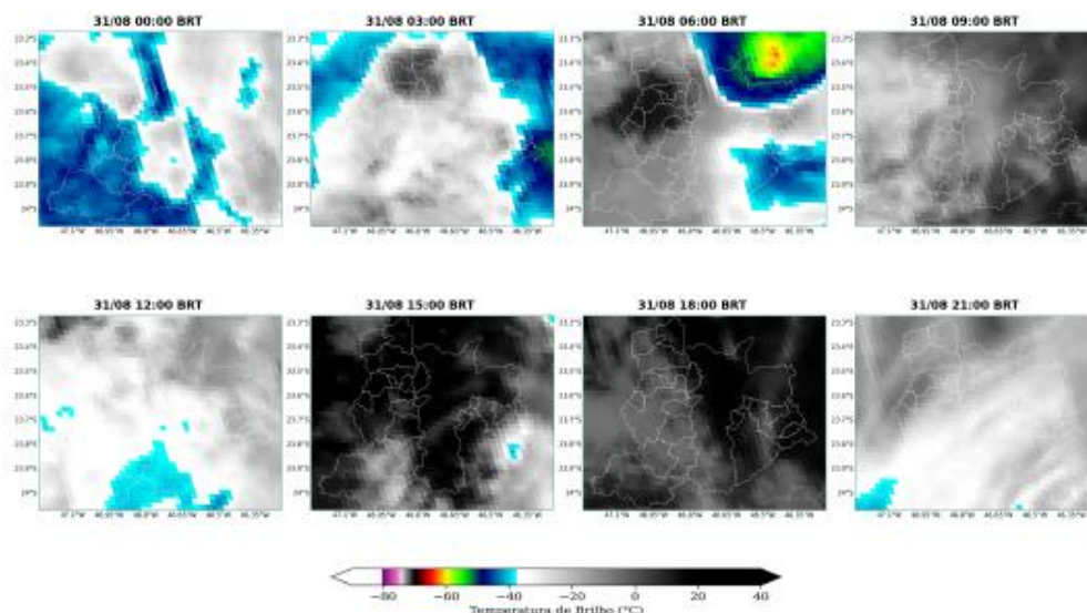
Figura 3: Imagens realçadas do satélite GOES-19 das 00 BRT até 21 BRT (a cada 3 horas) para o dia 31 de Agosto.
