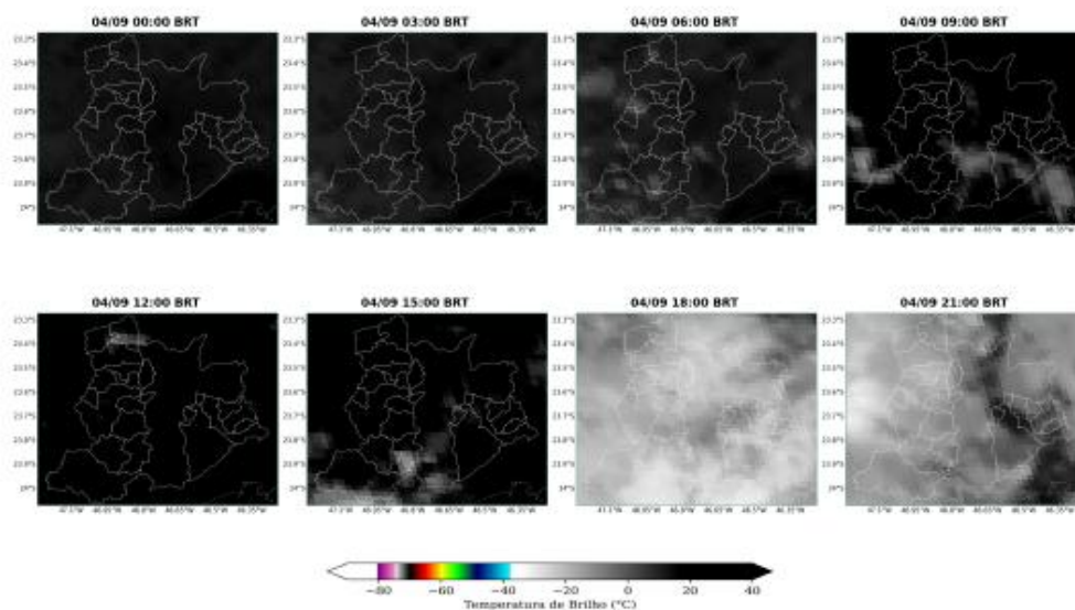
Figura 7: Imagens realçadas do satélite GOES-19 das 00 BRT até 21 BRT (a cada 3 horas) para o dia 04 de Setembro.
