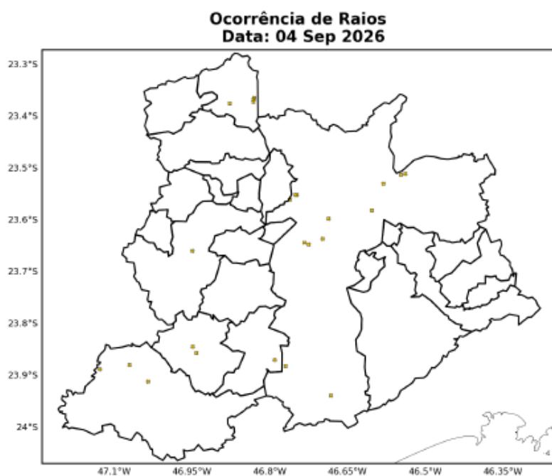
Figura 15: Ocorrências de descargas atmosféricas nuvem-solo detectadas pelo sistema Earth Networks para o dia 04 de Setembro sobre a área de concessão da ENEL-SP.
