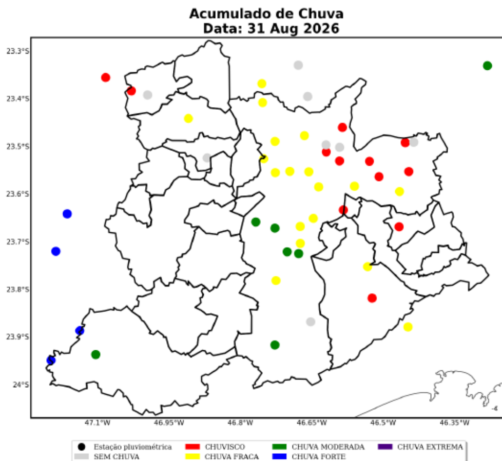
Figura 20: Acumulado diário de precipitação sobre a área de concessão da ENEL-SP para o dia 31 de Agosto, baseado nas estações meteorológicas do INMET e CEMADEN.
