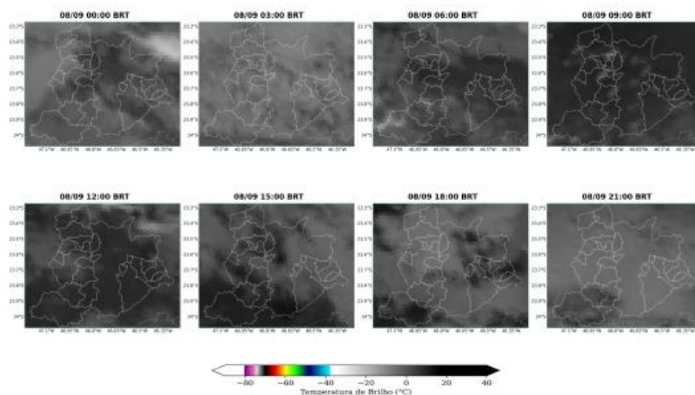
Figura 11: Imagens realçadas do satélite GOES-19 das 00 BRT até 21 BRT (a cada 3 horas) para o dia 08 de Setembro.
