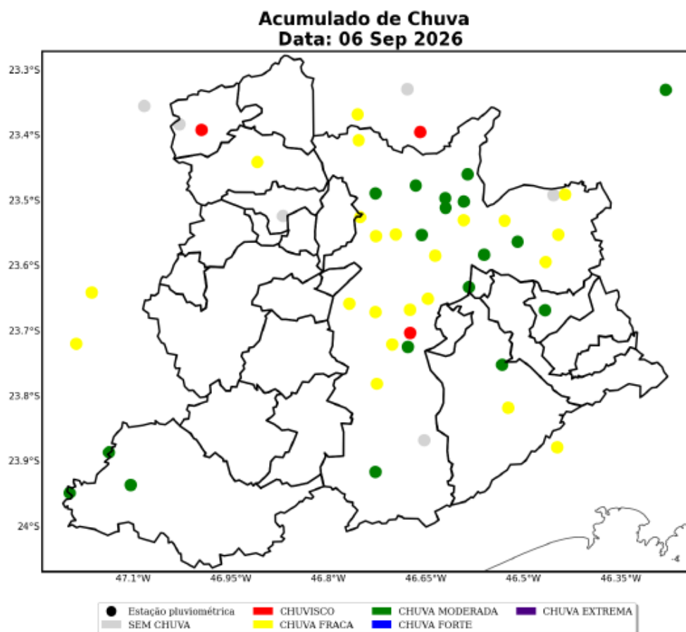
Figura 26: Acumulado diário de precipitação sobre a área de concessão da ENEL-SP para o dia 06 de Setembro, baseado nas estações meteorológicas do INMET e CEMADEN.
