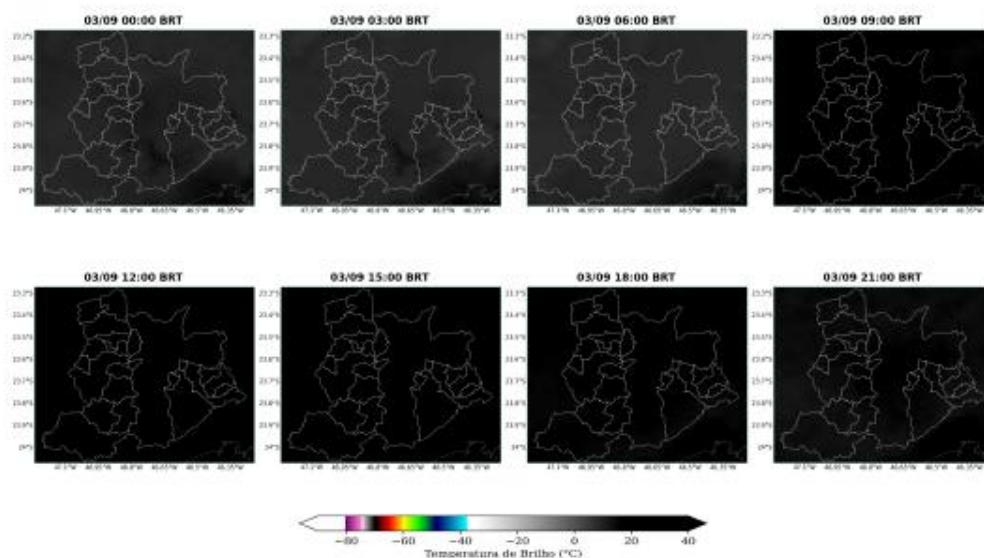
Figura 6: Imagens realçadas do satélite GOES-19 das 00 BRT até 21 BRT (a cada 3 horas) para o dia 03 de Setembro.
