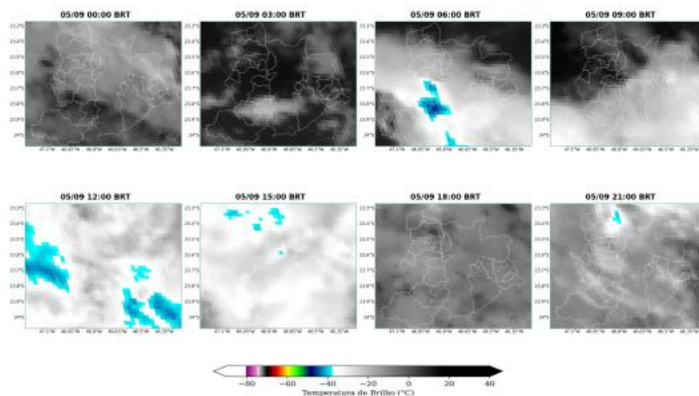
Figura 8: Imagens realçadas do satélite GOES-19 das 00 BRT até 21 BRT (a cada 3 horas) para o dia 05 de Setembro.
