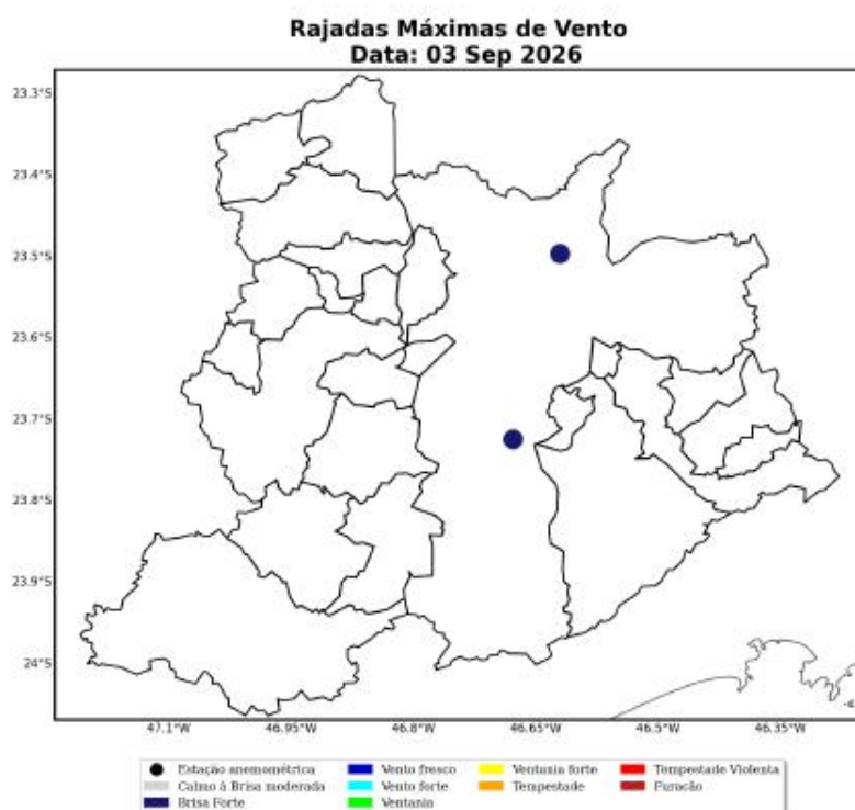
Figura 34: Máxima rajada de vento diária sobre a área de concessão da ENEL-SP para o dia 03 de Setembro, baseado nas estações meteorológicas do INMET.
