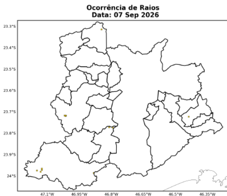
Figura 17: Ocorrências de descargas atmosféricas nuvem-solo detectadas pelo sistema Earth Networks para o dia 07 de Setembro sobre a área de concessão da ENEL-SP.
