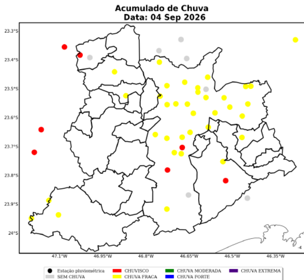
Figura 24: Acumulado diário de precipitação sobre a área de concessão da ENEL-SP para o dia 04 de Setembro, baseado nas estações meteorológicas do INMET e CEMADEN.
