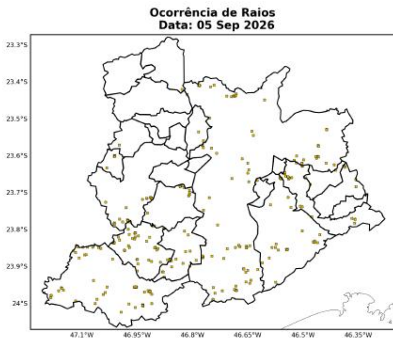
Figura 16: Ocorrências de descargas atmosféricas nuvem-solo detectadas pelo sistema Earth Networks para o dia 05 de Setembro sobre a área de concessão da ENEL-SP.
