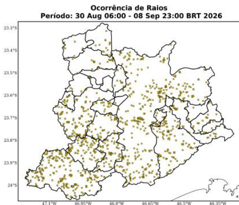
Figura 18: Ocorrências de descargas atmosféricas nuvem-solo detectadas pelo sistema Earth Networks para o período de 30 de Agosto a 08 de Setembro de 2026 sobre a área de concessão da ENEL-SP.
