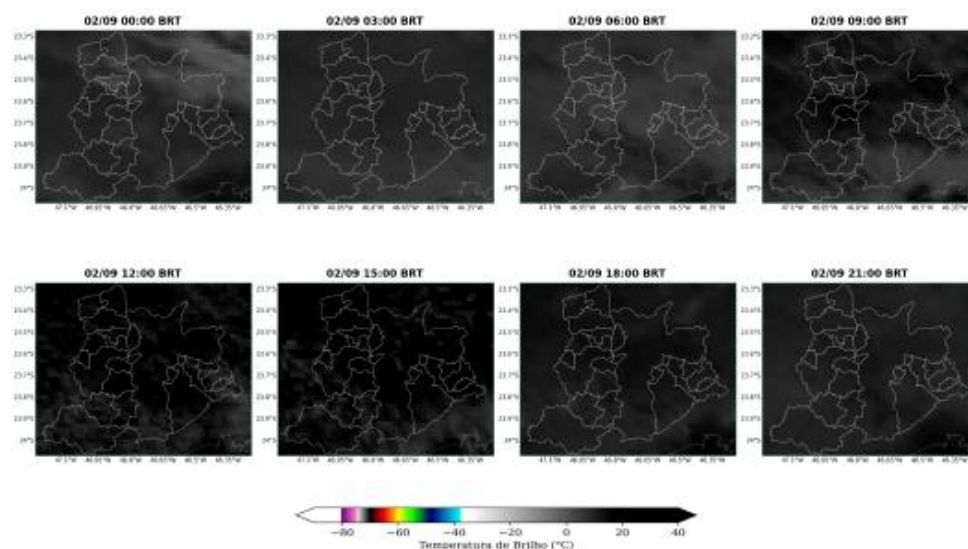
Figura 5: Imagens realçadas do satélite GOES-19 das 00 BRT até 21 BRT (a cada 3 horas) para o dia 02 de Setembro.
