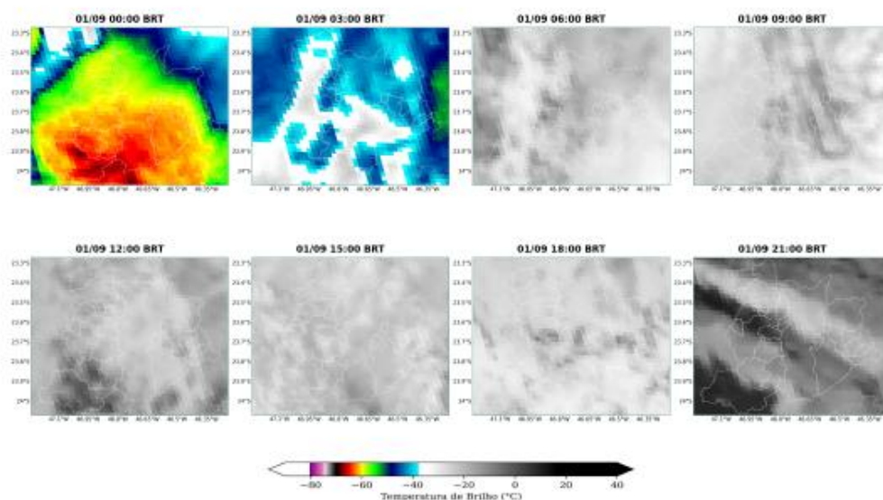
Figura 4: Imagens realçadas do satélite GOES-19 das 00 BRT até 21 BRT (a cada 3 horas) para o dia 01 de Setembro.
