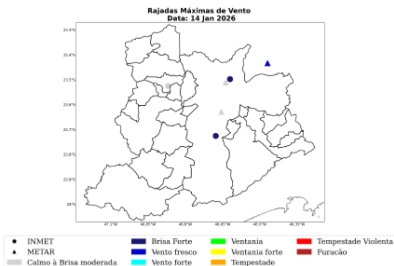
Figura 32: Máxima rajada de vento diária sobre a área de concessão da ENEL-SP para o dia 14 de Janeiro, baseado nas estações meteorológicas do INMET.
