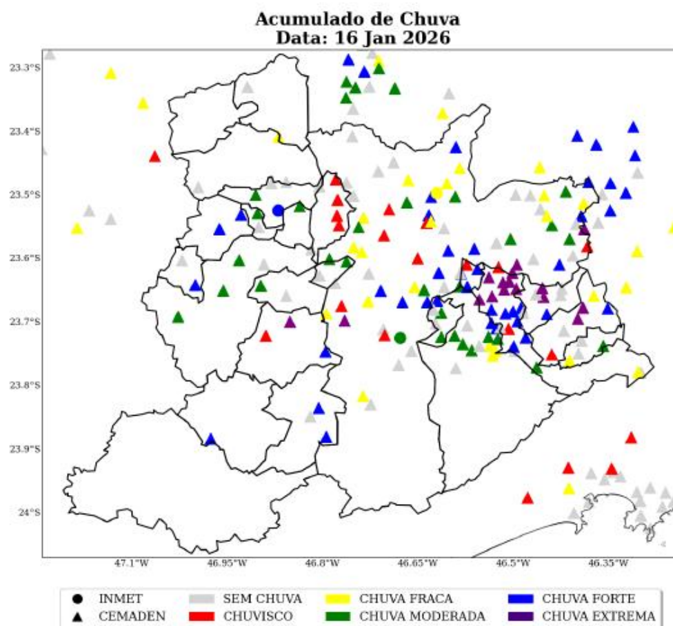
Figura 24: Acumulado diário de precipitação sobre a área de concessão da ENEL-SP para o dia 16 de Janeiro, baseado nas estações meteorológicas do INMET e CEMADEN.
