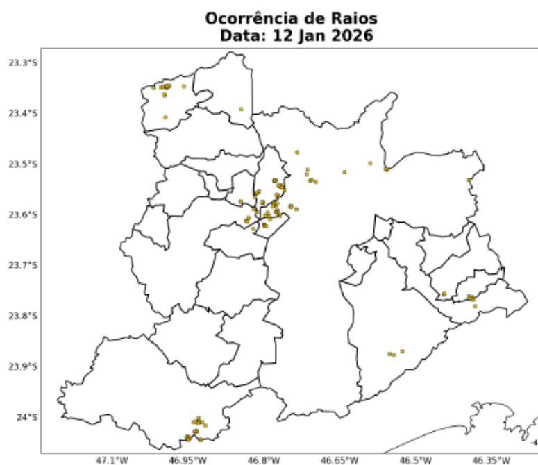
Figura 11: Ocorrências de descargas atmosféricas nuvem-solo detectadas pelo sistema Earth Networks para o dia 12 de Janeiro sobre a área de concessão da ENEL-SP.
