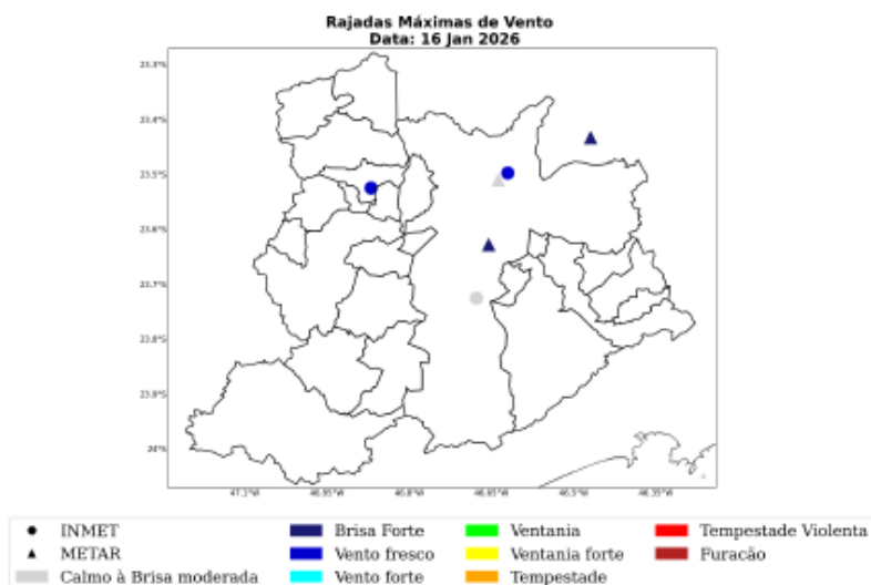
Figura 34: Máxima rajada de vento diária sobre a área de concessão da ENEL-SP para o dia 16 de Janeiro, baseado nas estações meteorológicas do INMET.
