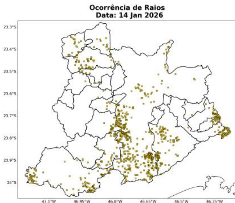
Figura 13: Ocorrências de descargas atmosféricas nuvem-solo detectadas pelo sistema Earth Networks para o dia 14 de Janeiro sobre a área de concessão da ENEL-SP.
