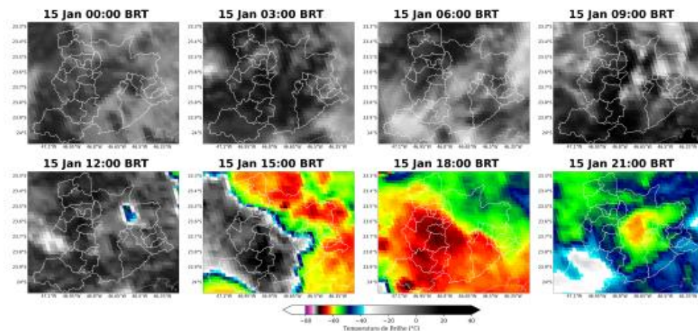
Figura 5: Imagens realçadas do satélite GOES-19 das 00 BRT até 21 BRT (a cada 3 horas) para o dia 15 de Janeiro.
