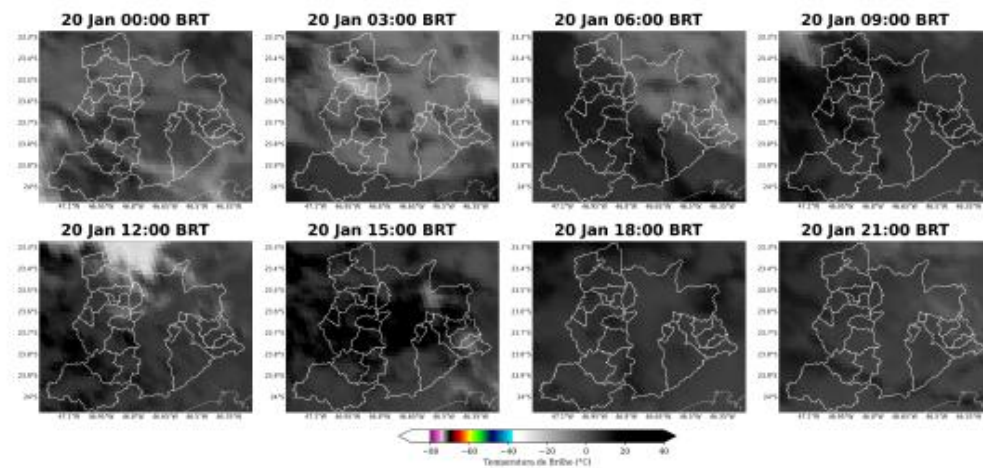
Figura 10: Imagens realçadas do satélite GOES-19 das 00 BRT até 21 BRT (a cada 3 horas) para o dia 20 de Janeiro.
