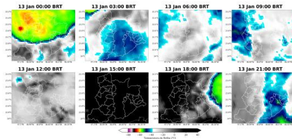
Figura 3: Imagens realçadas do satélite GOES-19 das 00 BRT até 21 BRT (a cada 3 horas) para o dia 13 de Janeiro.
