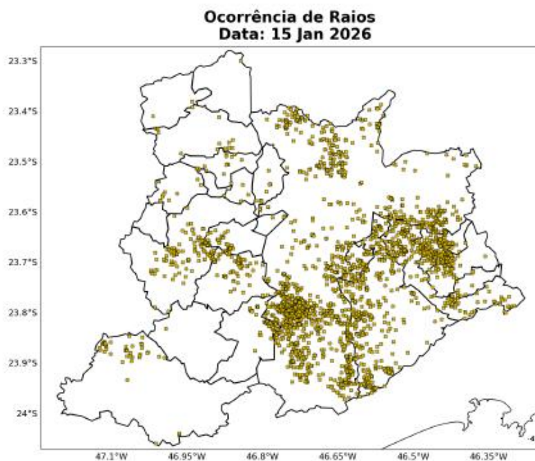
Figura 14: Ocorrências de descargas atmosféricas nuvem-solo detectadas pelo sistema Earth Networks para o dia 15 de Janeiro sobre a área de concessão da ENEL-SP.
