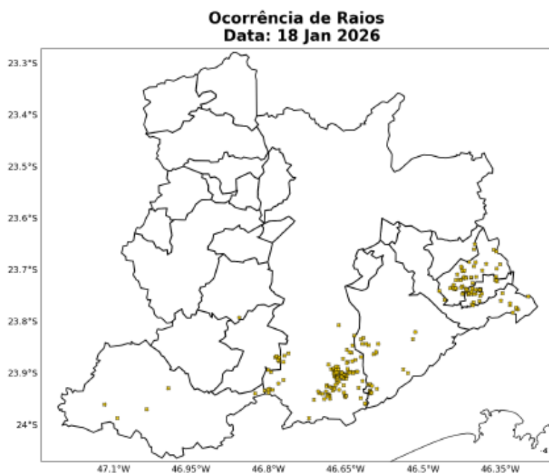
Figura 17: Ocorrências de descargas atmosféricas nuvem-solo detectadas pelo sistema Earth Networks para o dia 18 de Janeiro sobre a área de concessão da ENEL-SP.
