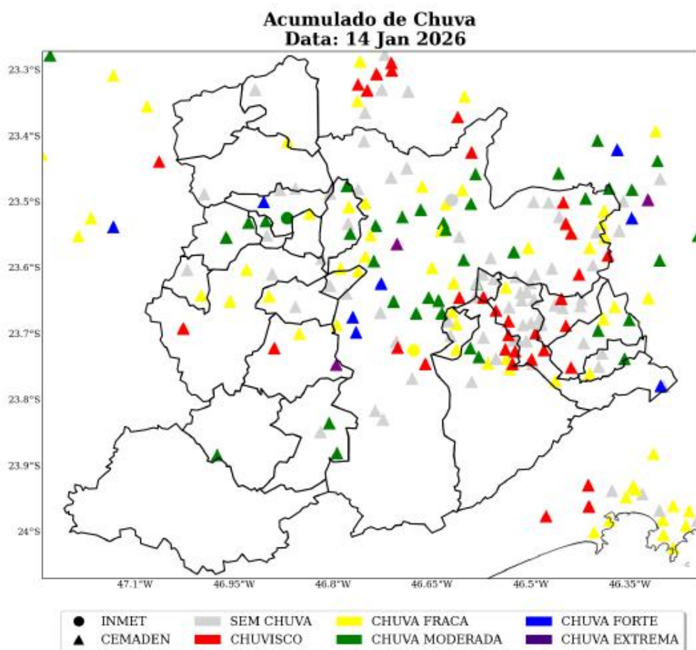
Figura 22: Acumulado diário de precipitação sobre a área de concessão da ENEL-SP para o dia 14 de Janeiro, baseado nas estações meteorológicas do INMET e CEMADEN.
