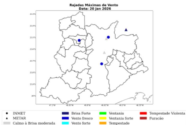
Figura 38: Máxima rajada de vento diária sobre a área de concessão da ENEL-SP para o dia 20 de Janeiro, baseado nas estações meteorológicas do INMET.
