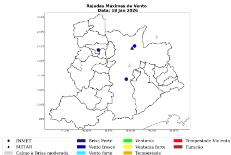
Figura 36: Máxima rajada de vento diária sobre a área de concessão da ENEL-SP para o dia 18 de Janeiro, baseado nas estações meteorológicas do INMET.
