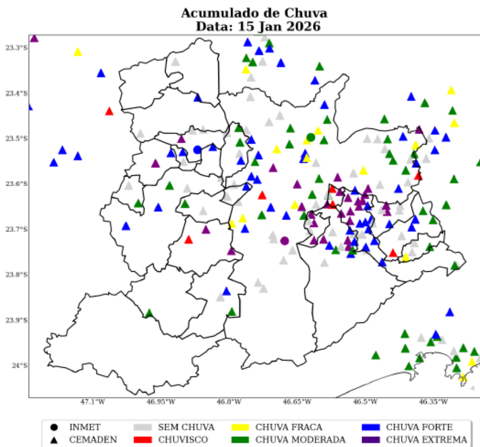
Figura 23: Acumulado diário de precipitação sobre a área de concessão da ENEL-SP para o dia 15 de Janeiro, baseado nas estações meteorológicas do INMET e CEMADEN.
