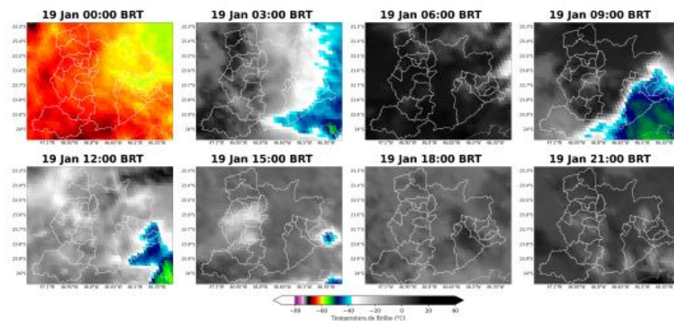
Figura 9: Imagens realçadas do satélite GOES-19 das 00 BRT até 21 BRT (a cada 3 horas) para o dia 19 de Janeiro.
