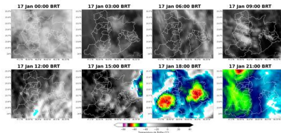
Figura 7: Imagens realçadas do satélite GOES-19 das 00 BRT até 21 BRT (a cada 3 horas) para o dia 17 de Janeiro.
