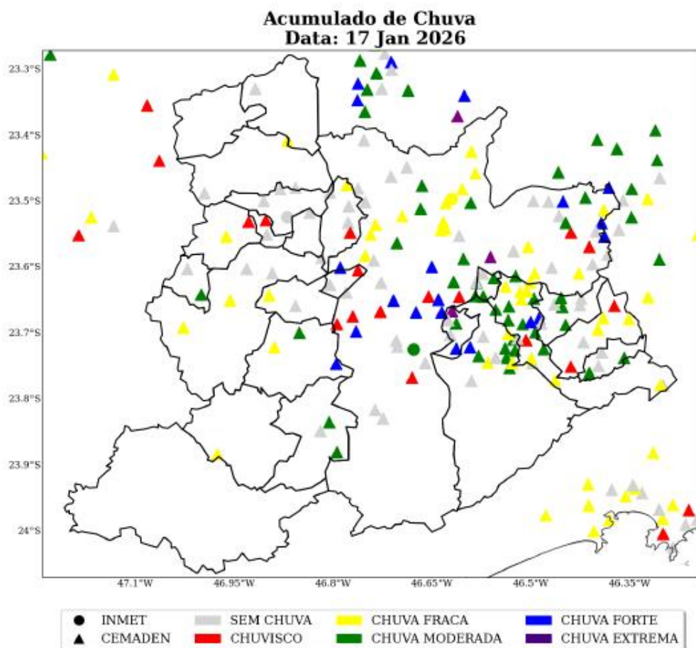
Figura 25: Acumulado diário de precipitação sobre a área de concessão da ENEL-SP para o dia 17 de Janeiro, baseado nas estações meteorológicas do INMET e CEMADEN.
