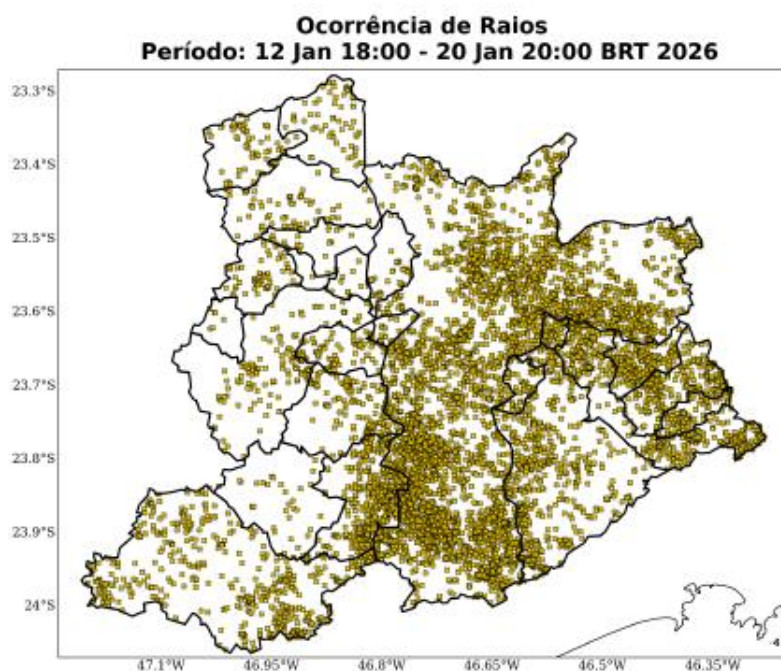
Figura 19: Ocorrências de descargas atmosféricas nuvem-solo detectadas pelo sistema Earth Networks para o período de 12 a 20 de Janeiro de 2026 sobre a área de concessão da ENEL-SP.
