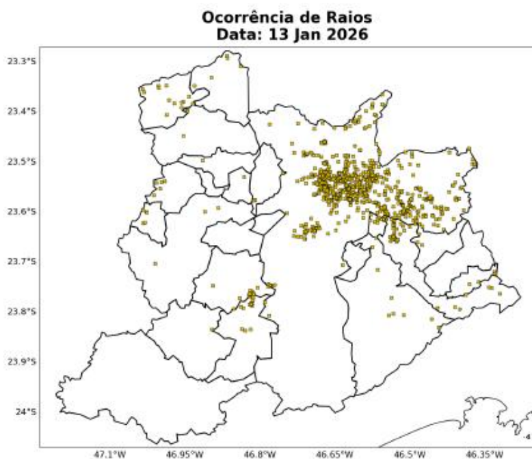
Figura 12: Ocorrências de descargas atmosféricas nuvem-solo detectadas pelo sistema Earth Networks para o dia 13 de Janeiro sobre a área de concessão da ENEL-SP.
