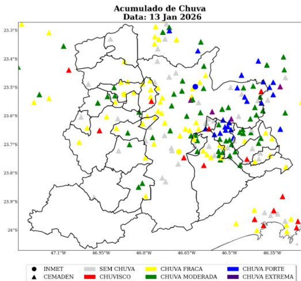
Figura 21: Acumulado diário de precipitação sobre a área de concessão da ENEL-SP para o dia 13 de Janeiro, baseado nas estações meteorológicas do INMET e CEMADEN.
