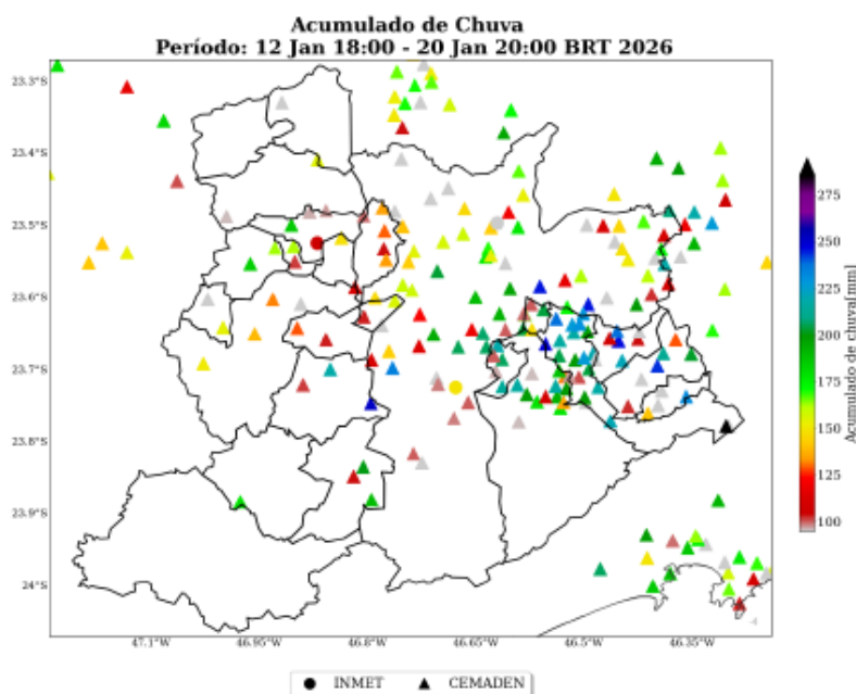
Figura 29: Acumulado de precipitação sobre o estado de São Paulo para o período do evento (dias 12 a 20 de Janeiro de 2026), baseado nas estações meteorológicas do INMET e CEMADEN.
