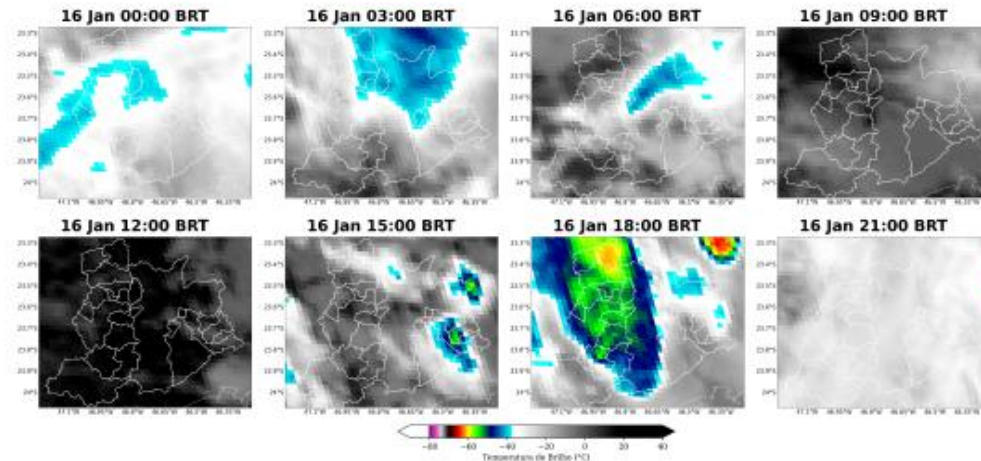
Figura 6: Imagens realçadas do satélite GOES-19 das 00 BRT até 21 BRT (a cada 3 horas) para o dia 16 de Janeiro.
