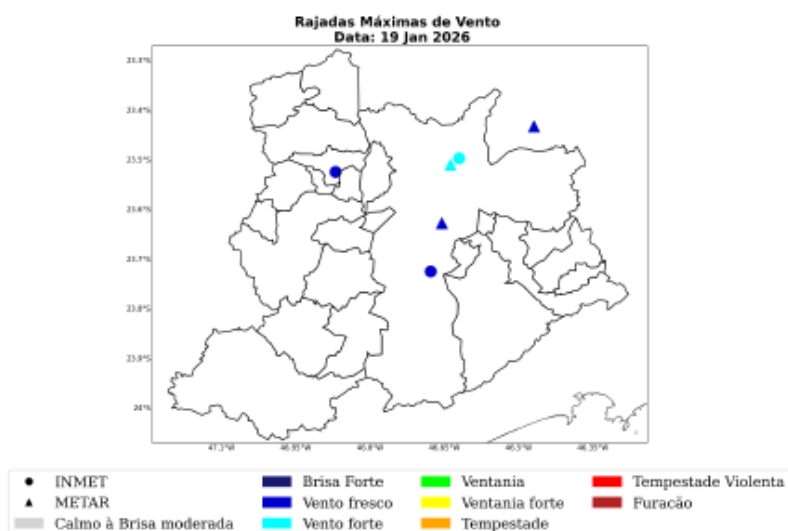
Figura 37: Máxima rajada de vento diária sobre a área de concessão da ENEL-SP para o dia 19 de Janeiro, baseado nas estações meteorológicas do INMET.
