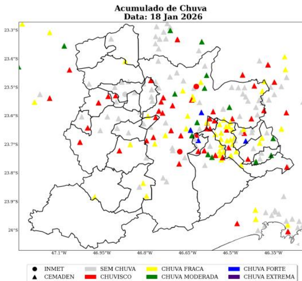
Figura 26: Acumulado diário de precipitação sobre a área de concessão da ENEL-SP para o dia 18 de Janeiro, baseado nas estações meteorológicas do INMET e CEMADEN.
