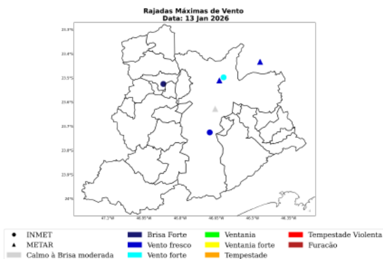
Figura 31: Máxima rajada de vento diária sobre a área de concessão da ENEL-SP para o dia 13 de Janeiro, baseado nas estações meteorológicas do INMET.
