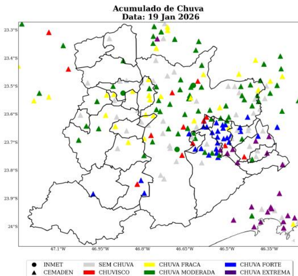
Figura 27: Acumulado diário de precipitação sobre a área de concessão da ENEL-SP para o dia 19 de Janeiro, baseado nas estações meteorológicas do INMET e CEMADEN.
