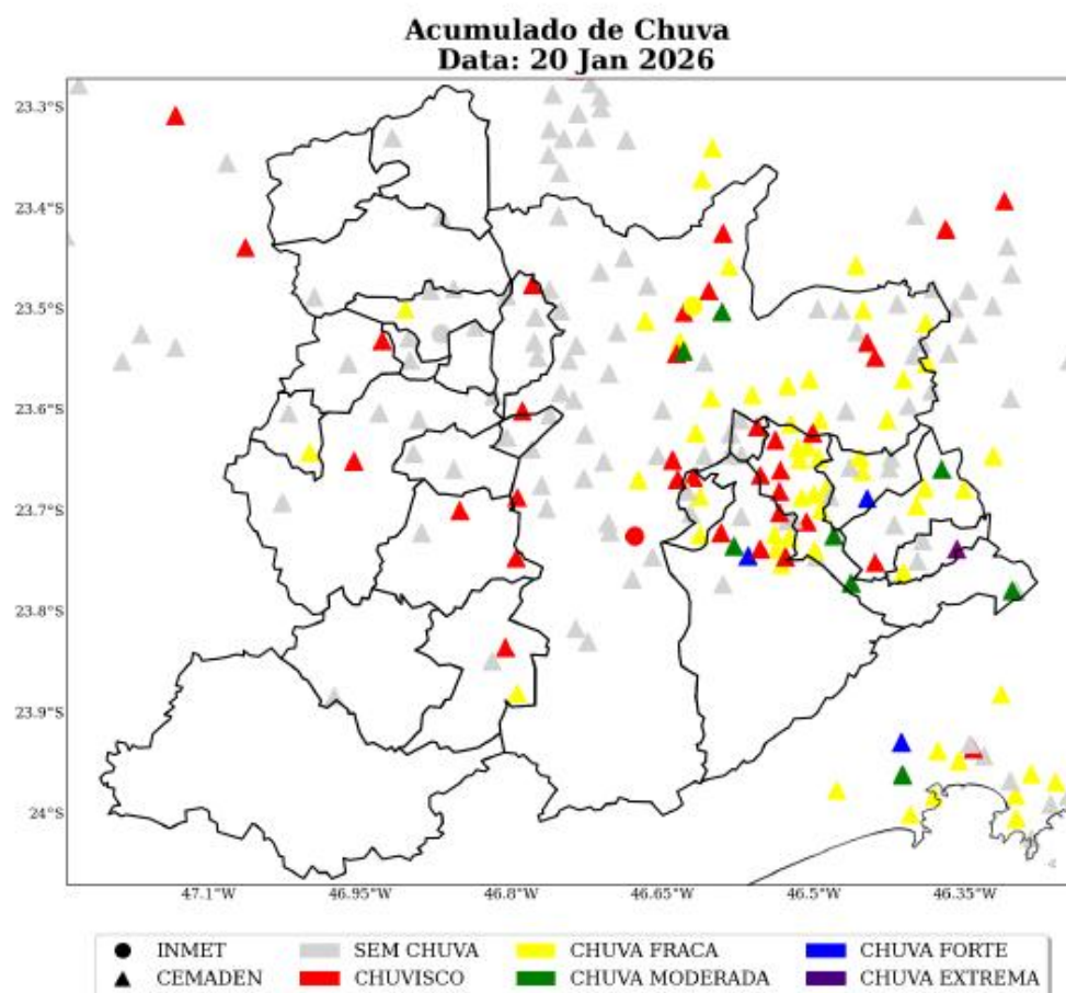
Figura 28: Acumulado diário de precipitação sobre a área de concessão da ENEL-SP para o dia 20 de Janeiro, baseado nas estações meteorológicas do INMET e CEMADEN.
