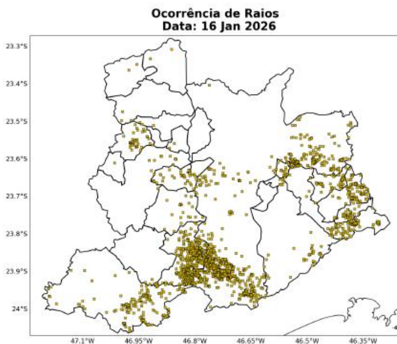
Figura 15: Ocorrências de descargas atmosféricas nuvem-solo detectadas pelo sistema Earth Networks para o dia 16 de Janeiro sobre a área de concessão da ENEL-SP.
