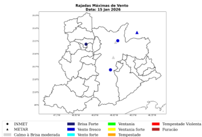
Figura 33: Máxima rajada de vento diária sobre a área de concessão da ENEL-SP para o dia 15 de Janeiro, baseado nas estações meteorológicas do INMET.
