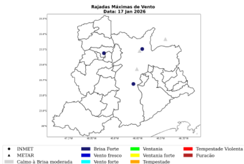
Figura 35: Máxima rajada de vento diária sobre a área de concessão da ENEL-SP para o dia 17 de Janeiro, baseado nas estações meteorológicas do INMET.
