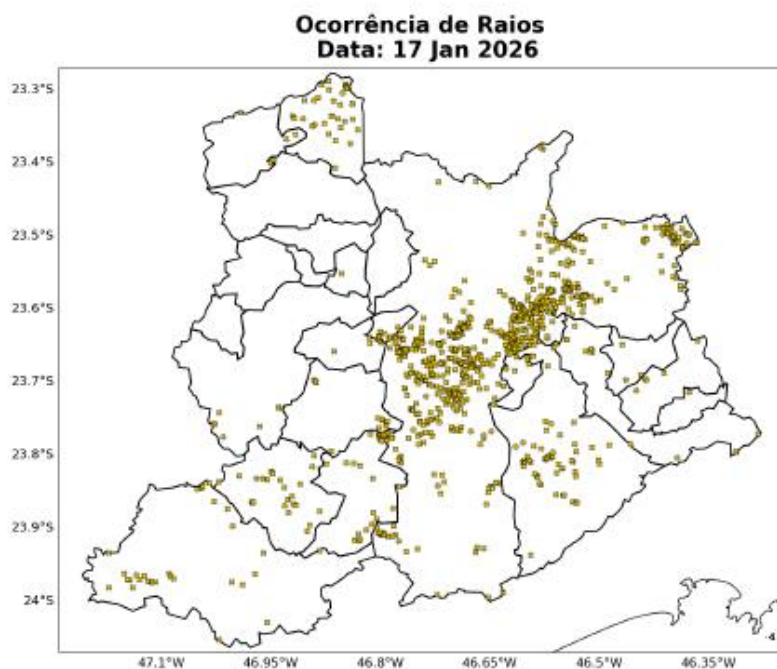
Figura 16: Ocorrências de descargas atmosféricas nuvem-solo detectadas pelo sistema Earth Networks para o dia 17 de Janeiro sobre a área de concessão da ENEL-SP.
