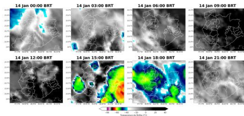
Figura 4: Imagens realçadas do satélite GOES-19 das 00 BRT até 21 BRT (a cada 3 horas) para o dia 14 de Janeiro.
