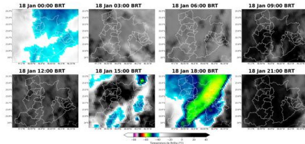
Figura 8: Imagens realçadas do satélite GOES-19 das 00 BRT até 21 BRT (a cada 3 horas) para o dia 18 de Janeiro.
