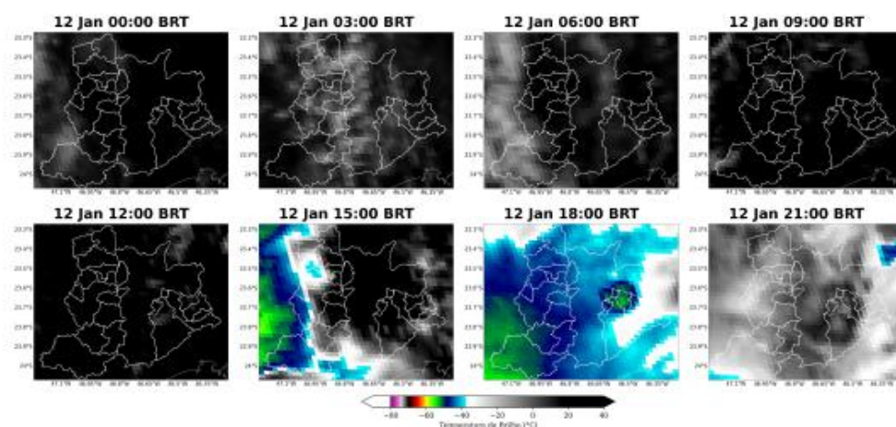
Figura 2: Imagens realçadas do satélite GOES-19 das 00 BRT até 21 BRT (a cada 3 horas) para o dia 12 de Janeiro.
