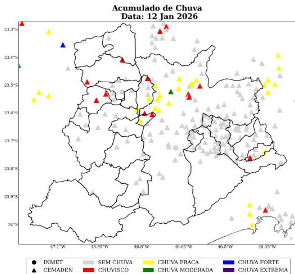
Figura 20: Acumulado diário de precipitação sobre a área de concessão da ENEL-SP para o dia 12 de Janeiro, baseado nas estações meteorológicas do INMET e CEMADEN.
