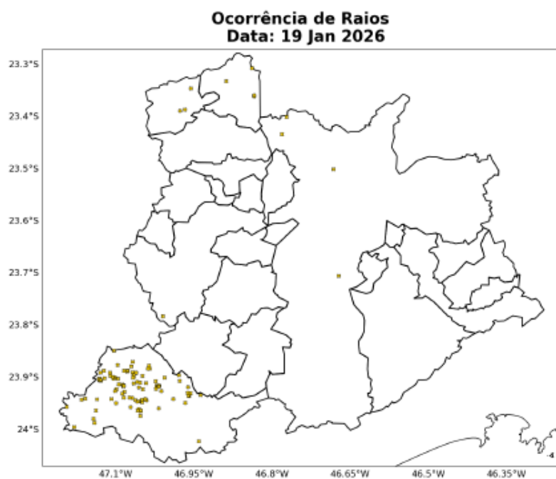
Figura 18: Ocorrências de descargas atmosféricas nuvem-solo detectadas pelo sistema Earth Networks para o dia 19 de Janeiro sobre a área de concessão da ENEL-SP.
