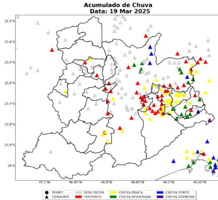
Figura 6: Acumulado diário de precipitação sobre a área de concessão da ENEL-SP para o dia 19 de Março, baseado nas estações meteorológicas do INMET e CEMADEN.
