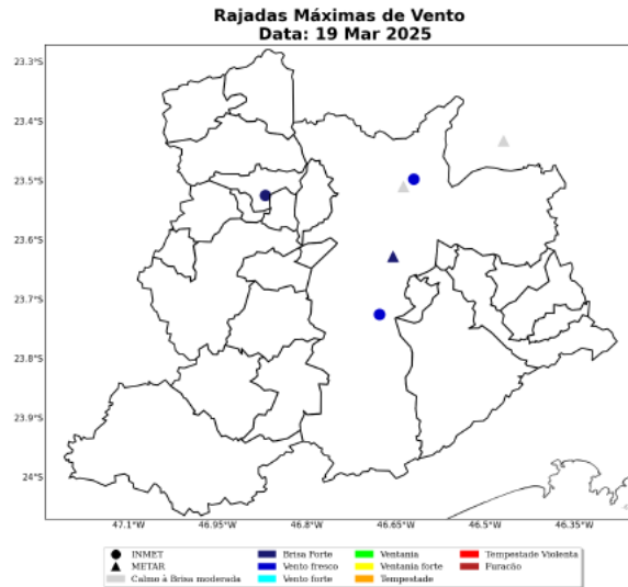
Figura 9: Máxima rajada de vento diária sobre a área de concessão da ENEL-SP para o dia 19 de Março, baseado nas estações meteorológicas do INMET.
