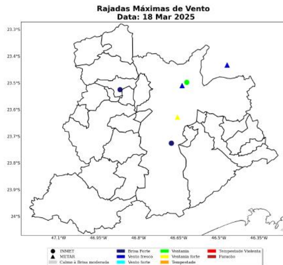
Figura 8: Máxima rajada de vento diária sobre a área de concessão da ENEL-SP para o dia 18 de Março, baseado nas estações meteorológicas do INMET.
