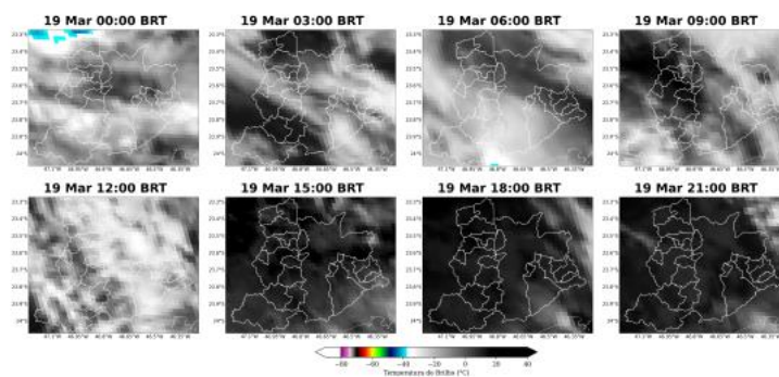
Figura 3: Imagens realçadas do satélite GOES-16 das 00 BRT até 21 BRT (a cada 3 horas) para o dia 19 de Março.
