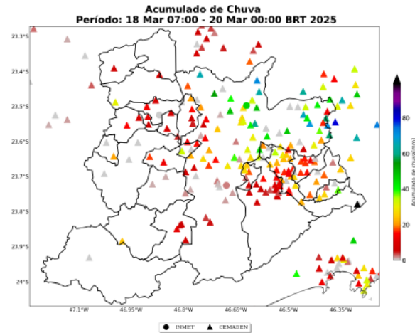
Figura 7: Acumulado de precipitação sobre o estado de São Paulo para o período do evento (dias 18 a 19 de Março de 2025), baseado nas estações meteorológicas do INMET e CEMADEN.
