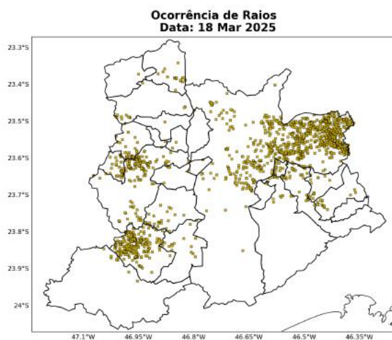
Figura 4: Ocorrências de descargas atmosféricas nuvem-solo detectadas pelo sistema Earth Networks para o dia 18 de Março sobre a área de concessão da ENEL-SP.
