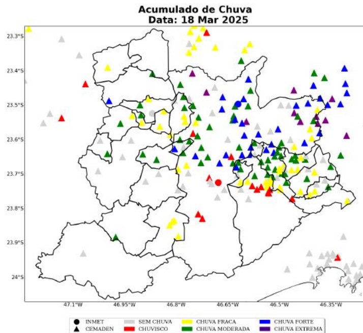
Figura 5: Acumulado diário de precipitação sobre a área de concessão da ENEL-SP para o dia 18 de Março, baseado nas estações meteorológicas do INMET e CEMADEN.
