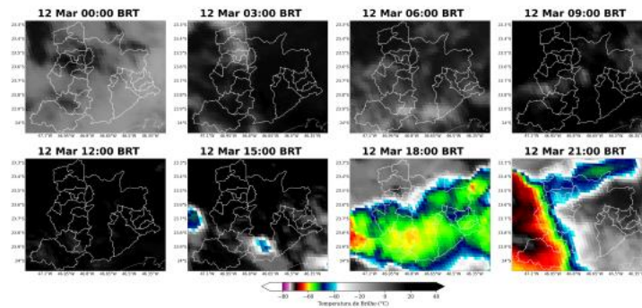
Figura 3: Imagens realçadas do satélite GOES-16 das 00 BRT até 21BRT (a cada 3 horas) para o dia 12 de Março.
