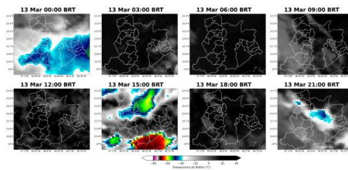
Figura 4: Imagens realçadas do satélite GOES-16 das 00 BRT até 21BRT (a cada 3 horas) para o dia 13 de Março.
