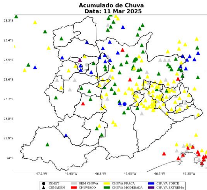
Figura 8: Acumulado diário de precipitação sobre a área de concessão da ENEL-SP para o dia 11 de Março, baseado nas estações meteorológicas do INMET e CEMADEN.
