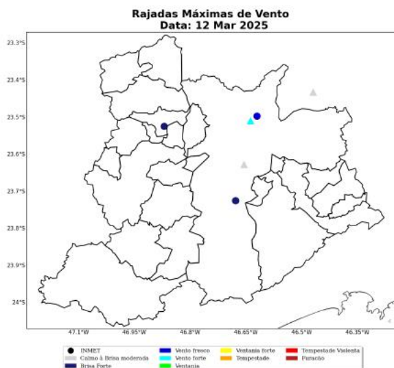
Figura 13: Máxima rajada de vento diária sobre a área de concessão da ENEL-SP para o dia 12 de Março, baseado nas estações meteorológicas do INMET.
