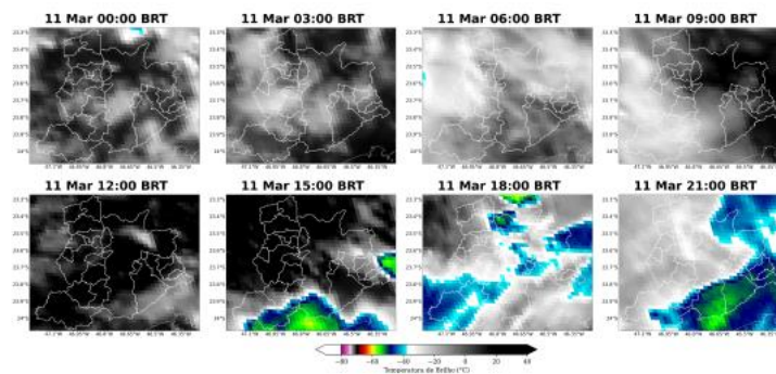
Figura 2: Imagens realçadas do satélite GOES-16 das 00 BRT até 21 BRT (a cada 3 horas) para o dia 11 de Março.
