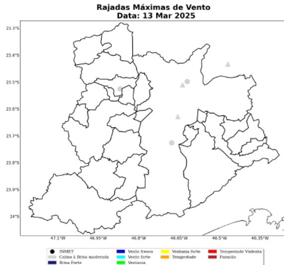
Figura 14: Máxima rajada de vento diária sobre a área de concessão da ENEL-SP para o dia 13 de Março, baseado nas estações meteorológicas do INMET.
