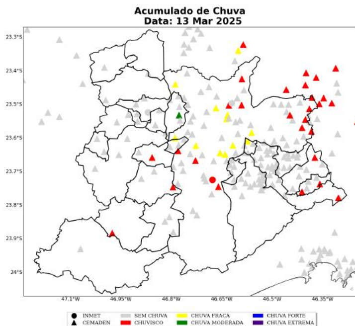
Figura 10: Acumulado diário de precipitação sobre a área de concessão da ENEL-SP para o dia 13 de Março, baseado nas estações meteorológicas do INMET e CEMADEN.
