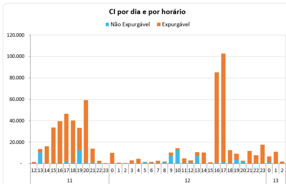
Figura 6 – CI por dia e por Horário
