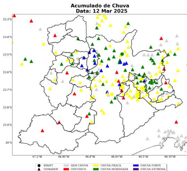
Figura 9: Acumulado diário de precipitação sobre a área de concessão da ENEL-SP para o dia 12 de Março, baseado nas estações meteorológicas do INMET e CEMADEN.
