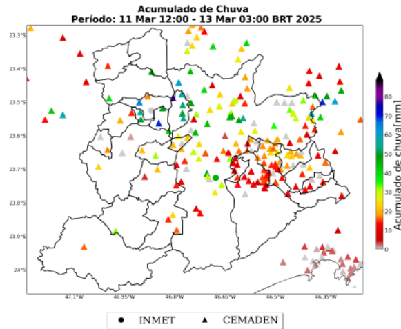
Figura 11: Acumulado de precipitação sobre o estado de São Paulo para o período do evento (dias 11 a 13 de Março de 2025), baseado nas estações meteorológicas do INMET e CEMADEN.
