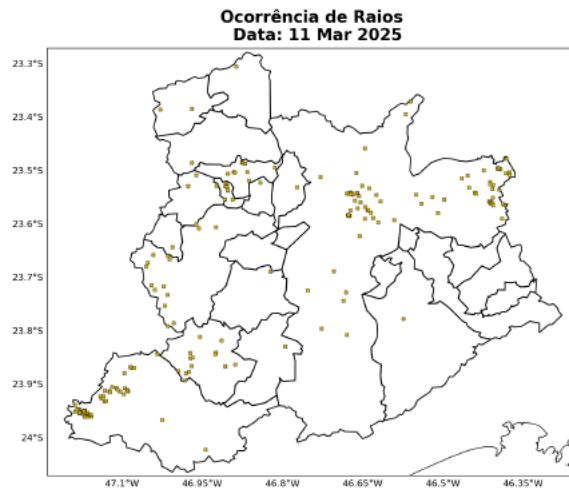
Figura 5: Ocorrências de descargas atmosféricas nuvem-solo detectadas pelo sistema Earth Networks para o dia 11 de Março sobre a área de concessão da ENEL-SP.
