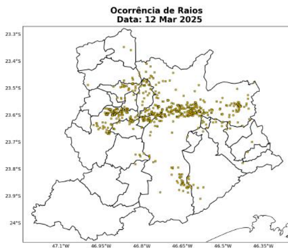
Figura 6: Ocorrências de descargas atmosféricas nuvem-solo detectadas pelo sistema Earth Networks para o dia 12 de Março sobre a área de concessão da ENEL-SP.
