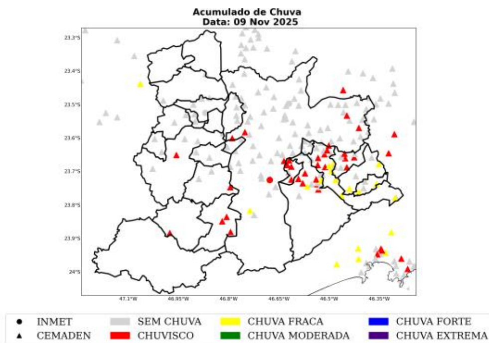
Figura 6: Acumulado diário de precipitação sobre a área de concessão da ENEL-SP para o dia 09 de Novembro, baseado nas estações meteorológicas do INMET e CEMADEN.
