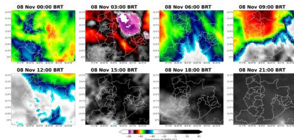
Figura 2: Imagens realçadas do satélite GOES-19 das 00 BRT até 21 BRT (a cada 3 horas) para o dia 08 de Novembro.
