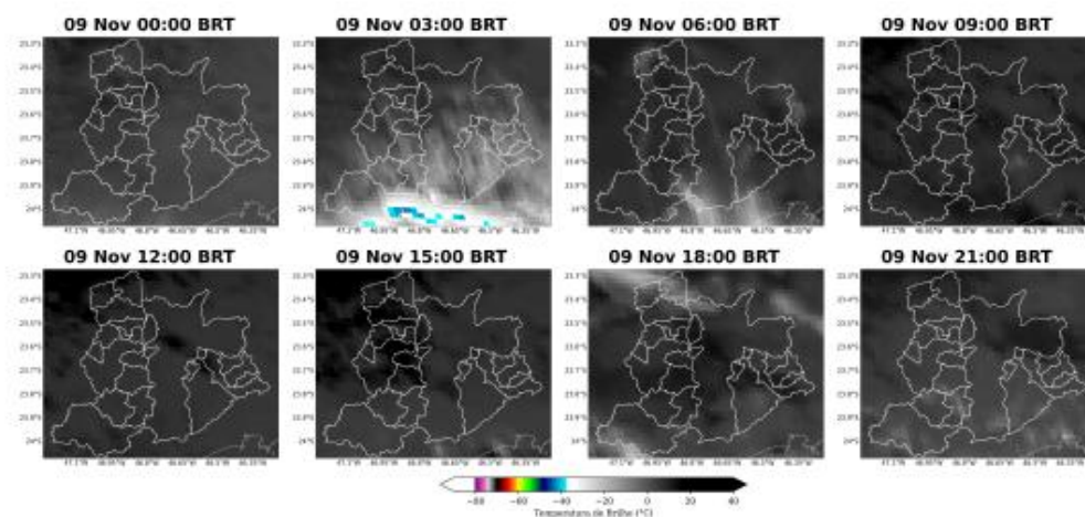
Figura 3: Imagens realçadas do satélite GOES-19 das 00 BRT até 21 BRT (a cada 3 horas) para o dia 09 de Novembro.
