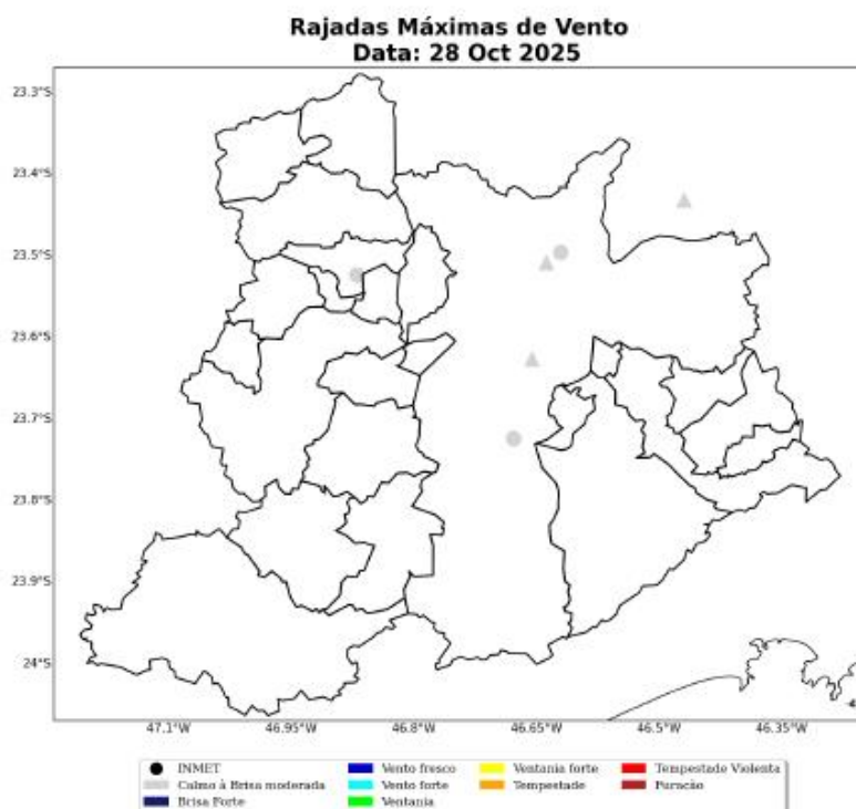
Figura 8: Máxima rajada de vento diária sobre a área de concessão da ENEL-SP para o dia 28 de Outubro, baseado nas estações meteorológicas do INMET.
