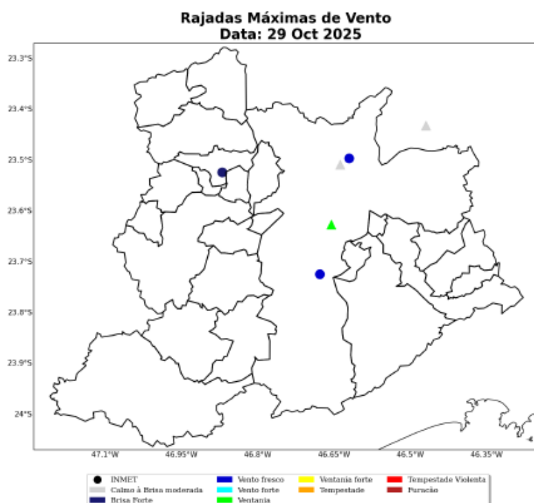
Figura 9: Máxima rajada de vento diária sobre a área de concessão da ENEL-SP para o dia 29 de Outubro, baseado nas estações meteorológicas do INMET.
