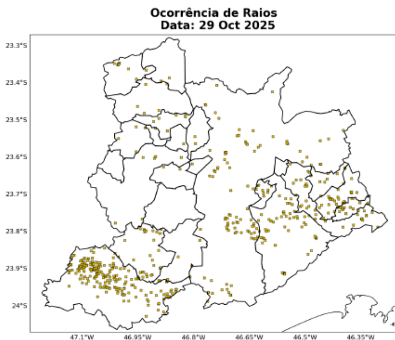
Figura 4: Ocorrências de descargas atmosféricas nuvem-solo detectadas pelo sistema Earth Networks para o dia 28 de Outubro sobre a área de concessão da ENEL-SP.
