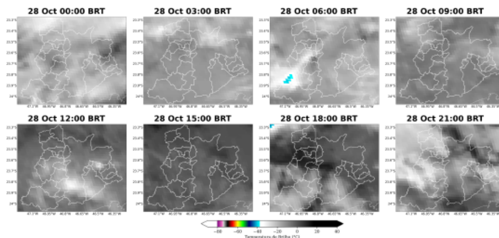
Figura 2: Imagens realçadas do satélite GOES-19 das 00 BRT até 21 BRT (a cada 3 horas) para o dia 28 de Outubro.
