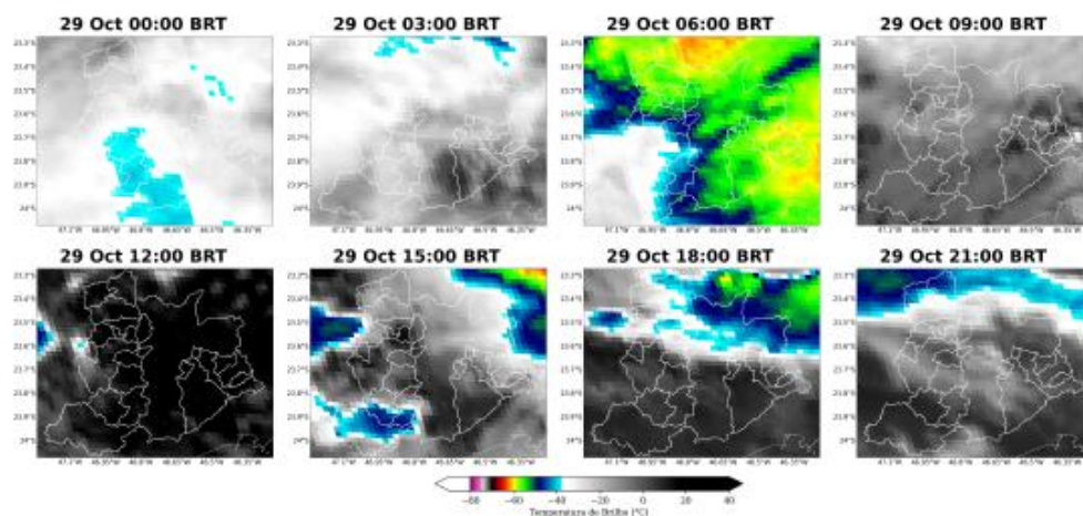
Figura 3: Imagens realçadas do satélite GOES-19 das 00 BRT até 21 BRT (a cada 3 horas) para o dia 29 de Outubro.
