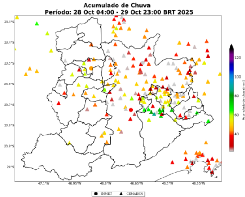
Figura 7: Acumulado de precipitação sobre a área de concessão da ENEL-SP para o período do evento (dias 28 a 29 de Outubro de 2025), baseado nas estações meteorológicas do INMET e CEMADEN.
