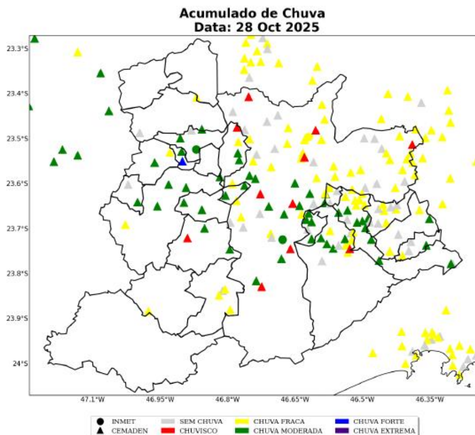
Figura 5: Acumulado diário de precipitação sobre a área de concessão da ENEL-SP para o dia 28 de Outubro, baseado nas estações meteorológicas do INMET e CEMADEN.
