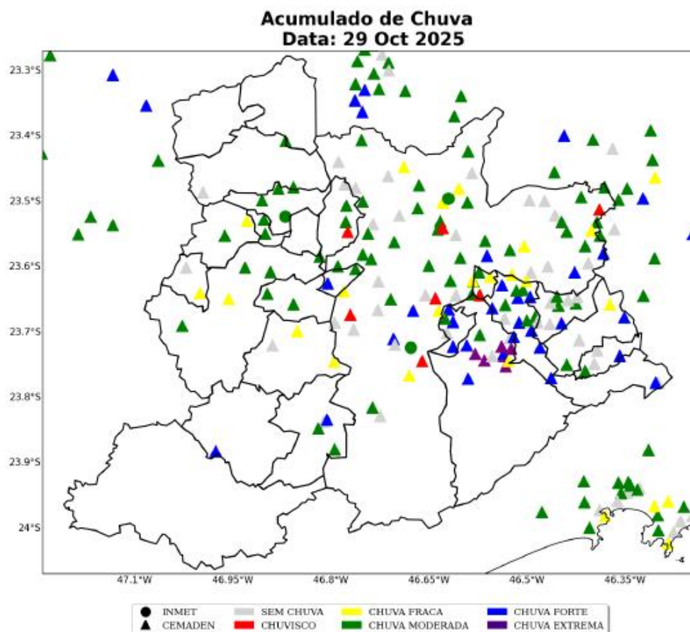
Figura 6: Acumulado diário de precipitação sobre a área de concessão da ENEL-SP para o dia 29 de Outubro, baseado nas estações meteorológicas do INMET e CEMADEN.
