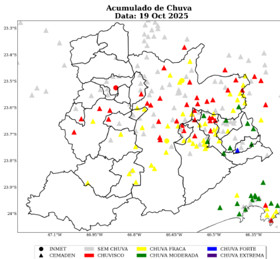
Figura 7: Acumulado diário de precipitação sobre a área de concessão da ENEL-SP para o dia 19 de Outubro, baseado nas estações meteorológicas do INMET e CEMADEN.
