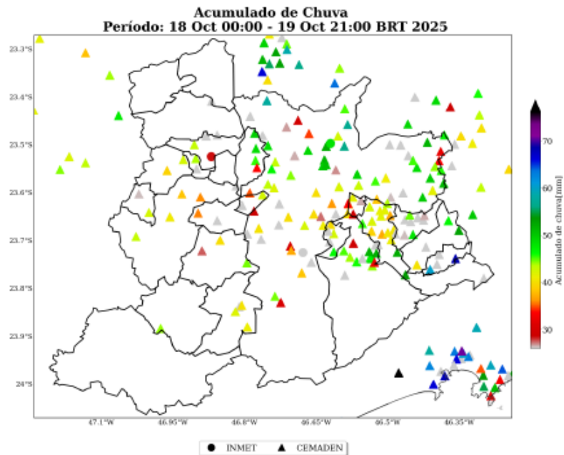
Figura 8: Acumulado de precipitação sobre o estado de São Paulo para o período do evento (dias 18 a 19 de Outubro de 2025), baseado nas estações meteorológicas do INMET e CEMADEN.
