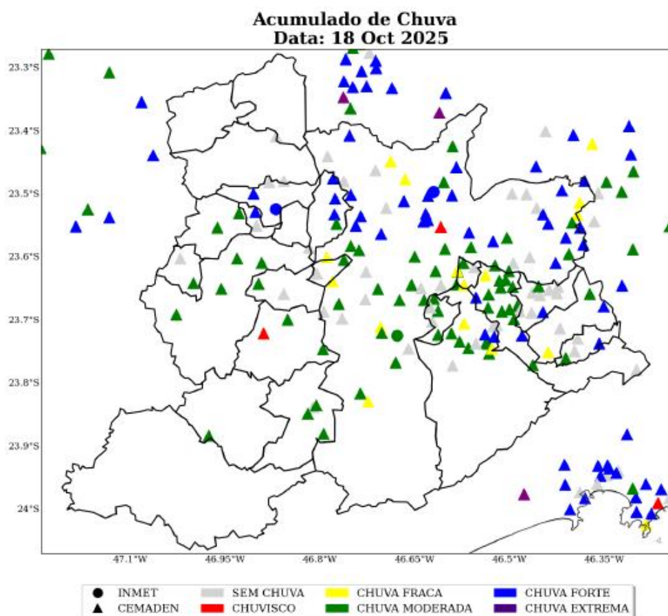
Figura 6: Acumulado diário de precipitação sobre a área de concessão da ENEL-SP para o dia 18 de Outubro, baseado nas estações meteorológicas do INMET e CEMADEN.
