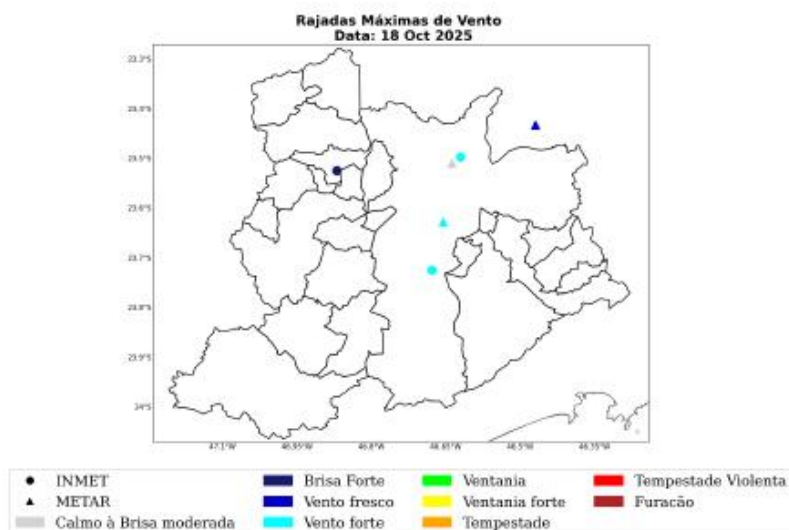
Figura 9: Máxima rajada de vento diária sobre a área de concessão da ENEL-SP para o dia 18 de Outubro, baseado nas estações meteorológicas do INMET.
