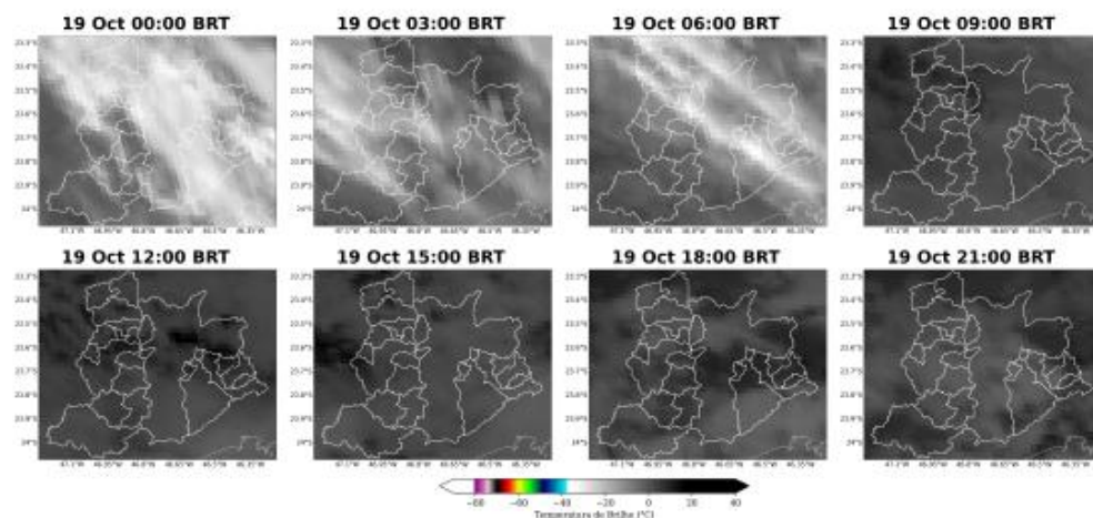
Figura 3: Imagens realçadas do satélite GOES-19 das 00 BRT até 21 BRT (a cada 3 horas) para o dia 19 de Outubro.
