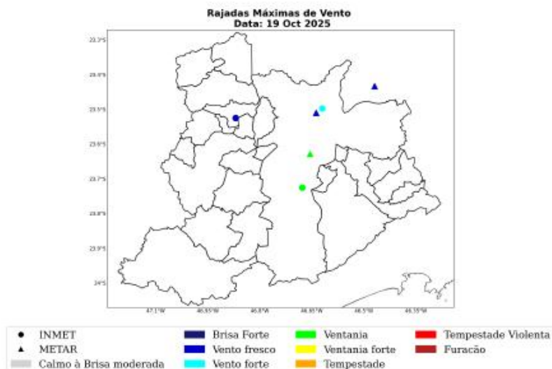
Figura 10: Máxima rajada de vento diária sobre a área de concessão da ENEL-SP para o dia 19 de Outubro, baseado nas estações meteorológicas do INMET.
