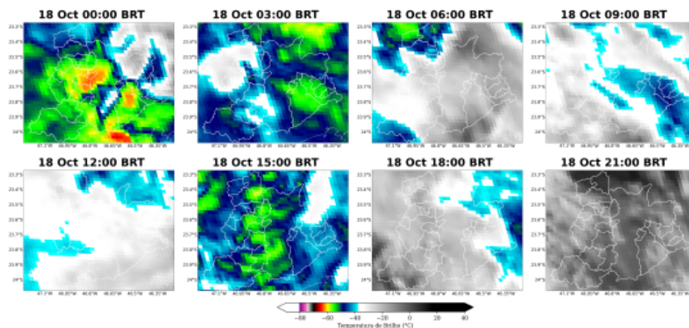
Figura 2: Imagens realçadas do satélite GOES-19 das 00 BRT até 21 BRT (a cada 3 horas) para o dia 18 de Outubro.
