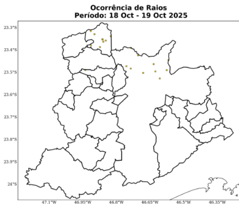
Figura 5: Ocorrências de descargas atmosféricas nuvem-solo detectadas pelo sistema Earth Networks para o período de 18 a 19 de Outubro de 2025 sobre a área de concessão da ENEL-SP.
