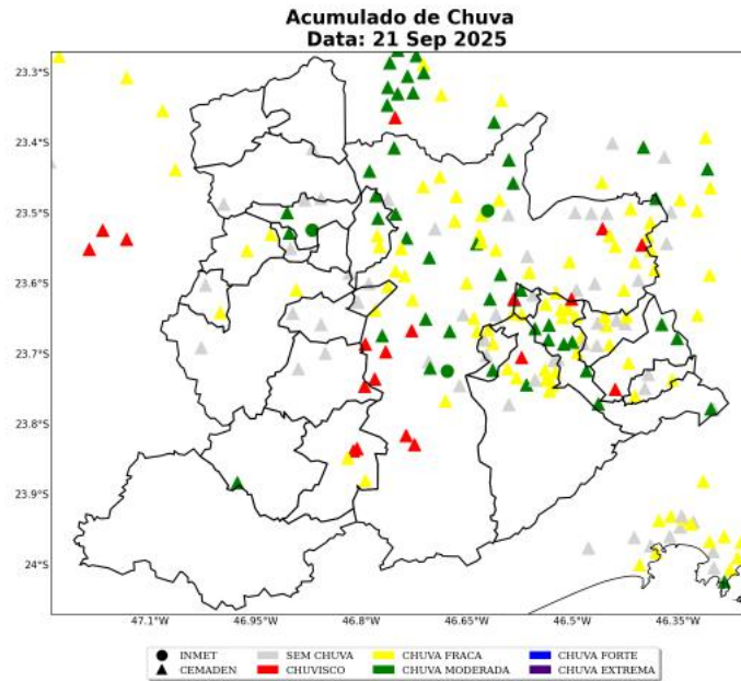
Figura 7: Acumulado diário de precipitação sobre a área de concessão da ENEL-SP para o dia 21 de Setembro, baseado nas estações meteorológicas do INMET e CEMADEN.
