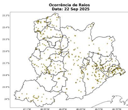
Figura 5: Ocorrências de descargas atmosféricas nuvem-solo detectadas pelo sistema Earth Networks para o dia 22 de Setembro sobre a área de concessão da ENEL-SP.
