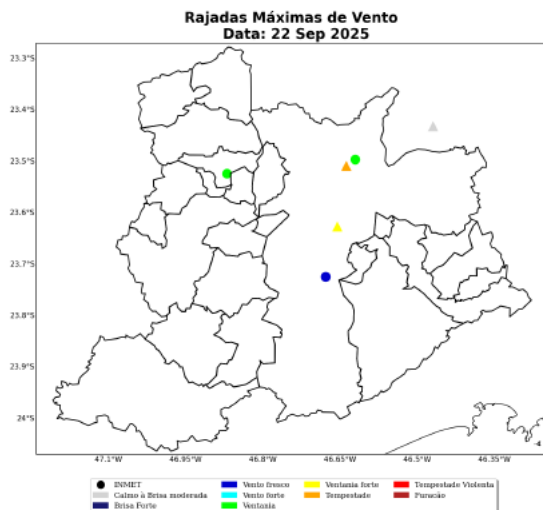
Figura 11: Máxima rajada de vento diária sobre a área de concessão da ENEL-SP para o dia 22 de Setembro, baseado nas estações meteorológicas do INMET.
