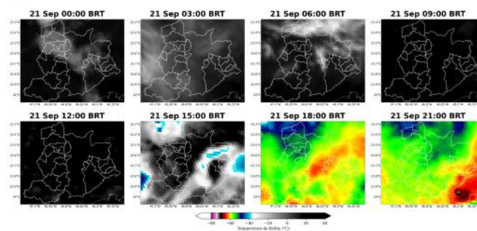
Figura 2: Imagens realçadas do satélite GOES-19 das 00 BRT até 21 BRT (a cada 3 horas) para o dia 21 de Setembro.
