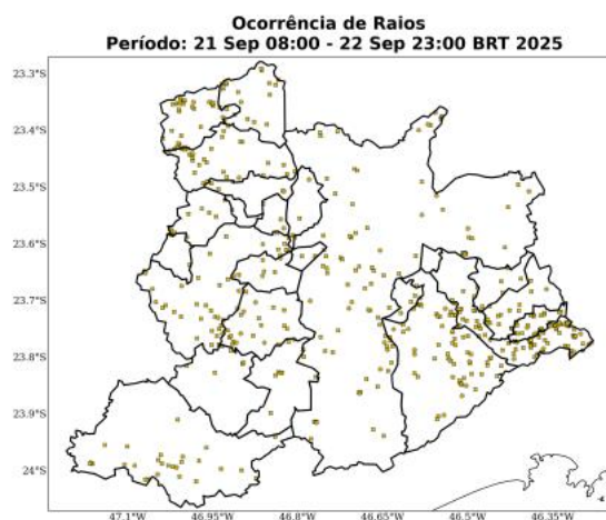
Figura 6: Ocorrências de descargas atmosféricas nuvem-solo detectadas pelo sistema Earth Networks para o período de 21 a 22 de Setembro de 2025 sobre a área de concessão da ENEL-SP.
