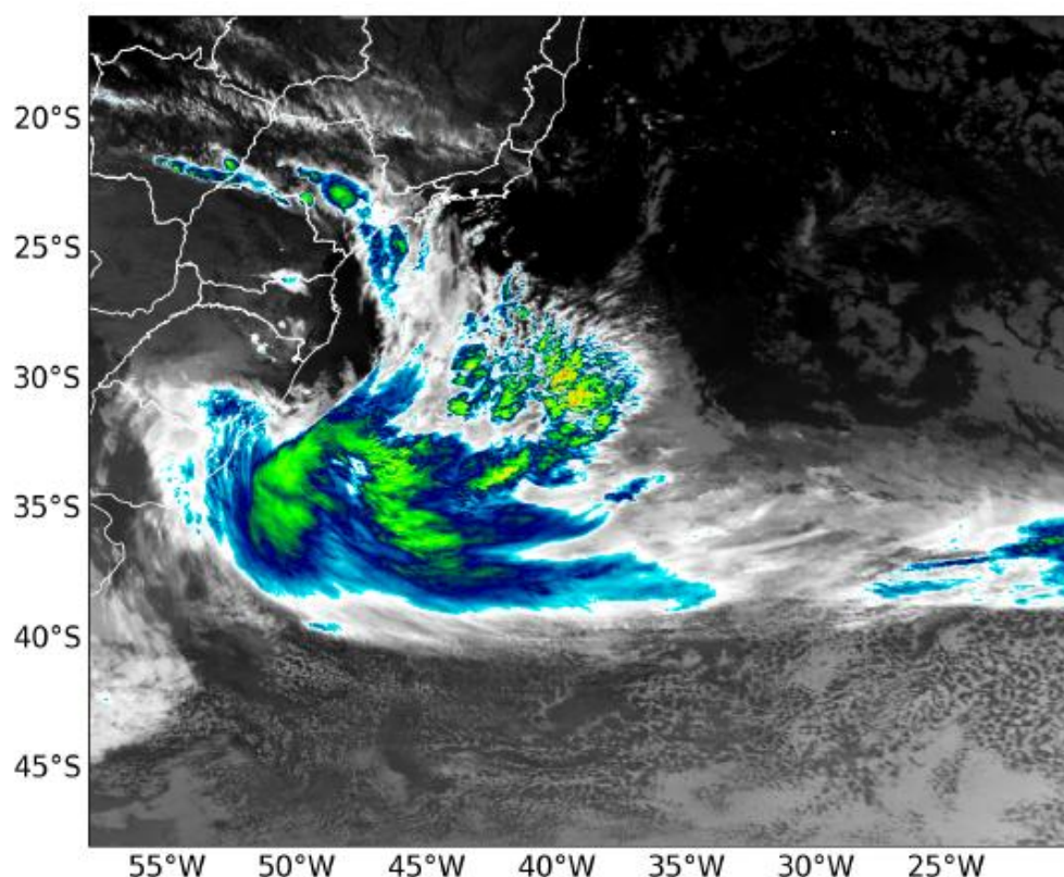
Figura 2: Imagem realçada do satélite GOES-19 das 06 BRT para o dia 28 de Julho.
