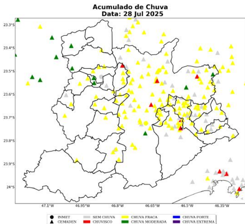
Figura 4: Acumulado diário de precipitação sobre a área de concessão da ENEL-SP para o dia 28 de Julho, baseado nas estações meteorológicas do INMET e CEMADEN.
