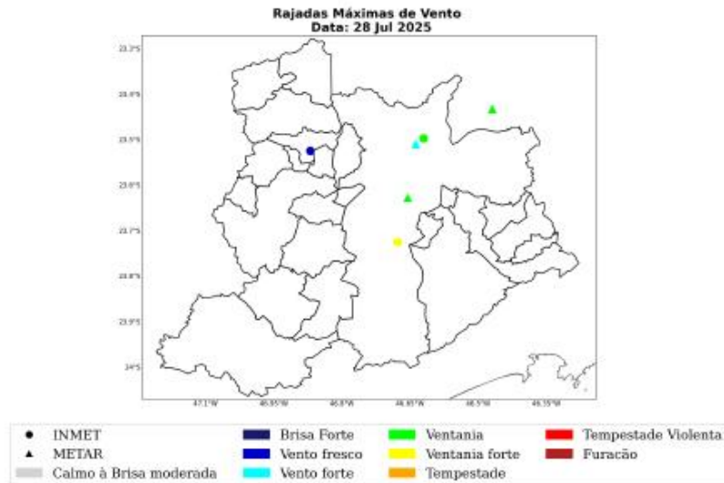
Figura 6: Máxima rajada de vento diária sobre a área de concessão da ENEL-SP para o dia 28 de Julho, baseado nas estações meteorológicas do INMET.
