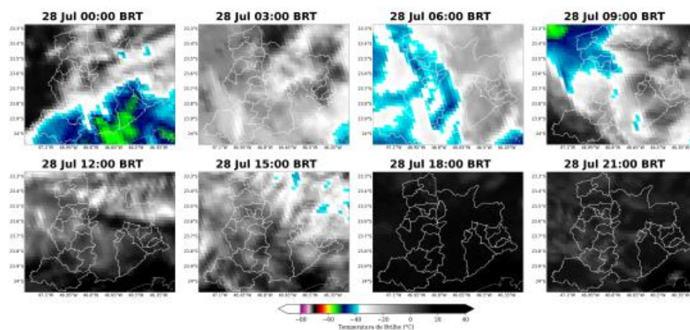
Figura 3: Imagens realçadas do satélite GOES-19 das 00 BRT até 21 BRT (a cada 3 horas) para o dia 28 de Julho.
