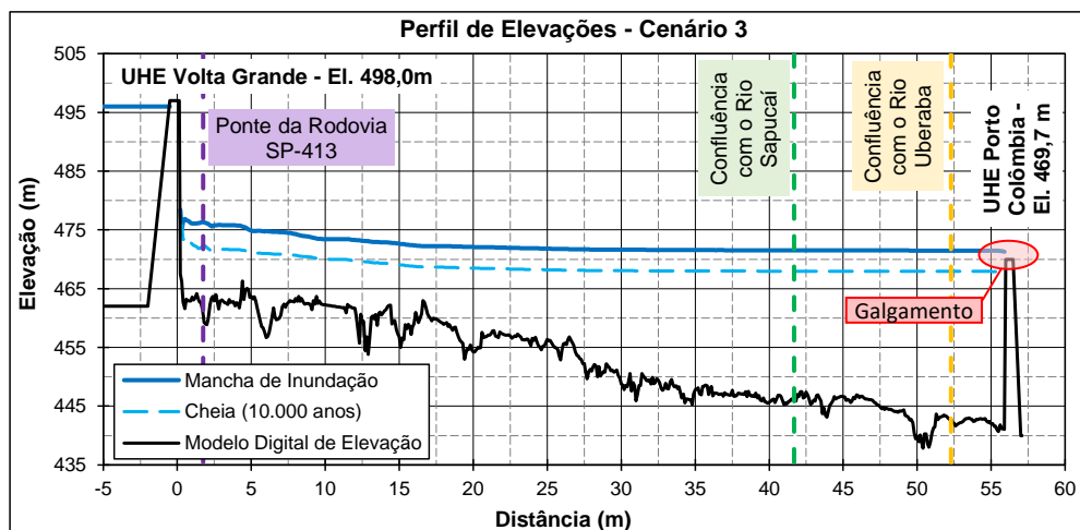
Figura 15 – Cenário 3: Elevações Máximas na Passagem da Onda
