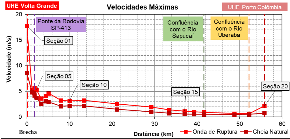
Figura 17 – Cenário 3: Velocidades Máximas na Passagem da Onda
