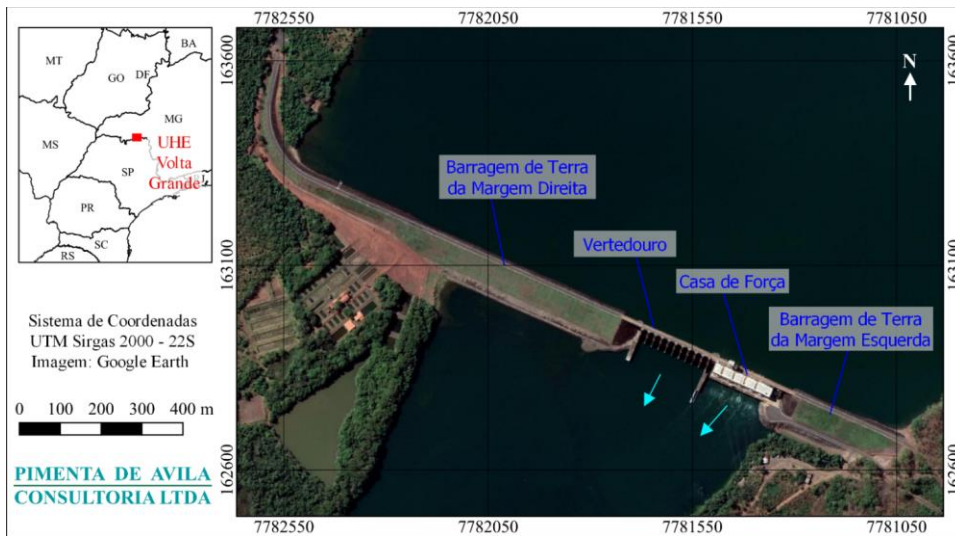
Figura 2 – Arranjo Geral da UHE Volta Grande
