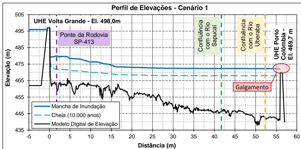
Figura 14 – Cenário 1: Elevações Máximas na Passagem da Onda
