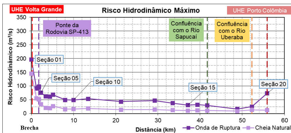
Figura 20 – Cenário 1: Risco Hidrodinâmico Máximo
