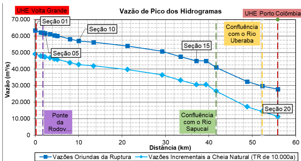
Figura 10 – Cenário 1: Hidrogramas ao Longo do Vale a Jusante
