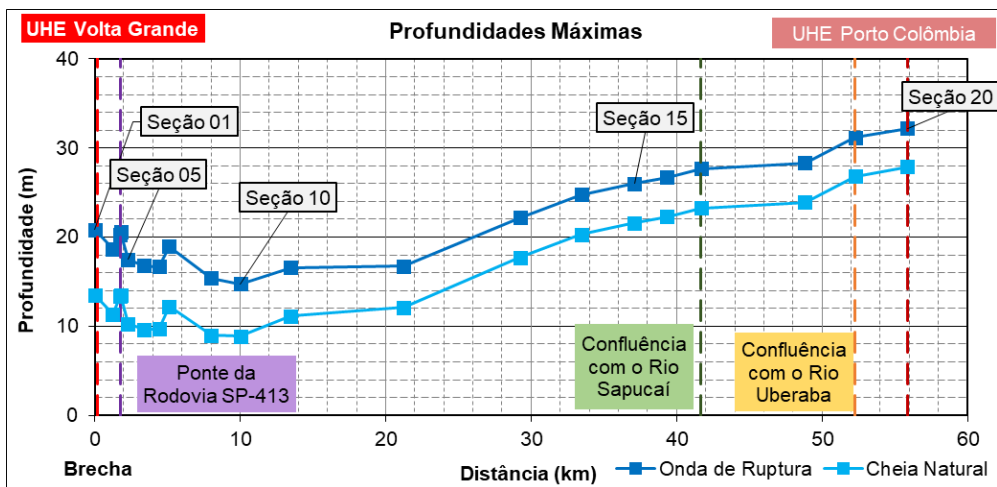
Figura 12 – Cenário 1: Profundidades Máximas na Passagem da Onda
