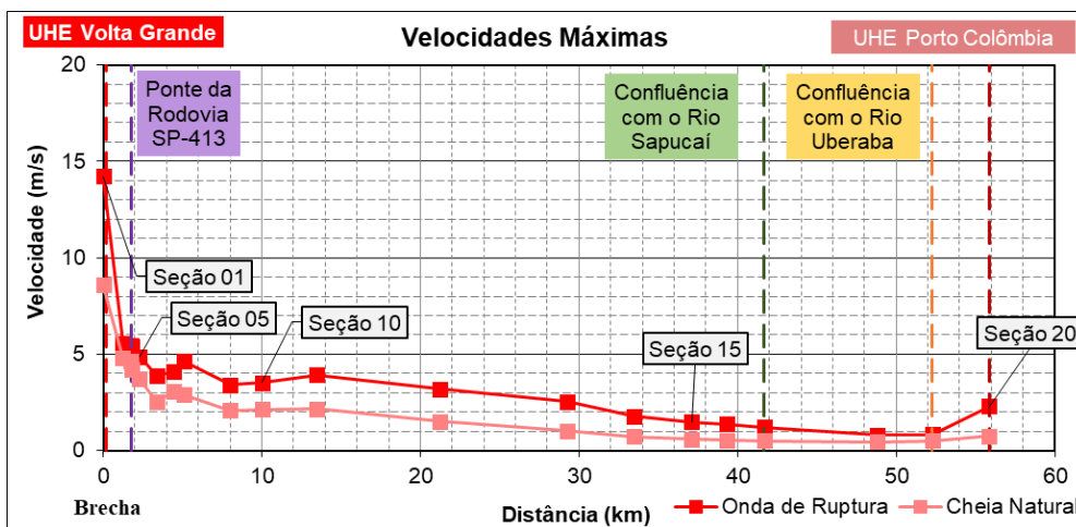
Figura 16 – Cenário 1: Velocidades Máximas na Passagem da Onda
