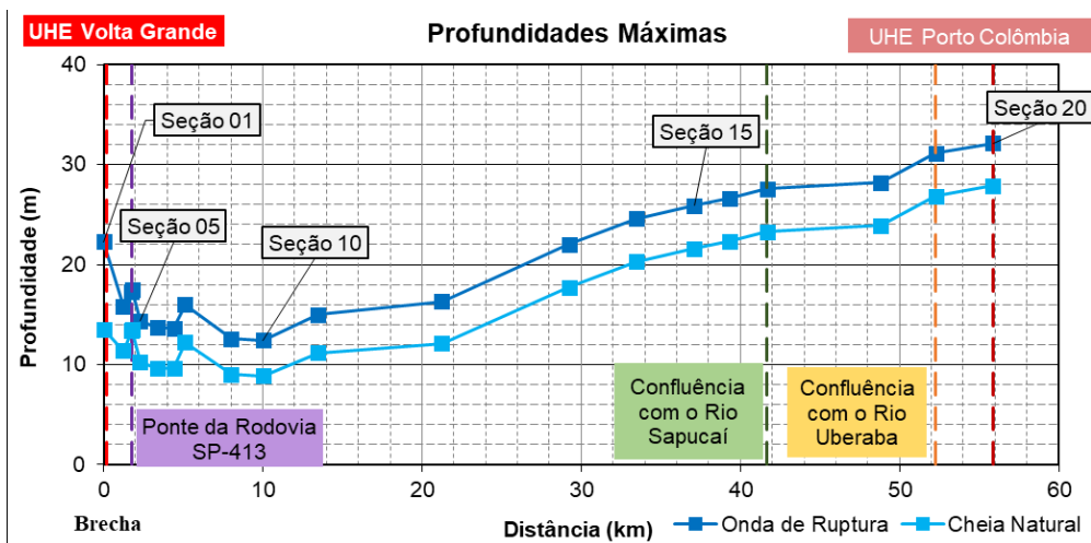
Figura 13 – Cenário 3: Profundidades Máximas na Passagem da Onda
