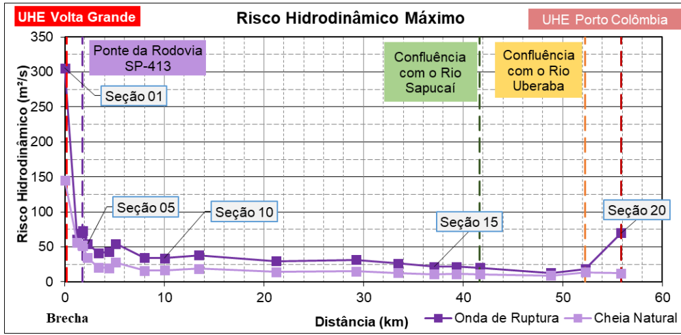
Figura 21 – Cenário 3: Risco Hidrodinâmico Máximo
