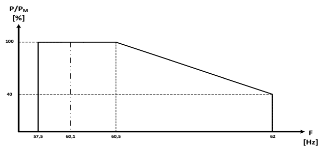
Figura 2 - Atenuação da potência injetada
