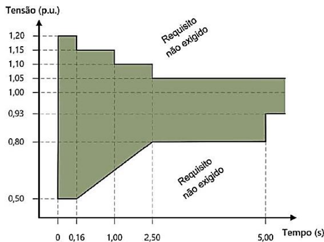
Gráfico 1 - Suportabilidade a subtensões e sobretensões dinâmicas no ponto de conexão
