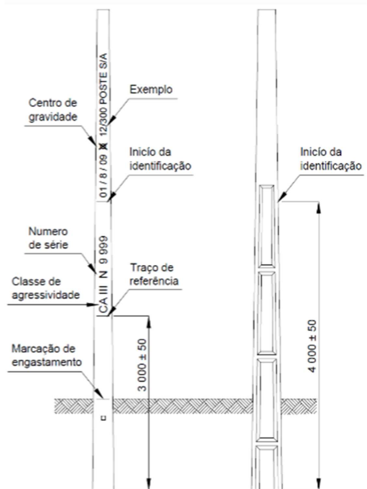
Figura 2 - Identificação no poste
