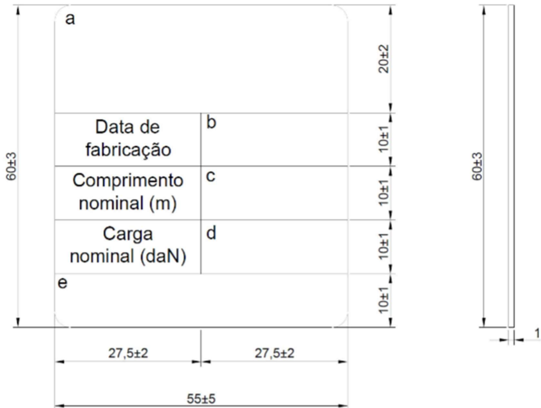
Figura 3 - Identificação na placa metálica
