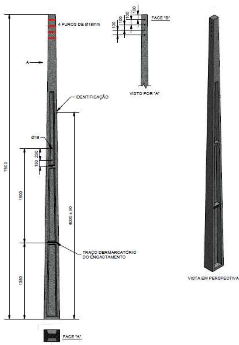
Figura 1 - Poste Duplo T
