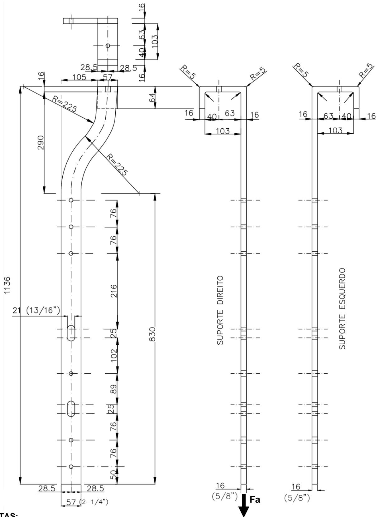
Figura 2 – Suporte de Transformador em Cruzeta - Tipo 2
