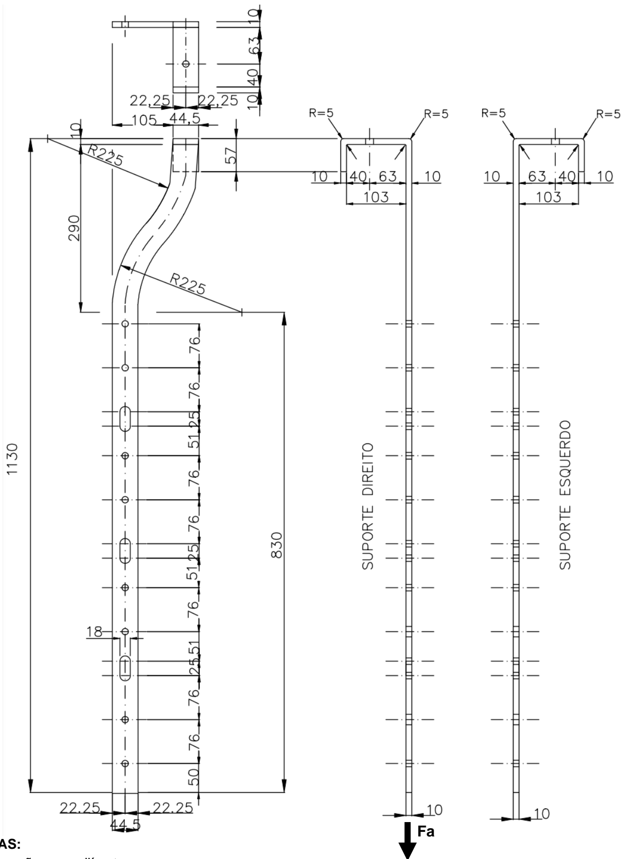
Figura 1 – Suporte de Transformador em Cruzeta - Tipo 1
