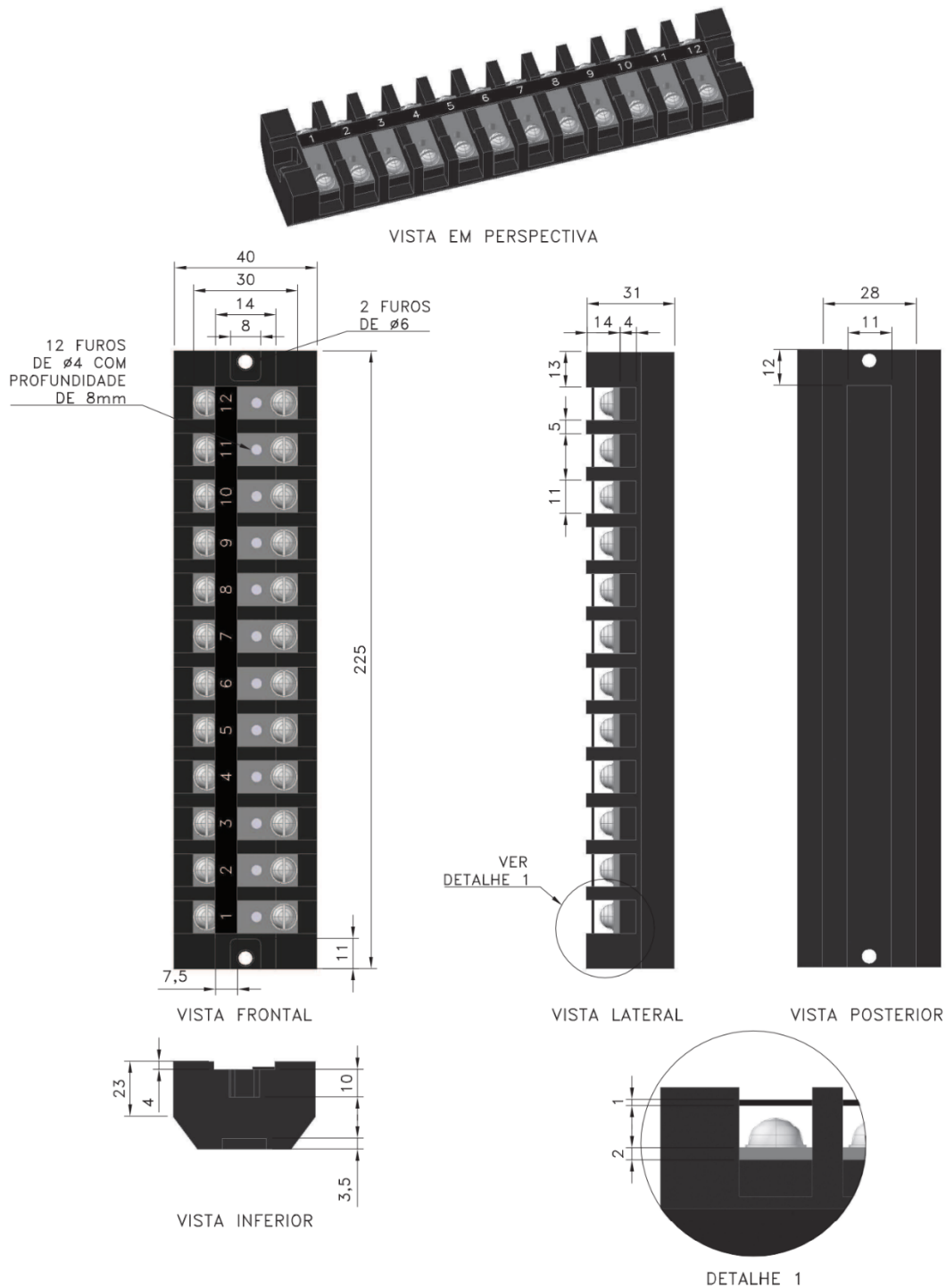
Figura 2 - Régua de bornes tipo 2 - 12 polos
