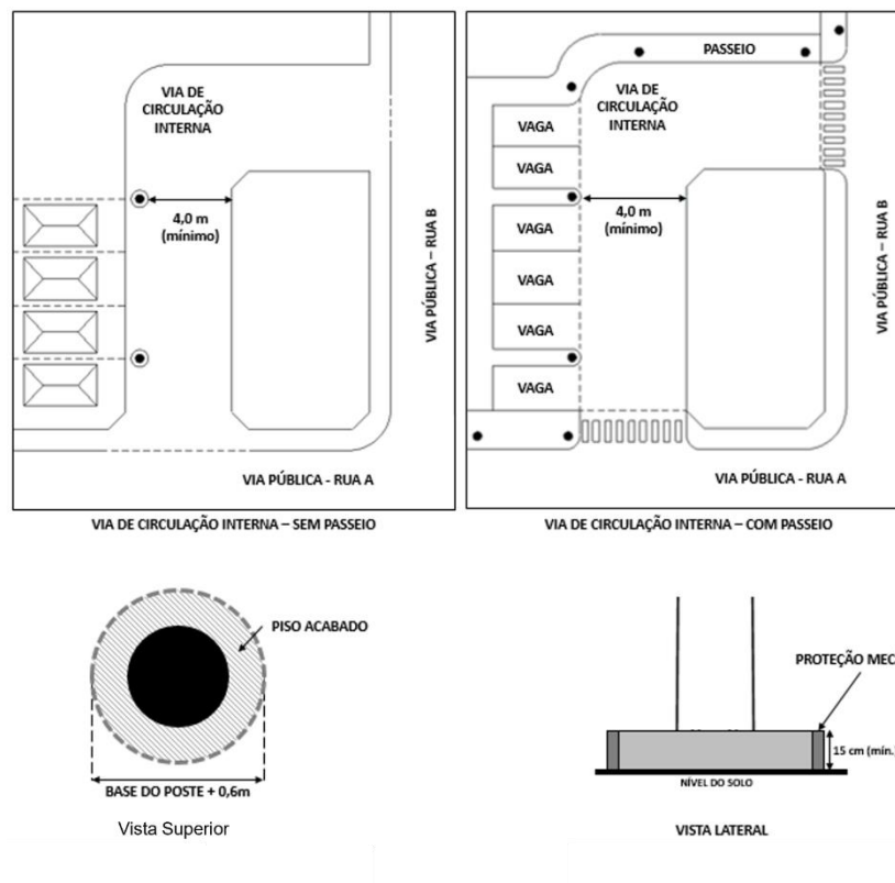
Figura 11 – Instalação de postes em empreendimentos particulares
