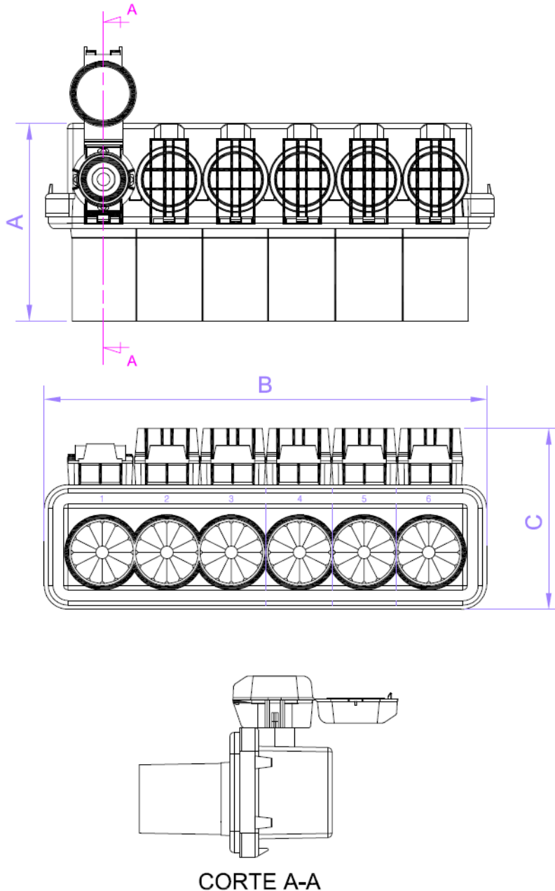
Figura 1 - Barramento modular isolado de 6 vias (exemplo)
