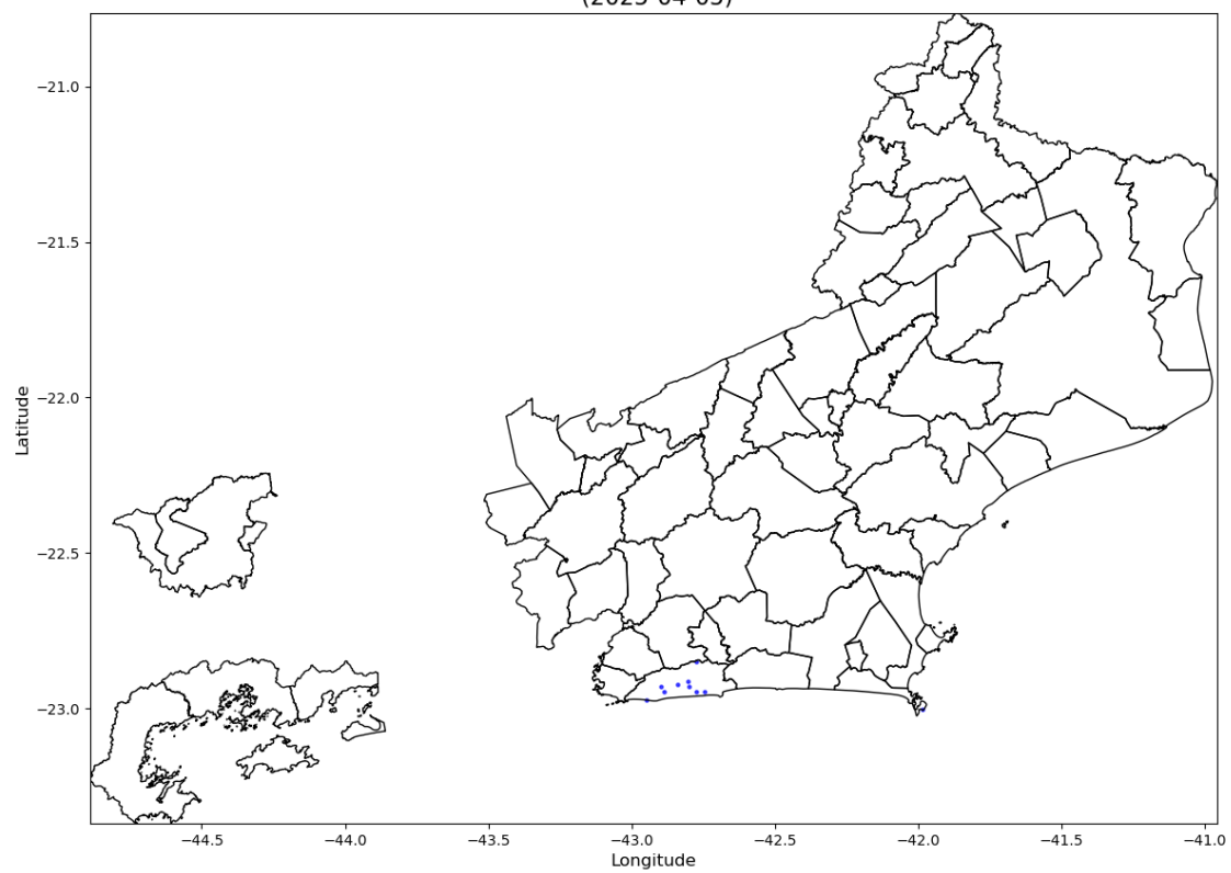
Número de Raios - 10 (2025-04-05)
