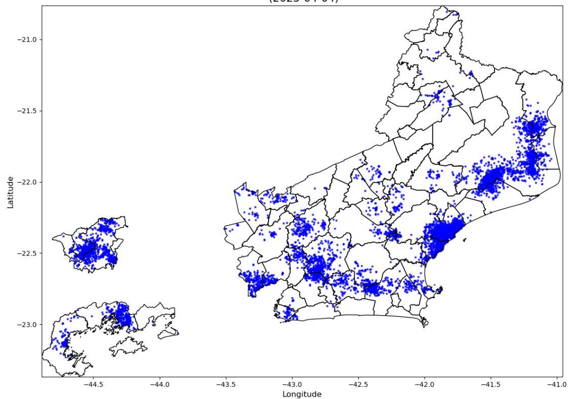
Número de Raios - 8370 (2025-04-04)
