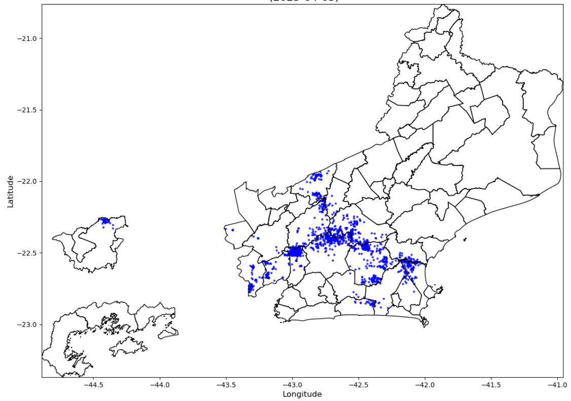
Número de Raios - 1513 (2025-04-03)
