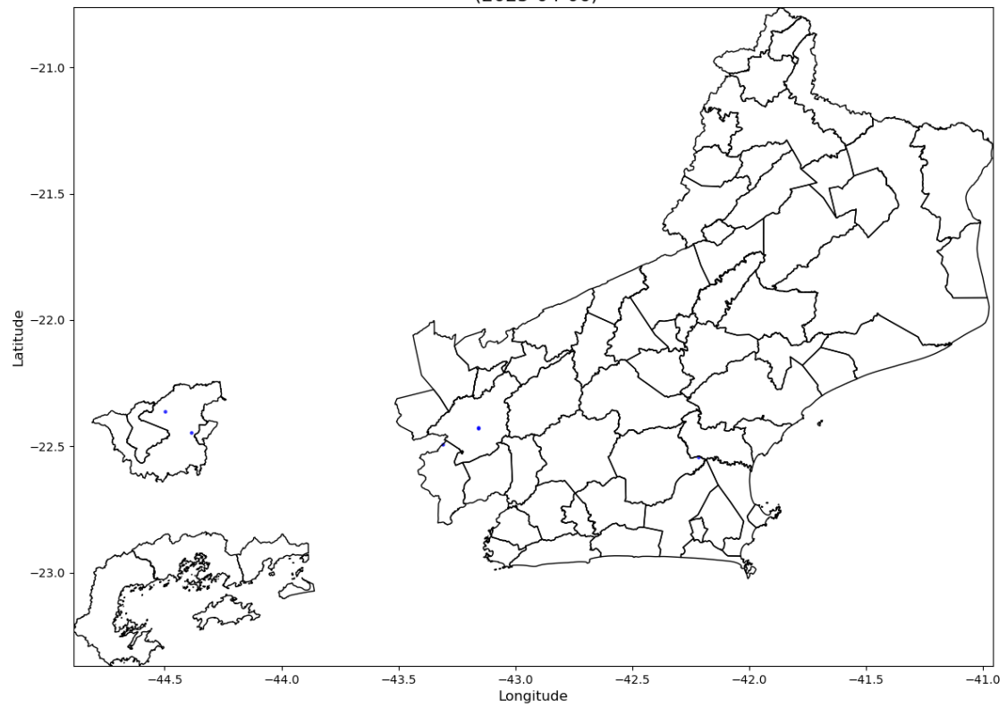
Número de Raios - 6 (2025-04-06)
