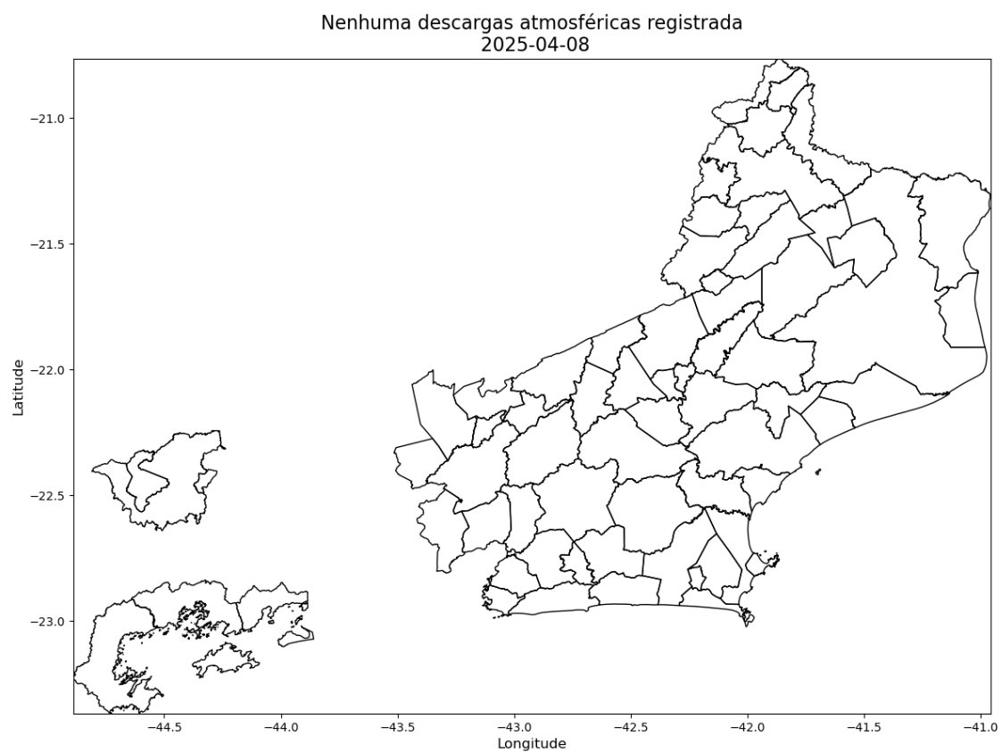
Figura 2 – Mapas de descargas atmosféricas para os dias 02 a 08/04.
