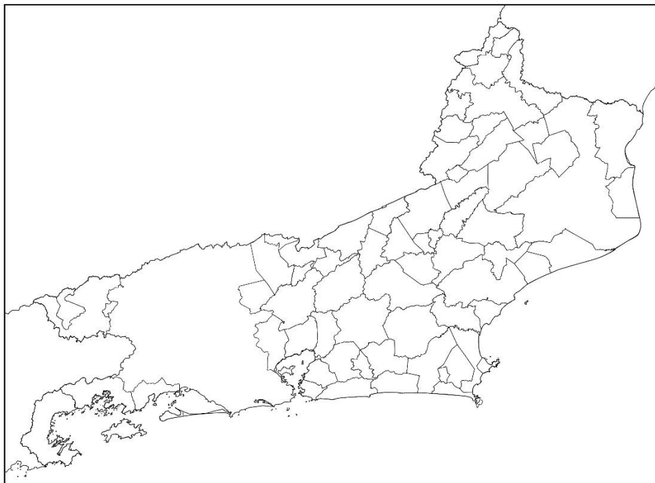
Mapa de Descargas Atmosféricas 2024-01-02
