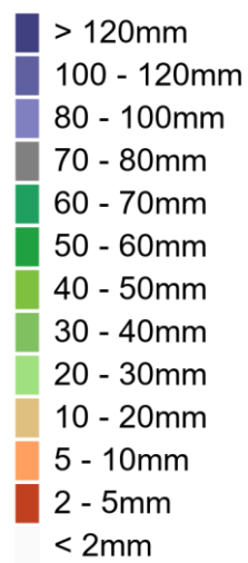
Figura 3 – Mapa de precipitação para os dias: (a) 02/01; (b) 03/01; (c) 04/01; (d) 05/01; e (e) 06/01.
