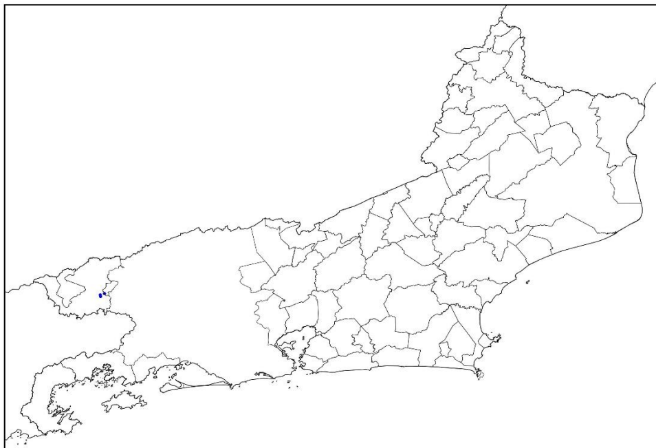
Mapa de Descargas Atmosféricas 2024-01-04
