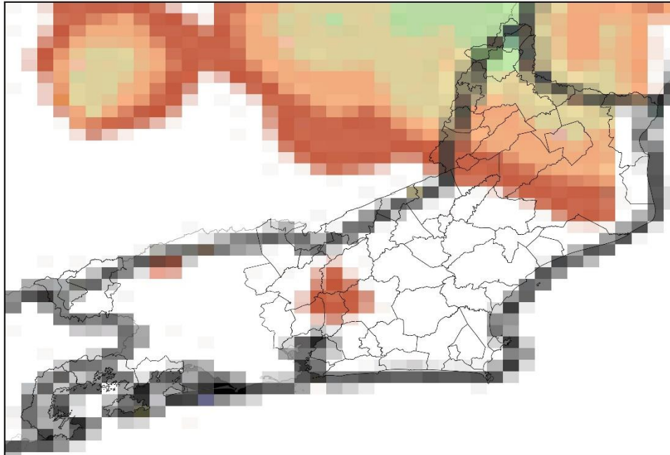
Mapa de Precipitação 2024-01-02
