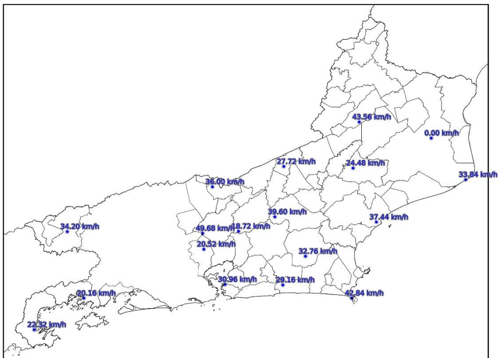
Mapa de Rajada Máxima 2024-01-05
