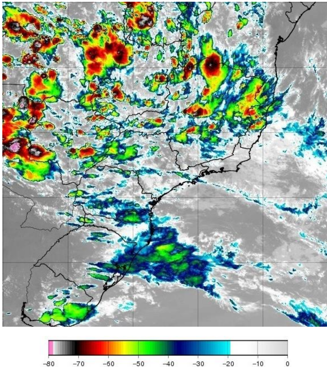
Figura 1 - Imagem de satélite no infravermelho com realce do satélite GOES-16 às 21:00 UT do dia 02/01/2024. As cores indicam diferentes temperaturas dos topos das nuvens.
