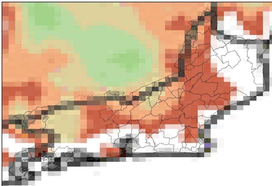
Mapa de Precipitação 2024-01-03
