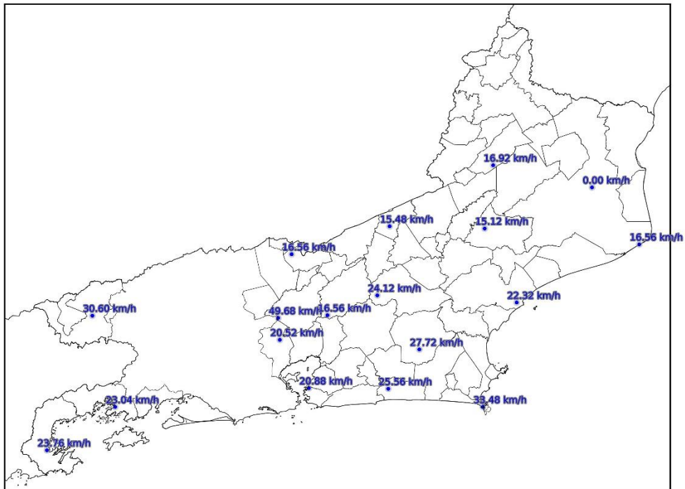
Mapa de Rajada Máxima 2024-01-02
