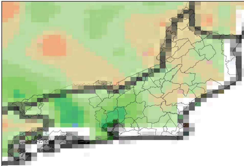
Mapa de Precipitação 2024-01-04
