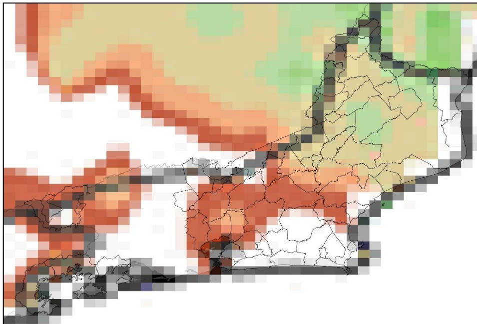
Mapa de Precipitação 2024-01-05
