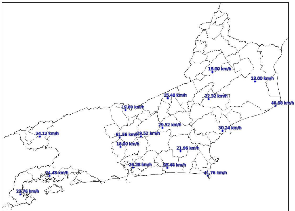
Mapa de Rajada Máxima 2024-01-03
