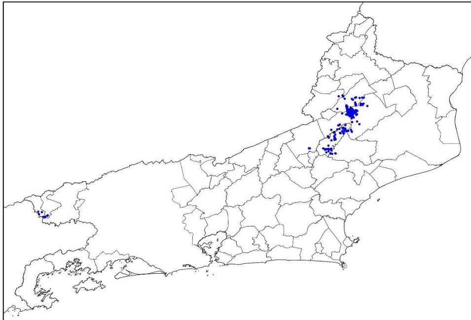
Mapa de Descargas Atmosféricas 2024-01-05
