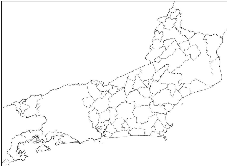
Mapa de Descargas Atmosféricas 2024-01-06
