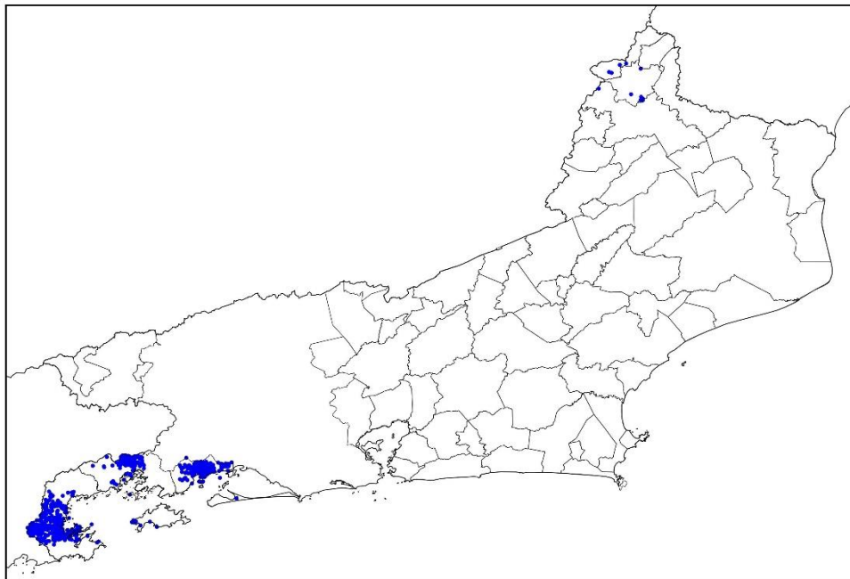
Mapa de Descargas Atmosféricas 2024-01-03
