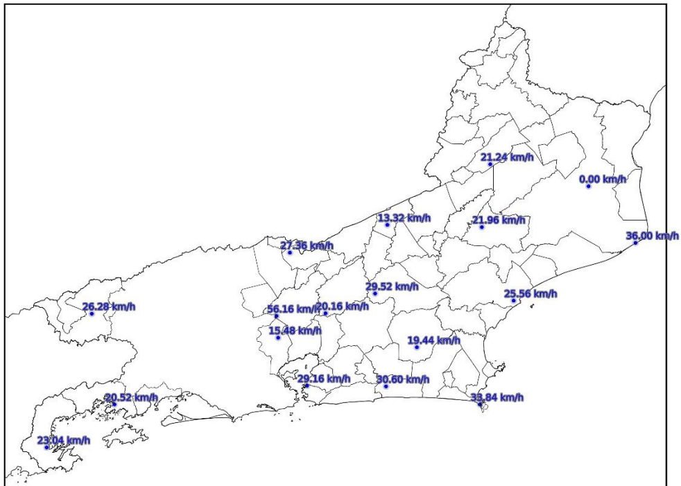
Mapa de Rajada Máxima 2024-01-04
