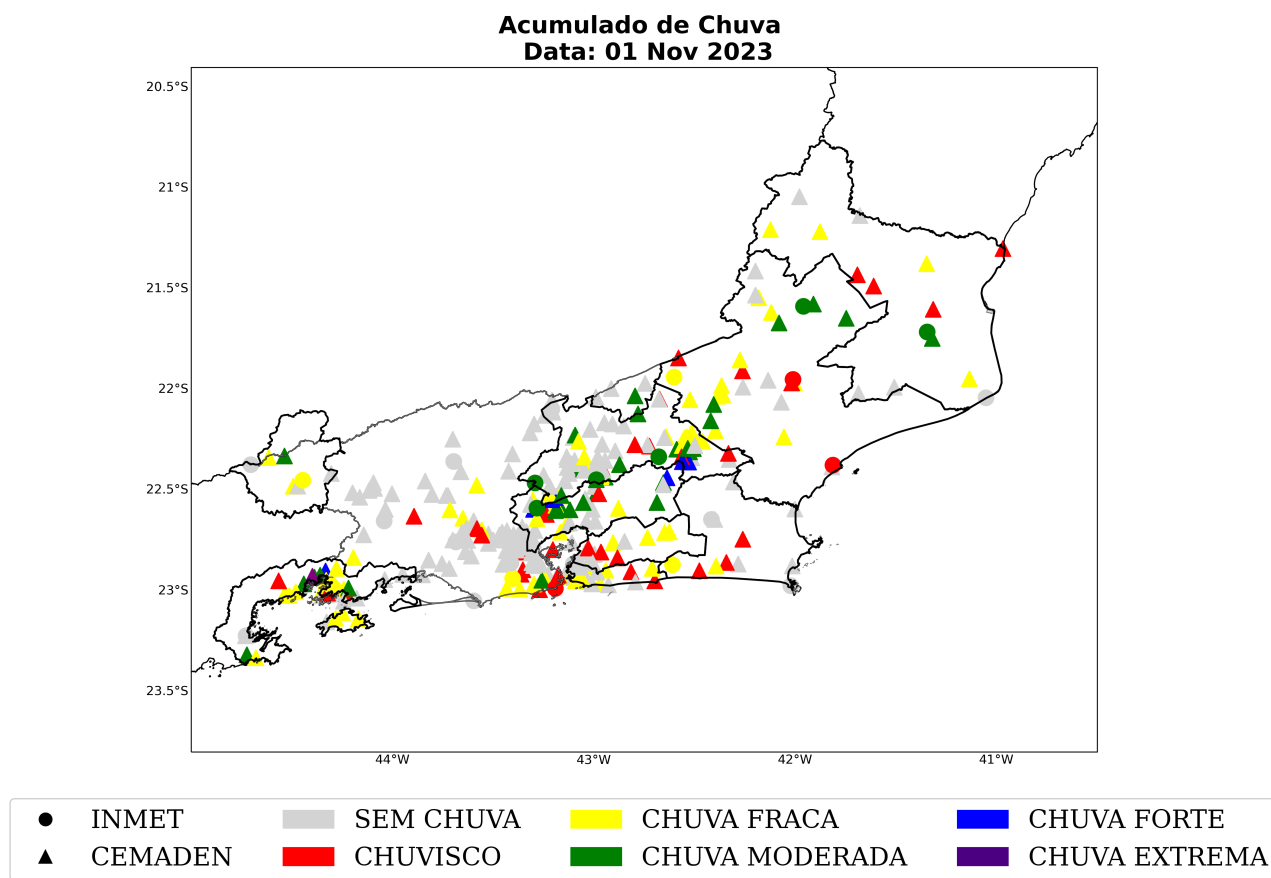
Figura 32: Acumulado diário de precipitação sobre a área de concessão da Enel-RJ para o dia 01 de novembro, baseado nas estações meteorológicas do INMET e CEMADEN.
