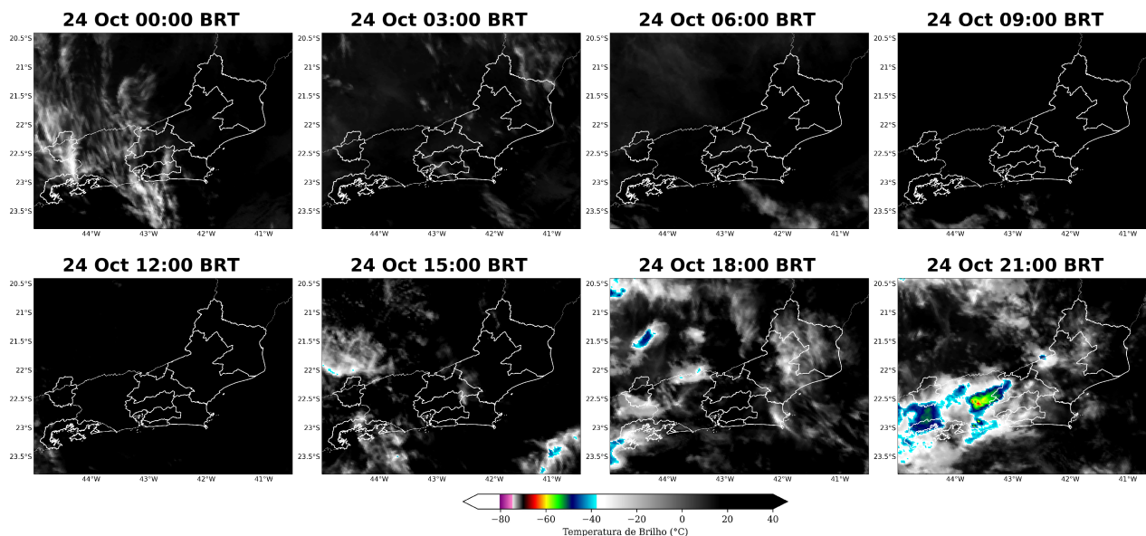
Figura 3: Imagens realçadas do satélite GOES-16 das 00 BRT até 21 BRT (a cada 3 horas) para o dia 24 de outubro.
