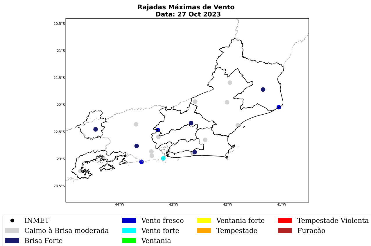
Figura 39: Máxima rajada de vento diária sobre a área de concessão da Enel-RJ para o dia 27 de outubro, baseado nas estações meteorológicas do INMET.
