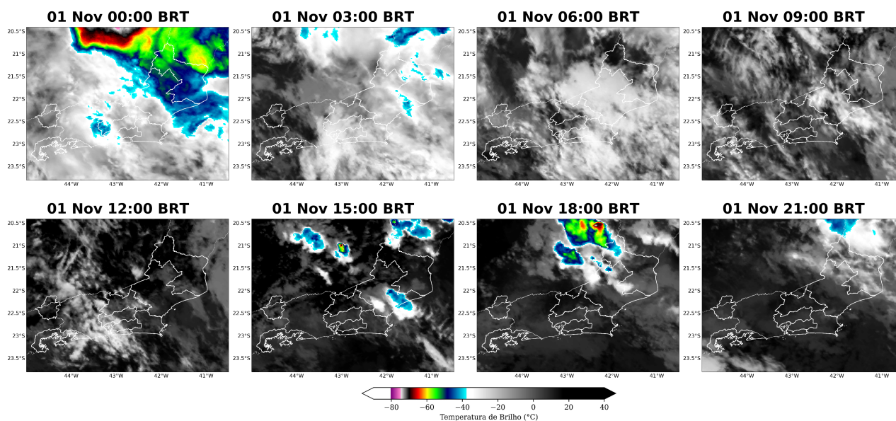
Figura 11: Imagens realçadas do satélite GOES-16 das 00 BRT até 21 BRT (a cada 3 horas) para o dia 01 de novembro.
