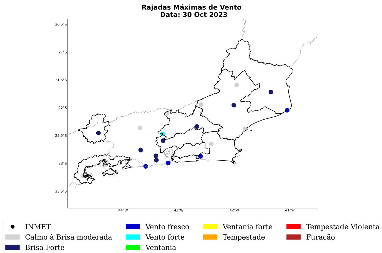
Figura 42: Máxima rajada de vento diária sobre a área de concessão da Enel-RJ para o dia 30 de outubro, baseado nas estações meteorológicas do INMET.
