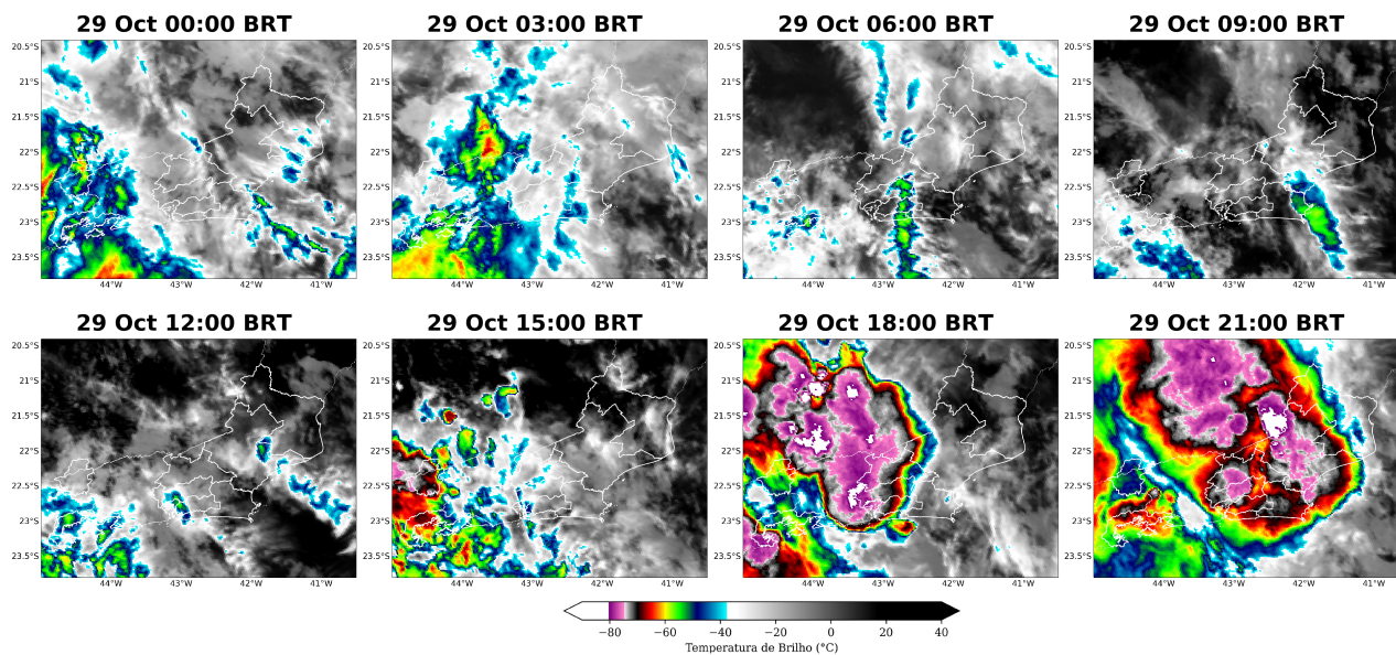
Figura 8: Imagens realçadas do satélite GOES-16 das 00 BRT até 21 BRT (a cada 3 horas) para o dia 29 de outubro.
