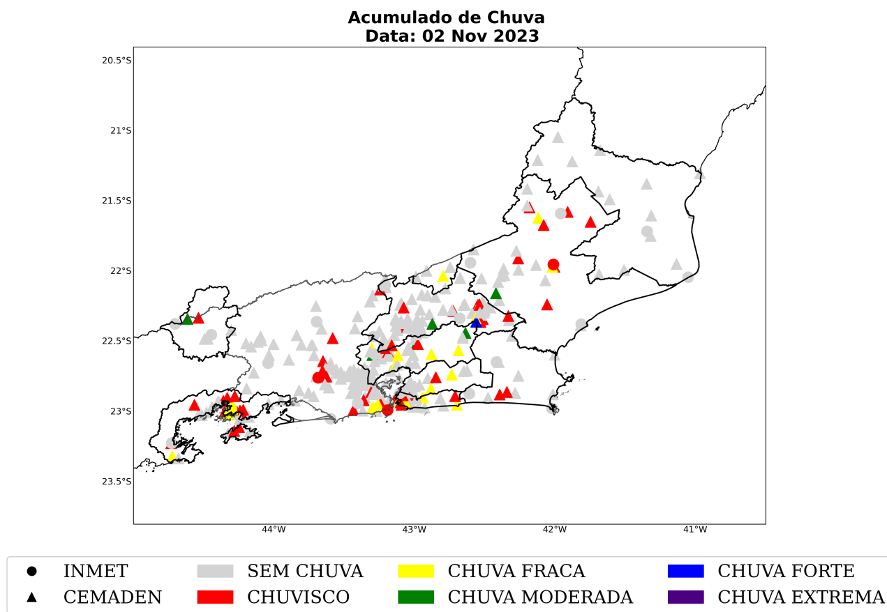
Figura 33: Acumulado diário de precipitação sobre a área de concessão da Enel-RJ para o dia 02 de novembro, baseado nas estações meteorológicas do INMET e CEMADEN.
