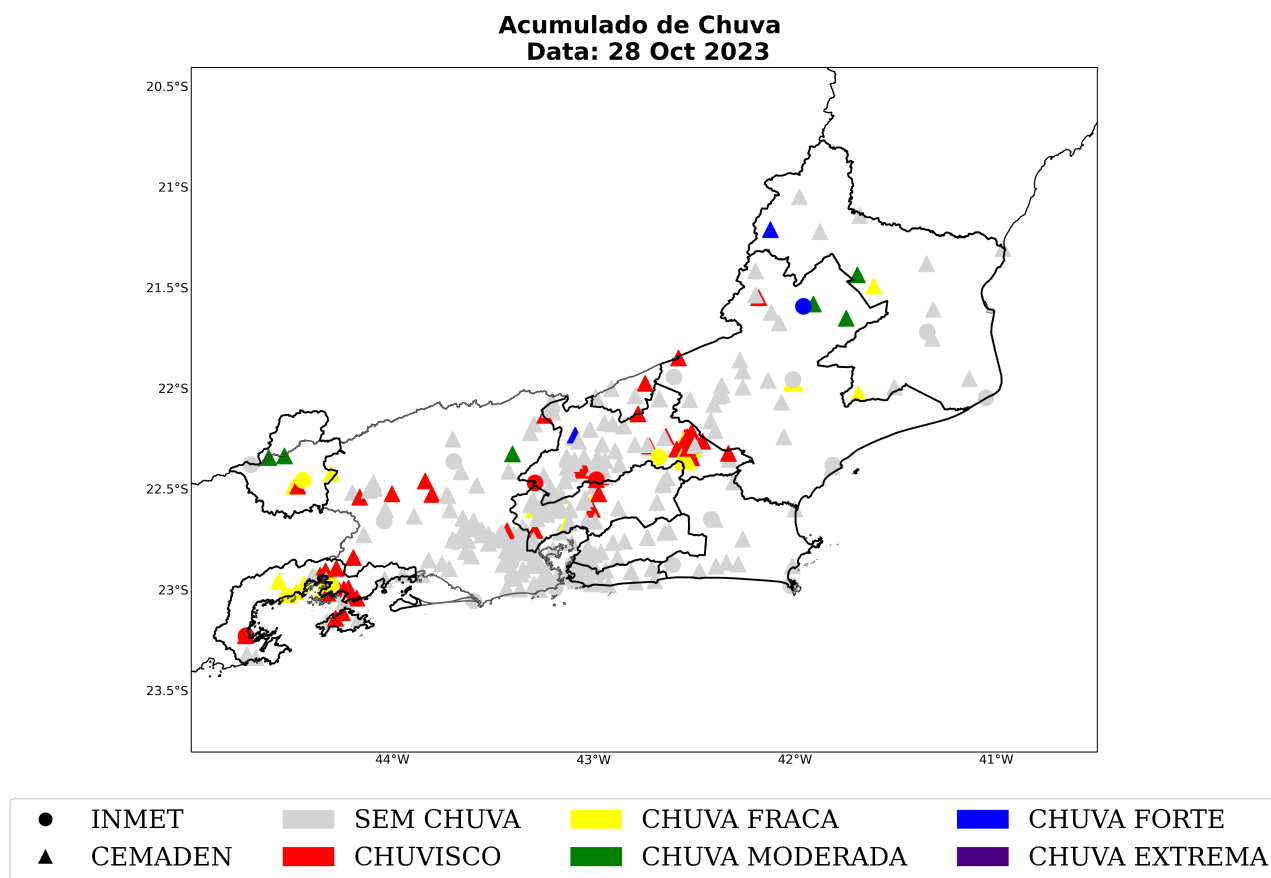
Figura 28: Acumulado diário de precipitação sobre a área de concessão da Enel-RJ para o dia 28 de outubro, baseado nas estações meteorológicas do INMET e CEMADEN.
