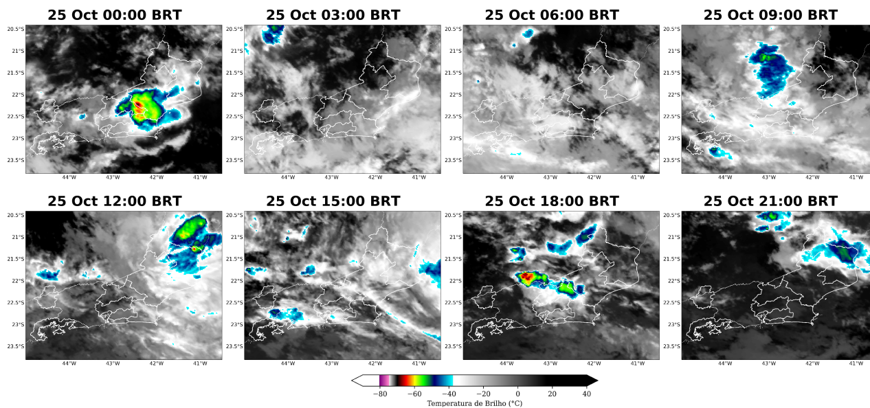
Figura 4: Imagens realçadas do satélite GOES-16 das 00 BRT até 21 BRT (a cada 3 horas) para o dia 25 de outubro.
