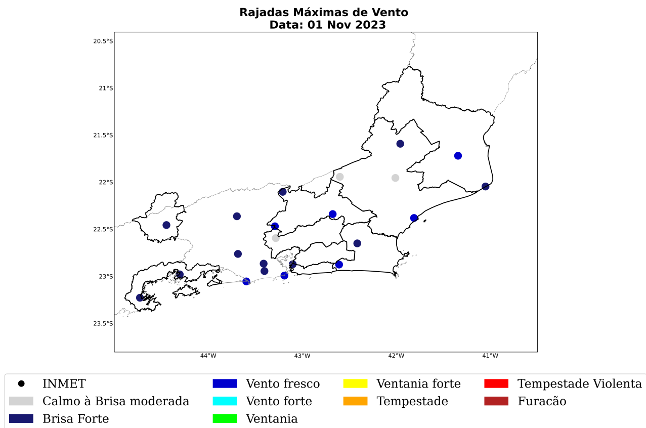
Figura 44: Máxima rajada de vento diária sobre a área de concessão da Enel-RJ para o dia 01 de novembro, baseado nas estações meteorológicas do INMET.
