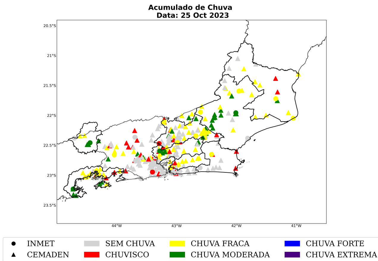
Figura 25: Acumulado diário de precipitação sobre a área de concessão da Enel-RJ para o dia 25 de outubro, baseado nas estações meteorológicas do INMET e CEMADEN.
