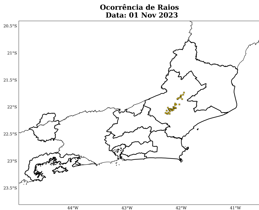
Figura 21: Densidade de descargas atmosféricas nuvem-solo detectadas pelo sistema Earth Networks para o dia 01 de novembro sobre a área de concessão da Enel-RJ.
