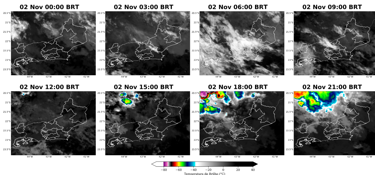
Figura 12: Imagens realçadas do satélite GOES-16 das 00 BRT até 21 BRT (a cada 3 horas) para o dia 02 de novembro.
