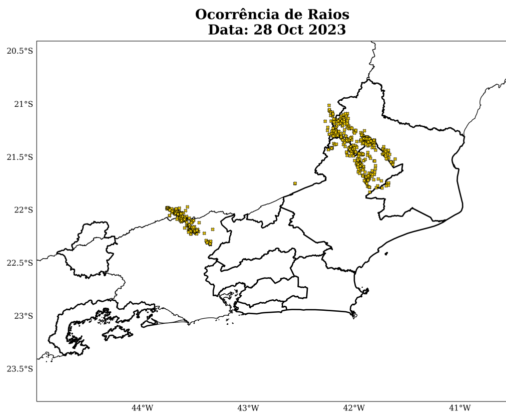
Figura 17: Densidade de descargas atmosféricas nuvem-solo detectadas pelo sistema Earth Networks para o dia 28 de outubro sobre a área de concessão da Enel-RJ.
