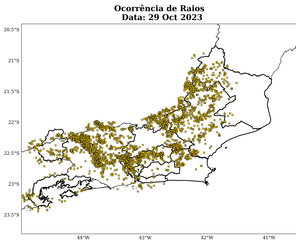
Figura 18: Densidade de descargas atmosféricas nuvem-solo detectadas pelo sistema Earth Networks para o dia 29 de outubro sobre a área de concessão da Enel-RJ.
