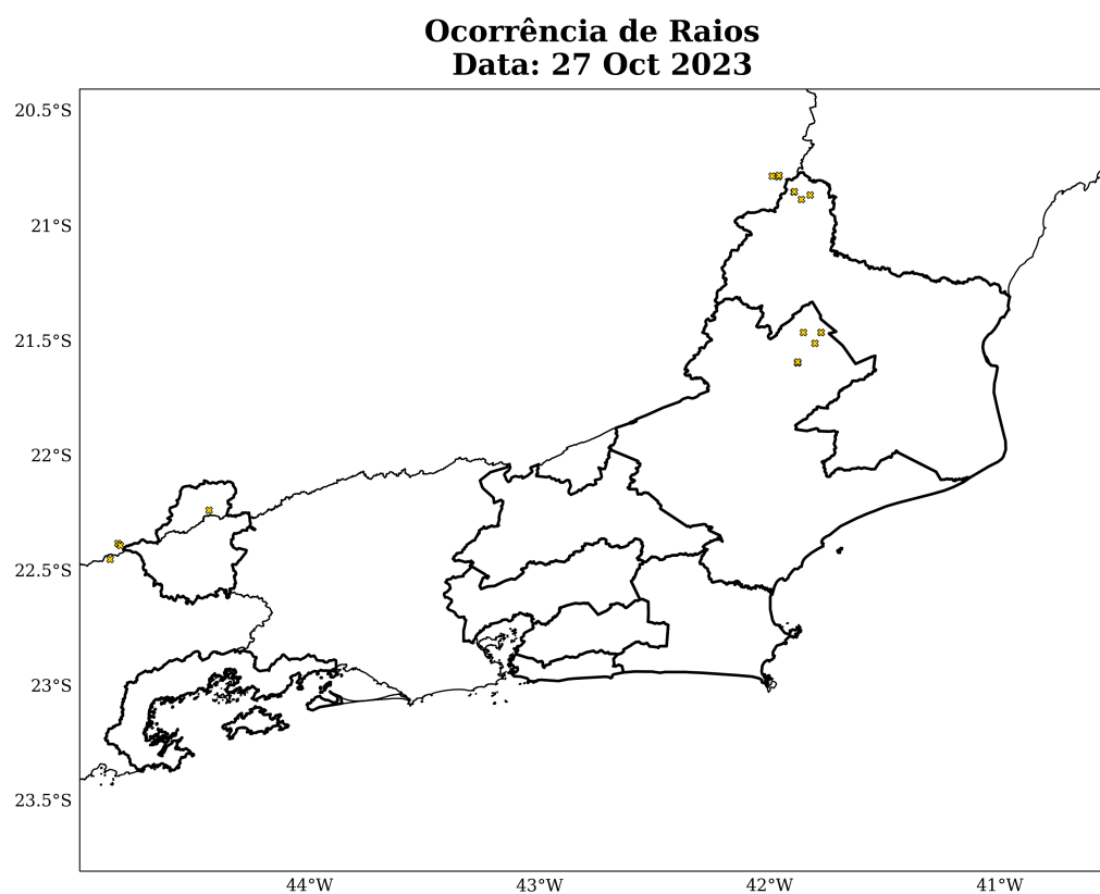
Figura 16: Densidade de descargas atmosféricas nuvem-solo detectadas pelo sistema Earth Networks para o dia 27 de outubro sobre a área de concessão da Enel-RJ.
