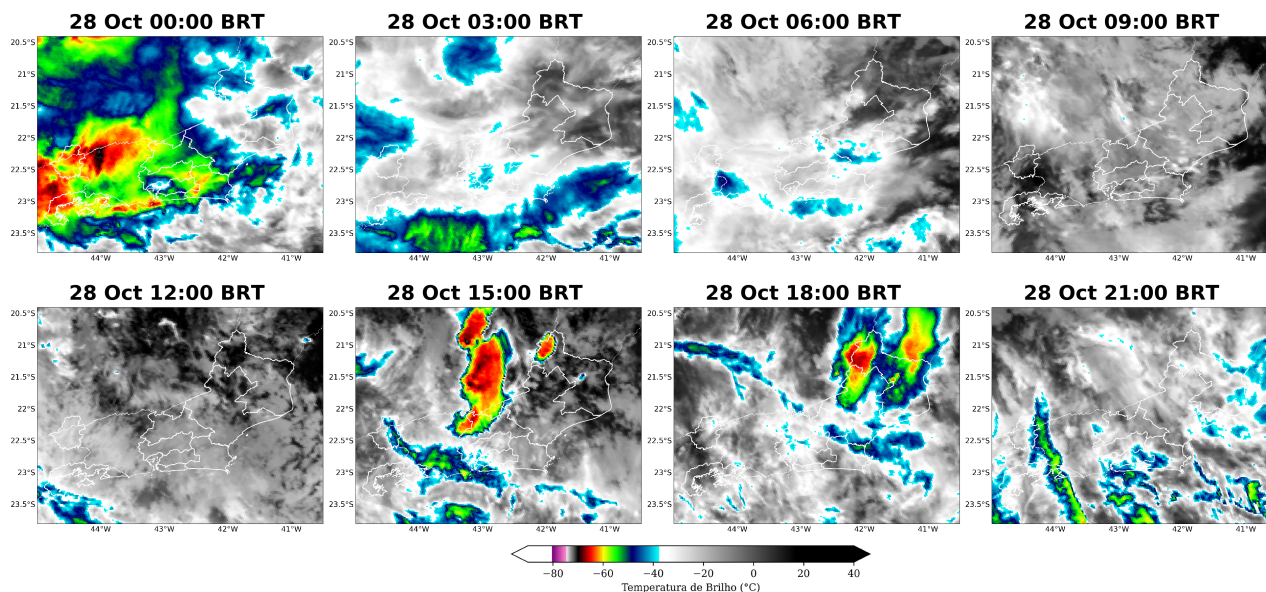
Figura 7: Imagens realçadas do satélite GOES-16 das 00 BRT até 21 BRT (a cada 3 horas) para o dia 28 de outubro.
