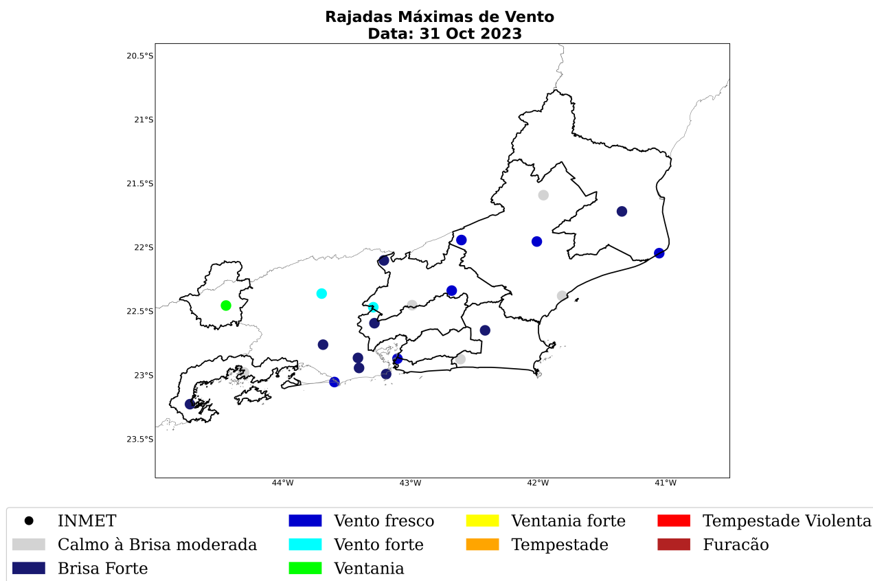
Figura 43: Máxima rajada de vento diária sobre a área de concessão da Enel-RJ para o dia 31 de outubro, baseado nas estações meteorológicas do INMET.
