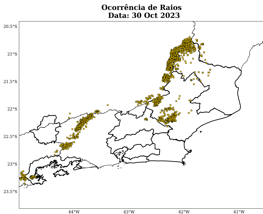
Figura 19: Densidade de descargas atmosféricas nuvem-solo detectadas pelo sistema Earth Networks para o dia 30 de outubro sobre a área de concessão da Enel-RJ.
