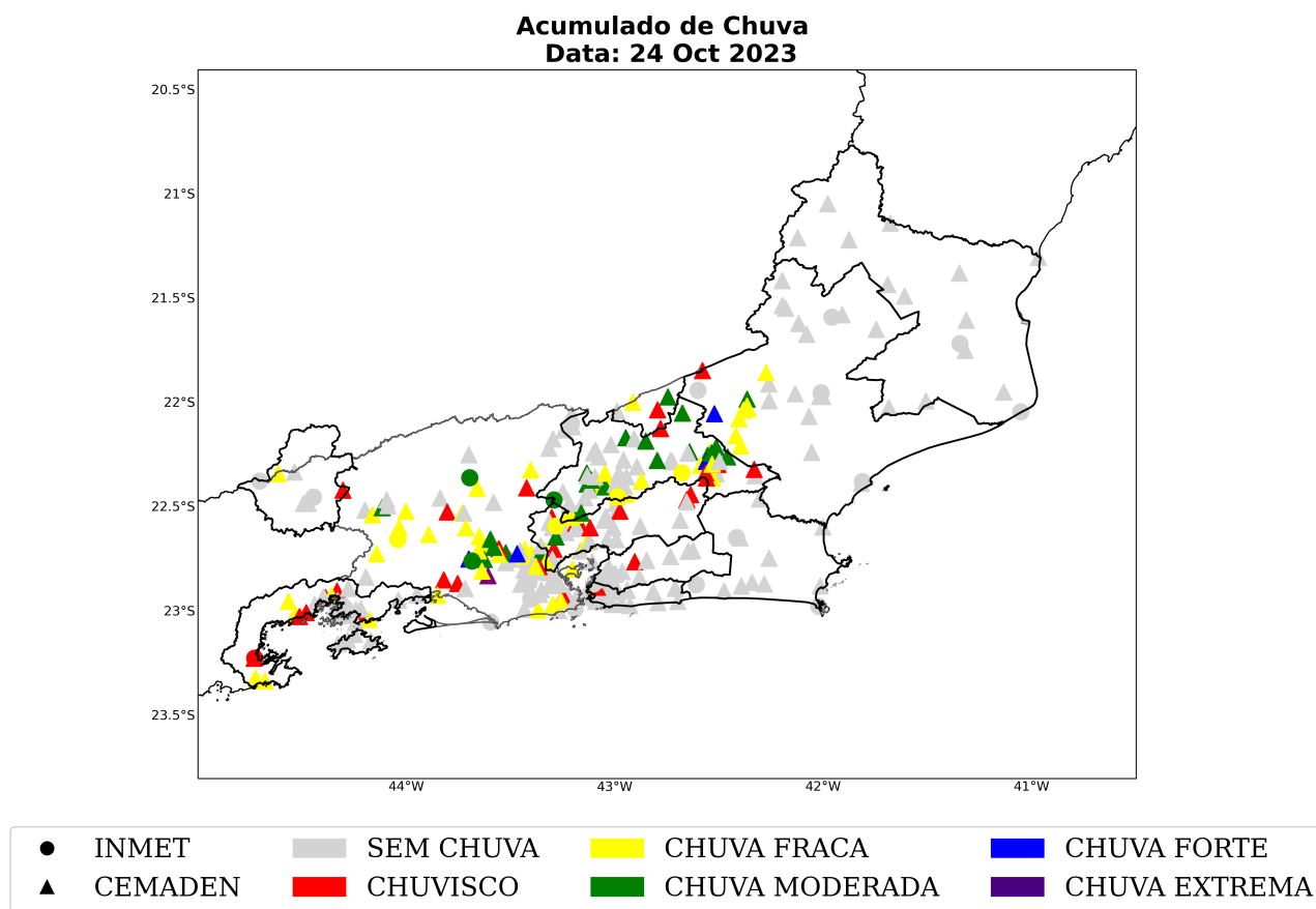
Figura 24: Acumulado diário de precipitação sobre a área de concessão da Enel-RJ para o dia 24 de outubro, baseado nas estações meteorológicas do INMET e CEMADEN.
