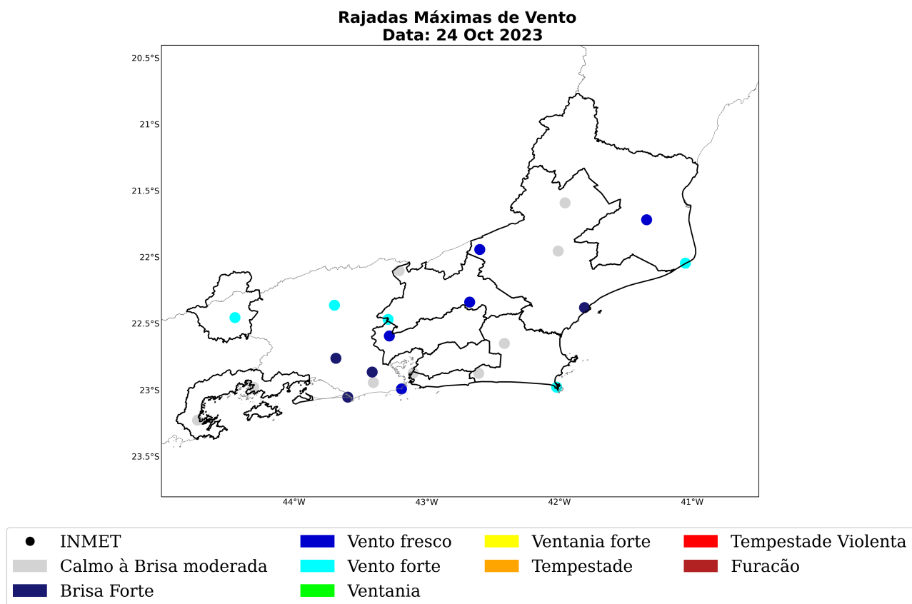
Figura 36: Máxima rajada de vento diária sobre a área de concessão da Enel-RJ para o dia 24 de outubro, baseado nas estações meteorológicas do INMET.
