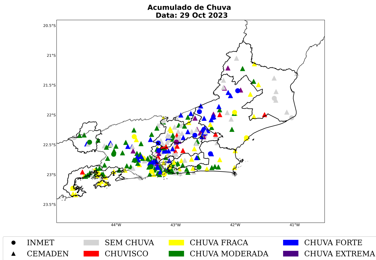
Figura 29: Acumulado diário de precipitação sobre a área de concessão da Enel-RJ para o dia 29 de outubro, baseado nas estações meteorológicas do INMET e CEMADEN.
