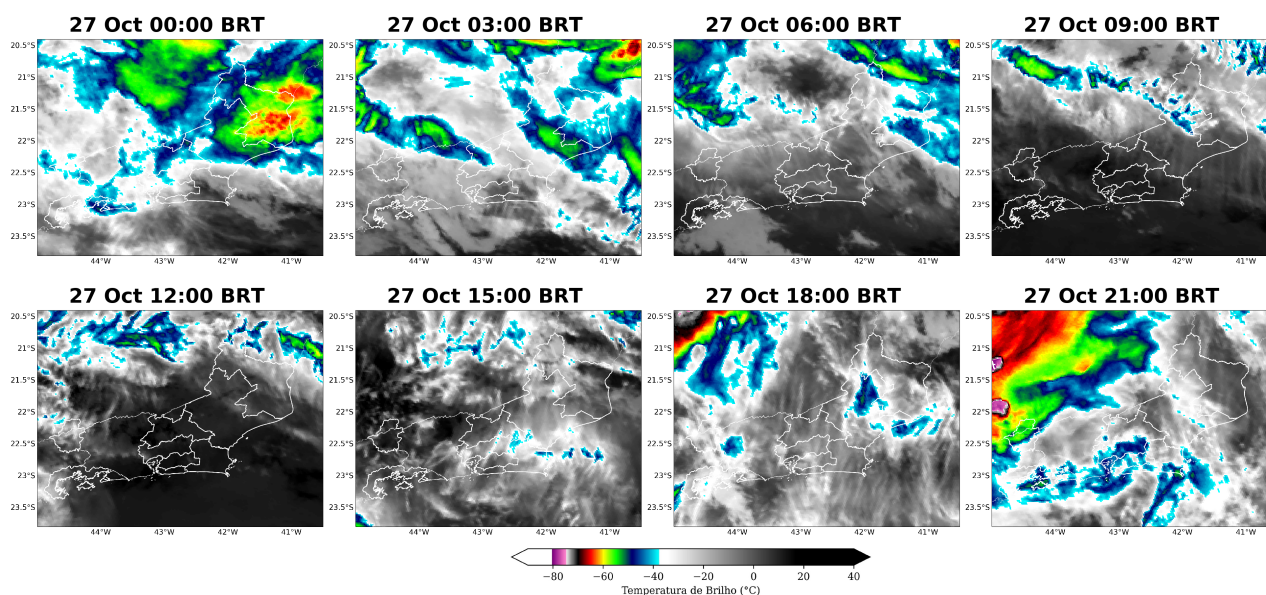
Figura 6: Imagens realçadas do satélite GOES-16 das 00 BRT até 21 BRT (a cada 3 horas) para o dia 27 de outubro.
