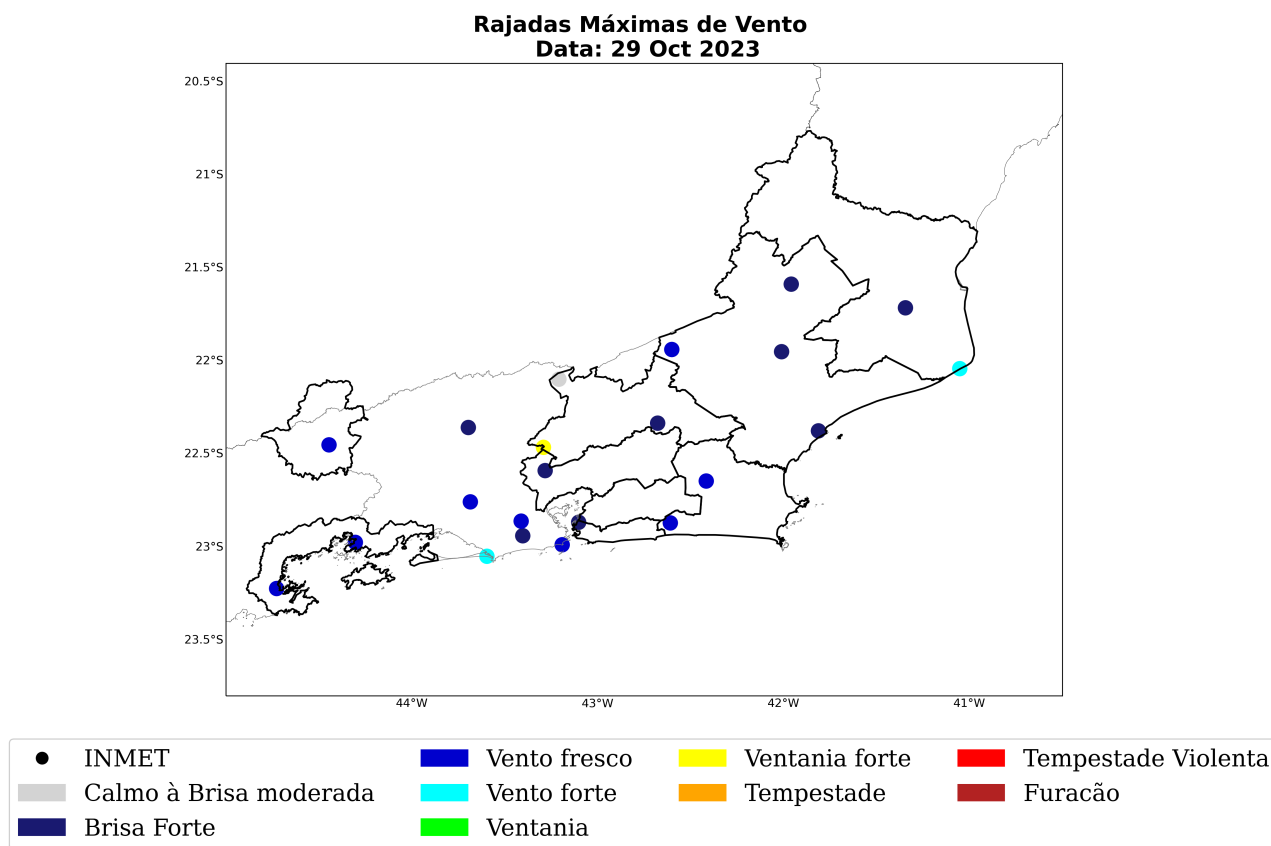
Figura 41: Máxima rajada de vento diária sobre a área de concessão da Enel-RJ para o dia 29 de outubro, baseado nas estações meteorológicas do INMET.
