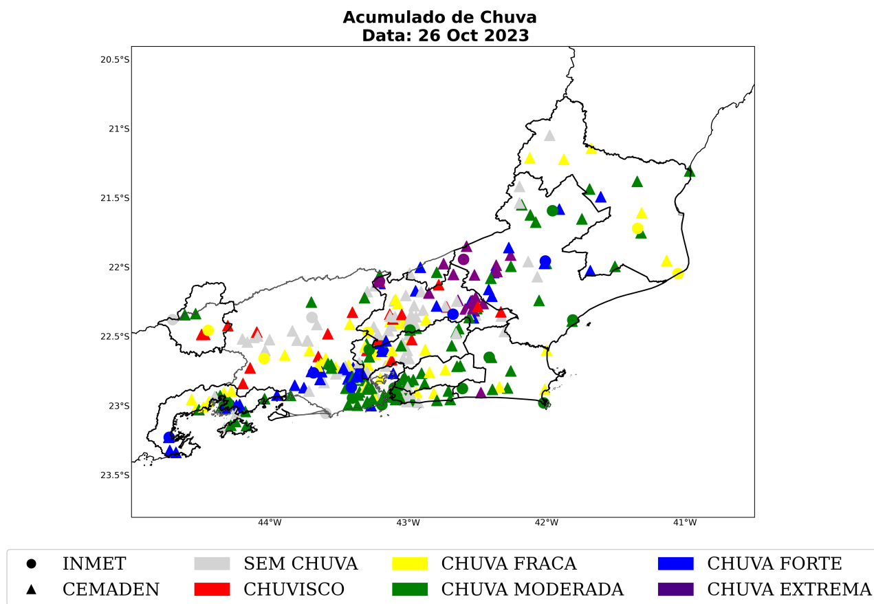
Figura 26: Acumulado diário de precipitação sobre a área de concessão da Enel-RJ para o dia 26 de outubro, baseado nas estações meteorológicas do INMET e CEMADEN.
