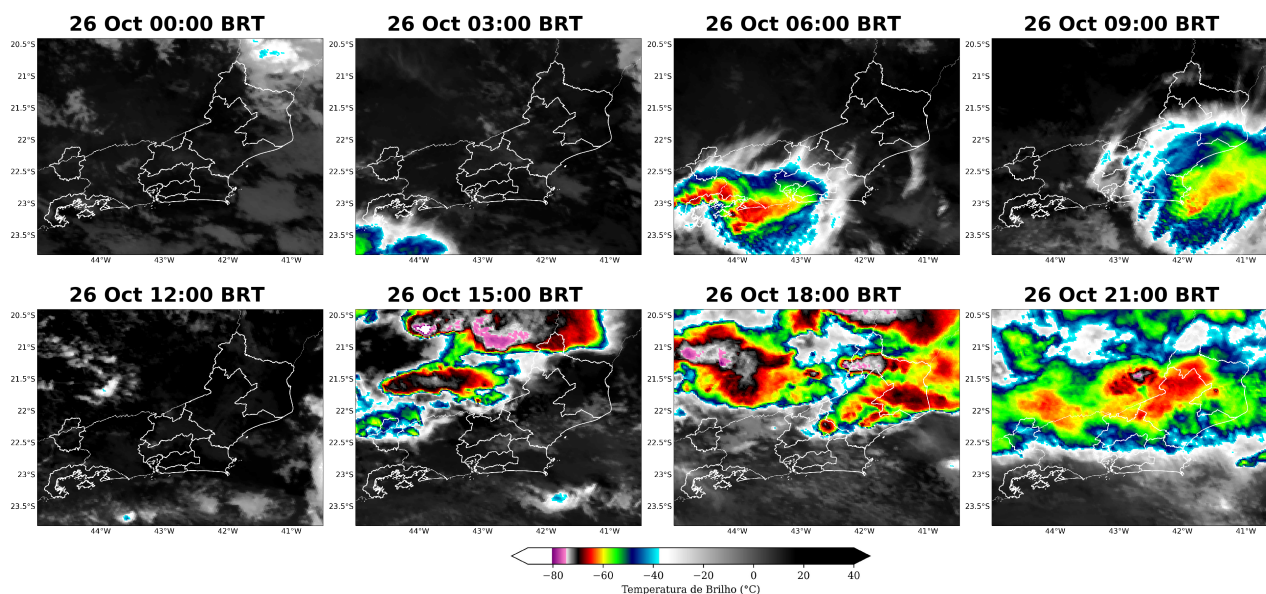
Figura 5: Imagens realçadas do satélite GOES-16 das 00 BRT até 21 BRT (a cada 3 horas) para o dia 26 de outubro.
