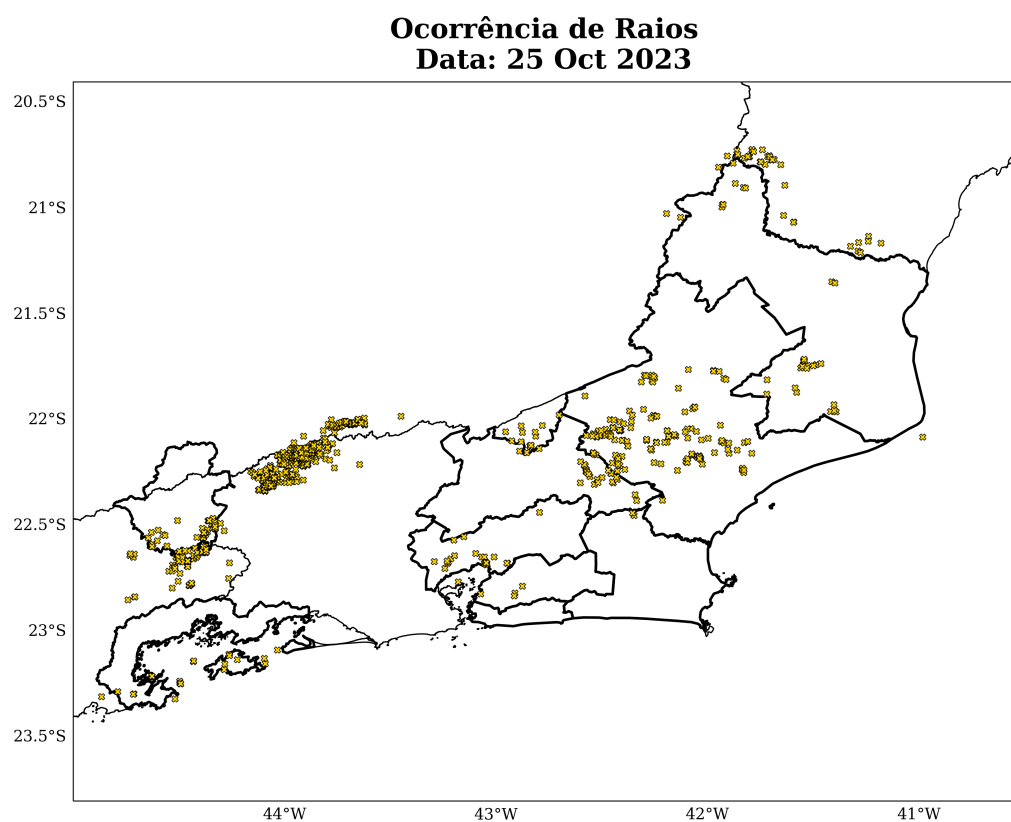
Figura 14: Densidade de descargas atmosféricas nuvem-solo detectadas pelo sistema Earth Networks para o dia 25 de outubro sobre a área de concessão da Enel-RJ.
