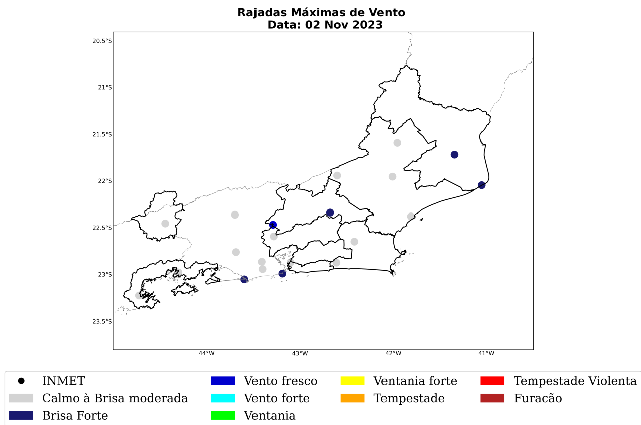
Figura 45: Máxima rajada de vento diária sobre a área de concessão da Enel-RJ para o dia 02 de novembro, baseado nas estações meteorológicas do INMET.
