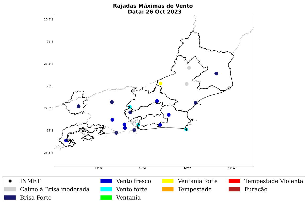
Figura 38: Máxima rajada de vento diária sobre a área de concessão da Enel-RJ para o dia 26 de outubro, baseado nas estações meteorológicas do INMET.
