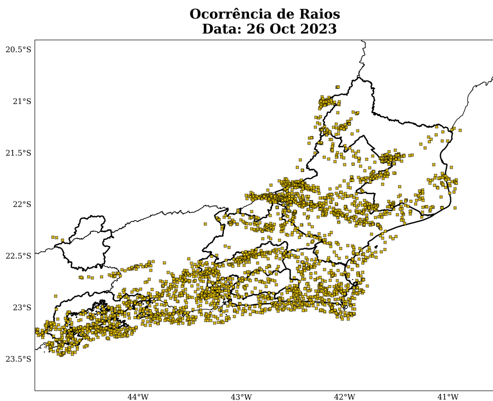
Figura 15: Densidade de descargas atmosféricas nuvem-solo detectadas pelo sistema Earth Networks para o dia 26 de outubro sobre a área de concessão da Enel-RJ.
