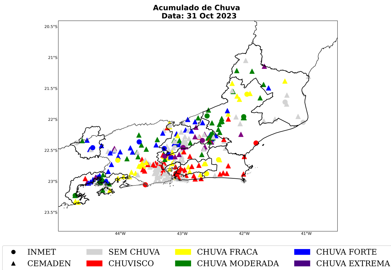
Figura 31: Acumulado diário de precipitação sobre a área de concessão da Enel-RJ para o dia 31 de outubro, baseado nas estações meteorológicas do INMET e CEMADEN.
