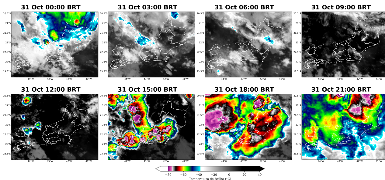
Figura 10: Imagens realçadas do satélite GOES-16 das 00 BRT até 21 BRT (a cada 3 horas) para o dia 31 de outubro.
