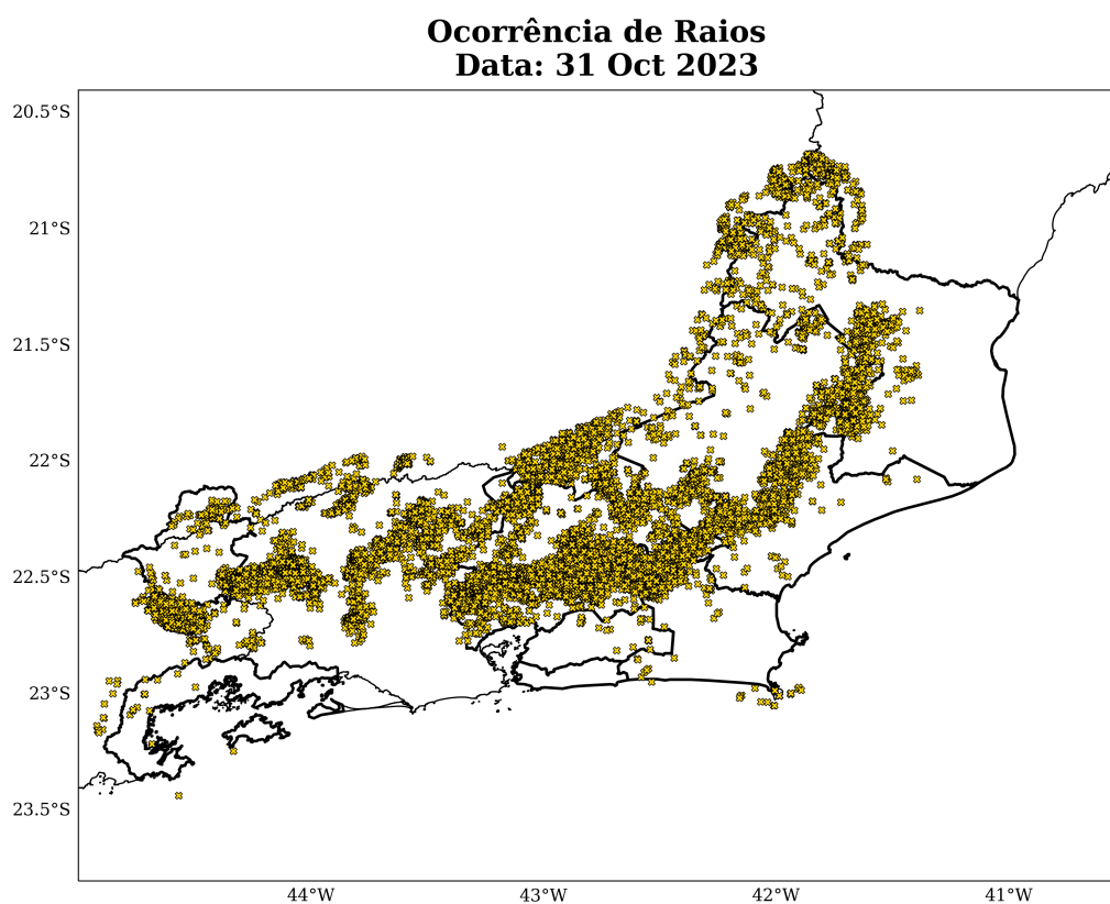
Figura 20: Densidade de descargas atmosféricas nuvem-solo detectadas pelo sistema Earth Networks para o dia 31 de outubro sobre a área de concessão da Enel-RJ.
