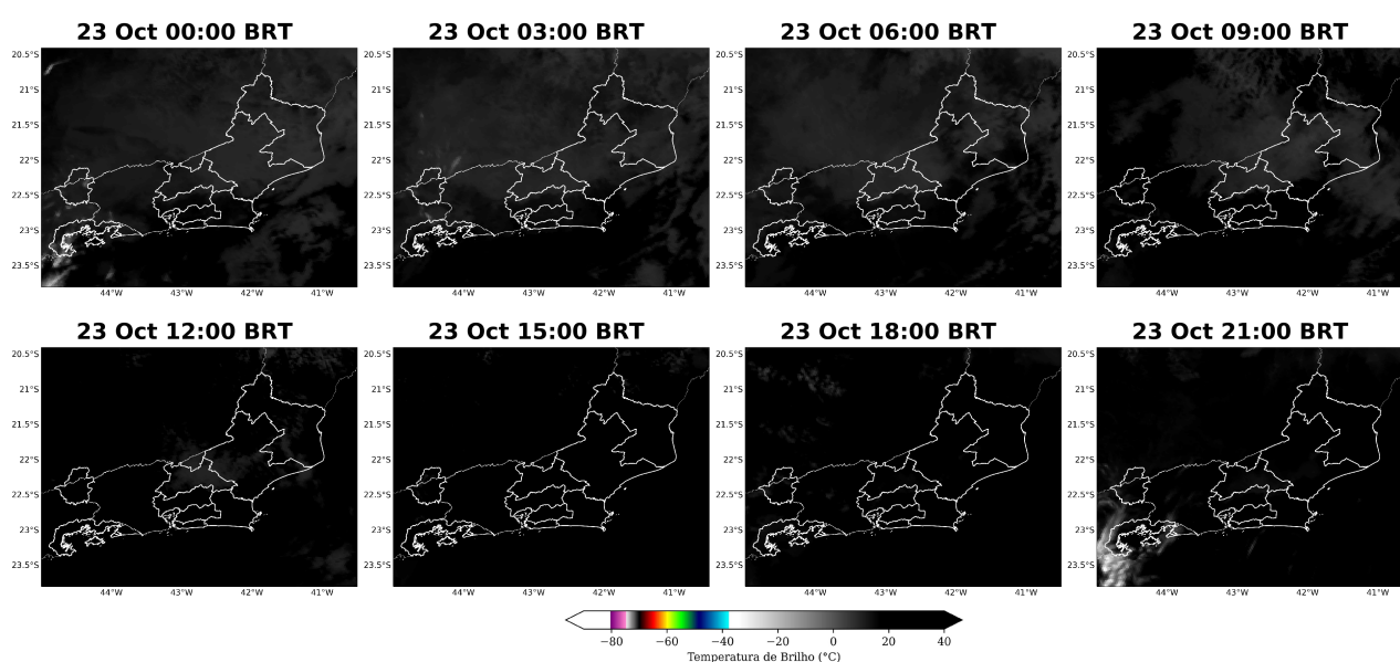
Figura 2: Imagens realçadas do satélite GOES-16 das 00 BRT até 21 BRT (a cada 3 horas) para o dia 23 de outubro.
