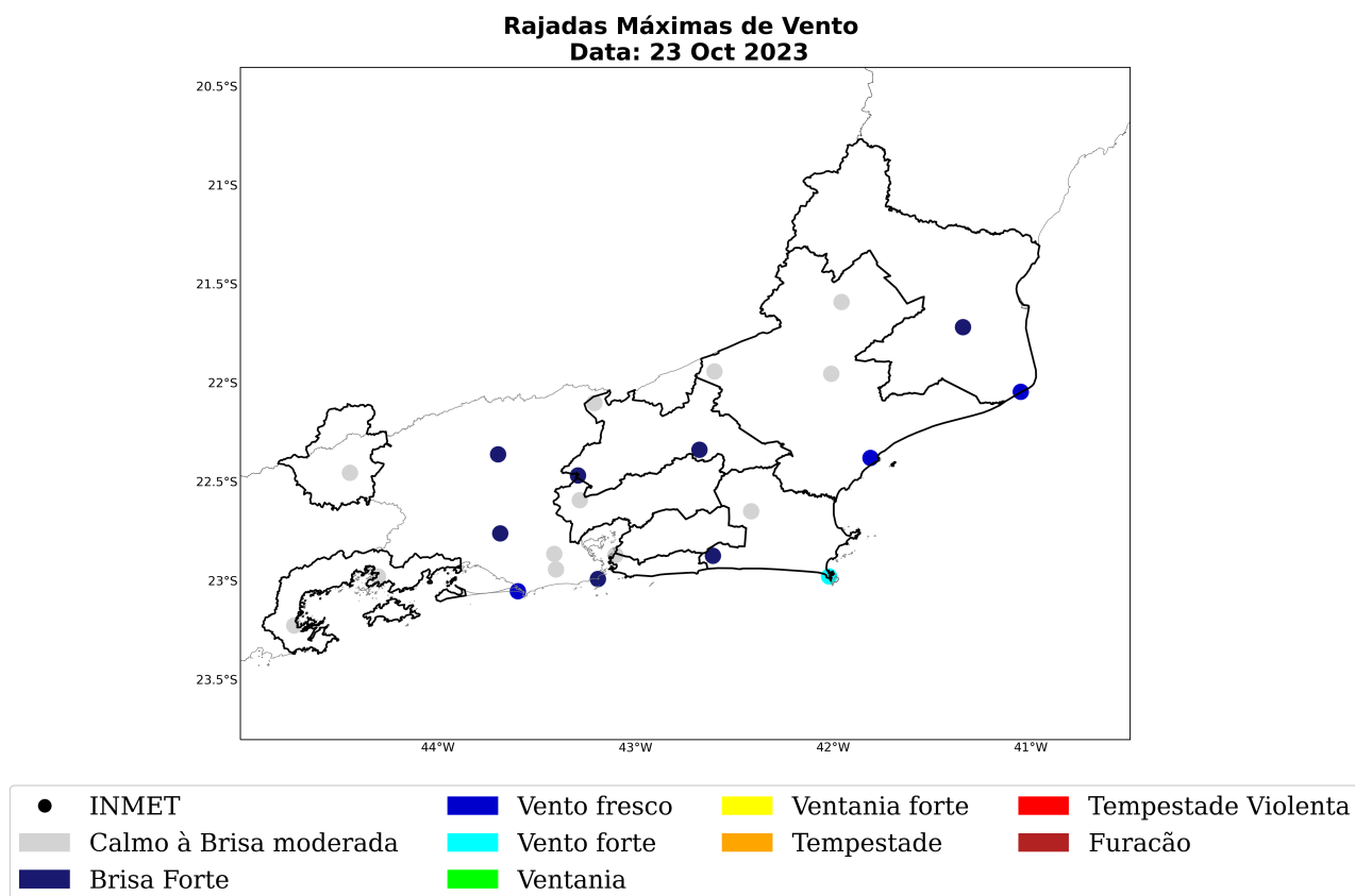
Figura 35: Máxima rajada de vento diária sobre a área de concessão da Enel-RJ para o dia 23 de outubro, baseado nas estações meteorológicas do INMET.
