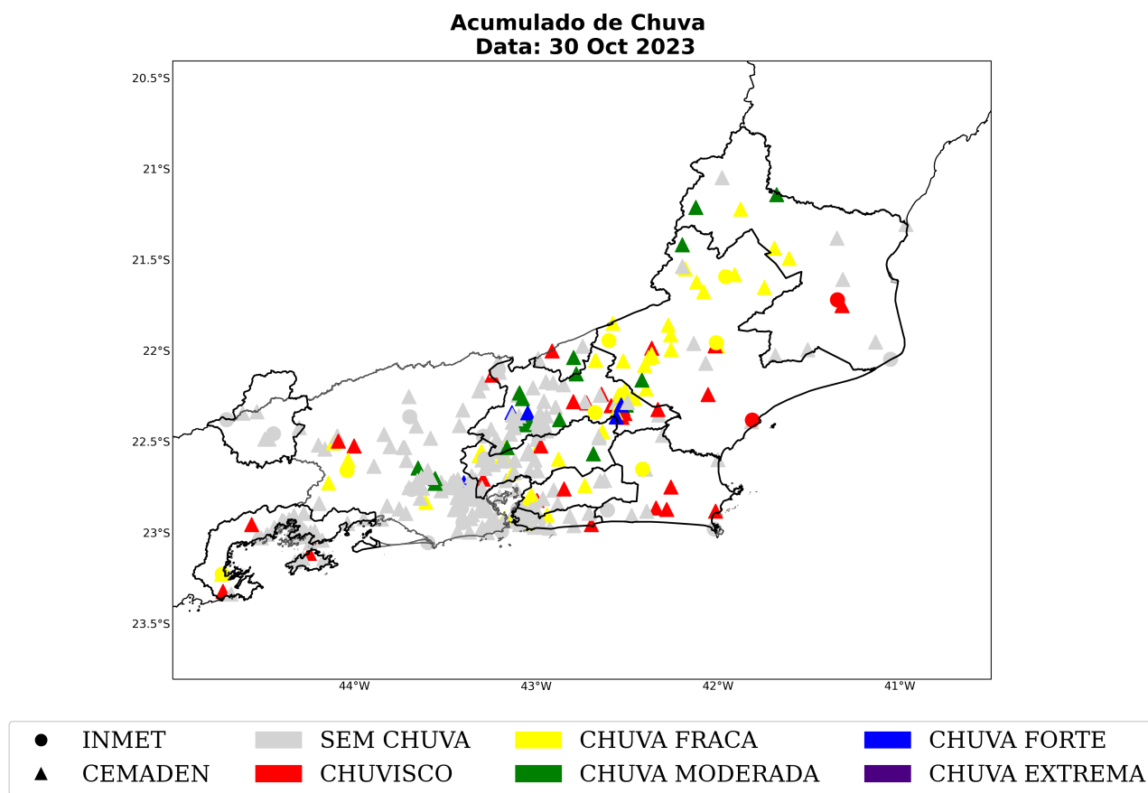
Figura 30: Acumulado diário de precipitação sobre a área de concessão da Enel-RJ para o dia 30 de outubro, baseado nas estações meteorológicas do INMET e CEMADEN.
