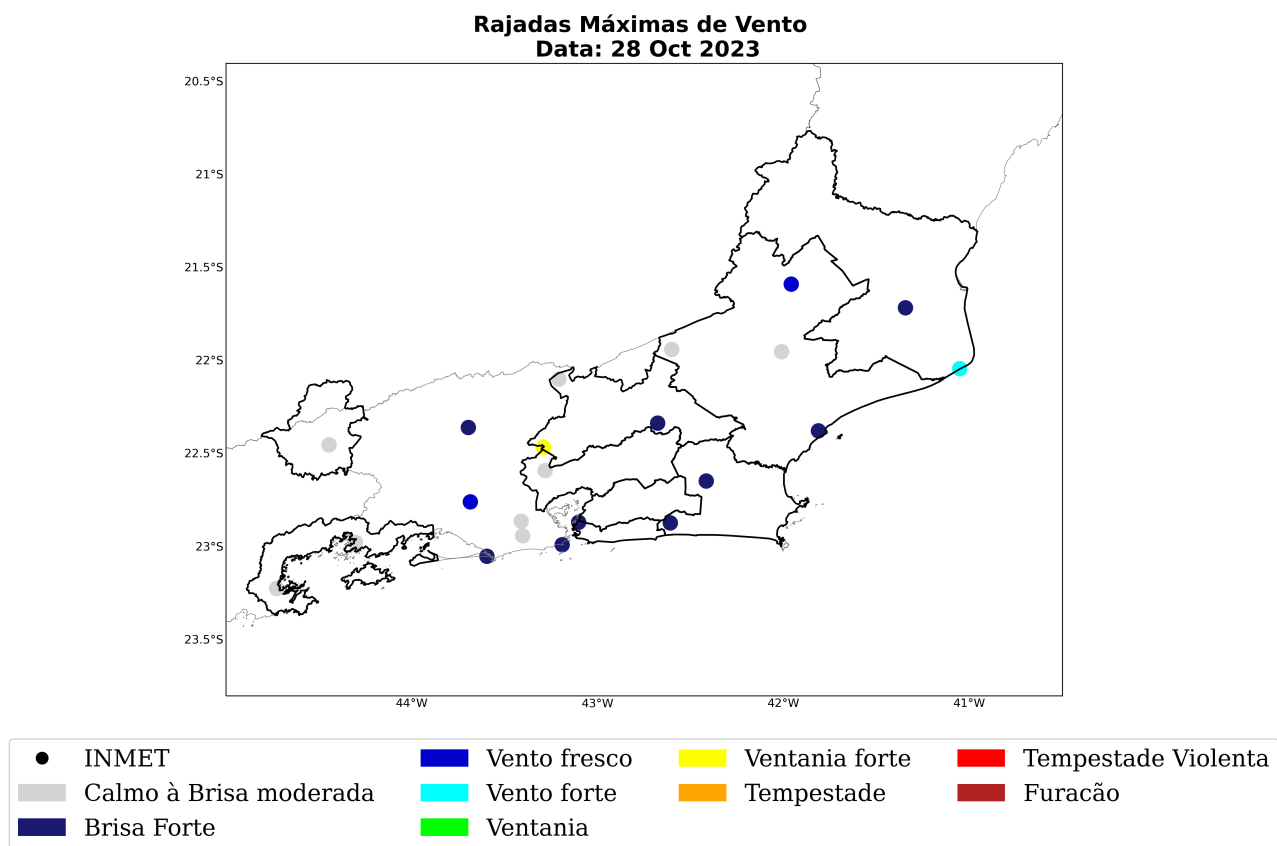
Figura 40: Máxima rajada de vento diária sobre a área de concessão da Enel-RJ para o dia 28 de outubro, baseado nas estações meteorológicas do INMET.
