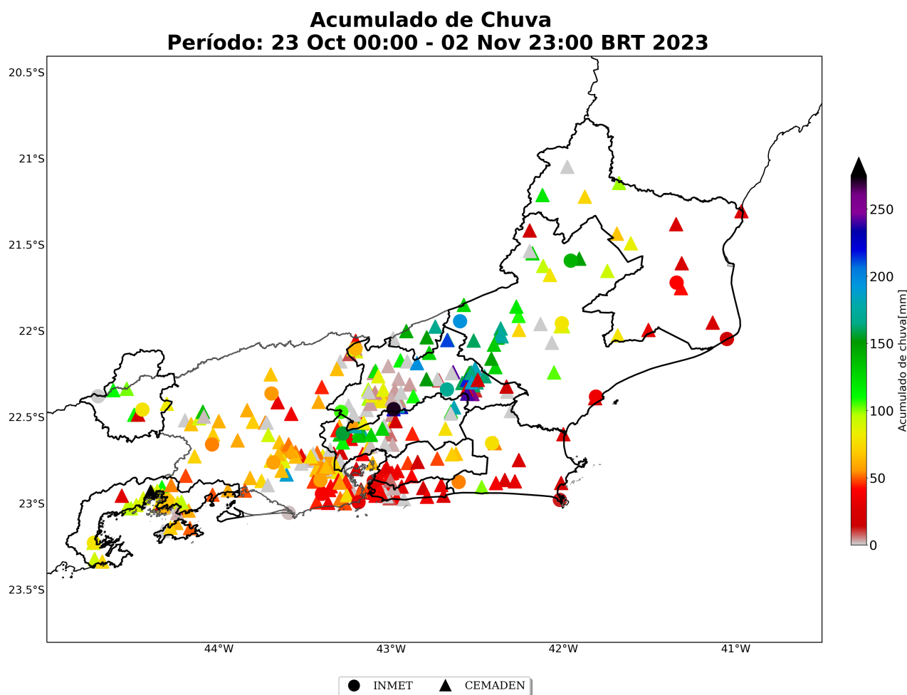
Figura 34: Acumulado de precipitação sobre o estado do Rio de Janeiro para o período do evento (dias 23 de outubro a 02 de novembro de 2023), baseado nas estações meteorológicas do INMET e CEMADEN.
