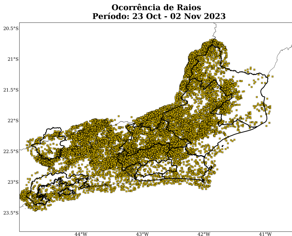
Figura 22: Total de descargas atmosféricas nuvem-solo detectadas pelo sistema Earth Networks durante o período de 23 de outubro a 02 de novembro de 2023 sobre a área de concessão da Enel-RJ.
