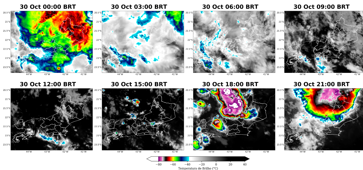
Figura 9: Imagens realçadas do satélite GOES-16 das 00 BRT até 21 BRT (a cada 3 horas) para o dia 30 de outubro.
