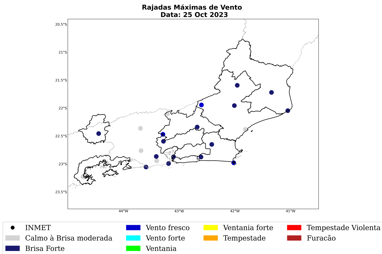
Figura 37: Máxima rajada de vento diária sobre a área de concessão da Enel-RJ para o dia 25 de outubro, baseado nas estações meteorológicas do INMET.
