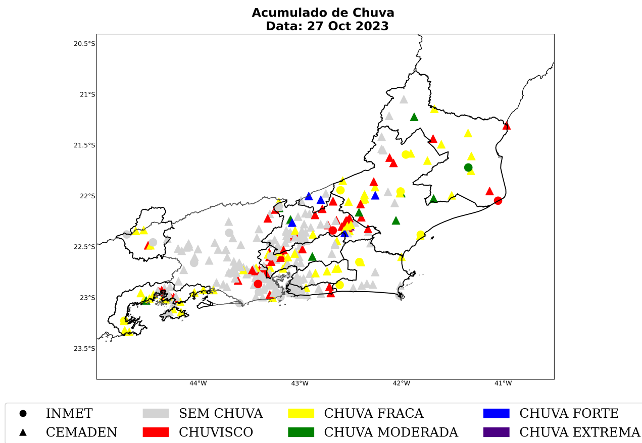
Figura 27: Acumulado diário de precipitação sobre a área de concessão da Enel-RJ para o dia 27 de outubro, baseado nas estações meteorológicas do INMET e CEMADEN.
