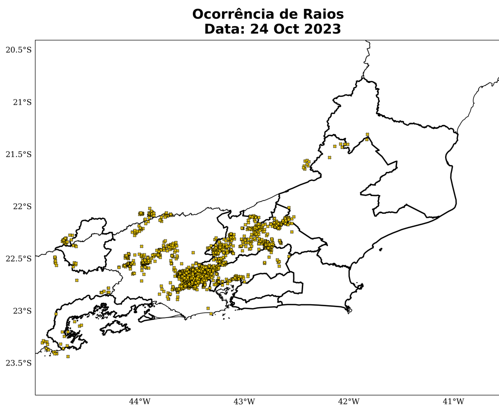
Figura 13: Total de descargas atmosféricas nuvem-solo detectadas pelo sistema Earth Networks para o dia 24 de outubro sobre a área de concessão da Enel-RJ.
