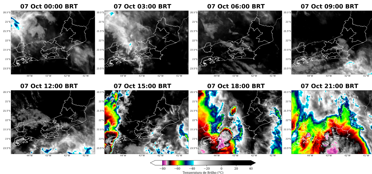
Figura 4: Imagens realçadas do satélite GOES-16 das 00 BRT até 21 BRT (a cada 3 horas) para o dia 07 de outubro.
