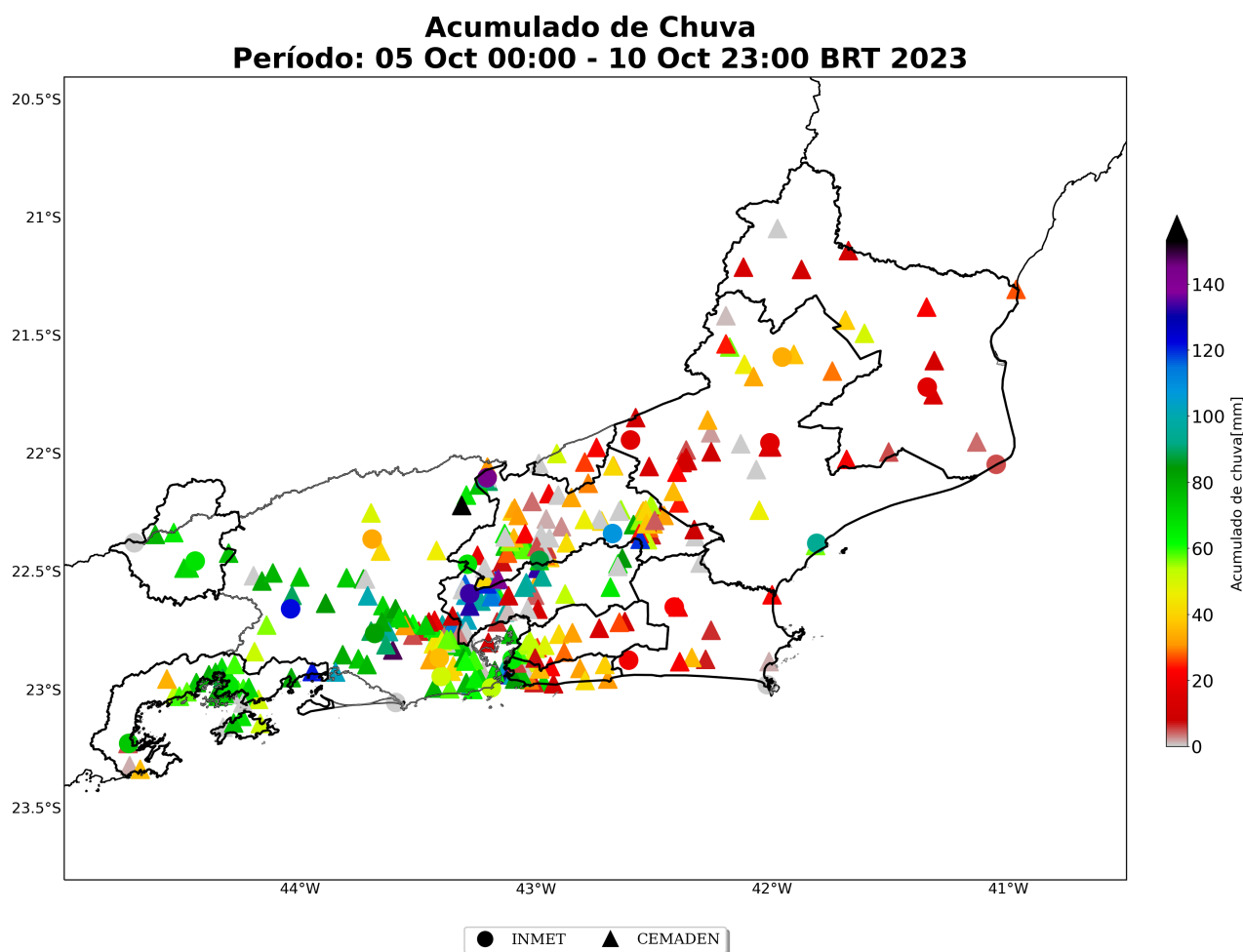
Figura 20: Acumulado de precipitação sobre o estado do Rio de Janeiro para o período do evento (dias 05 a 10 de outubro de 2023), baseado nas estações meteorológicas do INMET e CEMADEN.
