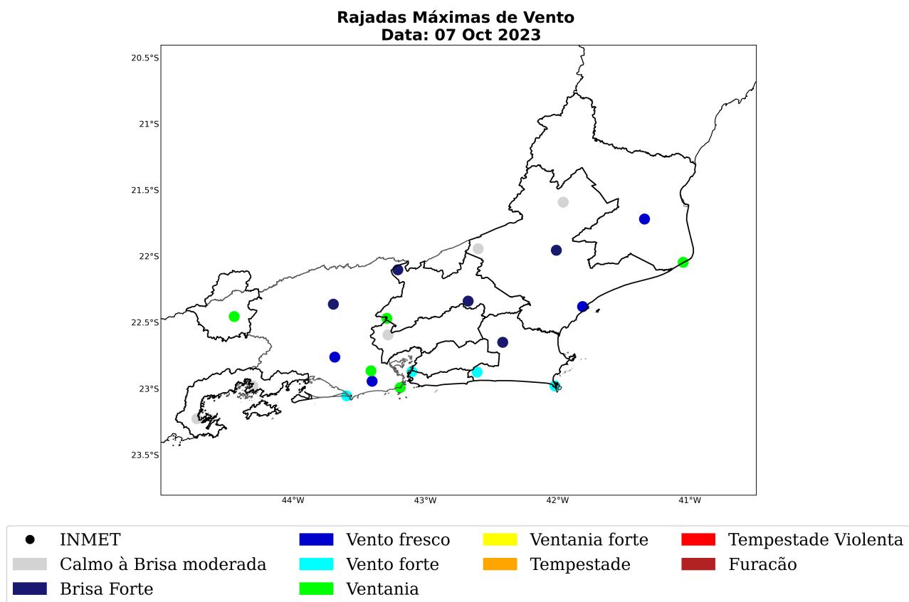
Figura 23: Máxima rajada de vento diária sobre a área de concessão da Enel-RJ para o dia 07 de outubro, baseado nas estações meteorológicas do INMET.
