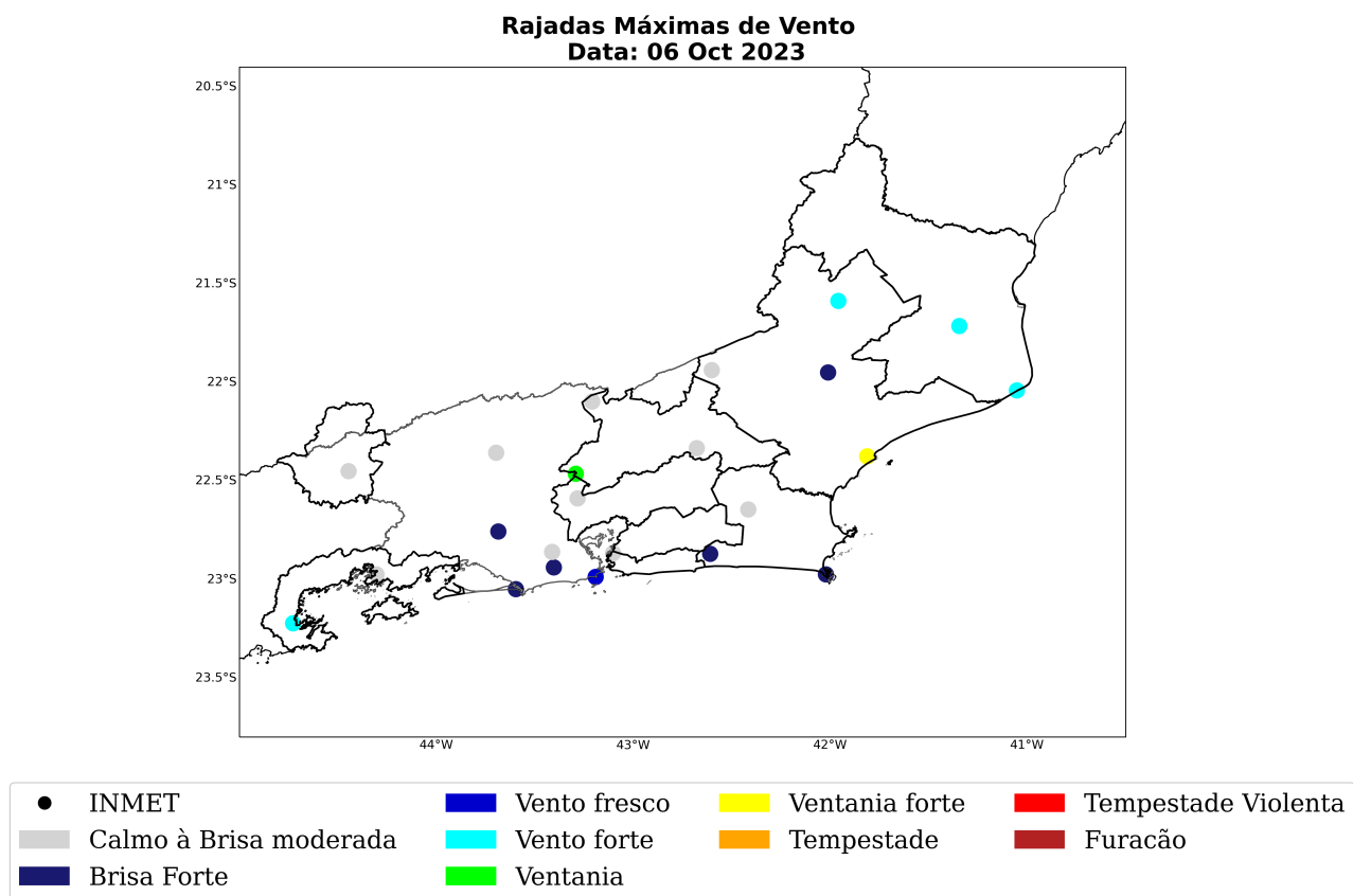
Figura 22: Máxima rajada de vento diária sobre a área de concessão da Enel-RJ para o dia 06 de outubro, baseado nas estações meteorológicas do INMET.
