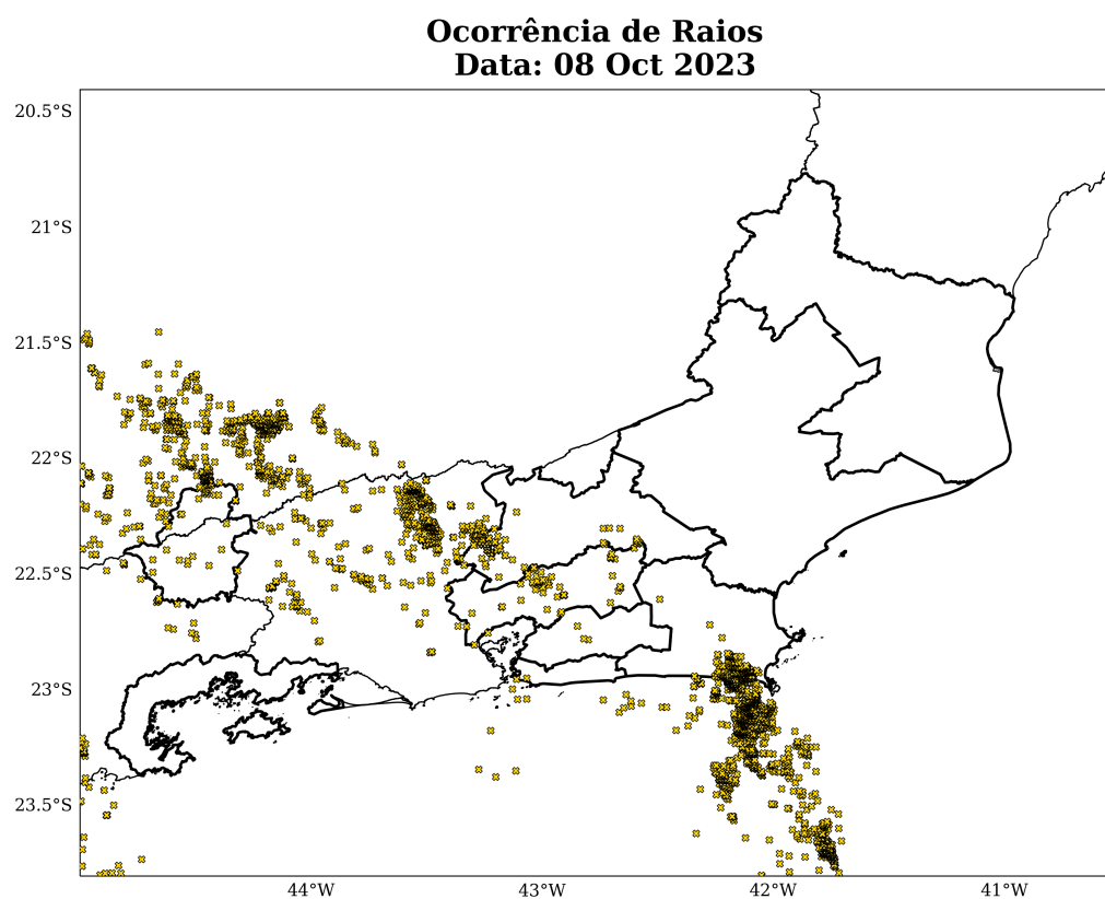
Figura 11: Total de descargas atmosféricas nuvem-solo detectadas pelo sistema Earth Networks para o dia 08 de outubro sobre a área de concessão da Enel-RJ.
