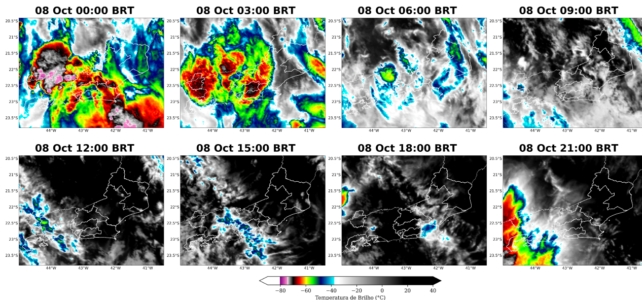
Figura 5: Imagens realçadas do satélite GOES-16 das 00 BRT até 21 BRT (a cada 3 horas) para o dia 08 de outubro.
