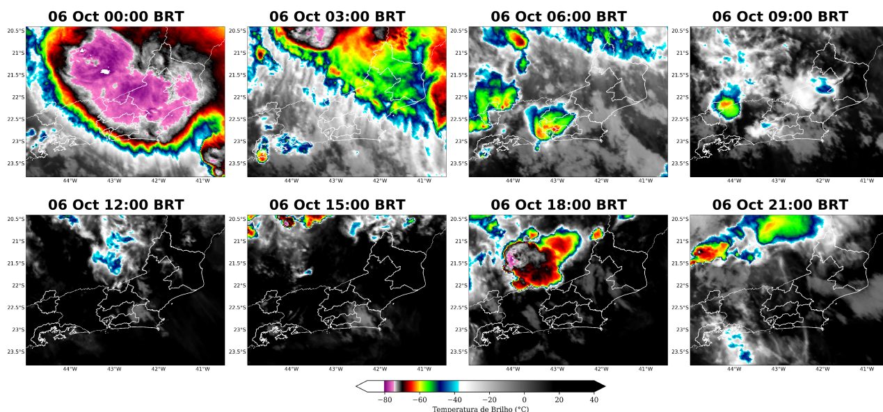
Figura 3: Imagens realçadas do satélite GOES-16 das 00 BRT até 21 BRT (a cada 3 horas) para o dia 06 de outubro.
