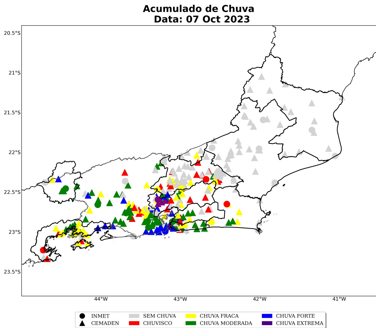
Figura 16: Acumulado diário de precipitação sobre a área de concessão da Enel-RJ para o dia 07 de outubro, baseado nas estações meteorológicas do INMET e CEMADEN.
