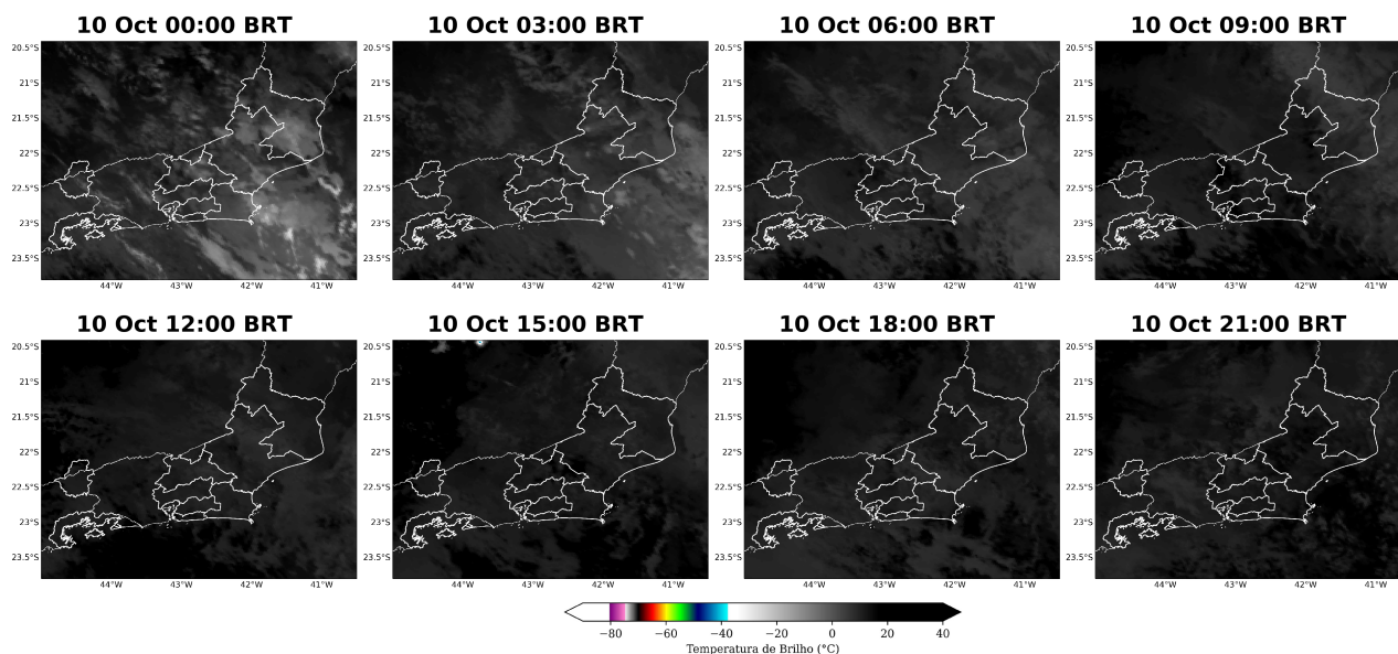
Figura 7: Imagens realçadas do satélite GOES-16 das 00 BRT até 21 BRT (a cada 3 horas) para o dia 10 de outubro.
