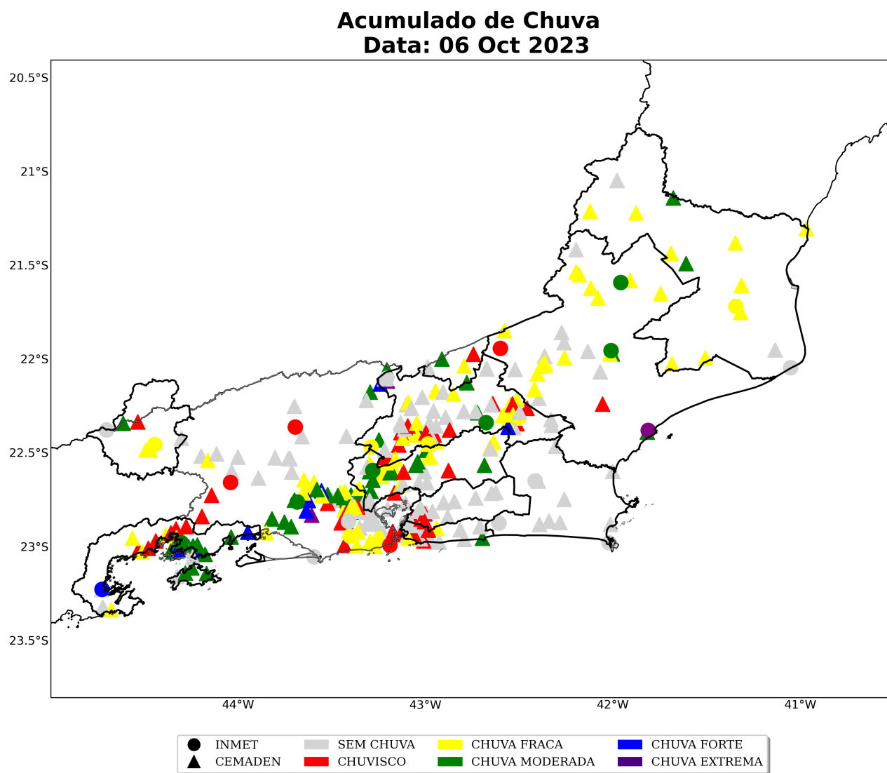
Figura 15: Acumulado diário de precipitação sobre a área de concessão da Enel-RJ para o dia 06 de outubro, baseado nas estações meteorológicas do INMET e CEMADEN.
