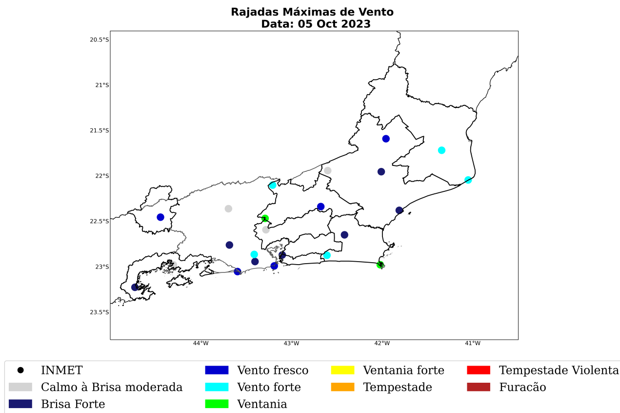
Figura 21: Máxima rajada de vento diária sobre a área de concessão da Enel-RJ para o dia 05 de outubro, baseado nas estações meteorológicas do INMET.
