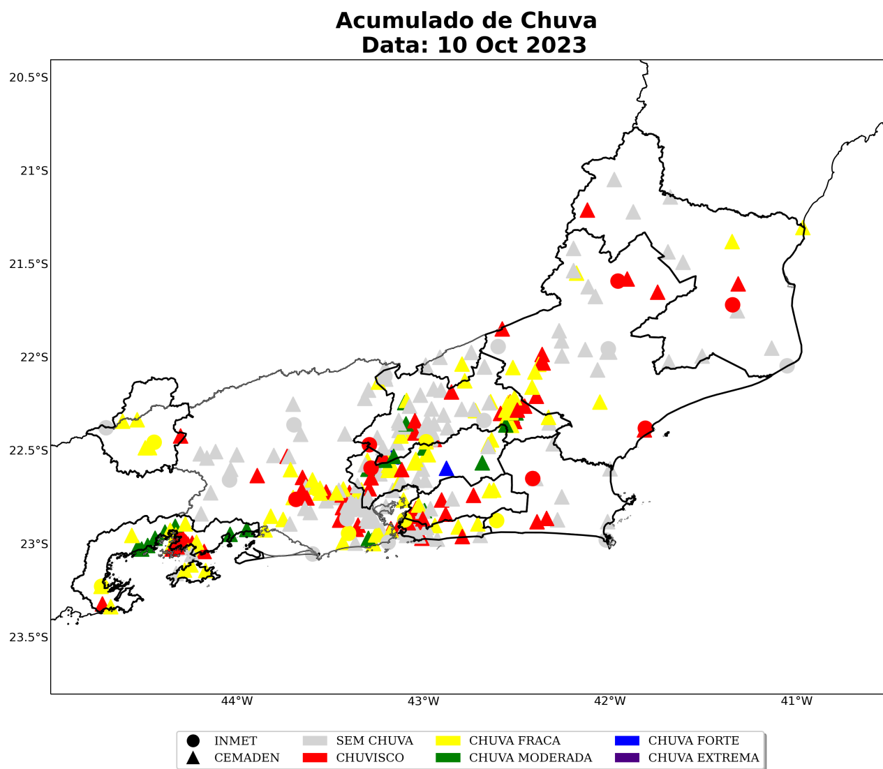
Figura 19: Acumulado diário de precipitação sobre a área de concessão da Enel-RJ para o dia 10 de outubro, baseado nas estações meteorológicas do INMET e CEMADEN.
