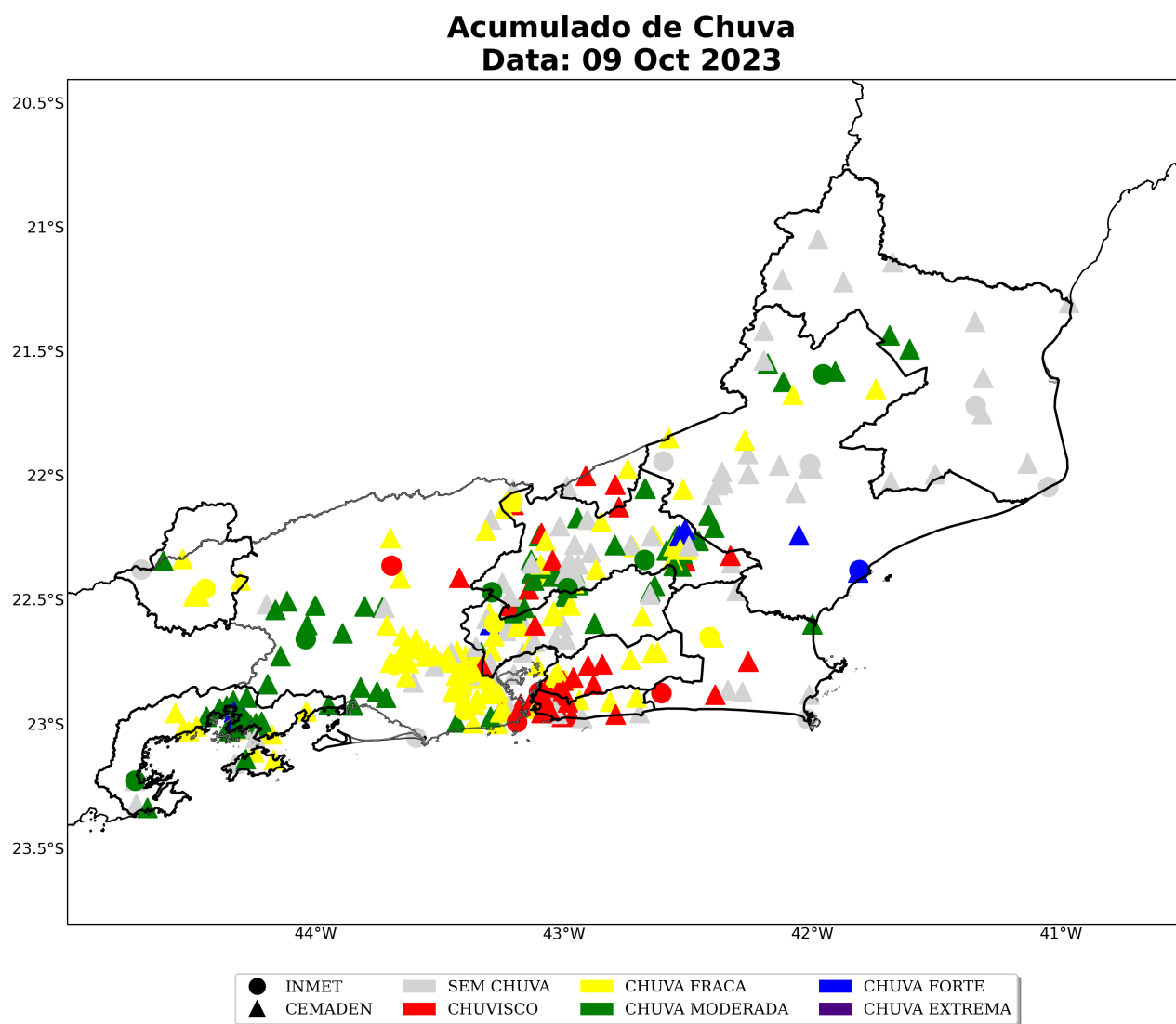
Figura 18: Acumulado diário de precipitação sobre a área de concessão da Enel-RJ para o dia 09 de outubro, baseado nas estações meteorológicas do INMET e CEMADEN.
