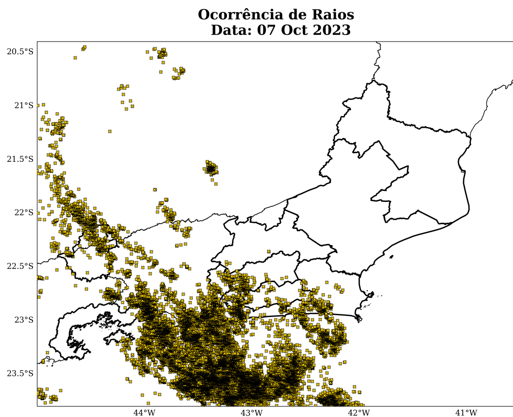
Figura 10: Total de descargas atmosféricas nuvem-solo detectadas pelo sistema Earth Networks para o dia 07 de outubro sobre a área de concessão da Enel-RJ.
