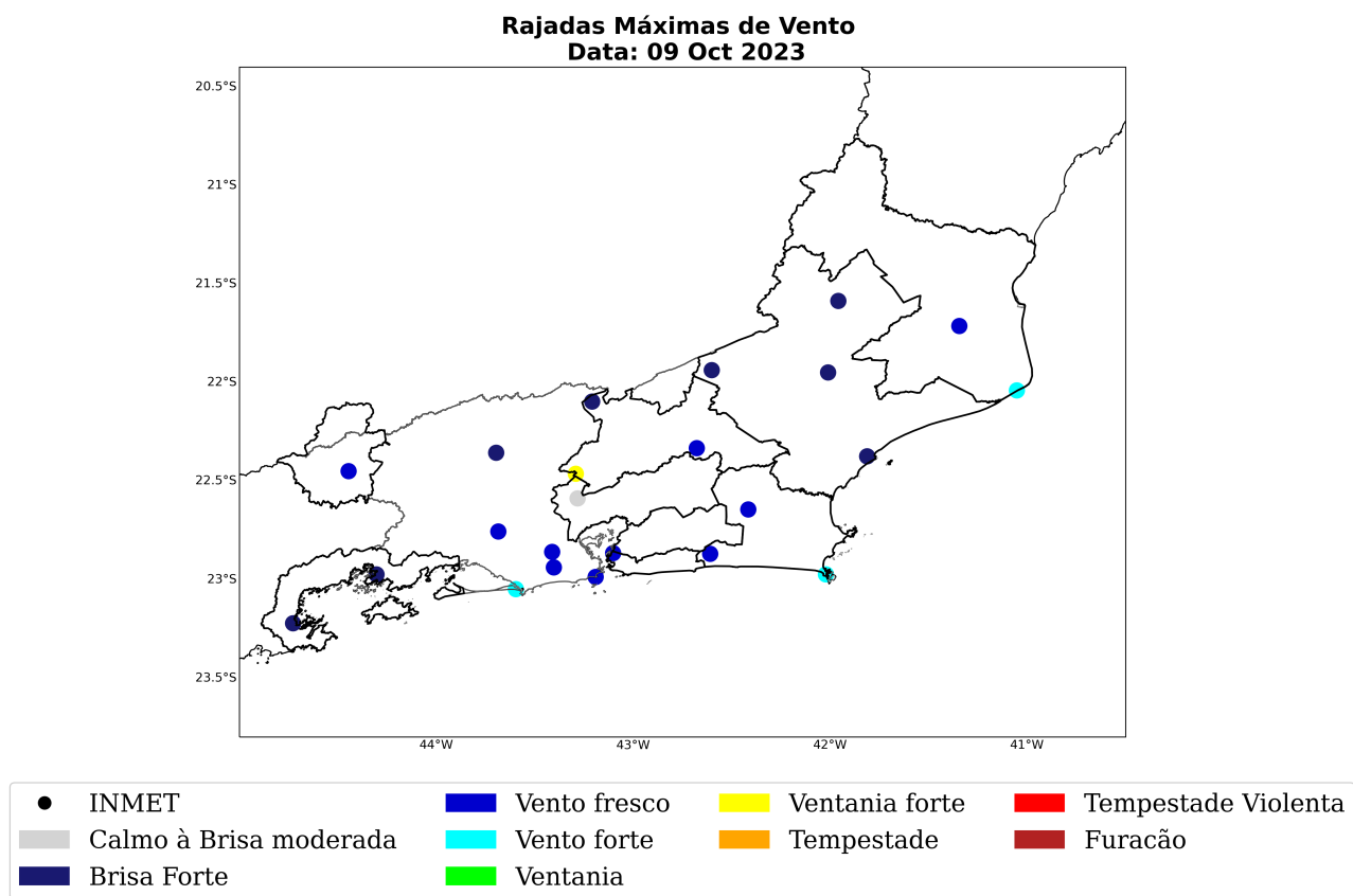
Figura 25: Máxima rajada de vento diária sobre a área de concessão da Enel-RJ para o dia 09 de outubro, baseado nas estações meteorológicas do INMET.
