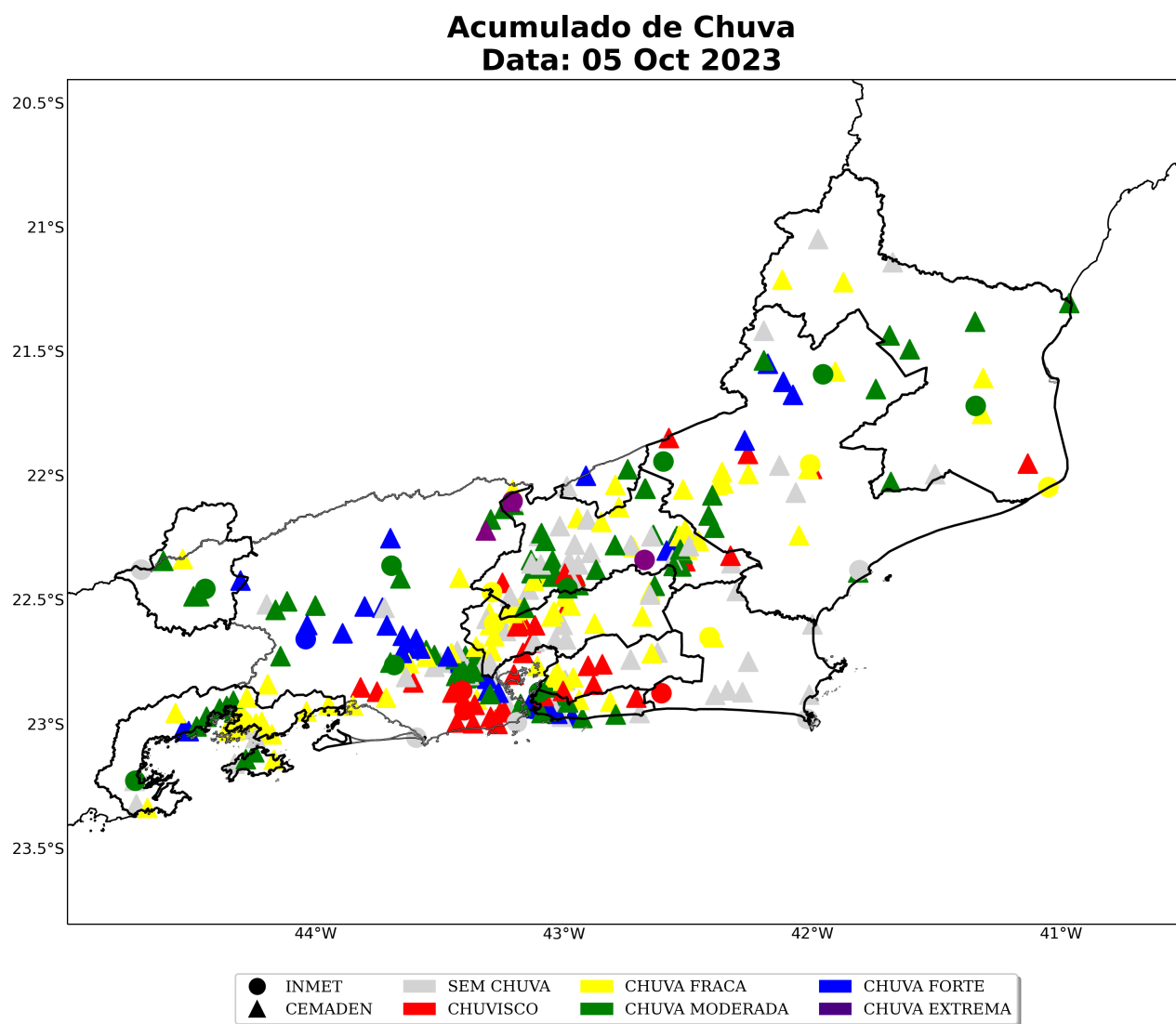
Figura 14: Acumulado diário de precipitação sobre a área de concessão da Enel-RJ para o dia 05 de outubro, baseado nas estações meteorológicas do INMET e CEMADEN.
