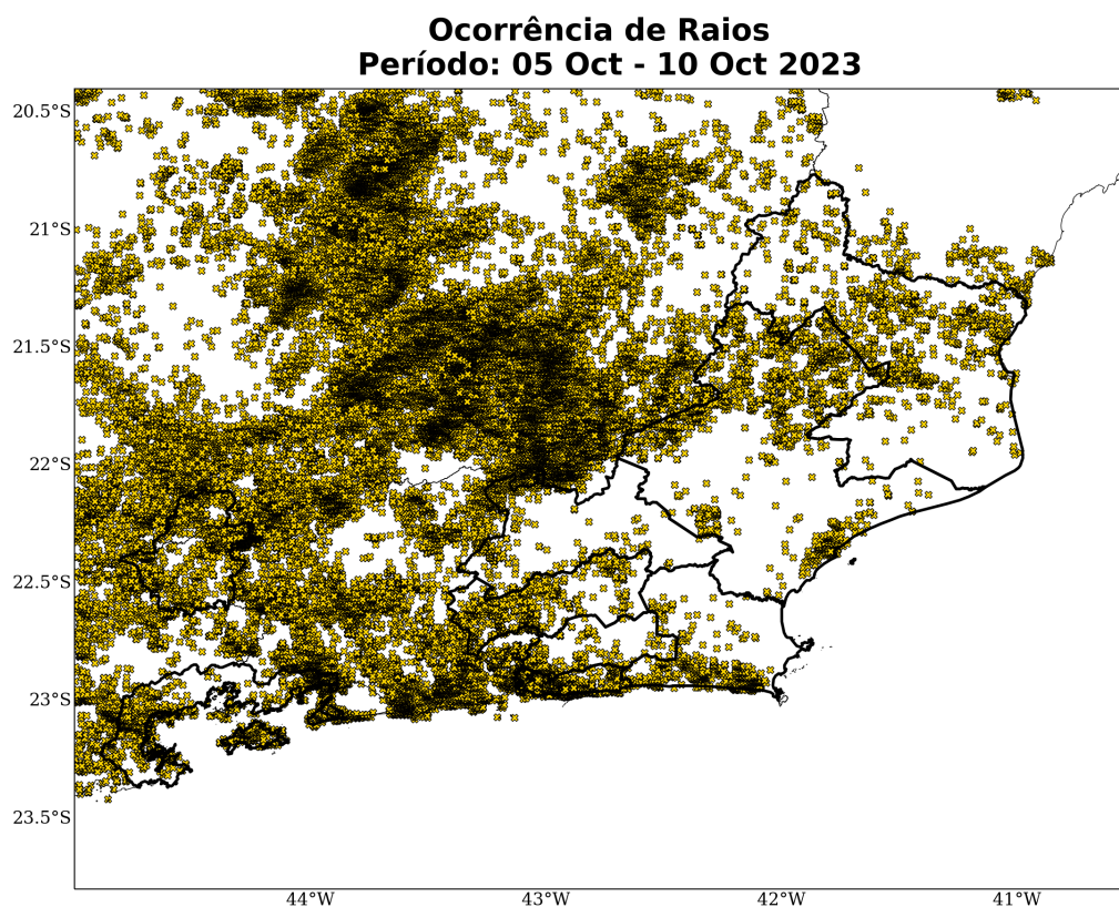
Figura 13: Total de descargas atmosféricas nuvem-solo detectadas pelo sistema Earth Networks durante o período de 05 a 10 de outubro de 2023 sobre a área de concessão da Enel-RJ.
