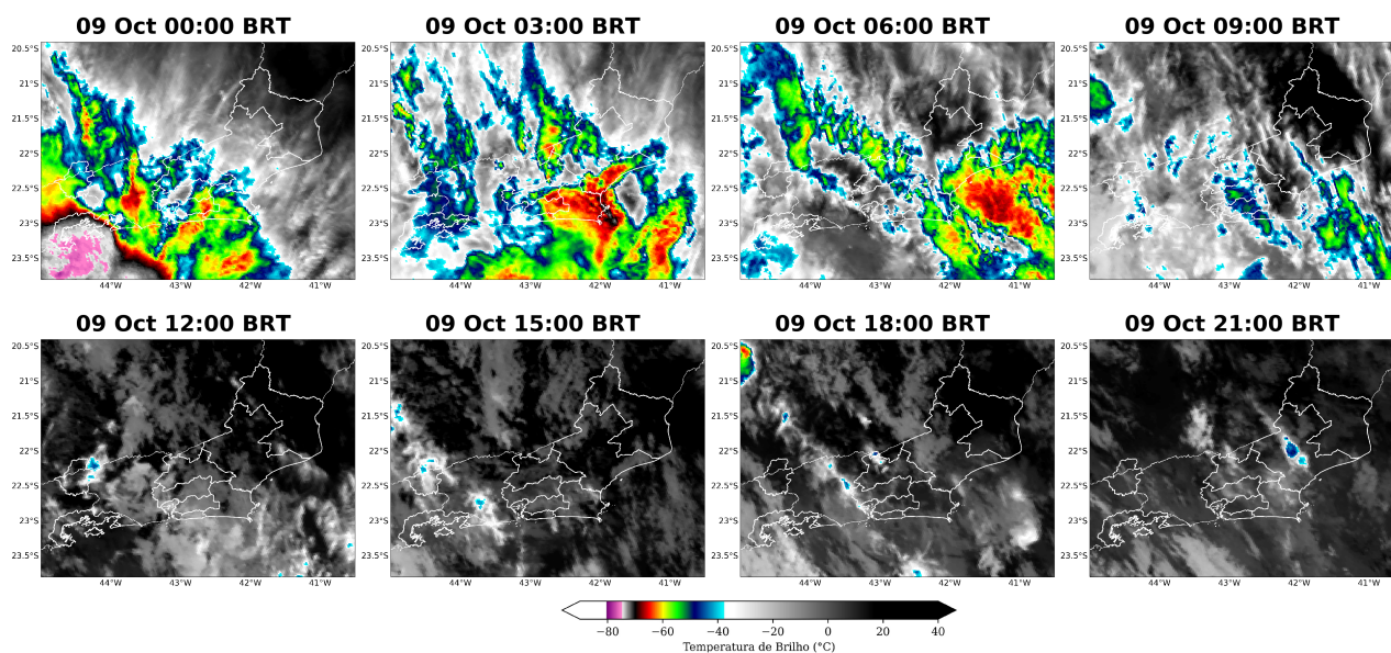
Figura 6: Imagens realçadas do satélite GOES-16 das 00 BRT até 21 BRT (a cada 3 horas) para o dia 09 de outubro.
