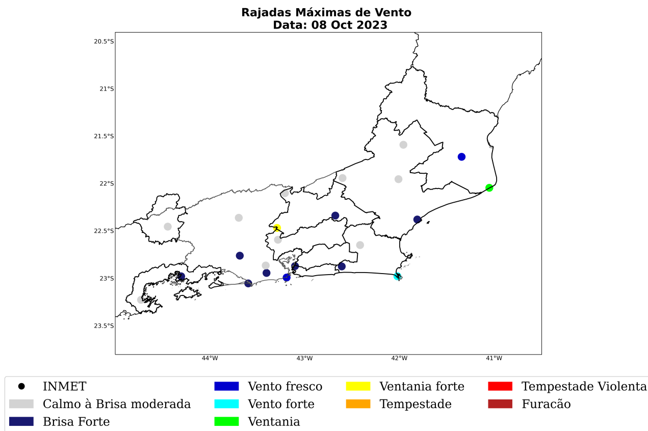
Figura 24: Máxima rajada de vento diária sobre a área de concessão da Enel-RJ para o dia 08 de outubro, baseado nas estações meteorológicas do INMET.
