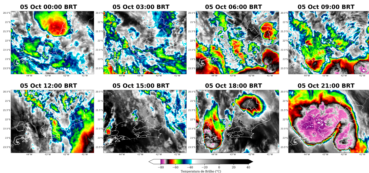
Figura 2: Imagens realçadas do satélite GOES-16 das 00 BRT até 21 BRT (a cada 3 horas) para o dia 05 de outubro.
