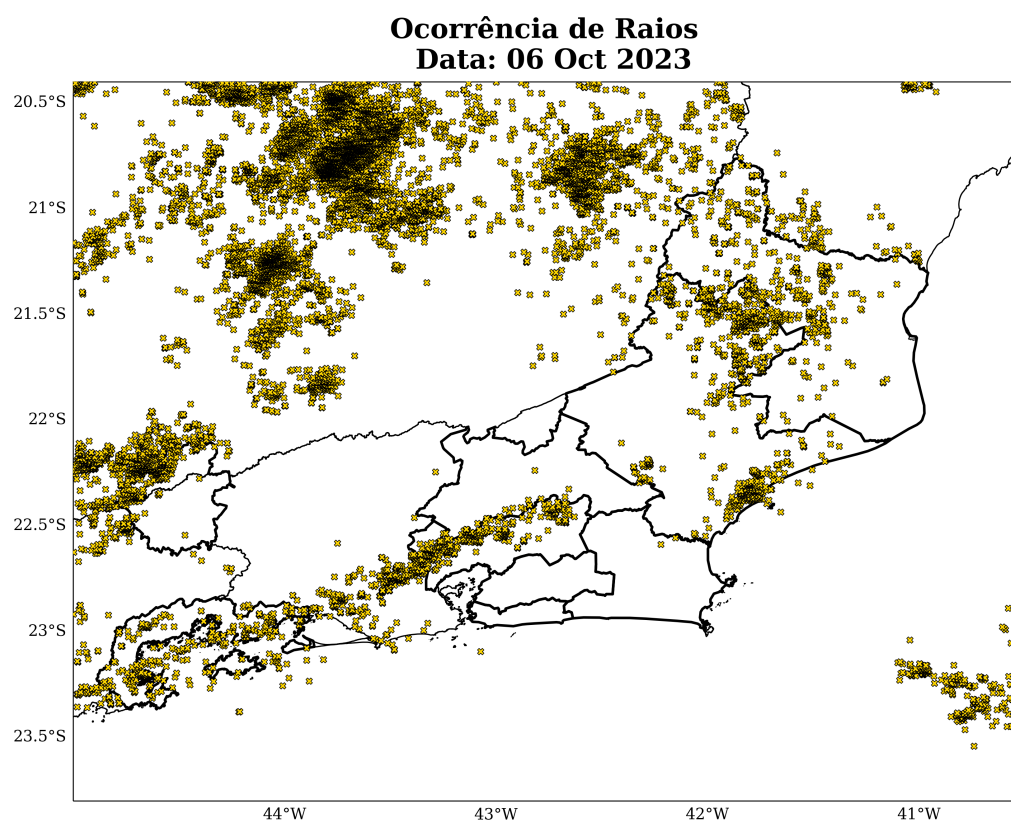
Figura 9: Total de descargas atmosféricas nuvem-solo detectadas pelo sistema Earth Networks para o dia 06 de outubro sobre a área de concessão da Enel-RJ.
