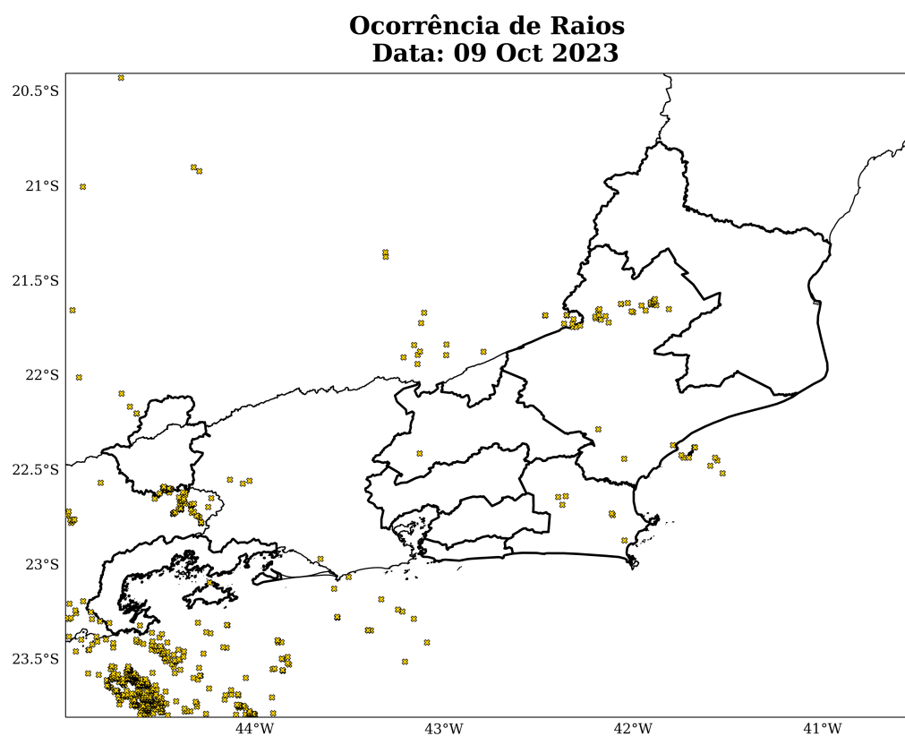
Figura 12: Total de descargas atmosféricas nuvem-solo detectadas pelo sistema Earth Networks para o dia 09 de outubro sobre a área de concessão da Enel-RJ.
