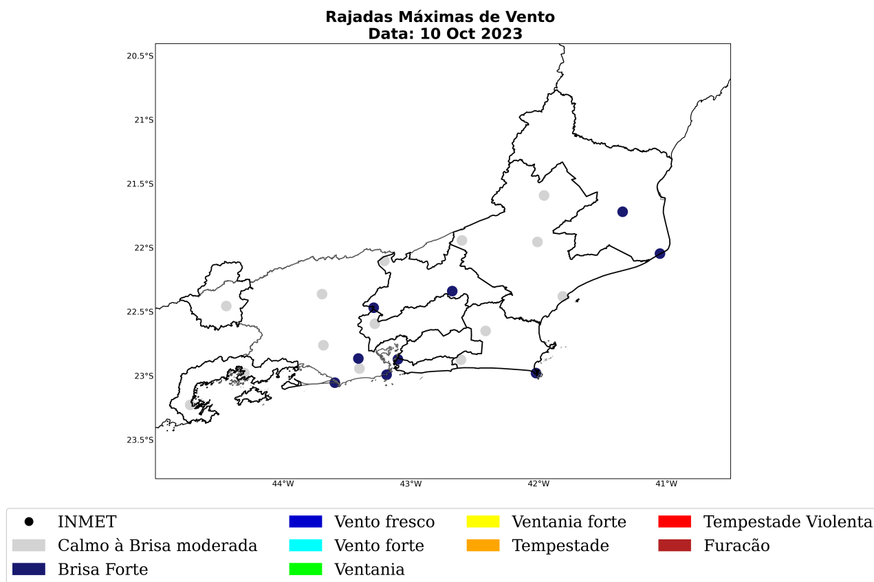
Figura 26: Máxima rajada de vento diária sobre a área de concessão da Enel-RJ para o dia 10 de outubro, baseado nas estações meteorológicas do INMET.
