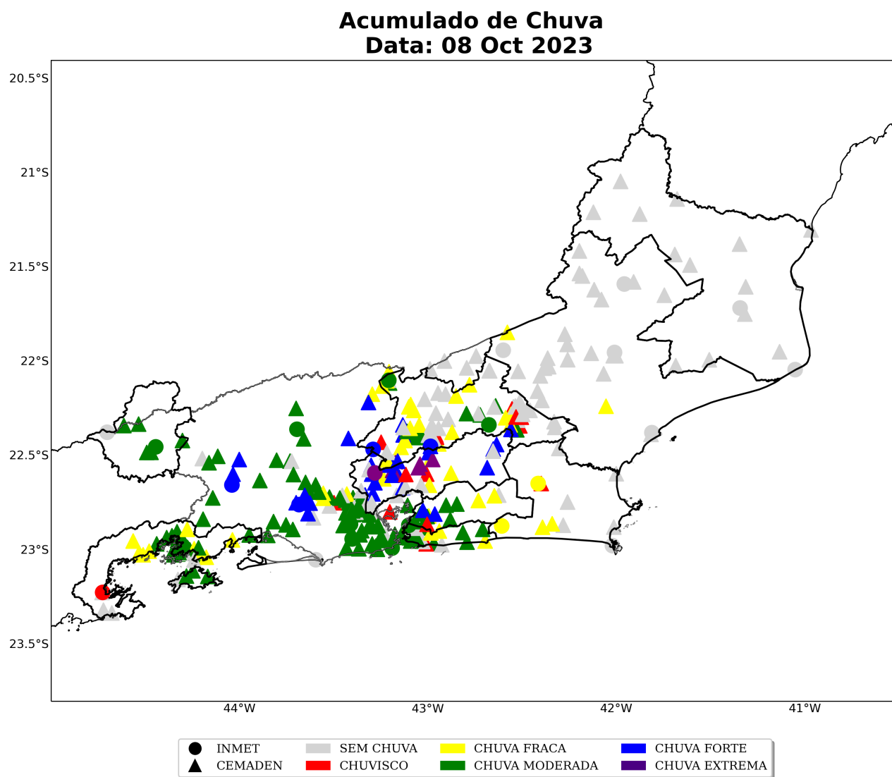
Figura 17: Acumulado diário de precipitação sobre a área de concessão da Enel-RJ para o dia 08 de outubro, baseado nas estações meteorológicas do INMET e CEMADEN.
