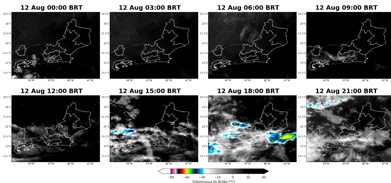
Figura 7: Imagens realçadas do satélite GOES-16 das 00 BRT até 21 BRT (a cada 3 horas) para o dia 12 de agosto.
