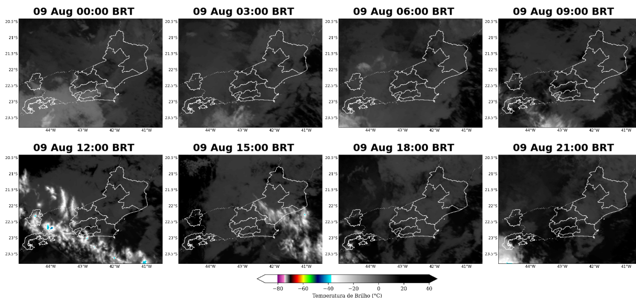
Figura 4: Imagens realçadas do satélite GOES-16 das 00 BRT até 21 BRT (a cada 3 horas) para o dia 09 de agosto.
