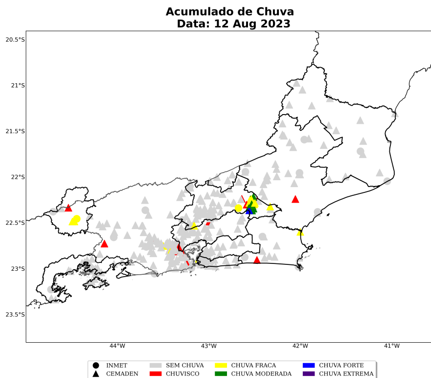
Figura 20: Acumulado diário de precipitação sobre a área de concessão da Enel-RJ para o dia 12 de agosto, baseado nas estações meteorológicas do INMET e CEMADEN.
