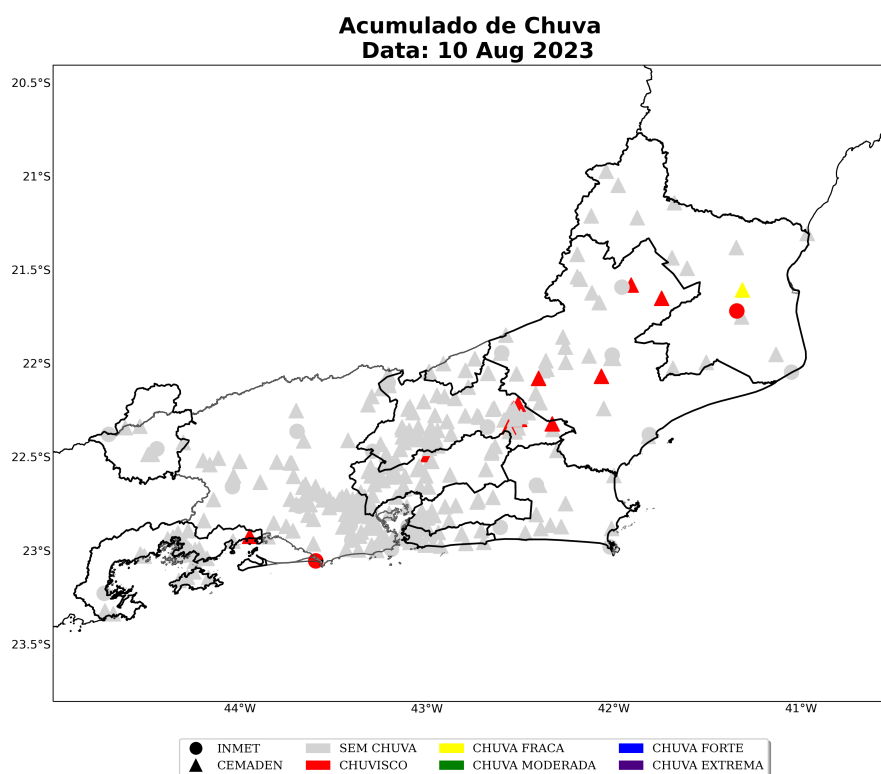
Figura 18: Acumulado diário de precipitação sobre a área de concessão da Enel-RJ para o dia 10 de agosto, baseado nas estações meteorológicas do INMET e CEMADEN.
