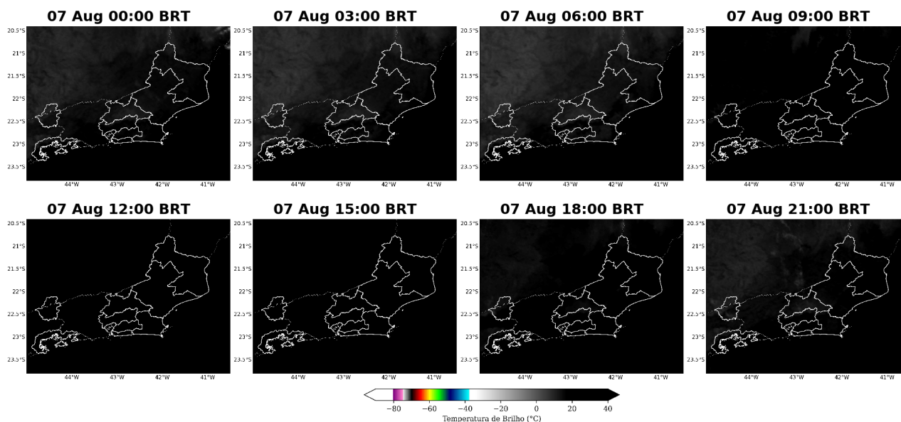
Figura 2: Imagens realçadas do satélite GOES-16 das 00 BRT até 21 BRT (a cada 3 horas) para o dia 07 de agosto.
