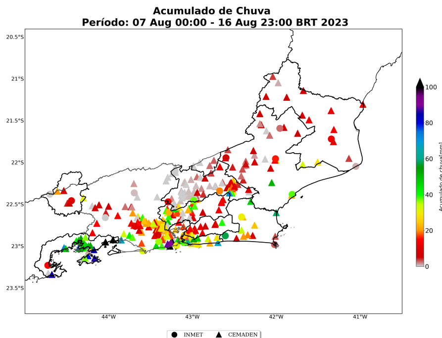
Figura 25: Acumulado total de precipitação sobre a área de concessão da Enel-RJ para o período de 07 a 16 de agosto de 2023, baseado nas estações meteorológicas do INMET e CEMADEN.
