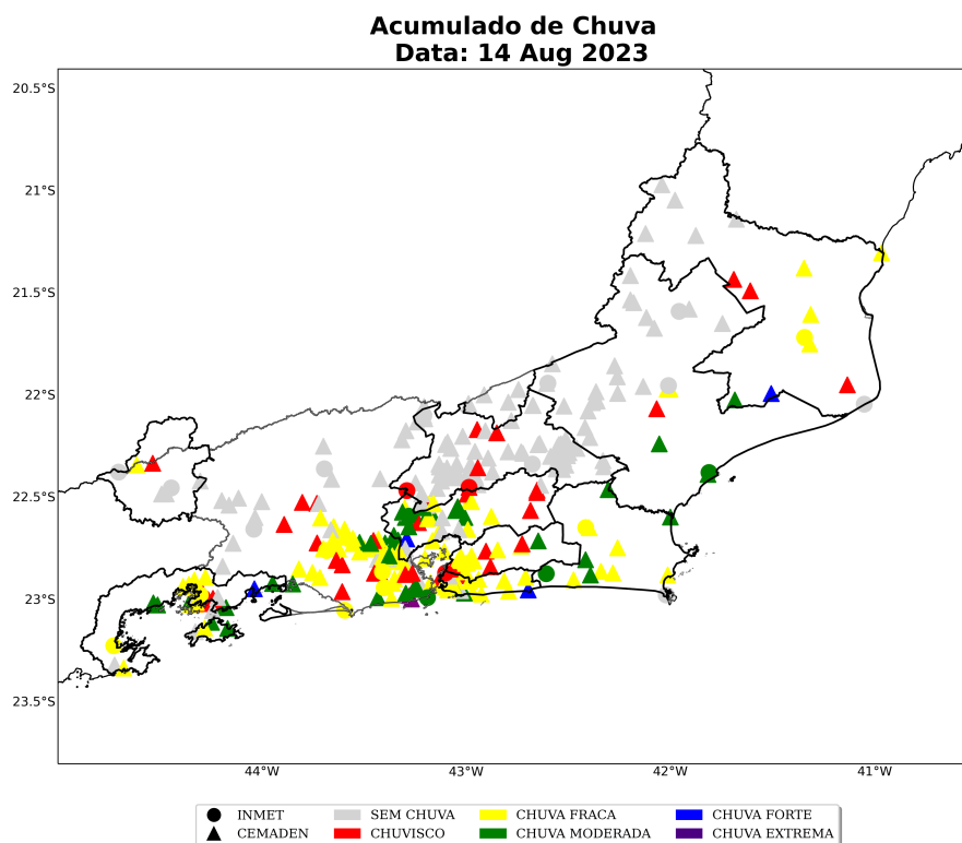
Figura 22: Acumulado diário de precipitação sobre a área de concessão da Enel-RJ para o dia 14 de agosto, baseado nas estações meteorológicas do INMET e CEMADEN.
