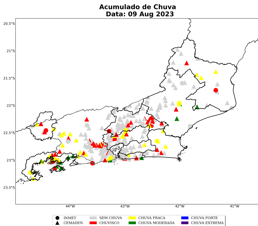
Figura 17: Acumulado diário de precipitação sobre a área de concessão da Enel-RJ para o dia 09 de agosto, baseado nas estações meteorológicas do INMET e CEMADEN.
