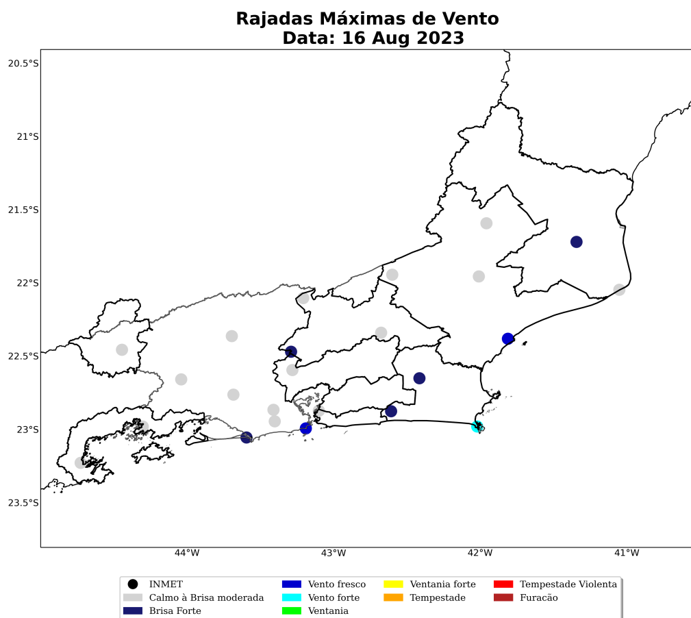
Figura 35: Máxima rajada de vento diária sobre a área de concessão da Enel-RJ para o dia 16 de agosto, baseado nas estações meteorológicas do INMET.
