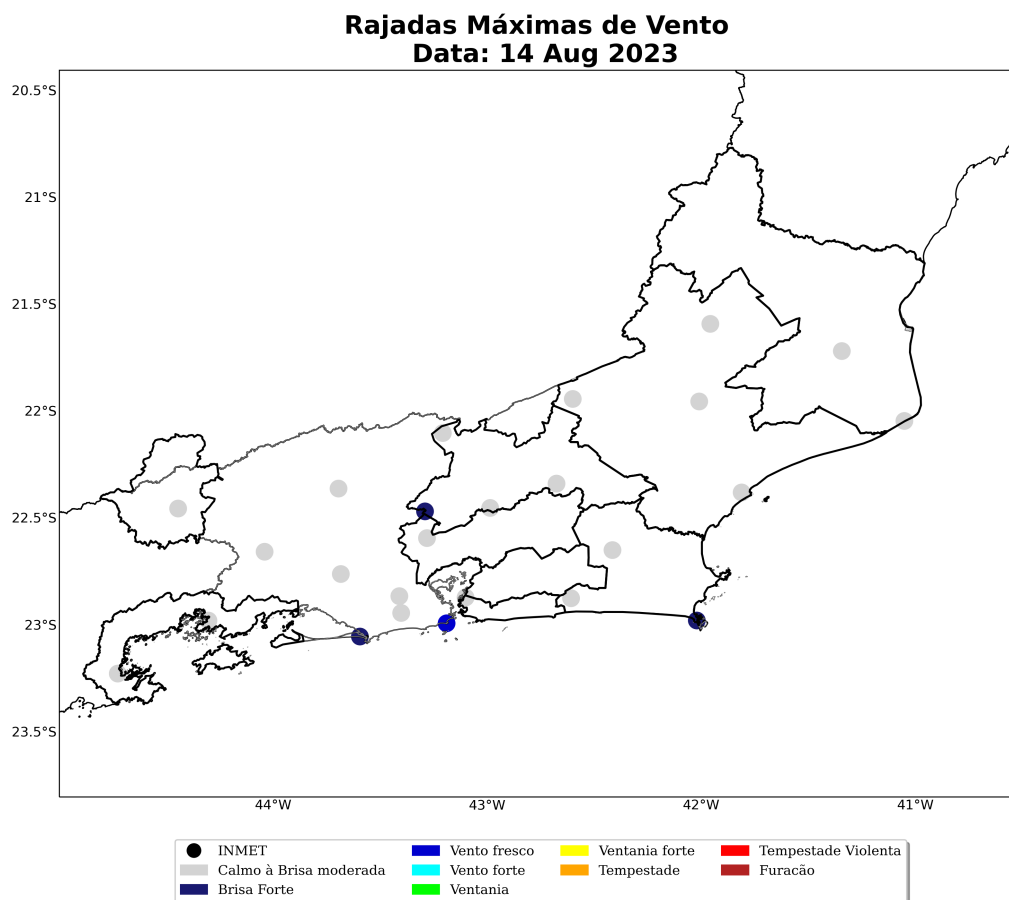
Figura 33: Máxima rajada de vento diária sobre a área de concessão da Enel-RJ para o dia 14 de agosto, baseado nas estações meteorológicas do INMET.
