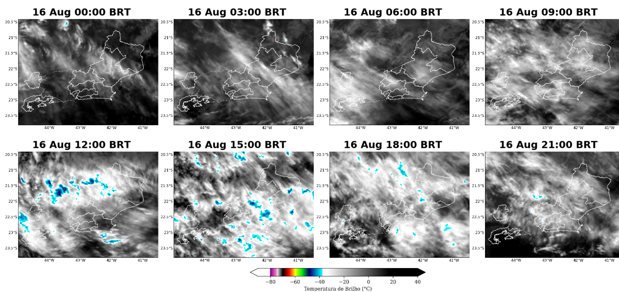
Figura 11: Imagens realçadas do satélite GOES-16 das 00 BRT até 21 BRT (a cada 3 horas) para o dia 16 de agosto.
