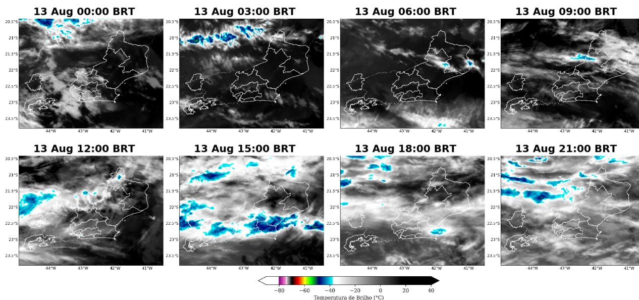
Figura 8: Imagens realçadas do satélite GOES-16 das 00 BRT até 21 BRT (a cada 3 horas) para o dia 13 de agosto.
