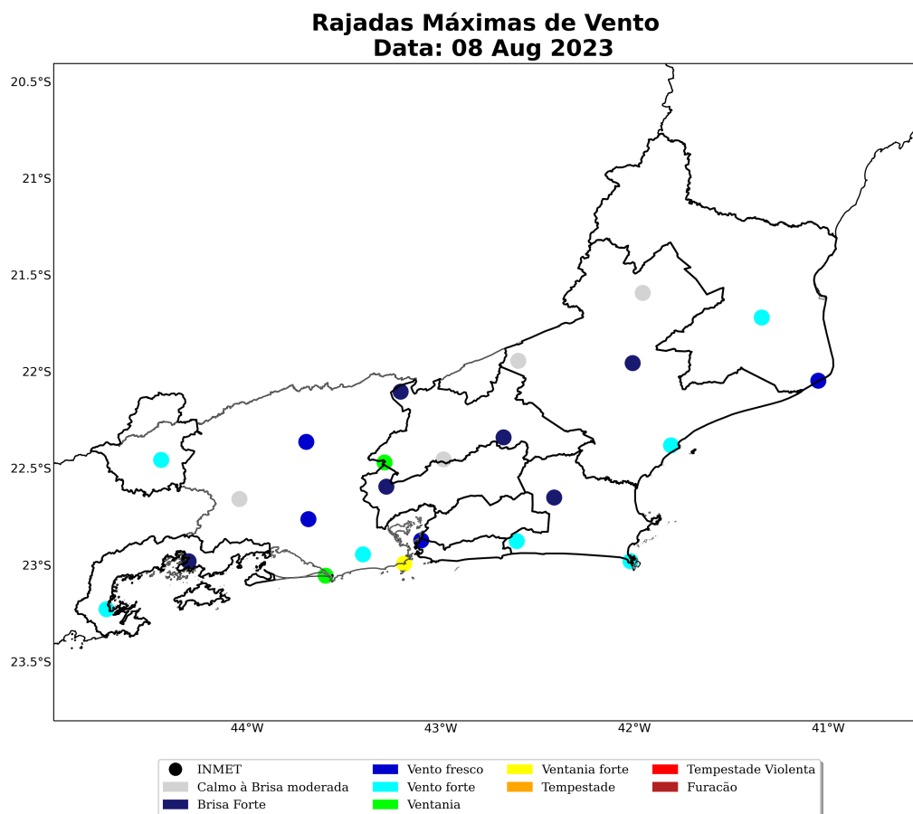
Figura 27: Máxima rajada de vento diária sobre a área de concessão da Enel-RJ para o dia 08 de agosto, baseado nas estações meteorológicas do INMET.
