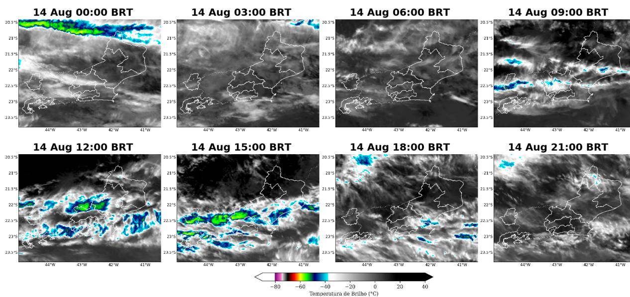
Figura 9: Imagens realçadas do satélite GOES-16 das 00 BRT até 21 BRT (a cada 3 horas) para o dia 14 de agosto.
