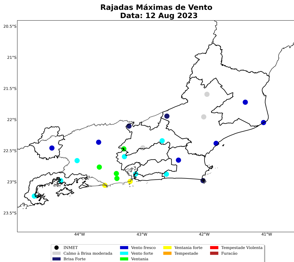
Figura 31: Máxima rajada de vento diária sobre a área de concessão da Enel-RJ para o dia 12 de agosto, baseado nas estações meteorológicas do INMET.
