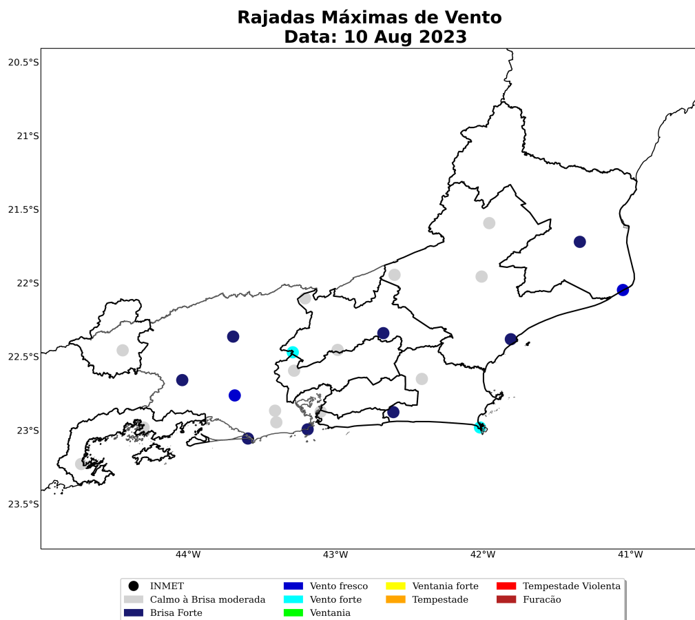
Figura 29: Máxima rajada de vento diária sobre a área de concessão da Enel-RJ para o dia 10 de agosto, baseado nas estações meteorológicas do INMET.
