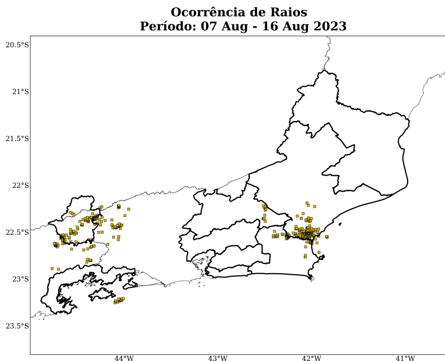
Figura 14: Densidade de descargas atmosféricas nuvem-solo detectadas pelo sistema Earth Networks durante o período de 07 a 16 de agosto de 2023 sobre a área de concessão da Enel-RJ.
