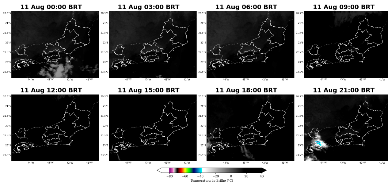
Figura 6: Imagens realçadas do satélite GOES-16 das 00 BRT até 21 BRT (a cada 3 horas) para o dia 11 de agosto.
