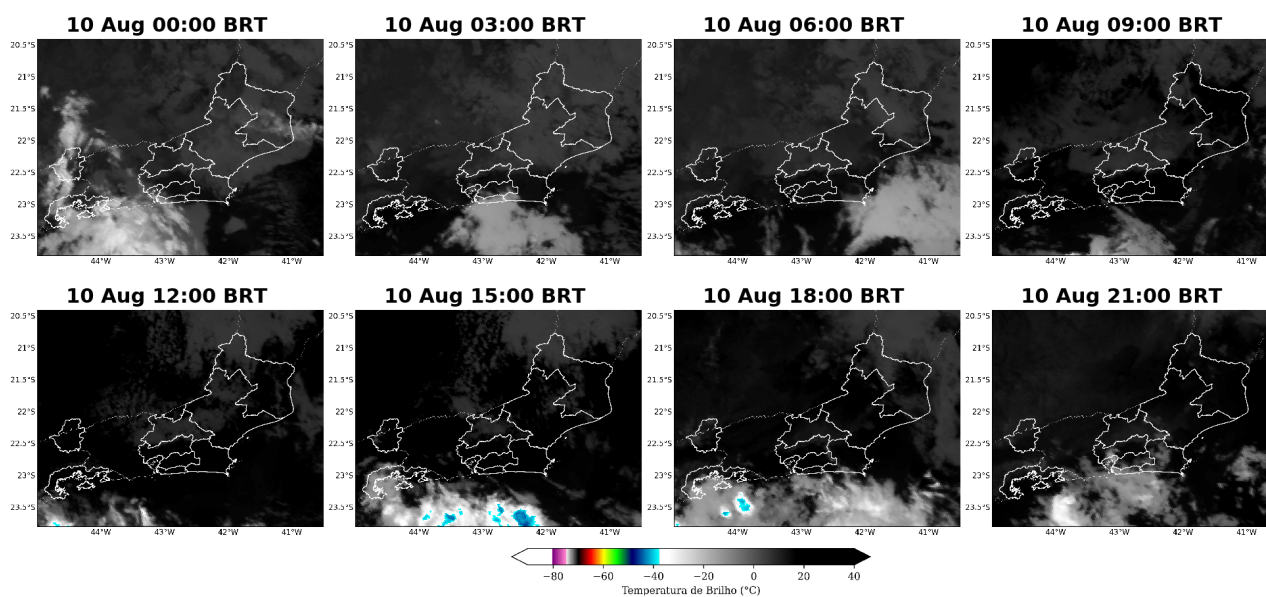
Figura 5: Imagens realçadas do satélite GOES-16 das 00 BRT até 21 BRT (a cada 3 horas) para o dia 10 de agosto.
