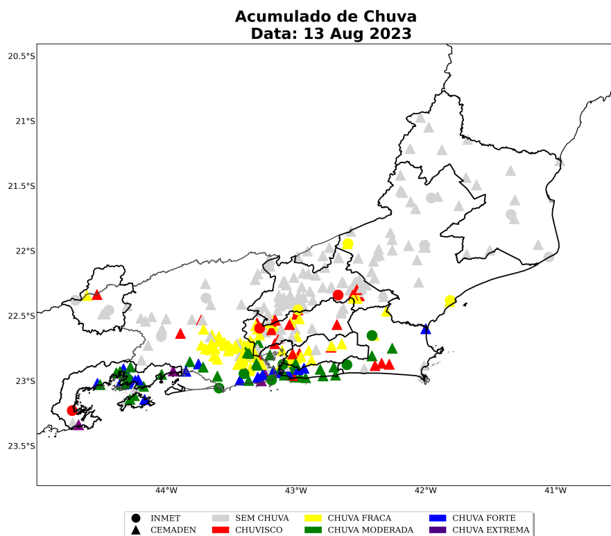
Figura 21: Acumulado diário de precipitação sobre a área de concessão da Enel-RJ para o dia 13 de agosto, baseado nas estações meteorológicas do INMET e CEMADEN.
