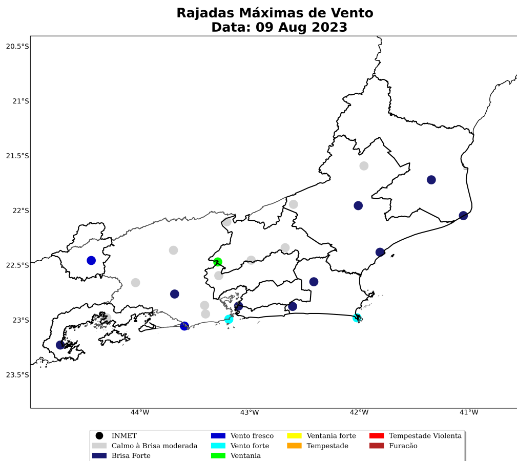
Figura 28: Máxima rajada de vento diária sobre a área de concessão da Enel-RJ para o dia 09 de agosto, baseado nas estações meteorológicas do INMET.
