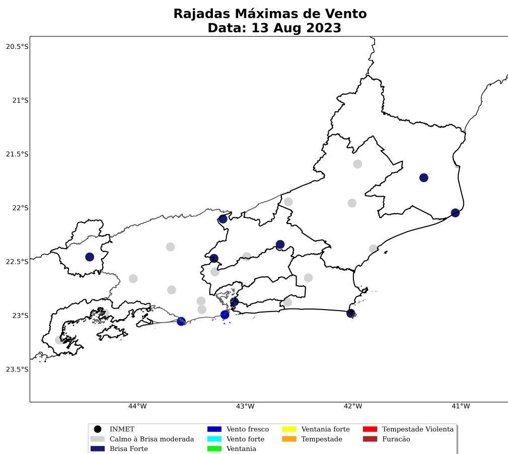
Figura 32: Máxima rajada de vento diária sobre a área de concessão da Enel-RJ para o dia 13 de agosto, baseado nas estações meteorológicas do INMET.
