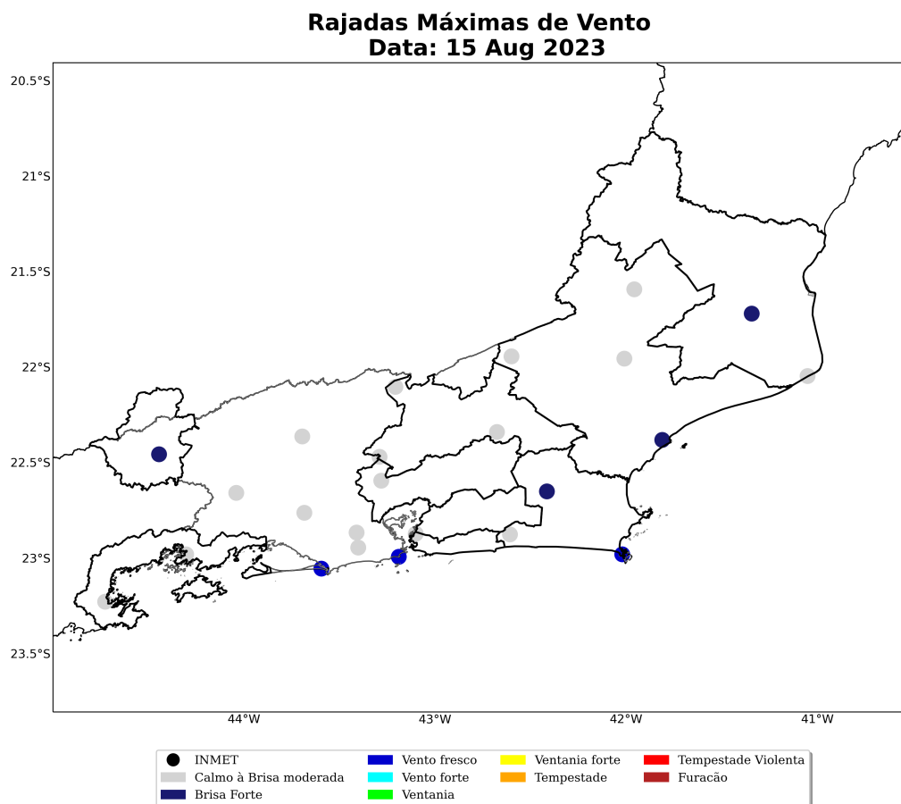
Figura 34: Máxima rajada de vento diária sobre a área de concessão da Enel-RJ para o dia 15 de agosto, baseado nas estações meteorológicas do INMET.
