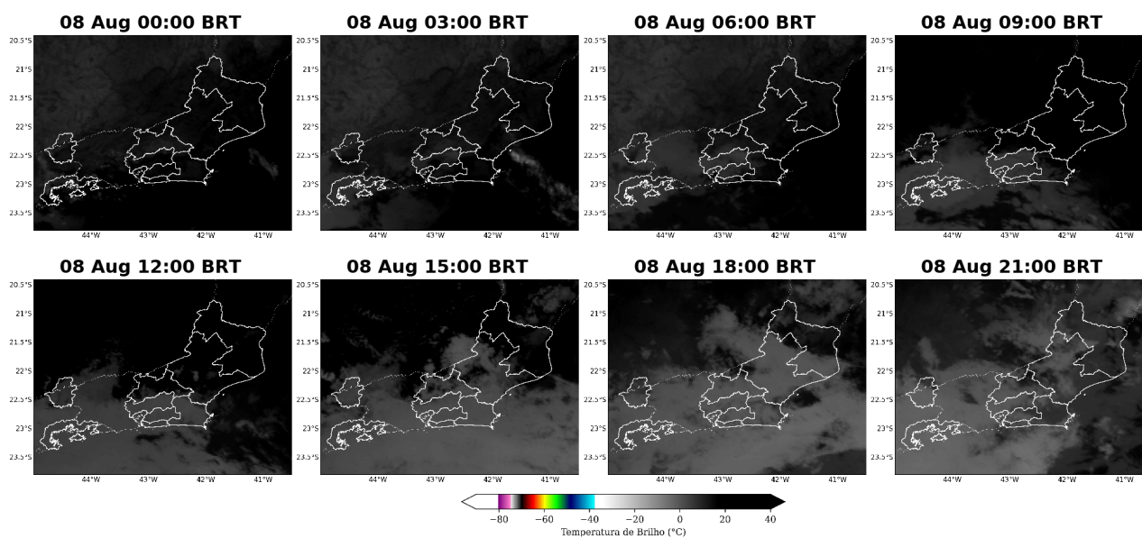
Figura 3: Imagens realçadas do satélite GOES-16 das 00 BRT até 21 BRT (a cada 3 horas) para o dia 08 de agosto.
