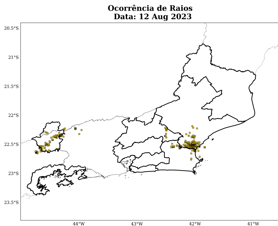
Figura 13: Densidade de descargas atmosféricas nuvem-solo detectadas pelo sistema Earth Networks para o dia 12 de agosto sobre a área de concessão da Enel-RJ.
