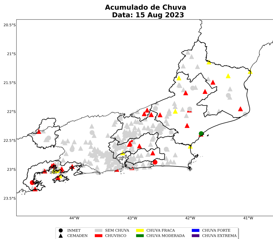
Figura 23: Acumulado diário de precipitação sobre a área de concessão da Enel-RJ para o dia 15 de agosto, baseado nas estações meteorológicas do INMET e CEMADEN.
