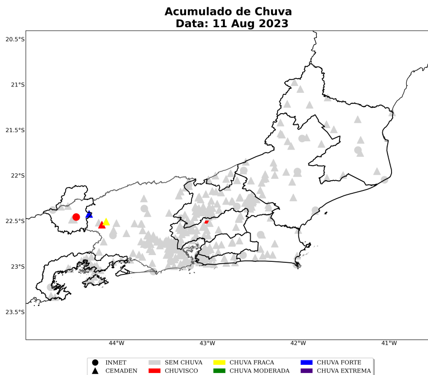
Figura 19: Acumulado diário de precipitação sobre a área de concessão da Enel-RJ para o dia 11 de agosto, baseado nas estações meteorológicas do INMET e CEMADEN.
