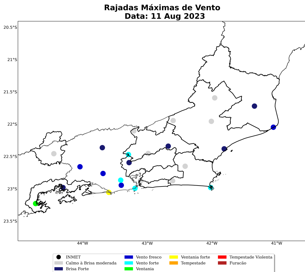
Figura 30: Máxima rajada de vento diária sobre a área de concessão da Enel-RJ para o dia 11 de agosto, baseado nas estações meteorológicas do INMET.
