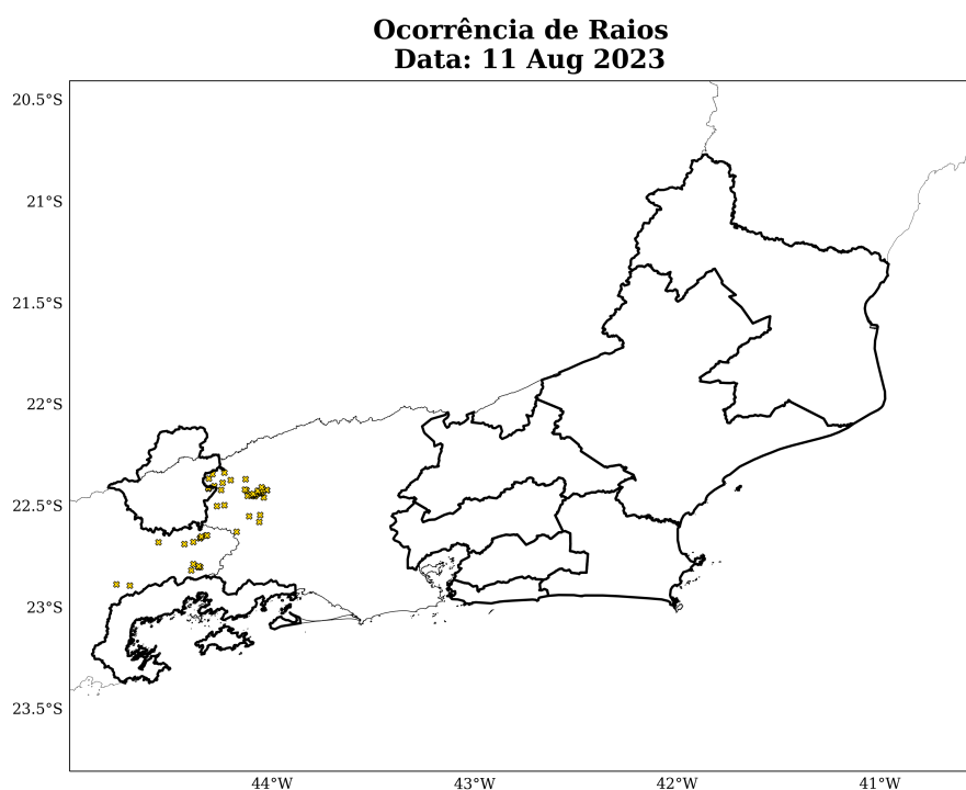
Figura 12: Densidade de descargas atmosféricas nuvem-solo detectadas pelo sistema Earth Networks para o dia 11 de agosto sobre a área de concessão da Enel-RJ.
