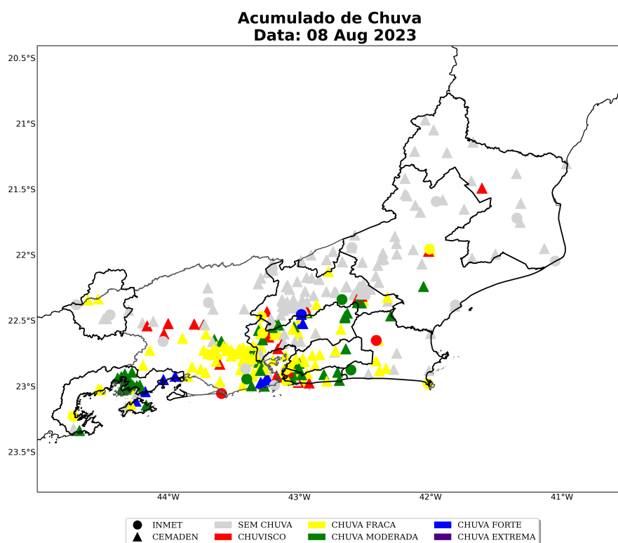
Figura 16: Acumulado diário de precipitação sobre a área de concessão da Enel-RJ para o dia 08 de agosto, baseado nas estações meteorológicas do INMET e CEMADEN.
