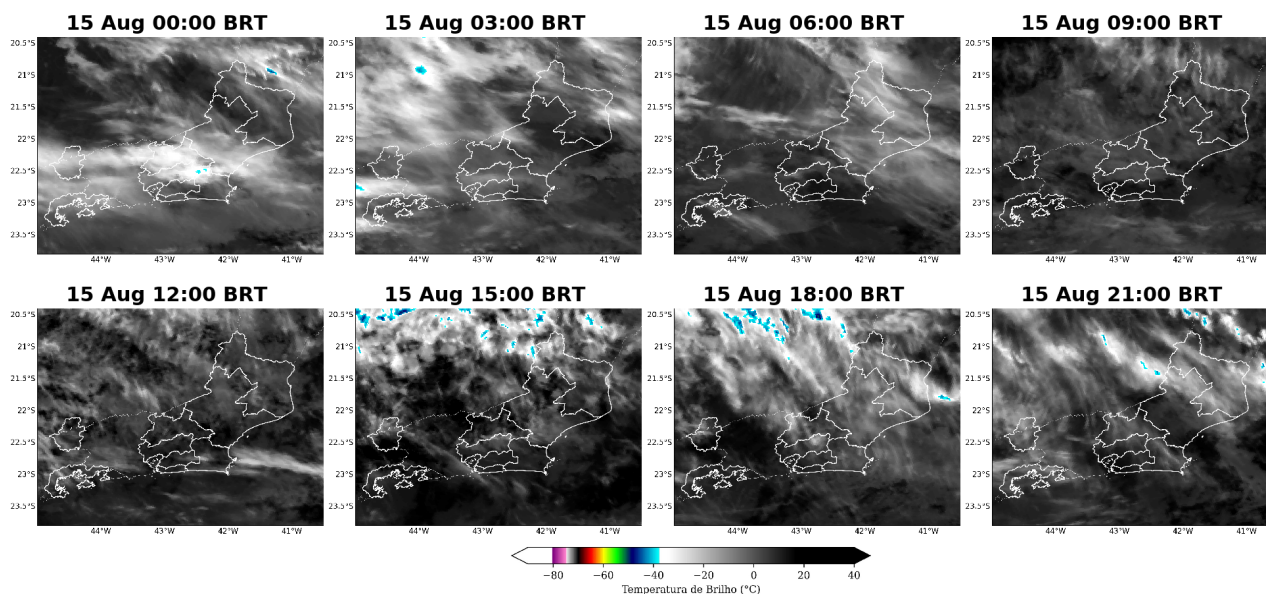
Figura 10: Imagens realçadas do satélite GOES-16 das 00 BRT até 21 BRT (a cada 3 horas) para o dia 15 de agosto.
