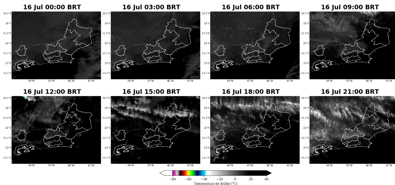
Figura 5: Imagens realçadas do satélite GOES-16 das 00 BRT até 21 BRT (a cada 3 horas) para o dia 16 de julho.
