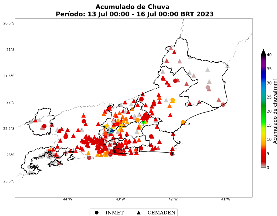
Figura 10: Acumulado total de precipitação sobre a área de concessão da Enel-RJ para o período de 13 a 16 de julho de 2023, baseado nas estações meteorológicas do INMET e CEMADEN.
