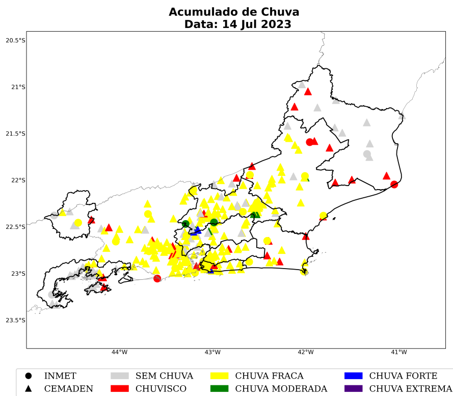
Figura 7: Acumulado diário de precipitação sobre a área de concessão da Enel-RJ para o dia 14 de julho, baseado nas estações meteorológicas do INMET e CEMADEN.
