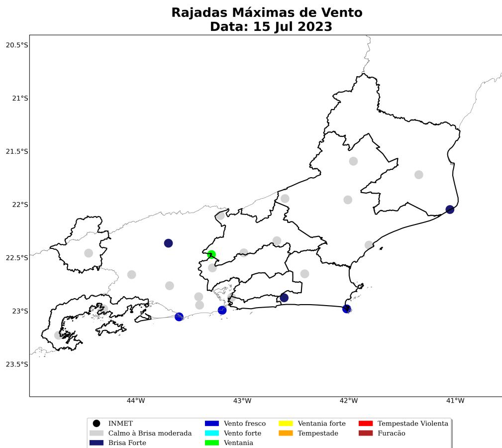
Figura 13: Máxima rajada de vento diária sobre a área de concessão da Enel-RJ para o dia 15 de julho, baseado nas estações meteorológicas do INMET.
