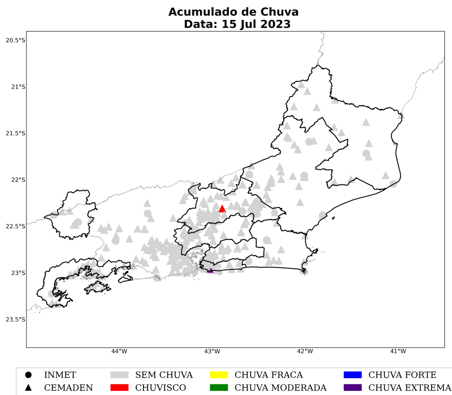
Figura 8: Acumulado diário de precipitação sobre a área de concessão da Enel-RJ para o dia 15 de julho, baseado nas estações meteorológicas do INMET e CEMADEN.
