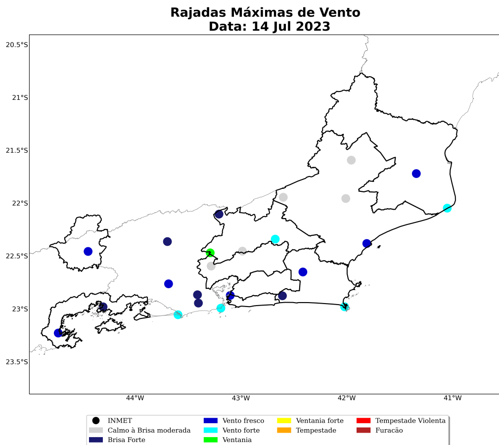
Figura 12: Máxima rajada de vento diária sobre a área de concessão da Enel-RJ para o dia 14 de julho, baseado nas estações meteorológicas do INMET.
