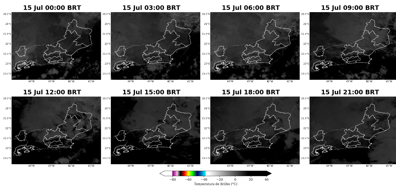
Figura 4: Imagens realçadas do satélite GOES-16 das 00 BRT até 21 BRT (a cada 3 horas) para o dia 15 de julho.
