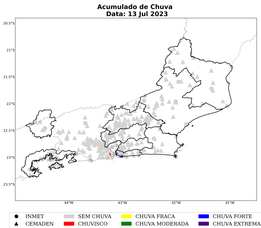
Figura 6: Acumulado diário de precipitação sobre a área de concessão da Enel-RJ para o dia 13 de julho, baseado nas estações meteorológicas do INMET e CEMADEN.
