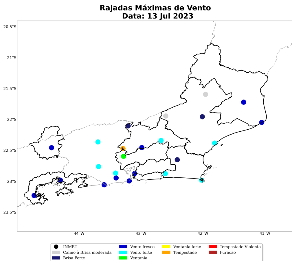
Figura 11: Máxima rajada de vento diária sobre a área de concessão da Enel-RJ para o dia 13 de julho, baseado nas estações meteorológicas do INMET.
