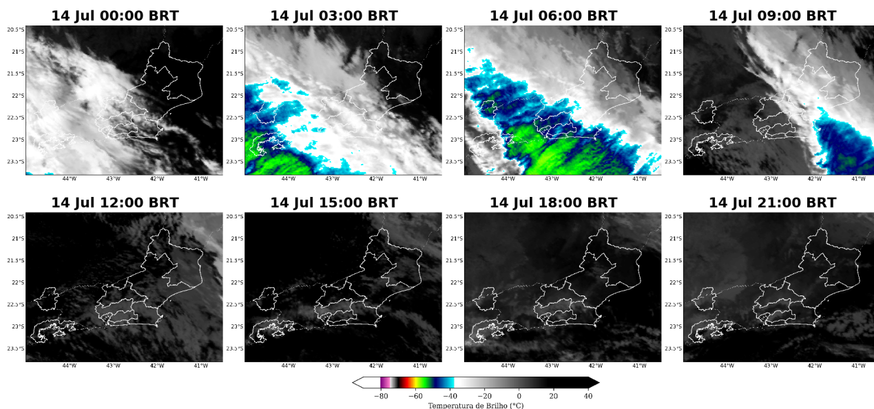
Figura 3: Imagens realçadas do satélite GOES-16 das 00 BRT até 21 BRT (a cada 3 horas) para o dia 14 de julho.
