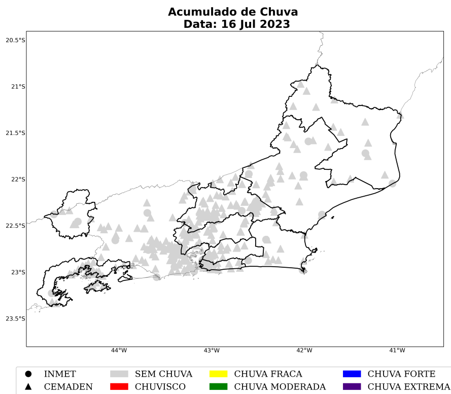
Figura 9: Acumulado diário de precipitação sobre a área de concessão da Enel-RJ para o dia 16 de julho, baseado nas estações meteorológicas do INMET e CEMADEN.
