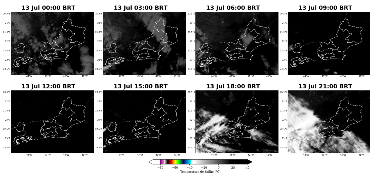
Figura 2: Imagens realçadas do satélite GOES-16 das 00 BRT até 21 BRT (a cada 3 horas) para o dia 13 de julho.
