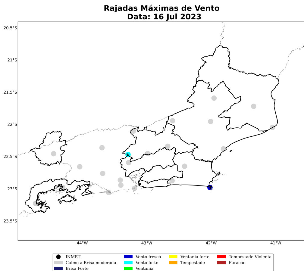
Figura 14: Máxima rajada de vento diária sobre a área de concessão da Enel-RJ para o dia 16 de julho, baseado nas estações meteorológicas do INMET.
