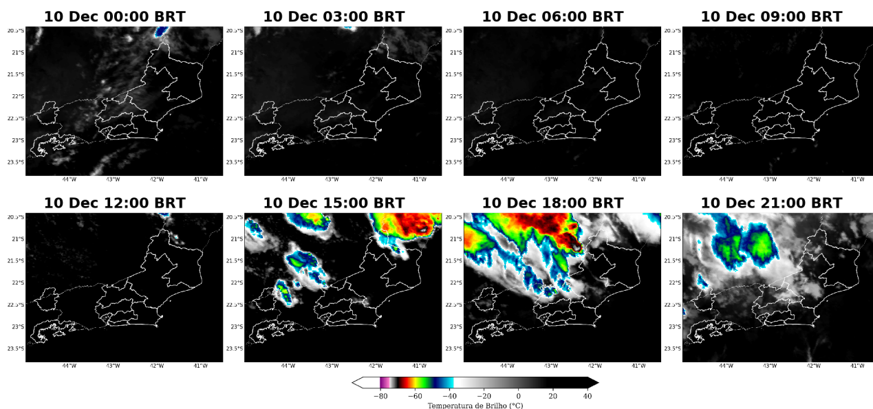
Figura 2: Imagens realçadas do satélite GOES-16 das 00 BRT até 21 BRT (a cada 3 horas) para o dia 10 de dezembro.
