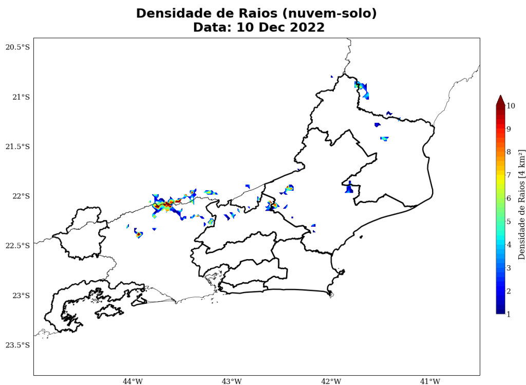
Figura 8: Densidade de descargas atmosféricas nuvem-solo detectadas pelo sistema Earth Networks para o dia 10 de dezembro sobre a área de concessão da Enel-RJ.
