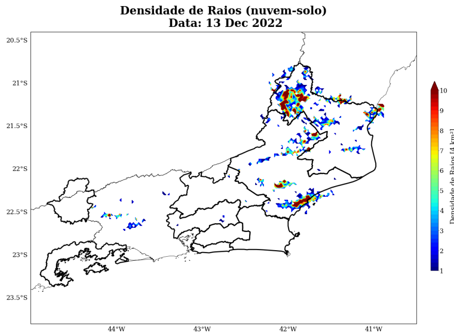
Figura 11: Densidade de descargas atmosféricas nuvem-solo detectadas pelo sistema Earth Networks para o dia 13 de dezembro sobre a área de concessão da Enel-RJ.
