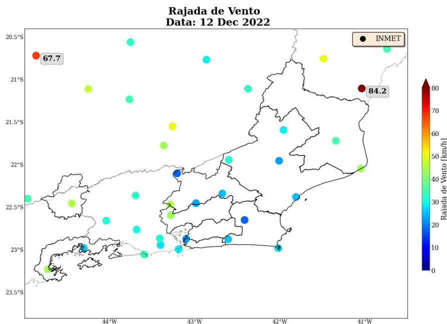
Figura 20: Máxima rajada de vento diária sobre a área de concessão da Enel-RJ para o dia 12 de dezembro, baseado nas estações meteorológicas do INMET.
