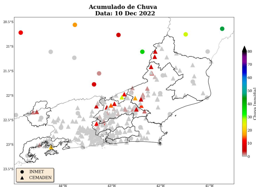
Figura 12: Acumulado diário de precipitação sobre a área de concessão da Enel-RJ para o dia 10 de dezembro, baseado nas estações meteorológicas do INMET e CEMADEN.
