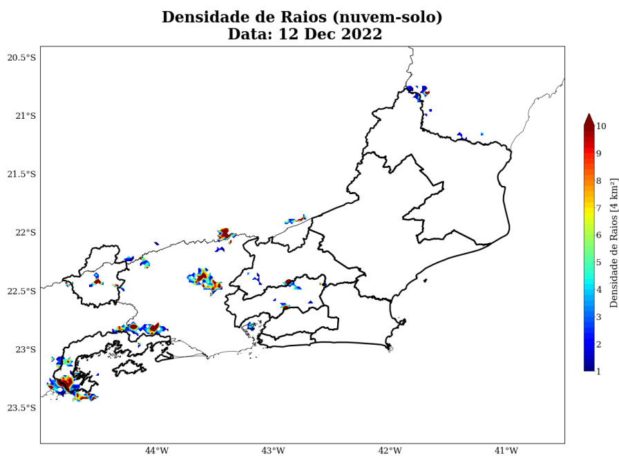
Figura 10: Densidade de descargas atmosféricas nuvem-solo detectadas pelo sistema Earth Networks para o dia 12 de dezembro sobre a área de concessão da Enel-RJ.
