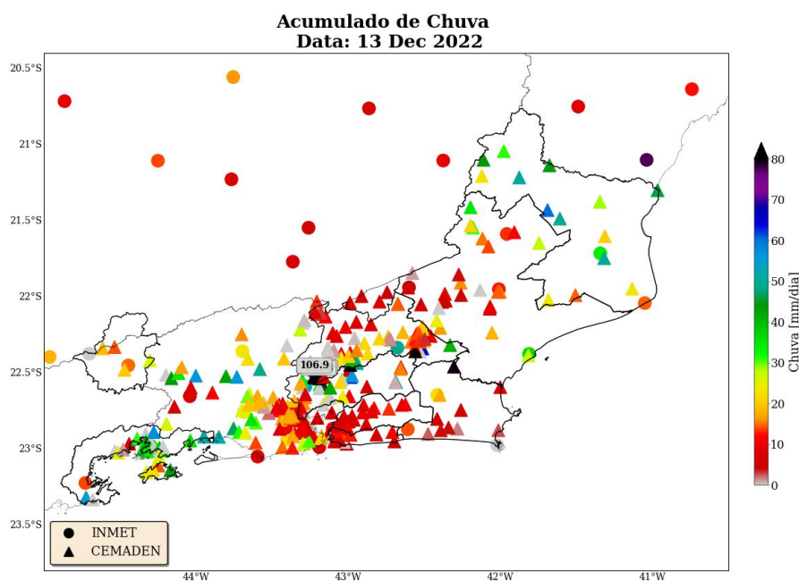
Figura 15: Acumulado diário de precipitação sobre a área de concessão da Enel-RJ para o dia 13 de dezembro, baseado nas estações meteorológicas do INMET e CEMADEN.
