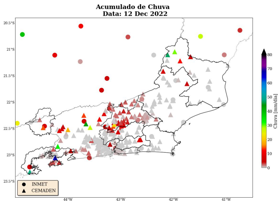
Figura 14: Acumulado diário de precipitação sobre a área de concessão da Enel-RJ para o dia 12 de dezembro, baseado nas estações meteorológicas do INMET e CEMADEN.
