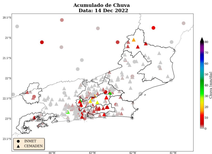
Figura 16: Acumulado diário de precipitação sobre a área de concessão da Enel-RJ para o dia 14 de dezembro, baseado nas estações meteorológicas do INMET e CEMADEN.
