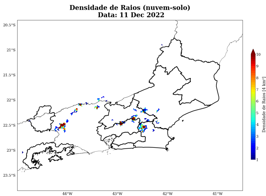
Figura 9: Densidade de descargas atmosféricas nuvem-solo detectadas pelo sistema Earth Networks para o dia 11 de dezembro sobre a área de concessão da Enel-RJ.
