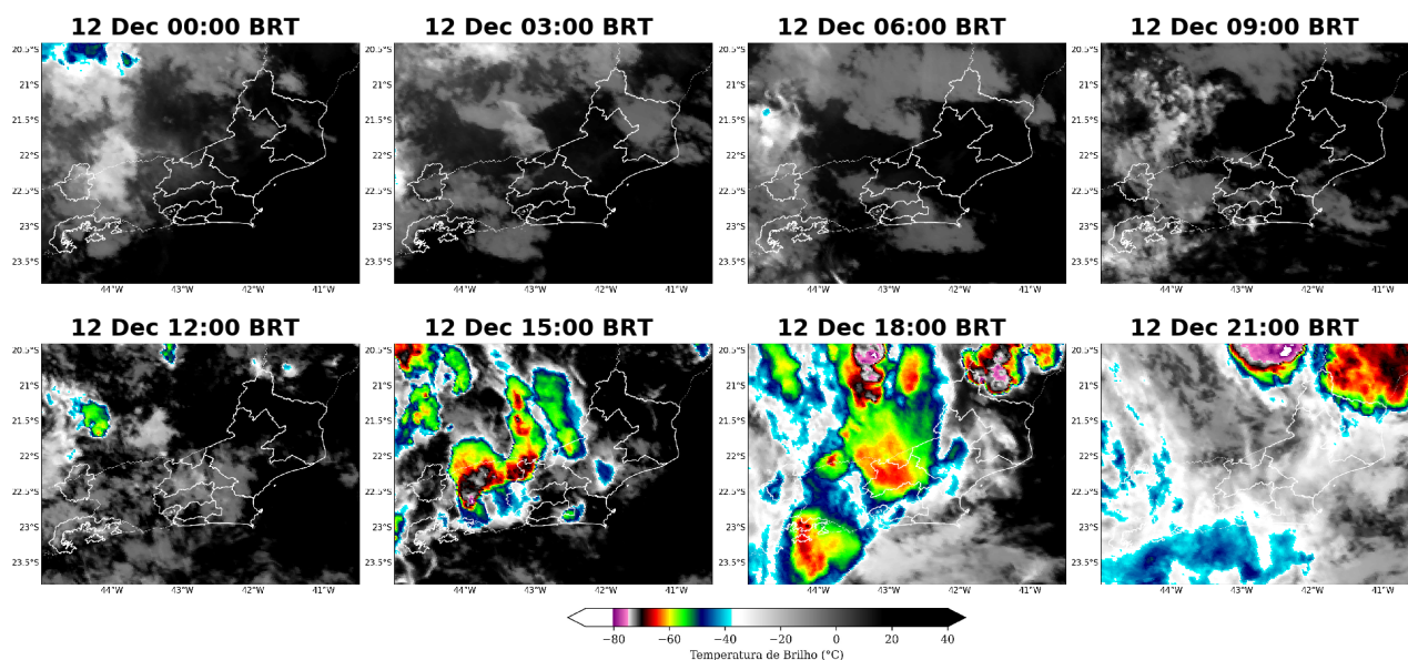
Figura 4: Imagens realçadas do satélite GOES-16 das 00 BRT até 21 BRT (a cada 3 horas) para o dia 12 de dezembro.
