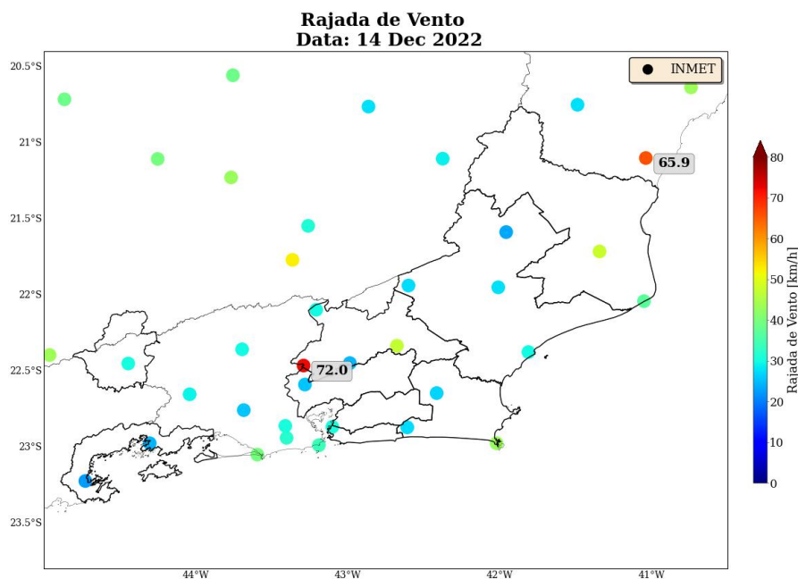
Figura 22: Máxima rajada de vento diária sobre a área de concessão da Enel-RJ para o dia 14 de dezembro, baseado nas estações meteorológicas do INMET.
