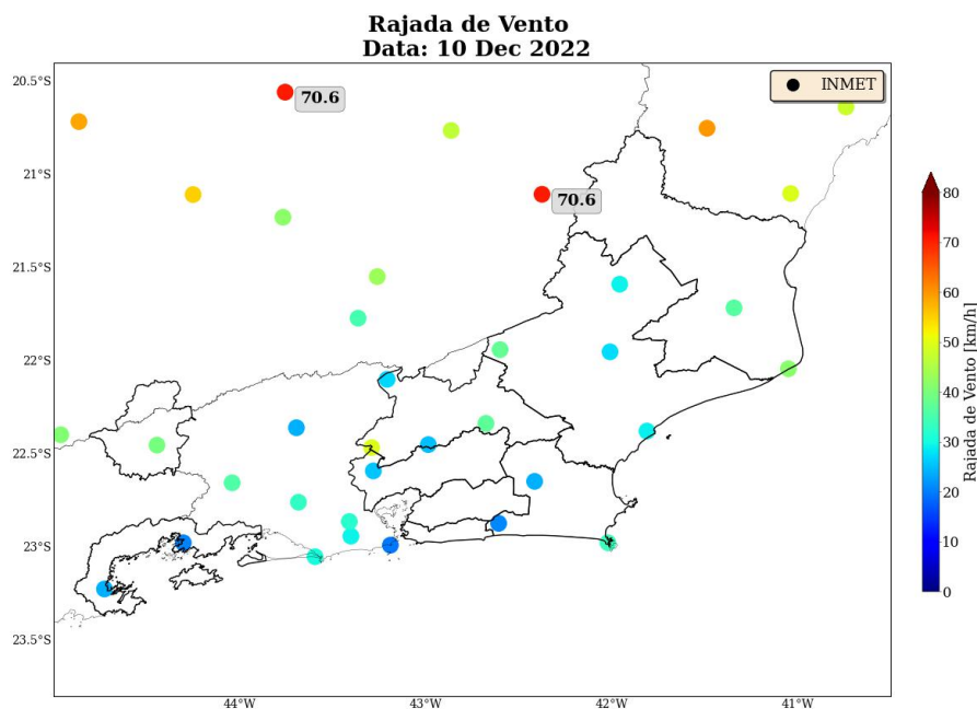
Figura 18: Máxima rajada de vento diária sobre a área de concessão da Enel-RJ para o dia 10 de dezembro, baseado nas estações meteorológicas do INMET.
