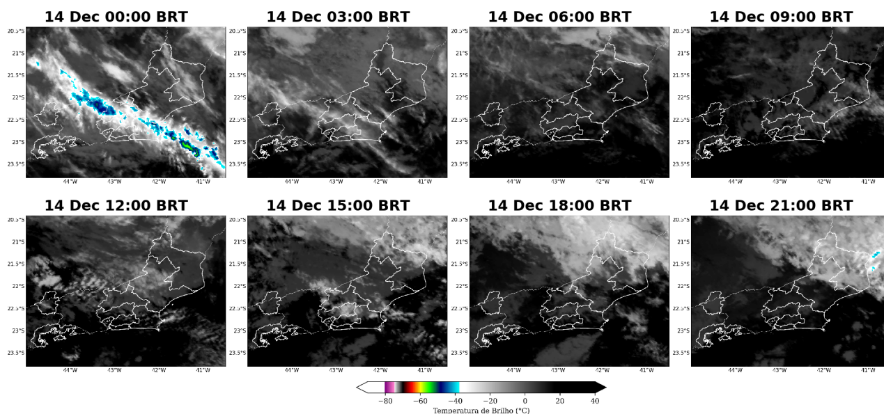
Figura 6: Imagens realçadas do satélite GOES-16 das 00 BRT até 21 BRT (a cada 3 horas) para o dia 14 de dezembro.
