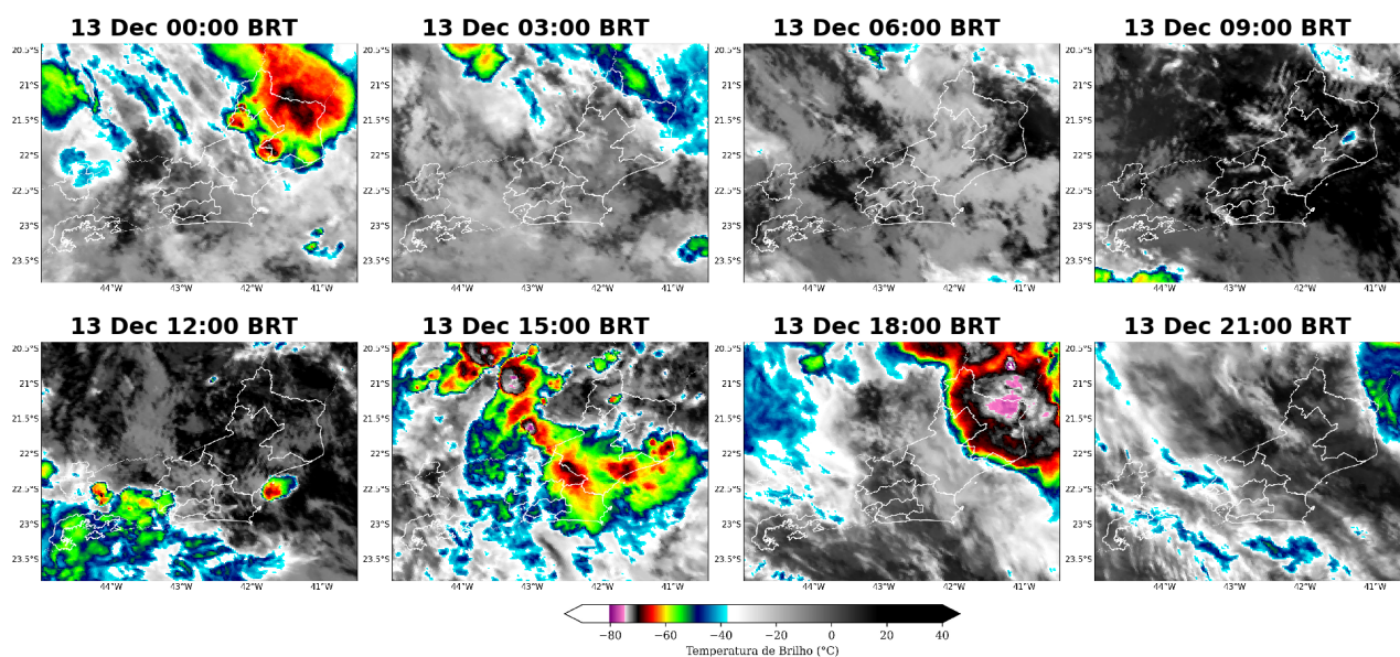
Figura 5: Imagens realçadas do satélite GOES-16 das 00 BRT até 21 BRT (a cada 3 horas) para o dia 13 de dezembro.
