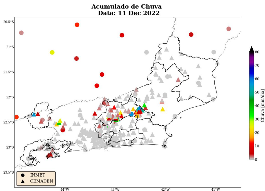
Figura 13: Acumulado diário de precipitação sobre a área de concessão da Enel-RJ para o dia 11 de dezembro, baseado nas estações meteorológicas do INMET e CEMADEN.
