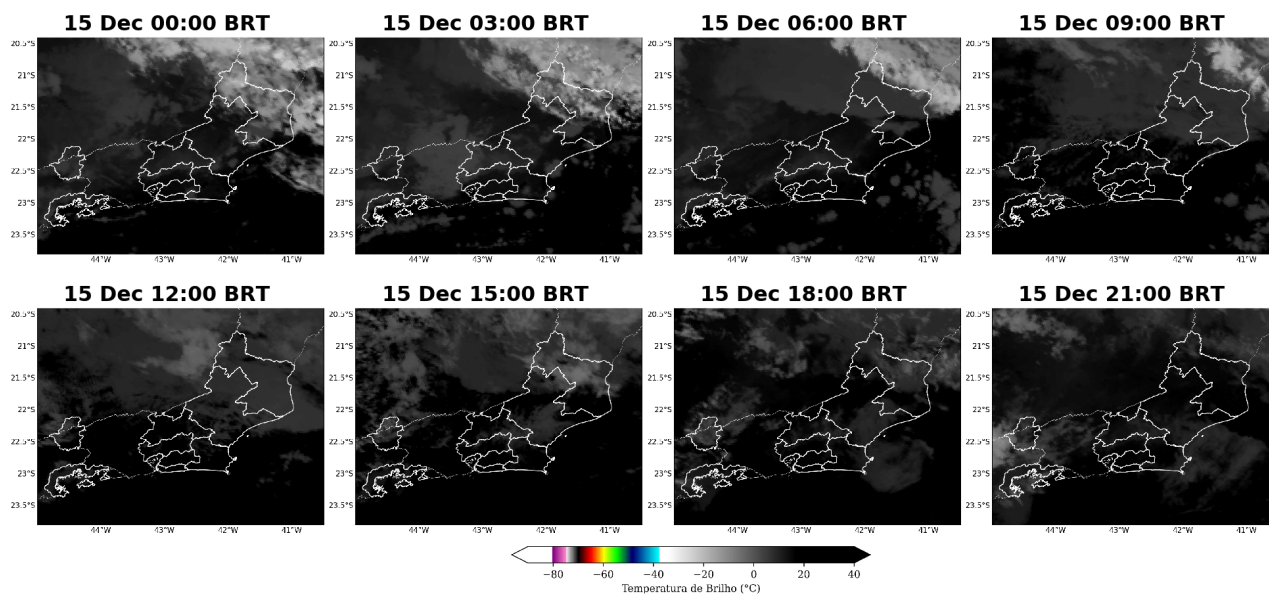
Figura 7: Imagens realçadas do satélite GOES-16 das 00 BRT até 21 BRT (a cada 3 horas) para o dia 15 de dezembro.
