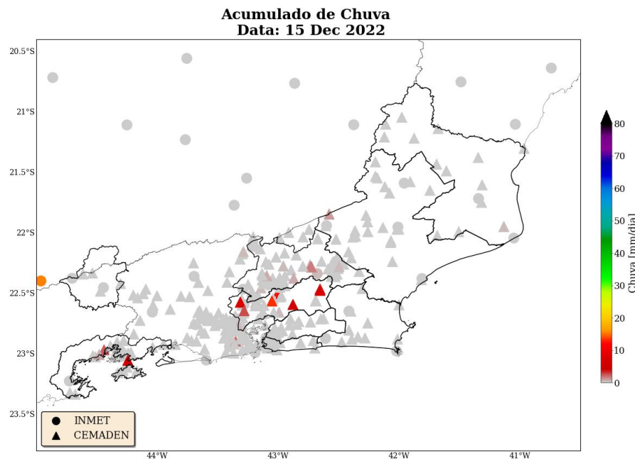
Figura 17: Acumulado diário de precipitação sobre a área de concessão da Enel-RJ para o dia 15 de dezembro, baseado nas estações meteorológicas do INMET e CEMADEN.
