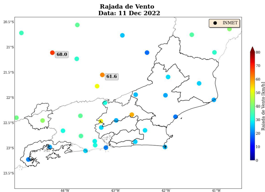
Figura 19: Máxima rajada de vento diária sobre a área de concessão da Enel-RJ para o dia 11 de dezembro, baseado nas estações meteorológicas do INMET.
