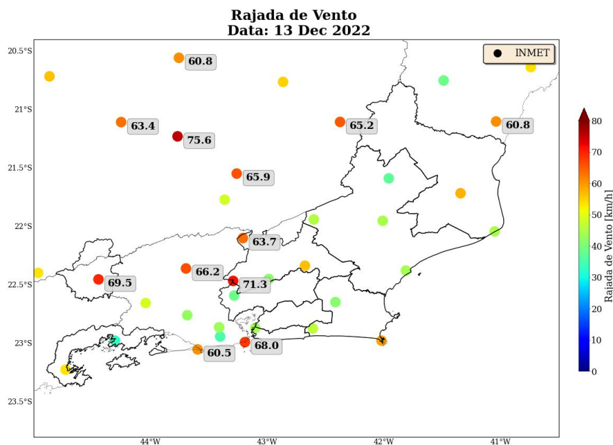
Figura 21: Máxima rajada de vento diária sobre a área de concessão da Enel-RJ para o dia 13 de dezembro, baseado nas estações meteorológicas do INMET.
