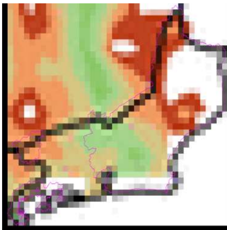
Figura 2 - Mapa de incidência de descargas atmosféricas nuvem-solo e intranuvem nos dias: (a) 14/02; (b) 15/02; (c) 16/02; e (d) 17/02. Cada ponto preto corresponde ao local de ocorrência de uma descarga.
