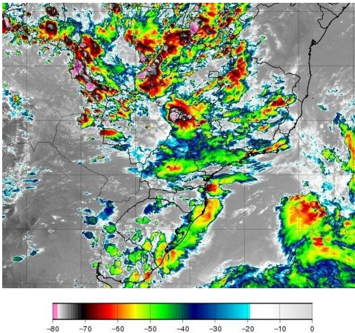
Figura 1 - Imagem de satélite no infravermelho com realce do satélite GOES-16 às 20:00 UT do dia 14/02/2021. As cores indicam diferentes temperaturas dos topos das nuvens.
