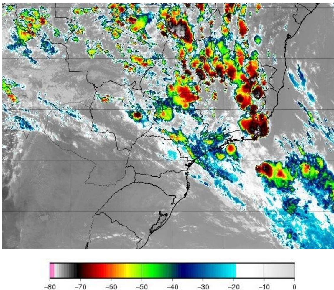
Figura 1 - Imagem de satélite no infravermelho com realce do satélite GOES-16 às 20:00 UT do dia 28/02. As cores indicam diferentes temperaturas dos topos das nuvens.
