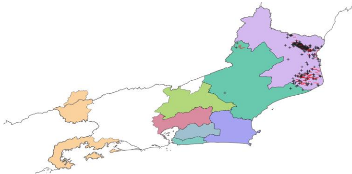
Figura - Descargas atmosféricas registradas pelo sistema de detecção da EarthNetworks entre 12h30 e 16h50 do dia 01 de março de 2020
