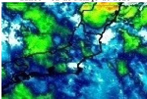
Figura 5 – Imagens realçadas do satélite GOES-16 das 21h00 do dia 01 de Março de 2020. FONTE: Cptec/INPE.
