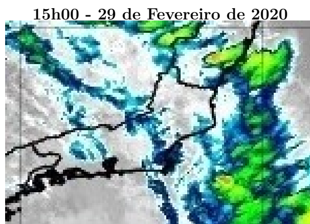
Figura 3 – Imagens realçadas do satélite GOES-16 das 15h00 do dia 29 de Fevereiro de 2020. FONTE: Cptec/INPE.
