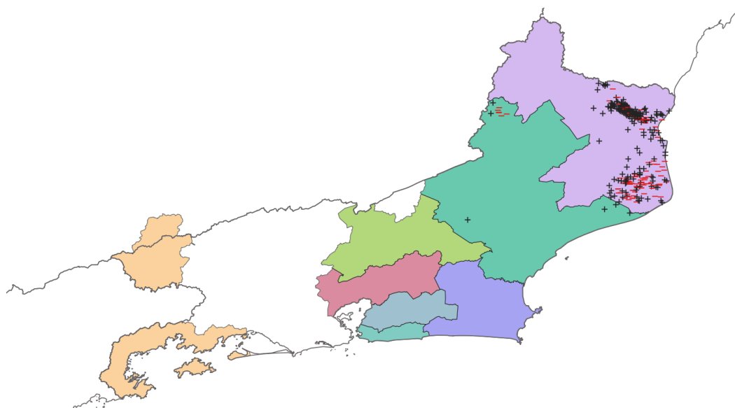
Figura 2 – Descargas atmosféricas registradas pelo sistema de detecção da EarthNetworks entre 12h30 e 16h50 do dia 01 de março de 2020.
