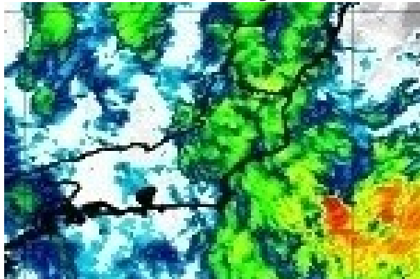
Figura 8 – Imagens realçadas do satélite GOES-16 das 15h00 do dia 02 de Março de 2020. FONTE: Cptec/INPE.
