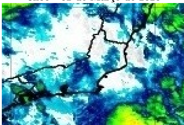
Figura 6 – Imagens realçadas do satélite GOES-16 das 3h00 do dia 02 de Março de 2020. FONTE: Cptec/INPE.
