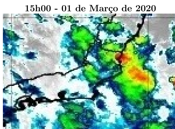
Figura 4 – Imagens realçadas do satélite GOES-16 das 15h00 do dia 01 de Março de 2020. FONTE: Cptec/INPE.
