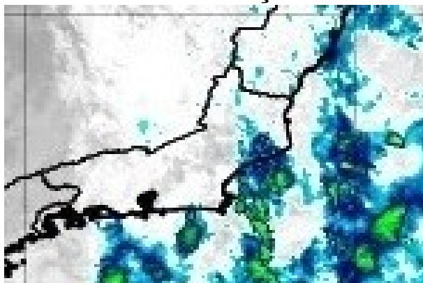
Figura 9 – Imagens realçadas do satélite GOES-16 das 21h00 do dia 02 de Março de 2020. FONTE: Cptec/INPE.
