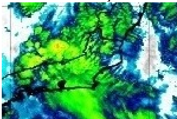
Figura 7 – Imagens realçadas do satélite GOES-16 das 9h00 do dia 02 de Março de 2020. FONTE: Cptec/INPE.
