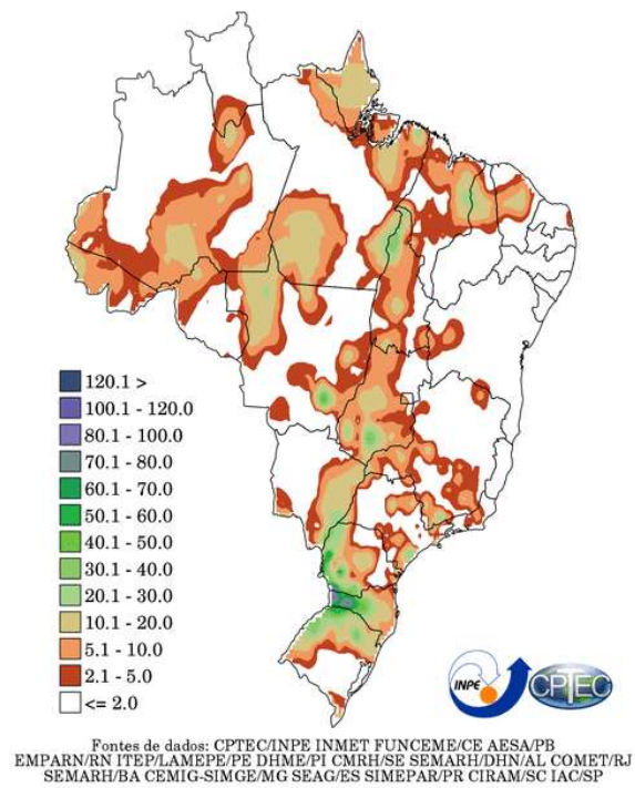
Precipitacao Observada (mm) - 30/01/2020
