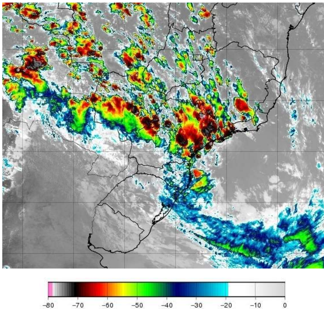
Figura 1 - Imagem de satélite no infravermelho com realce do satélite GOES-16 às 20:00 UT do dia 30/01. As cores indicam diferentes temperaturas dos topos das nuvens.
