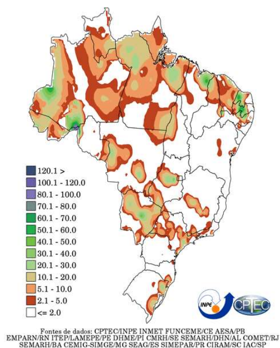
Precipitacao Observada (mm) - 01/02/2020
