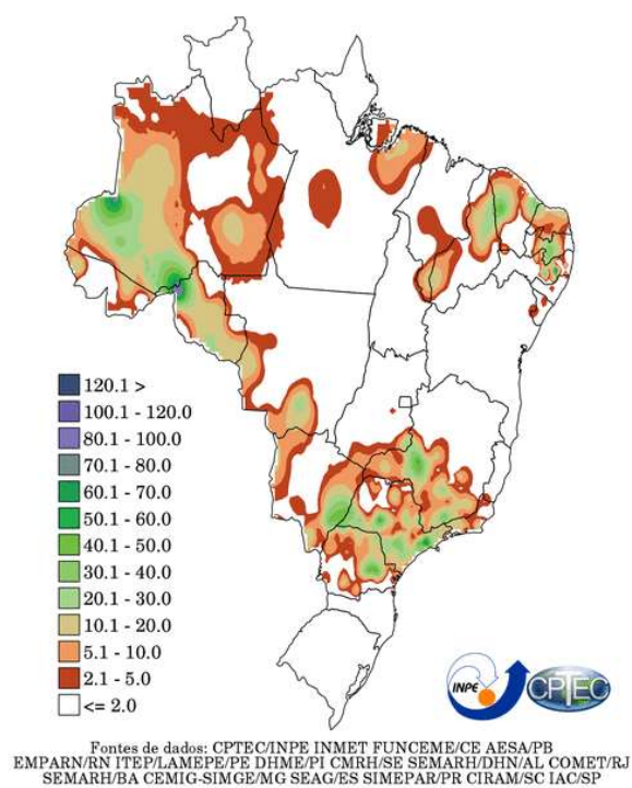
Precipitacao Observada (mm) - 02/02/2020
