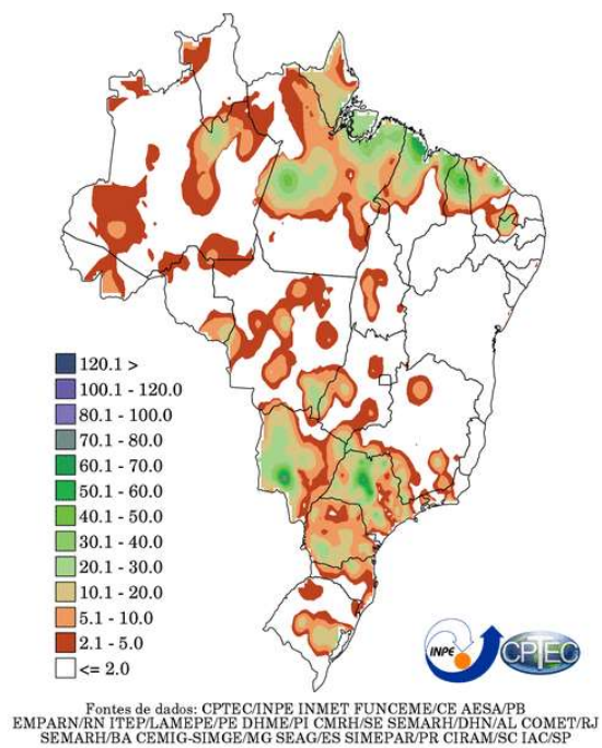
Precipitacao Observada (mm) - 31/01/2020
