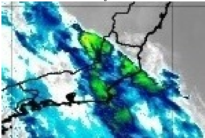
Figura 4 – Imagens realçadas do satélite GOES-16 das 17h00 e 19h00 do dia 03 de junho de 2019. FONTE: Cptec/INPE.
