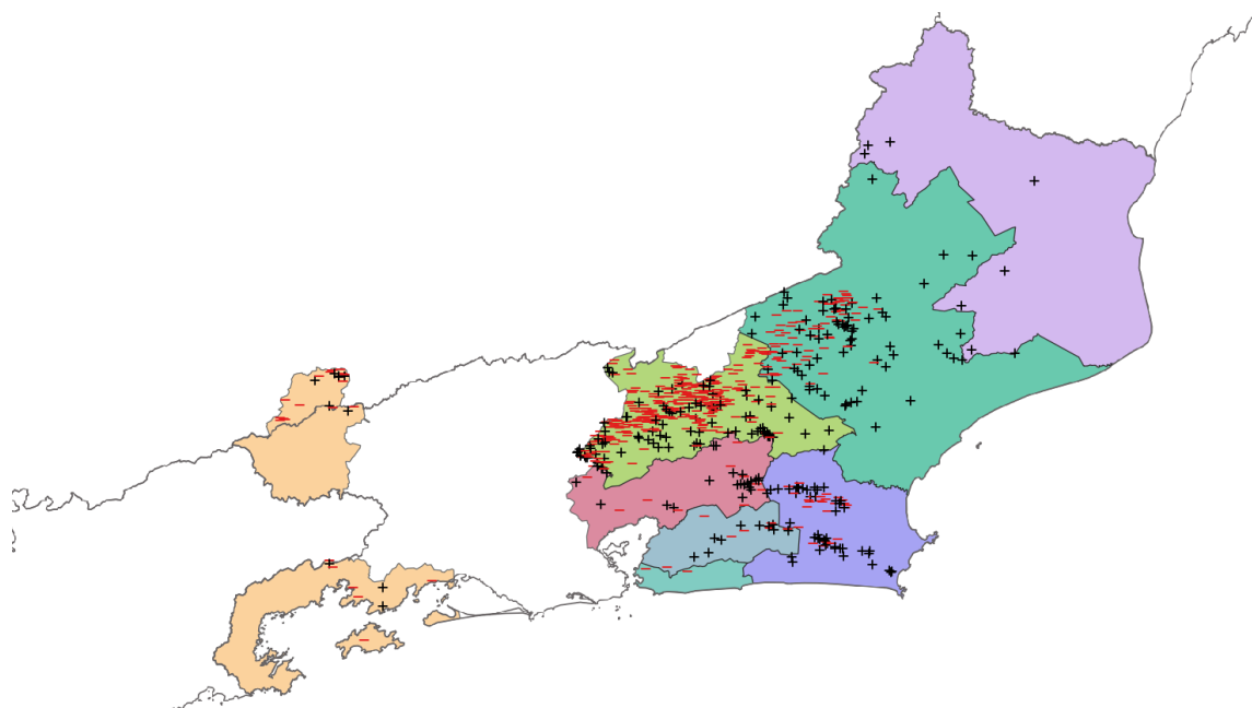
Figura 2 – Descargas atmosféricas nuvem-solo (raios) detectadas pelo sistema Earth Networks entre as 12h20 e 20h10 do dia 03 de junho de 2019.
