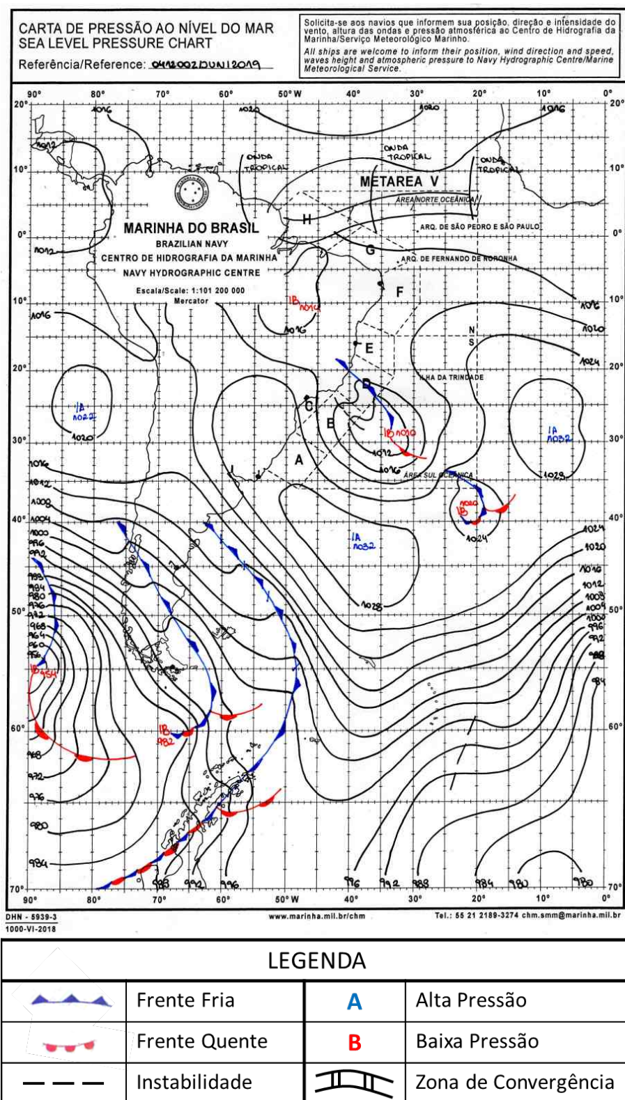
Figura A3 - Carta sinótica da Marinha do Brasil para as 1200Z do dia 04 de junho de 2019 (09h00 do dia 04 de junho de 2019, hora local).
