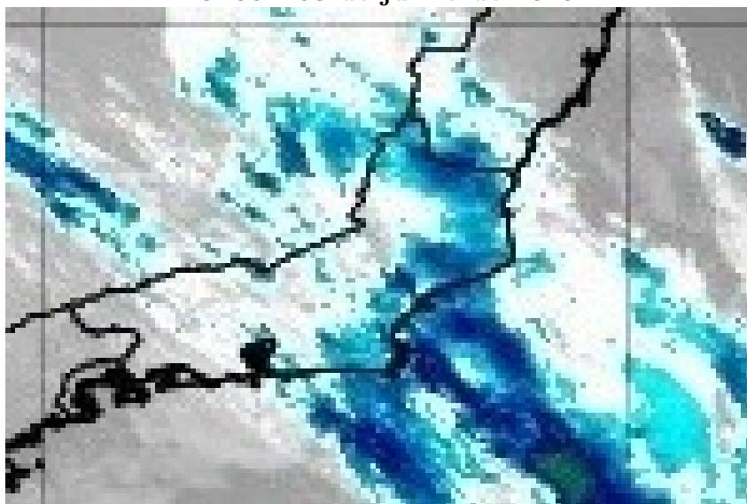
Figura 5 – Imagens realçadas do satélite GOES-16 das 21h00 e 23h00 do dia 03 de junho de 2019. FONTE: Cptec/INPE.
