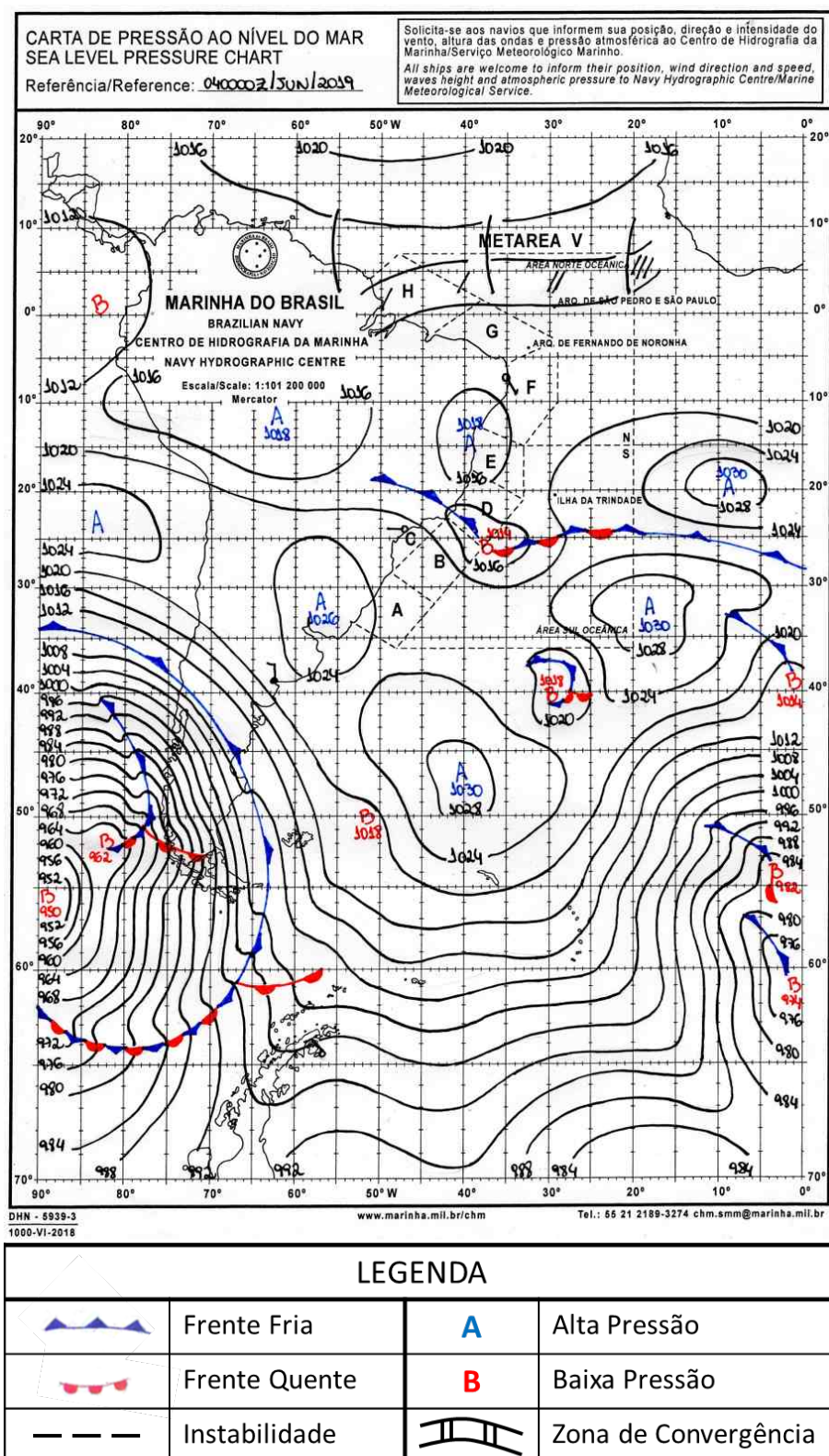
Figura A2 - Carta sinótica da Marinha do Brasil para as 0000Z do dia 04 de junho de 2019 (21h00 do dia 03 de junho de 2019, hora local).
