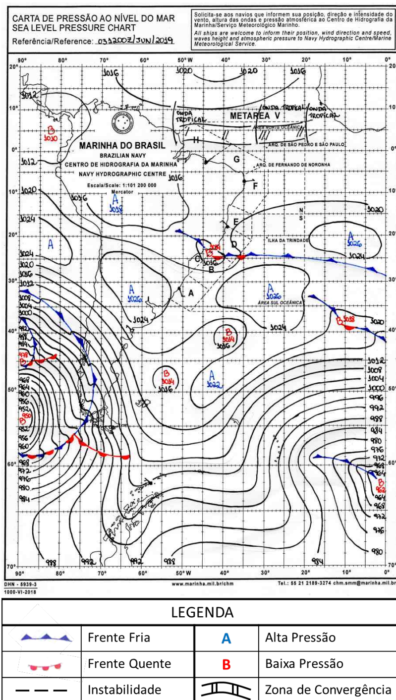
Figura A1 - Carta sinótica da Marinha do Brasil para as 1200Z do dia 03 de junho de 2019 (09h00 do dia 03 de junho de 2019, hora local).
