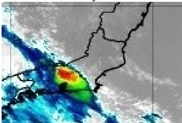
Figura 3 – Imagens realçadas do satélite GOES-16 das 13h00 e 15h00 do dia 03 de junho de 2019. FONTE: Cptec/INPE.
