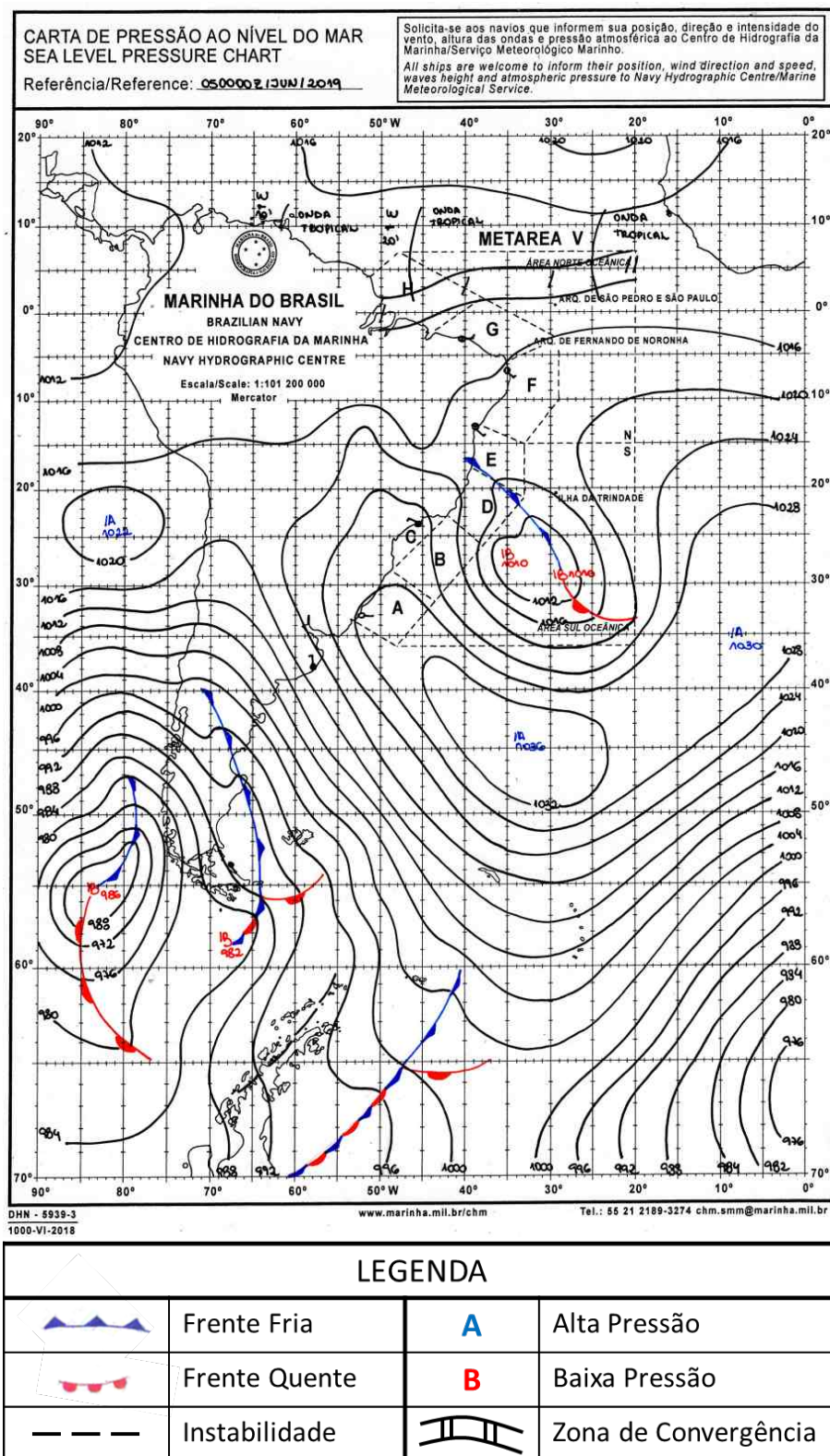
Figura A4 - Carta sinótica da Marinha do Brasil para as 0000Z do dia 05 de junho de 2019 (21h00 do dia 05 de junho de 2019, hora local).
