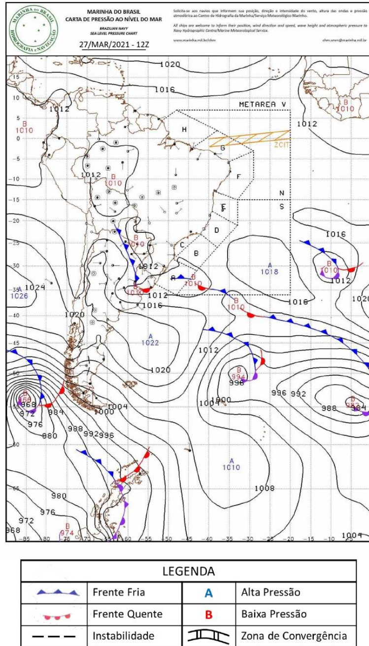
Figura A4 - Carta sinótica da Marinha do Brasil para as 1200Z do dia 27 de março de 2021 (09h00 do dia 27 de março de 2021, hora local. FONTE: Marinha do Brasil).
