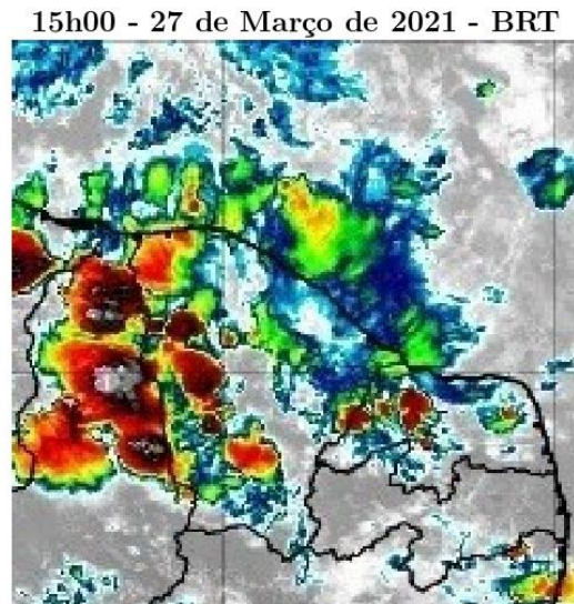
Figura 26 – Imagens realçadas do satélite GOES-16 das 15h00 do dia 27 de Março de 2021. FONTE: Cptec/INPE.
