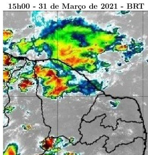
Figura 47 – Imagens realçadas do satélite GOES-16 das 15h00 do dia 31 de Março de 2021. FONTE: Cptec/INPE.
