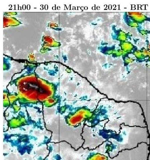
Figura 43 – Imagens realçadas do satélite GOES-16 das 21h00 do dia 30 de Março de 2021. FONTE: Cptec/INPE.
