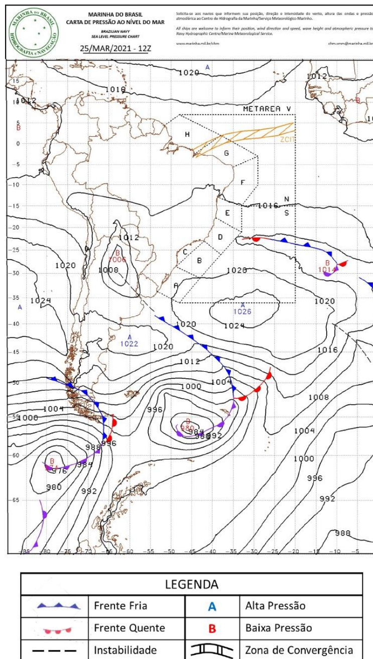
Figura A2 - Carta sinótica da Marinha do Brasil para as 1200Z do dia 25 de março de 2021 (09h00 do dia 25 de março de 2021, hora local. FONTE: Marinha do Brasil).
