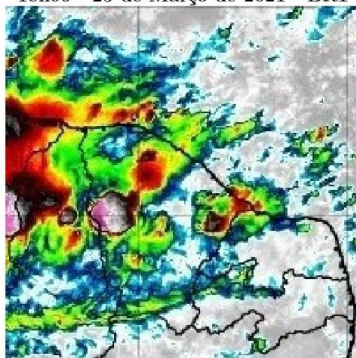
Figura 11 – Imagens realçadas do satélite GOES-16 das 18h00 do dia 25 de Março de 2021. FONTE: Cptec/INPE.
