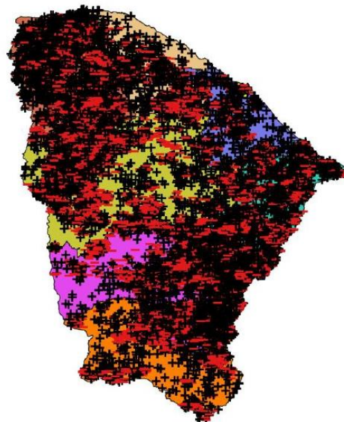
Figura 2 – Descargas atmosféricas nuvem-solo (em preto) e nuvem-nuvem (em vermelho) detectadas pelo sistema Earth Networks entre as 09h30 do dia 24 e 17h40 do dia 31 de março de 2021 sobre a área de concessão da ENEL Ceará.
