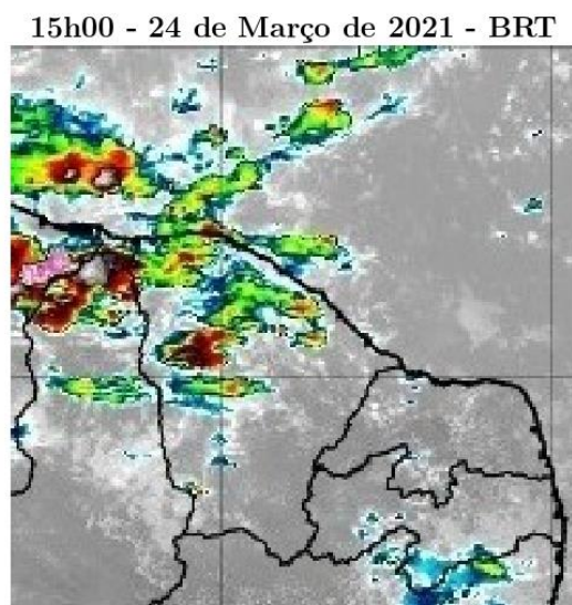
Figura 4 – Imagens realçadas do satélite GOES-16 das 15h00 do dia 24 de Março de 2021. FONTE: Cptec/INPE.
