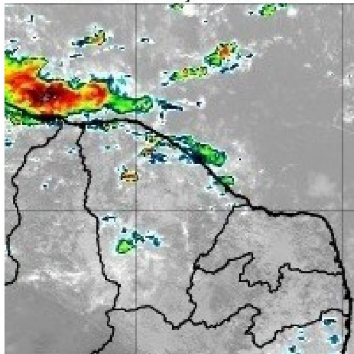
Figura 3 – Imagens realçadas do satélite GOES-16 das 12h00 do dia 24 de Março de 2021. FONTE: Cptec/INPE.
