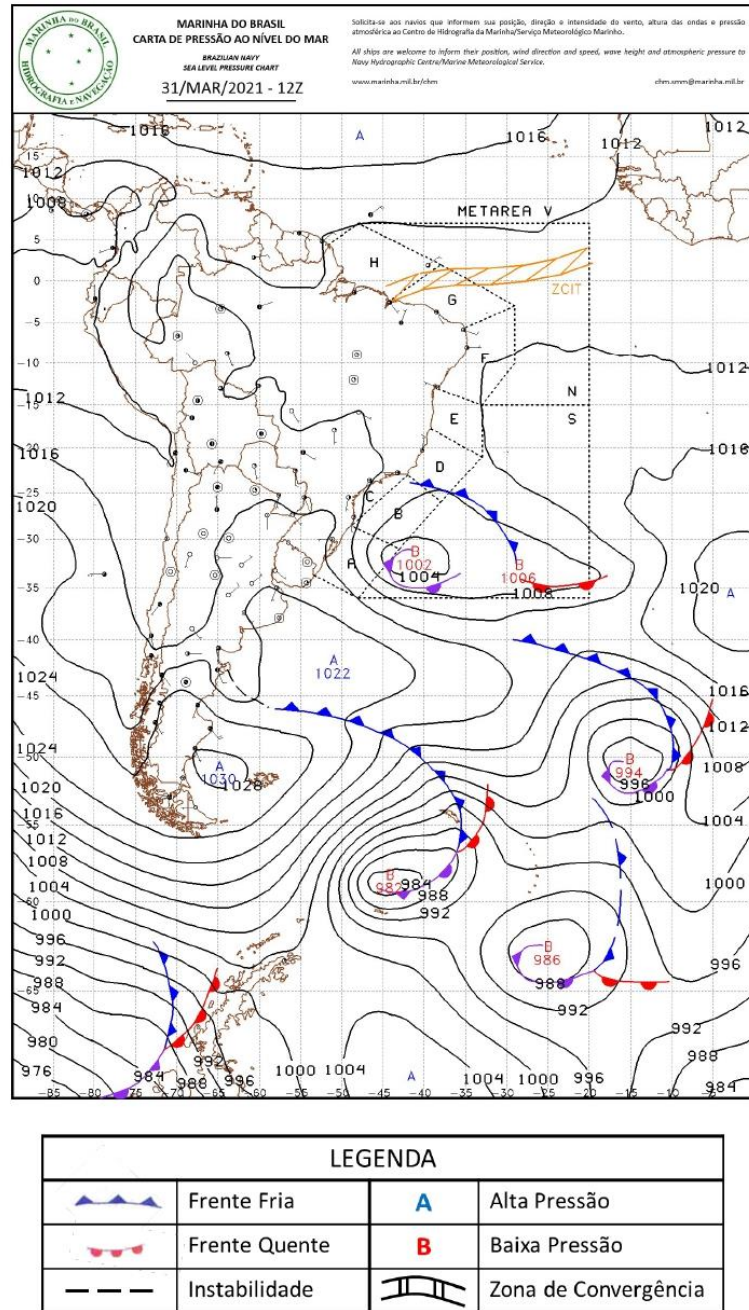
Figura A8 - Carta sinótica da Marinha do Brasil para as 1200Z do dia 31 de março de 2021 (09h00 do dia 31 de março de 2021, hora local. FONTE: Marinha do Brasil).
