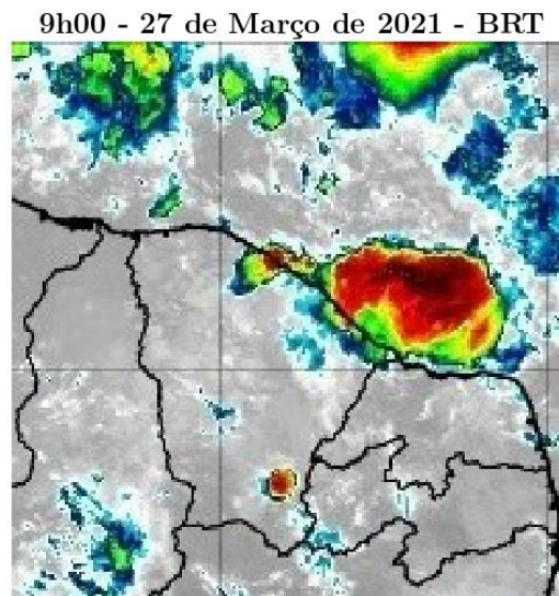
Figura 24 – Imagens realçadas do satélite GOES-16 das 9h00 do dia 27 de Março de 2021. FONTE: Cptec/INPE.
