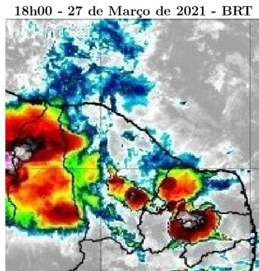
Figura 27 – Imagens realçadas do satélite GOES-16 das 18h00 do dia 27 de Março de 2021. FONTE: Cptec/INPE.
