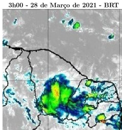
Figura 30 – Imagens realçadas do satélite GOES-16 das 3h00 do dia 28 de Março de 2021. FONTE: Cptec/INPE.
