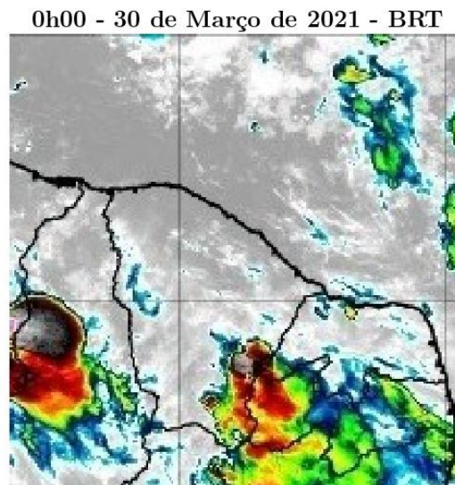
Figura 38 – Imagens realçadas do satélite GOES-16 das 0h00 do dia 30 de Março de 2021. FONTE: Cptec/INPE.
