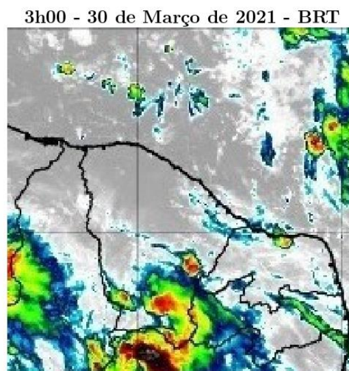
Figura 39 – Imagens realçadas do satélite GOES-16 das 3h00 do dia 30 de Março de 2021. FONTE: Cptec/INPE.
