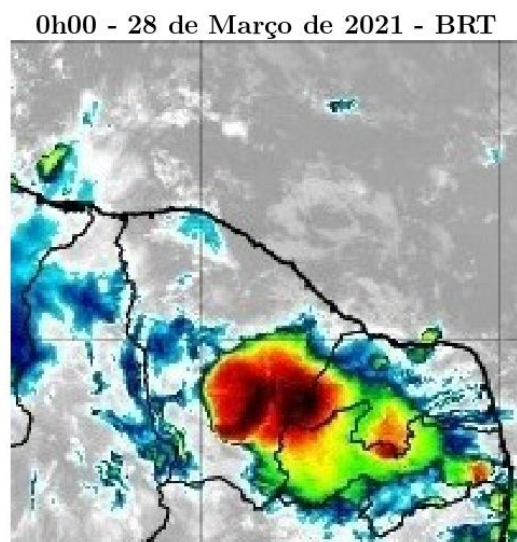
Figura 29 – Imagens realçadas do satélite GOES-16 das 0h00 do dia 28 de Março de 2021. FONTE: Cptec/INPE.
